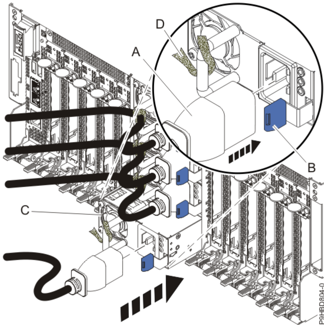
Figura 5. Sustitución de una fuente de alimentación
