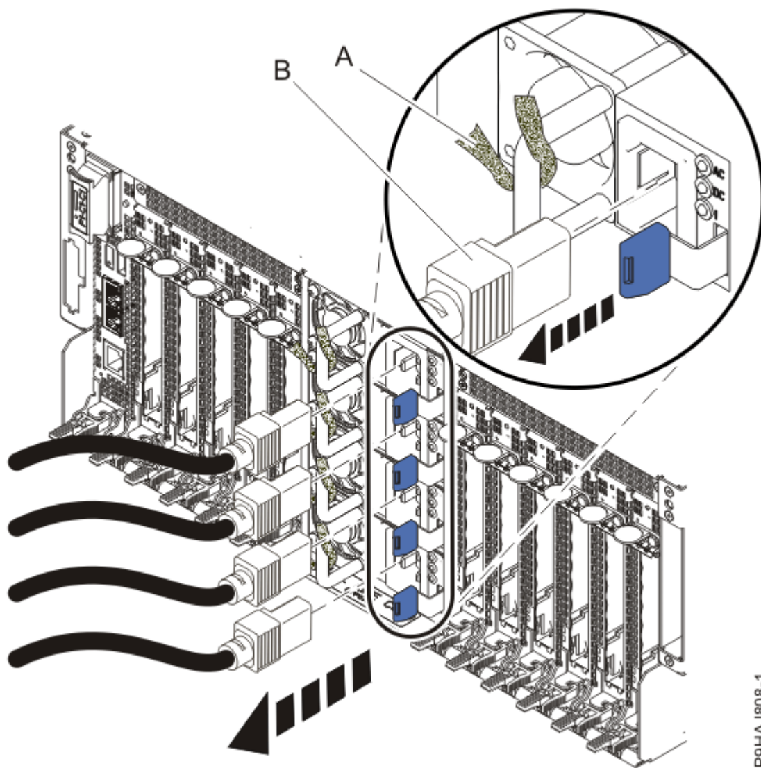
Figura 3. Extracción de los cables de alimentación
