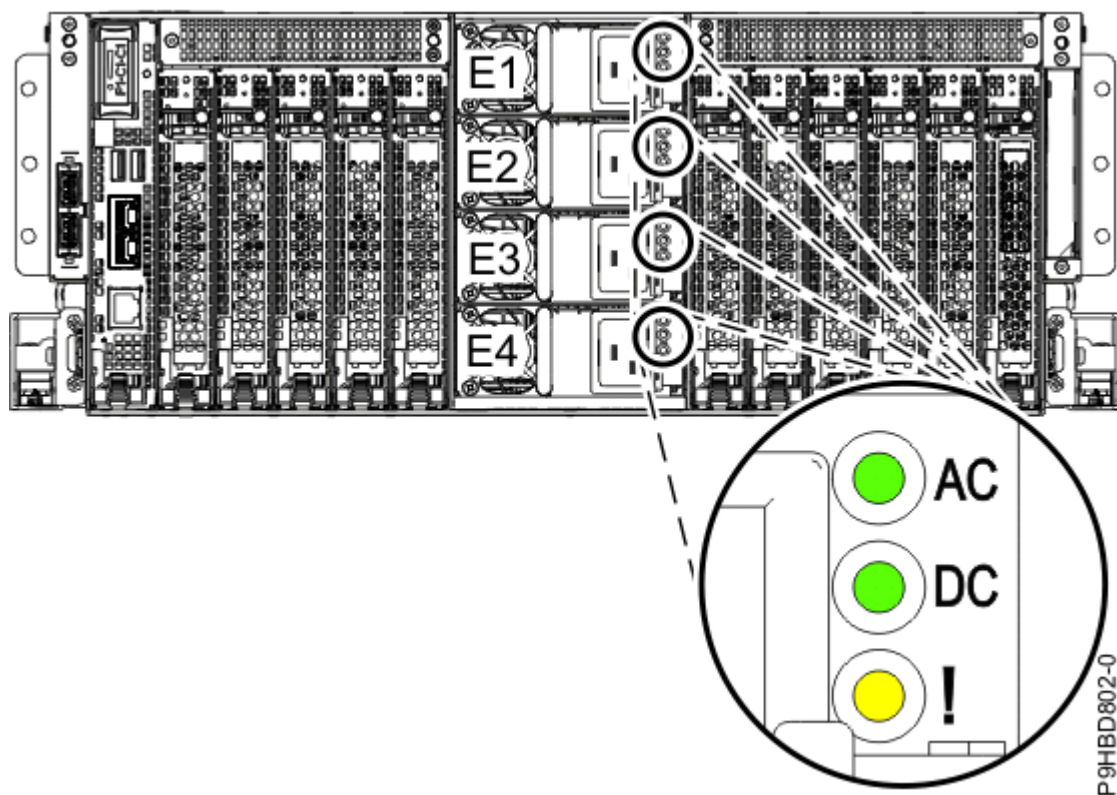
Figura 1. Ubicación de las fuentes de alimentación y LED
