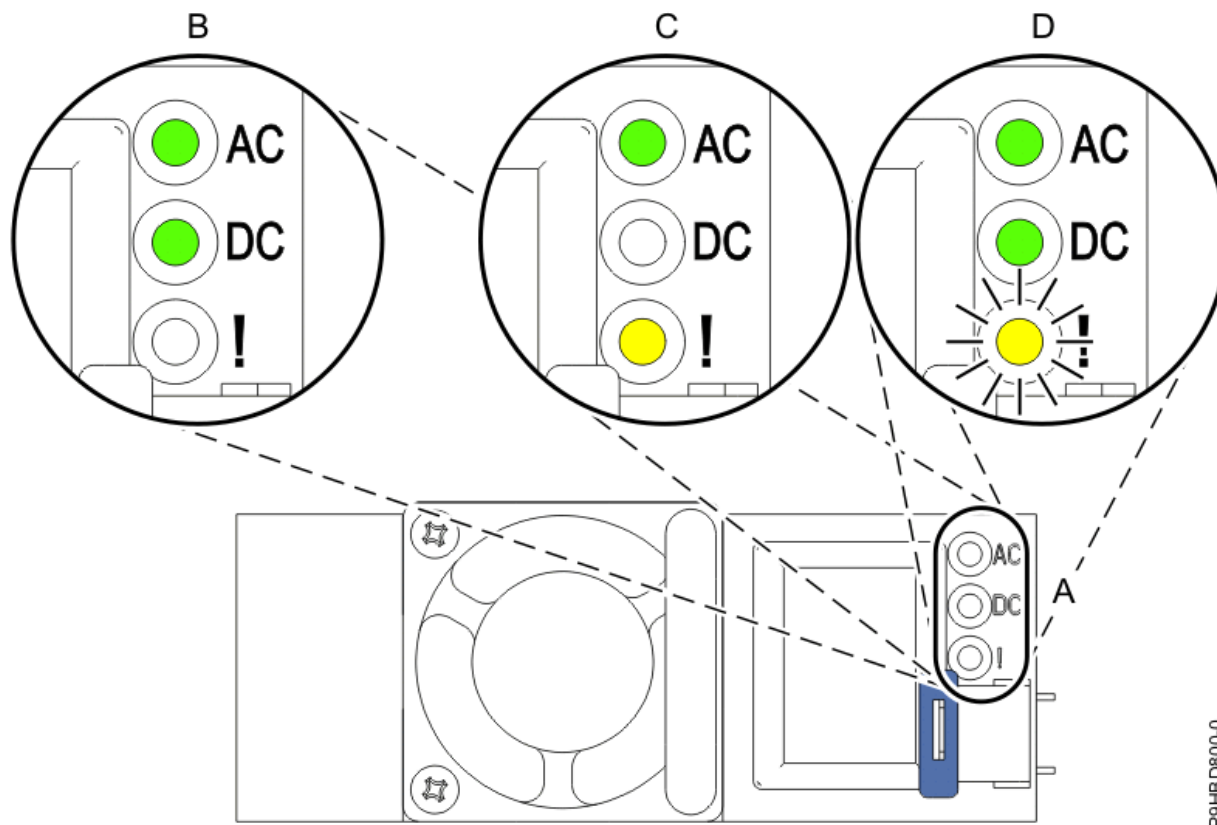
Figura 2. LED para una fuente de alimentación (B) en funcionamiento y (C, D) anómala en un sistema montado en bastidor
