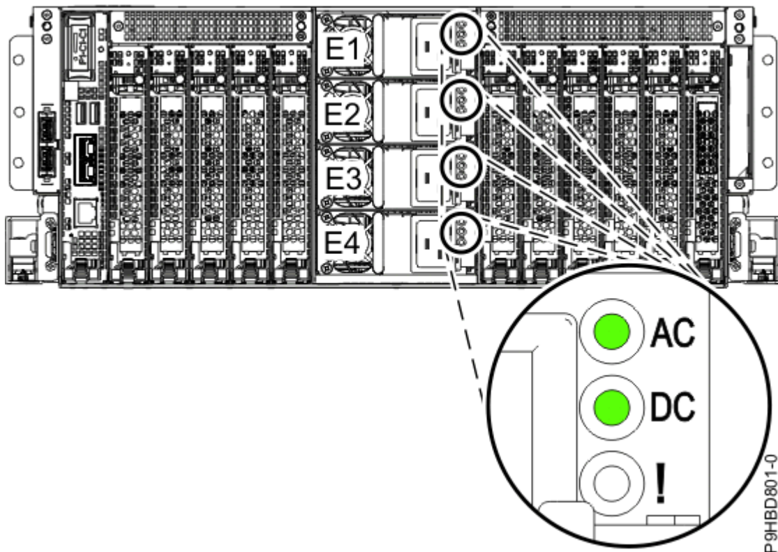
Figura 6. LED de una fuente de alimentación en funcionamiento
