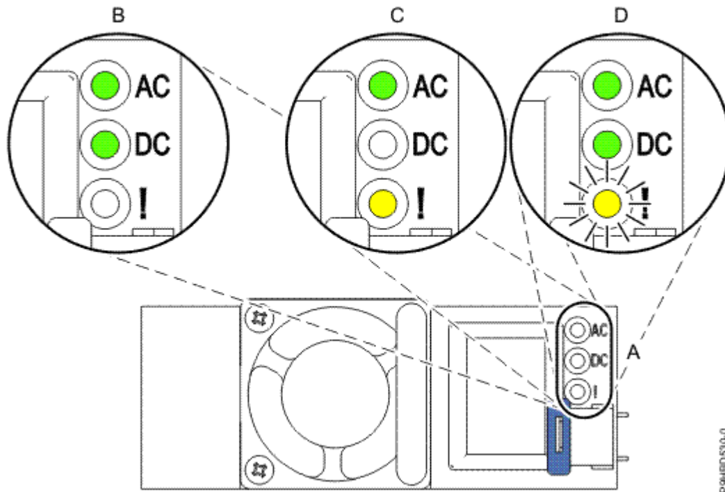
Figura 2. LED para una fuente de alimentación (B) en funcionamiento y (C, D) anómala
