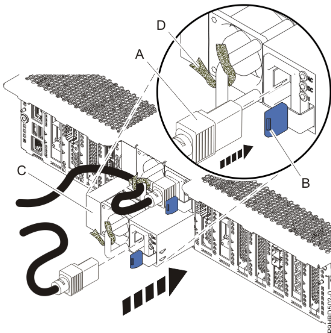
Figura 6. Sustitución de una fuente de alimentación
