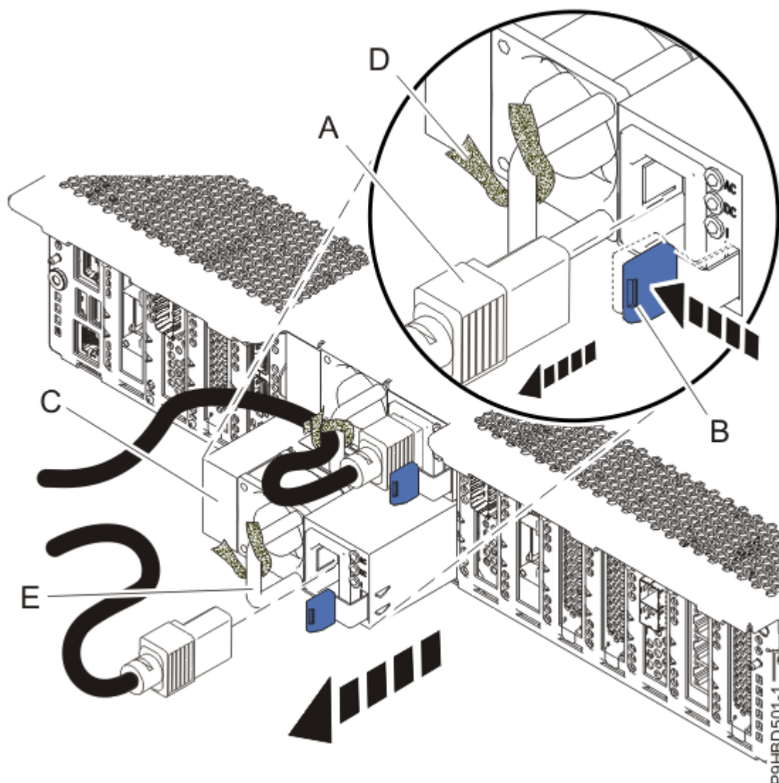
Figura 5. Extracción de una fuente de alimentación
