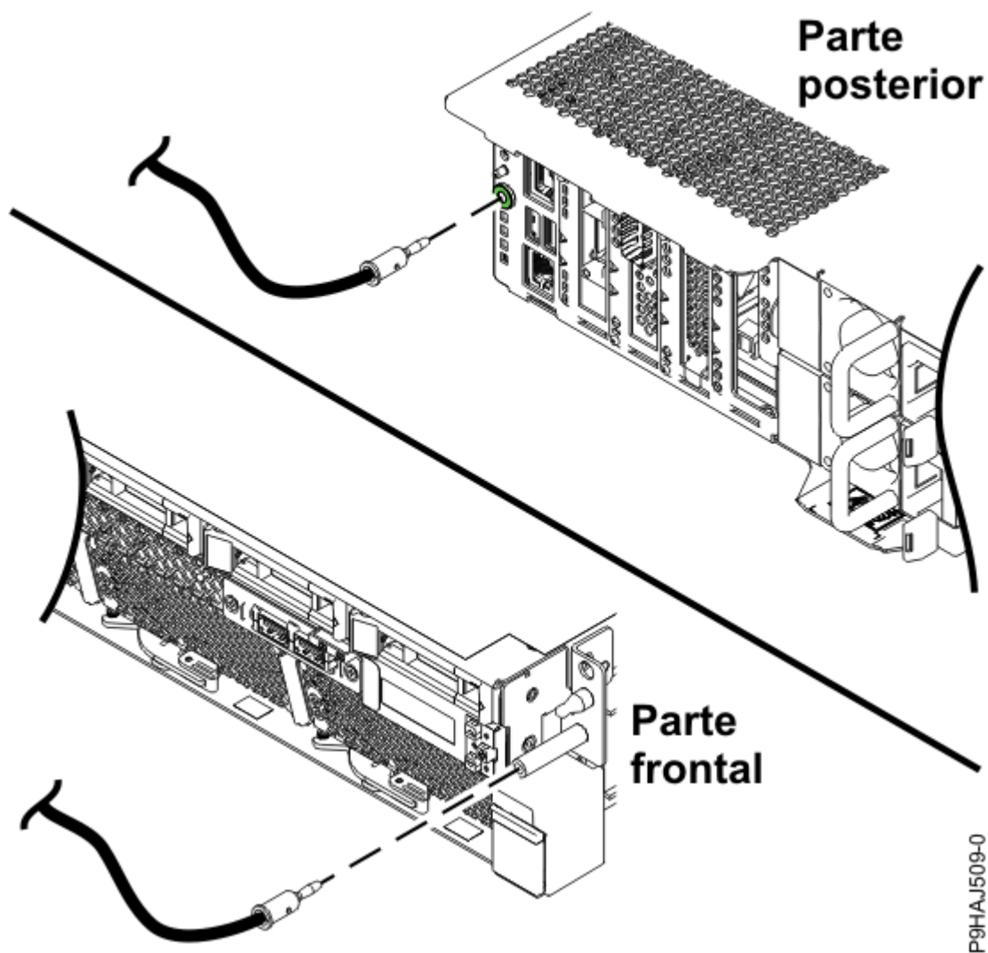
Figura 4. Ubicación de los enchufes ESD
