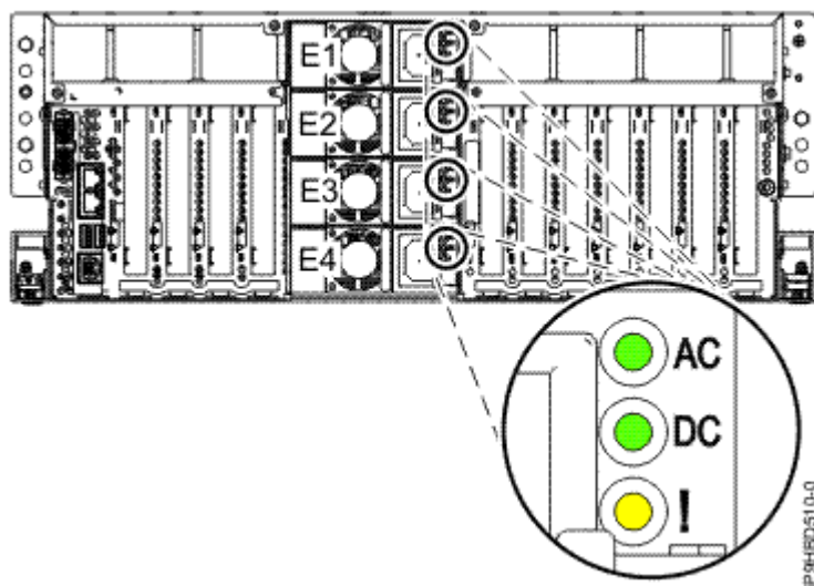
Figura 1. Ubicación de las fuentes de alimentación y LED en el sistema montado en bastidor
