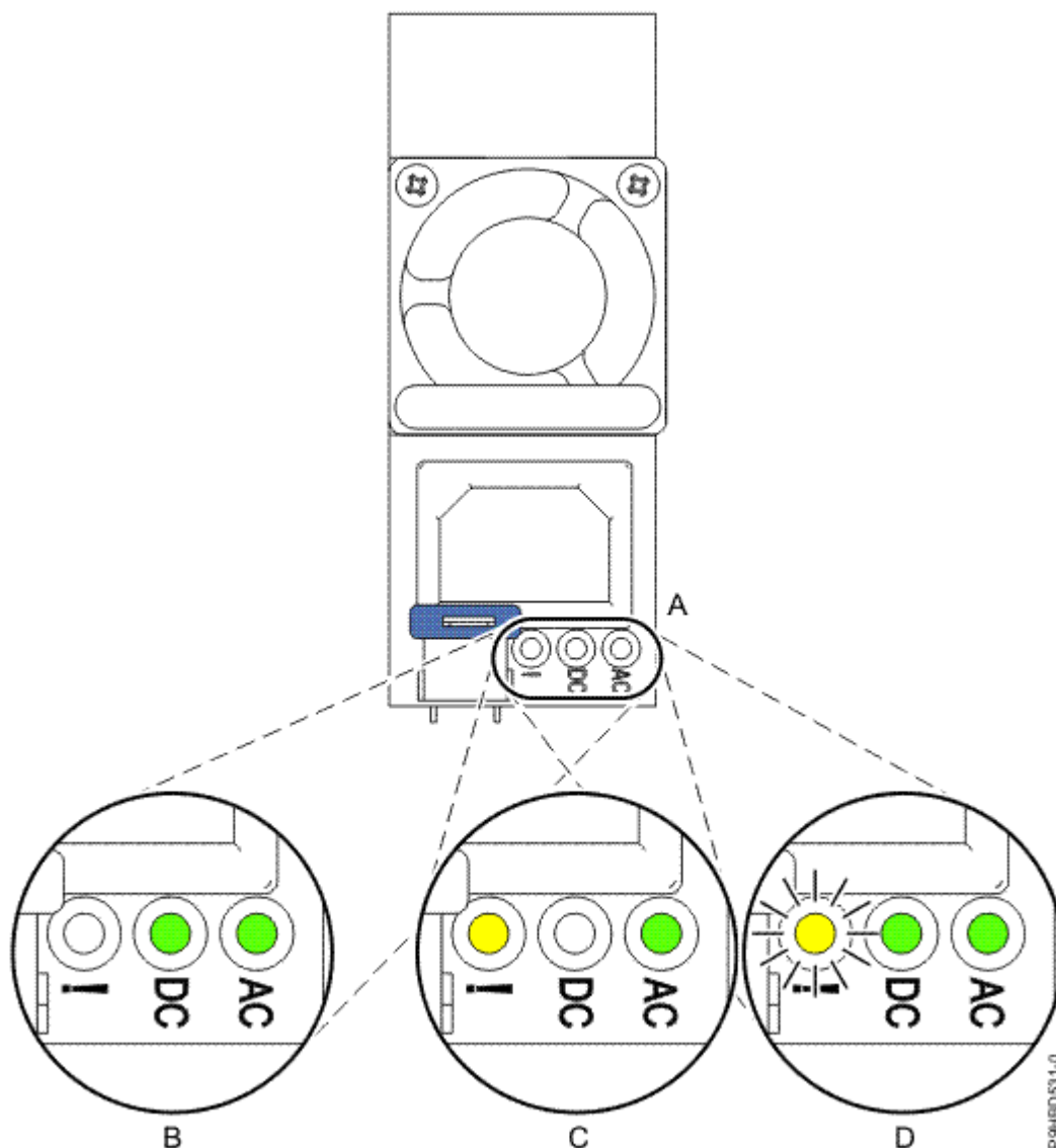
Figura 4. LED para una fuente de alimentación (B) en funcionamiento y (C, D) anómala en un sistema autónomo
