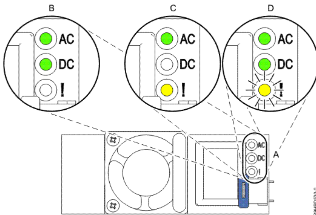
Figura 3. LED para una fuente de alimentación (B) en funcionamiento y (C, D) anómala en un sistema montado en bastidor
