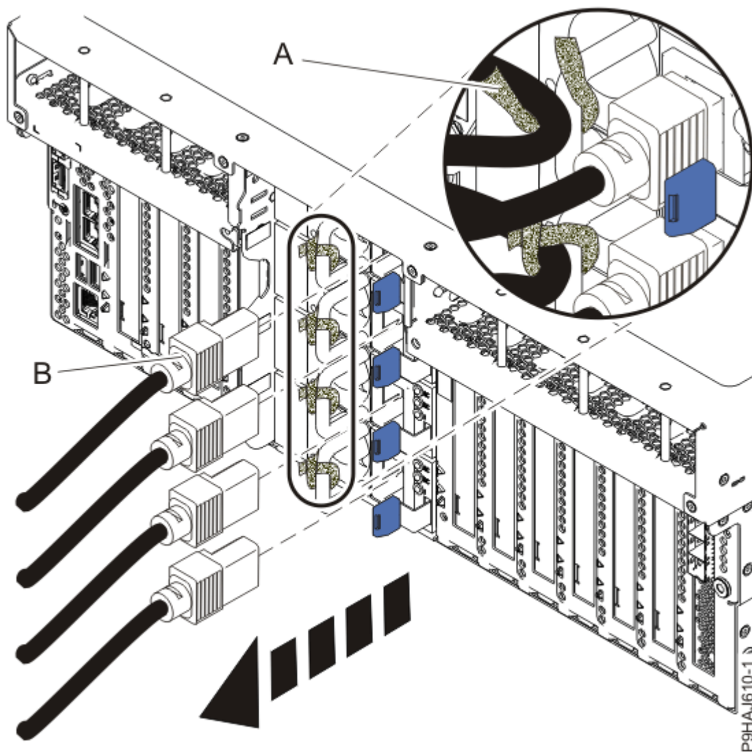
Figura 5. Extracción de los cables de alimentación de un servidor montado en bastidor
