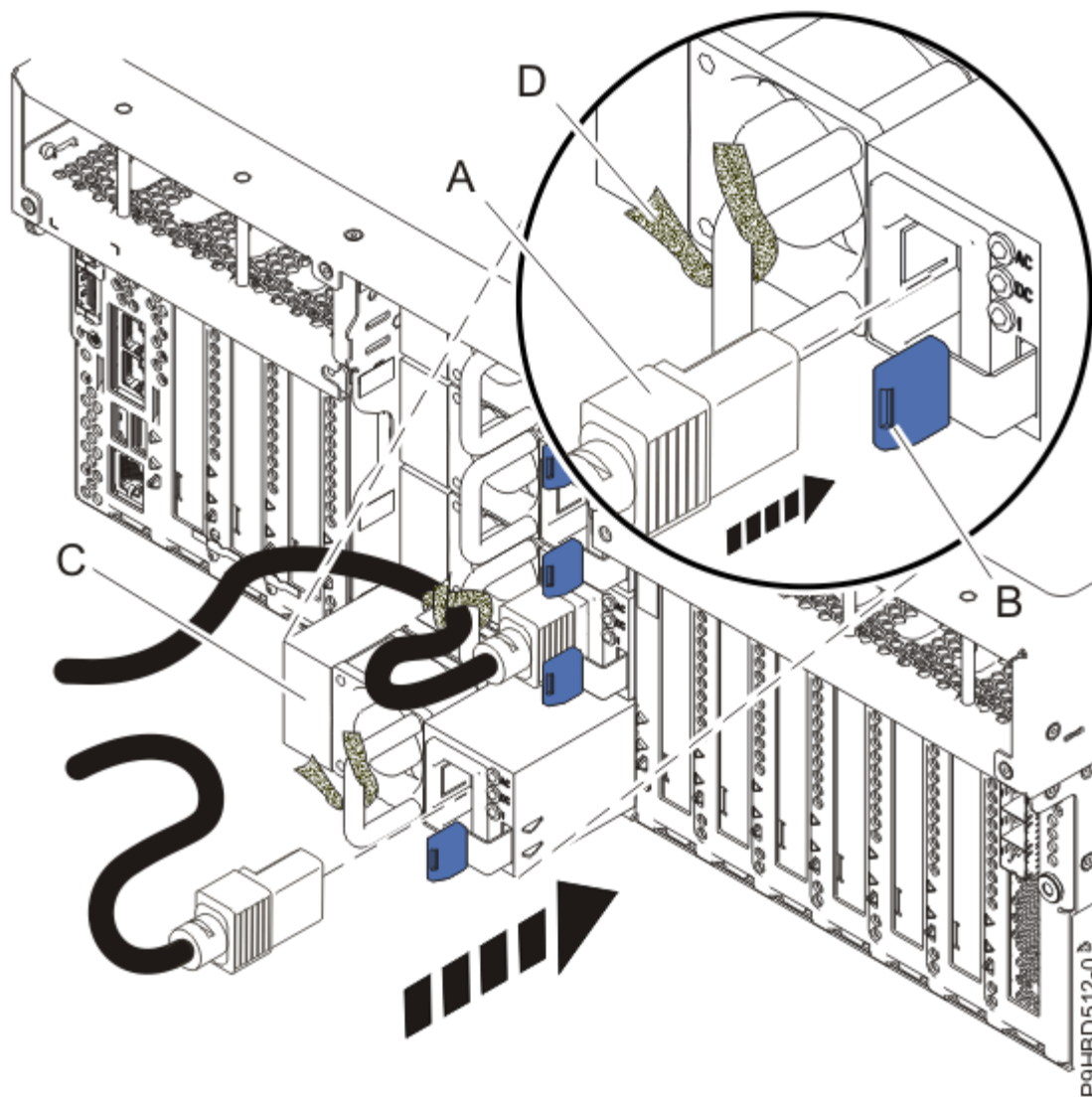
Figura 9. Sustitución de una fuente de alimentación
