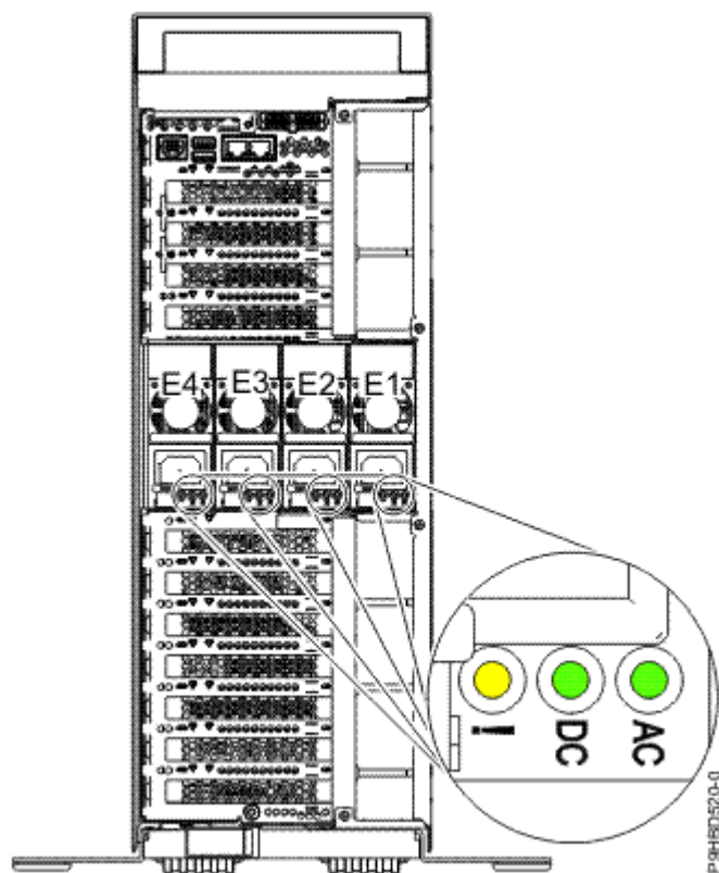
Figura 2. Ubicación de las fuentes de alimentación y LED en el sistema autónomo
