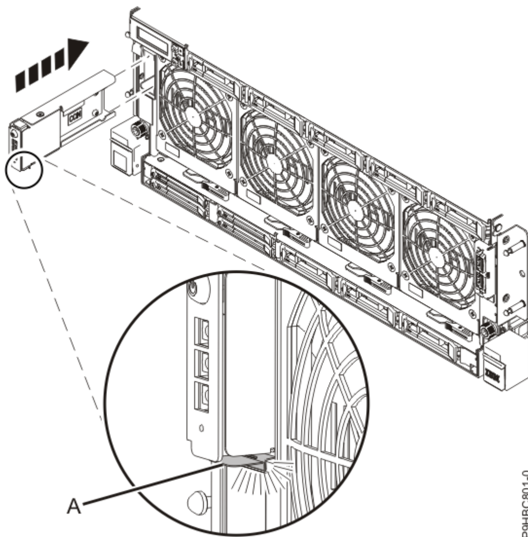
Figura 4. Instalación del panel de control
