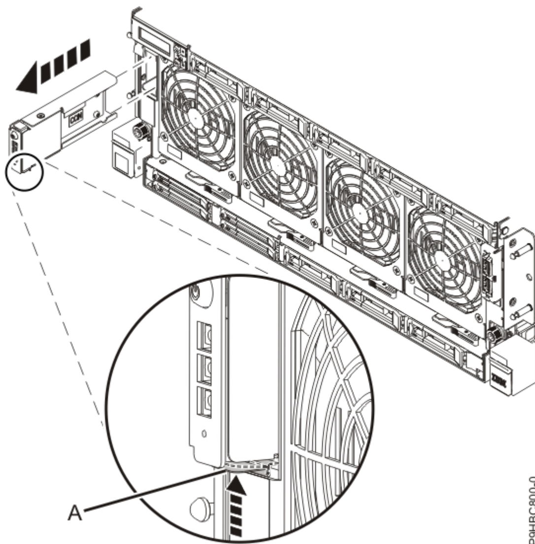
Figura 3. Cómo extraer el panel de control
