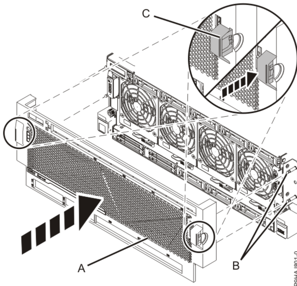
Figura 10. Instalación de la cubierta frontal
