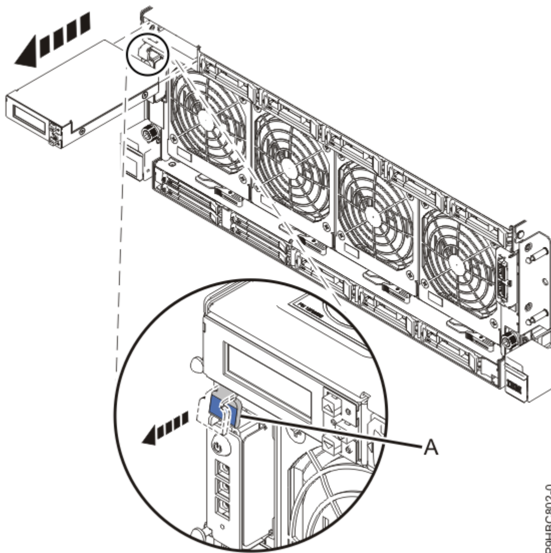
Figura 8. Extracción de la pantalla del panel de control
