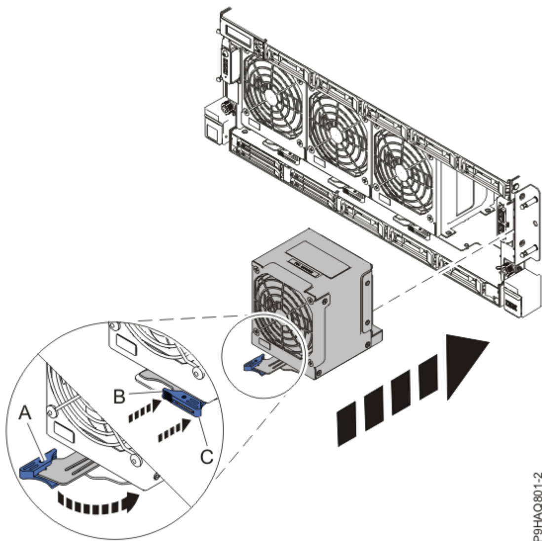
Figura 5. Sustitución de un ventilador en el sistema
