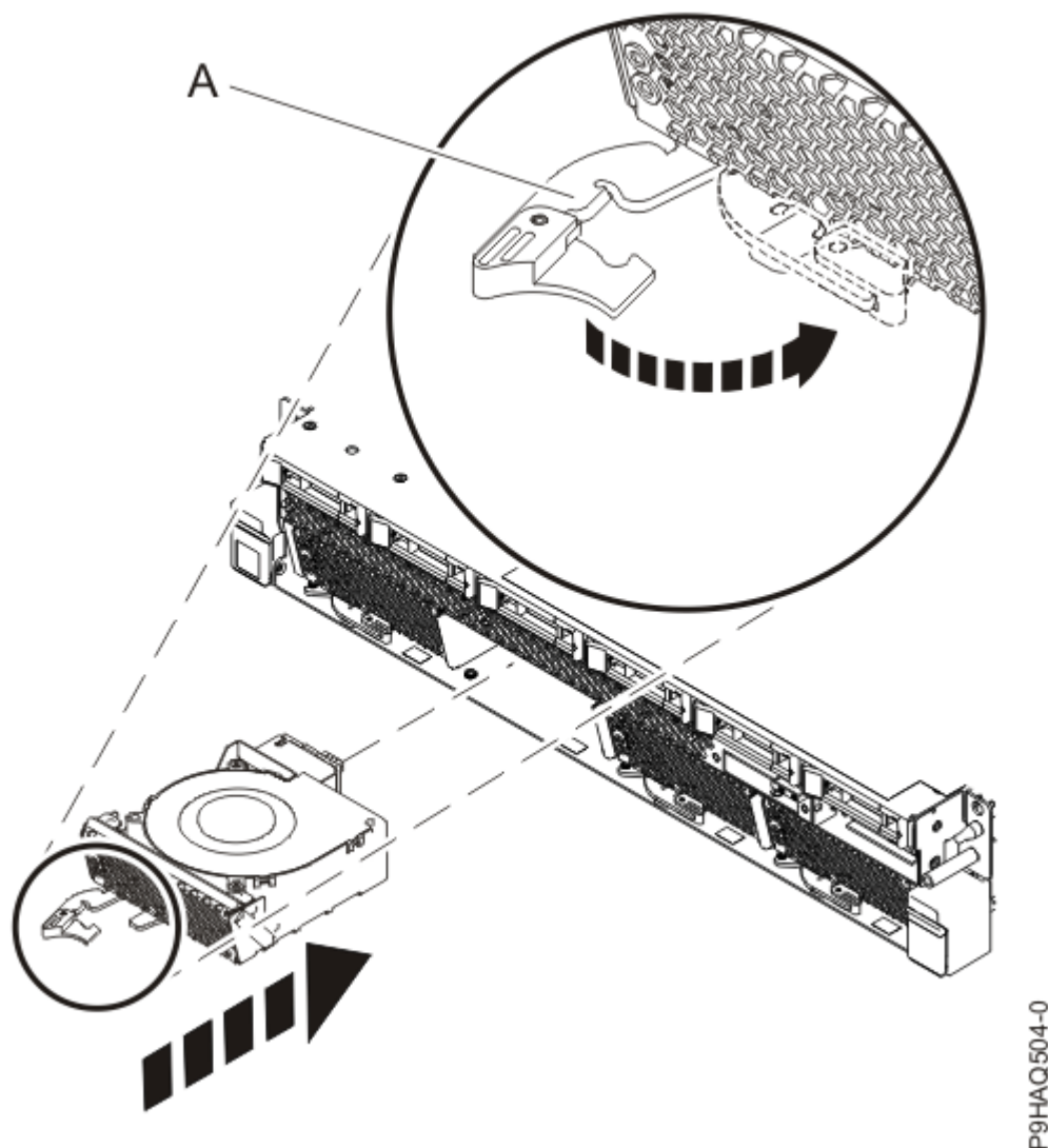
Figura 6. Sustitución de un ventilador en el sistema
