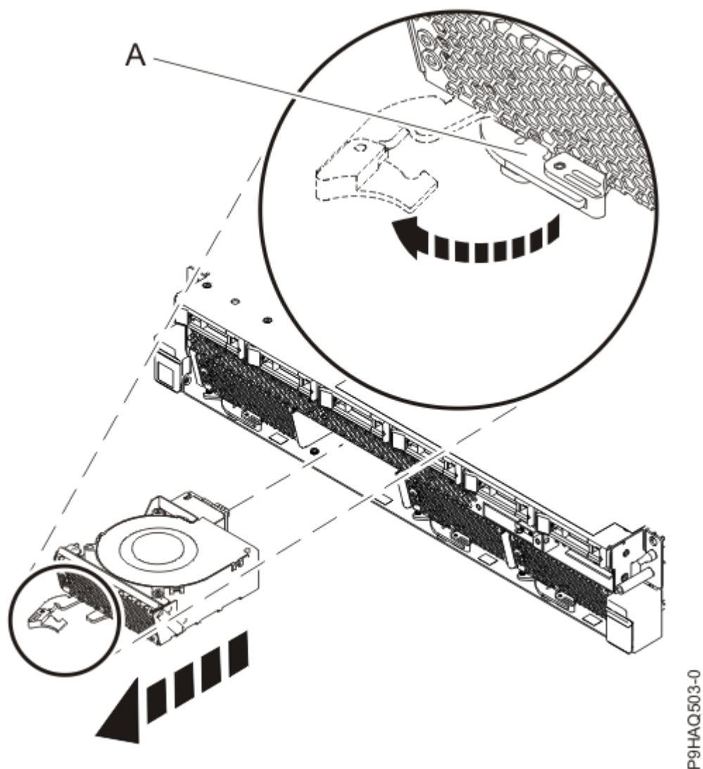
Figura 5. Extracción de un ventilador del sistema
