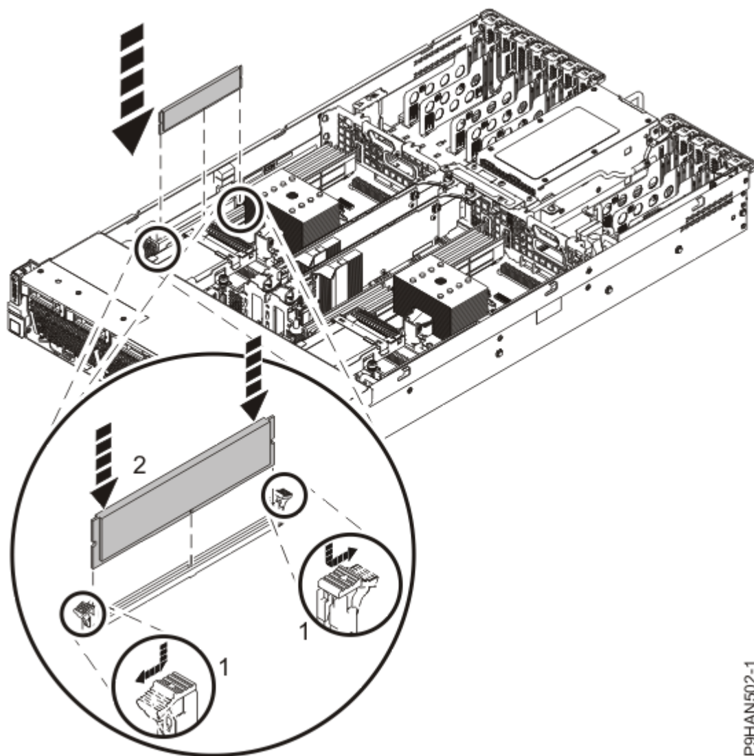
Figura 22. Sustitución de un módulo de memoria
