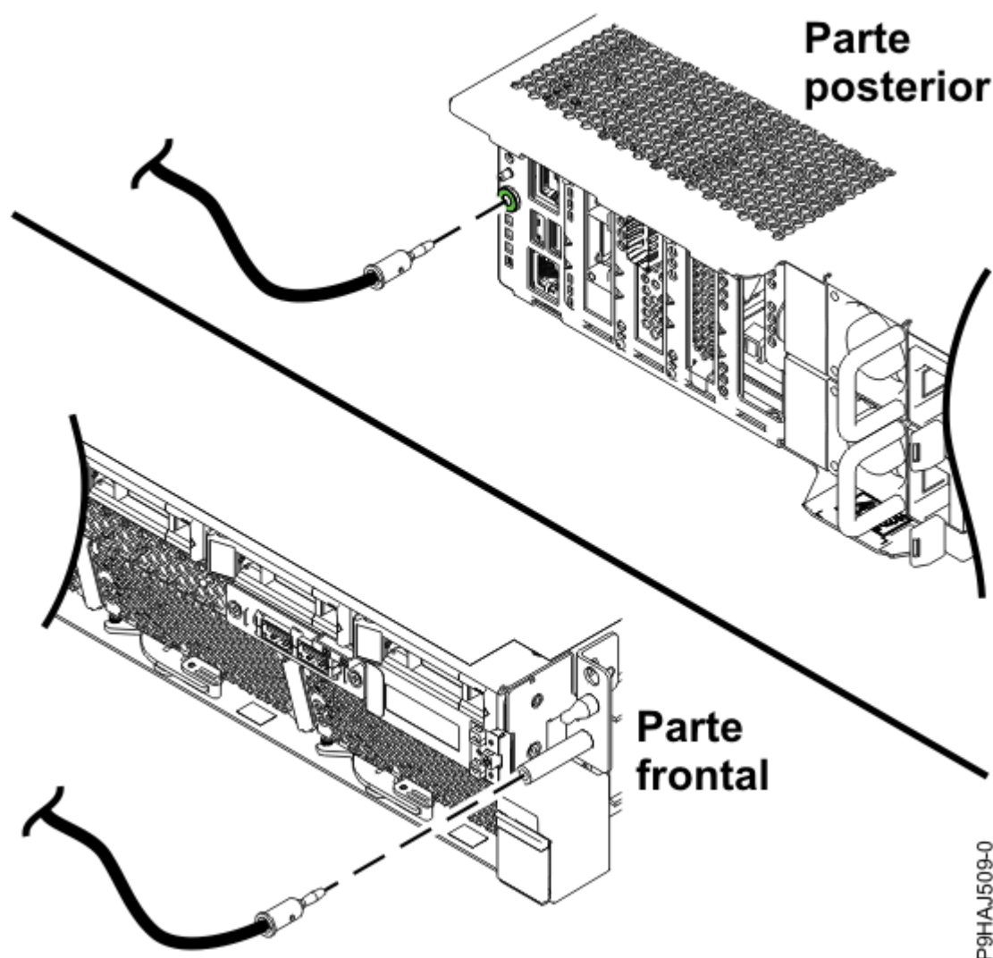
Figura 16. Ubicación de los enchufes ESD
