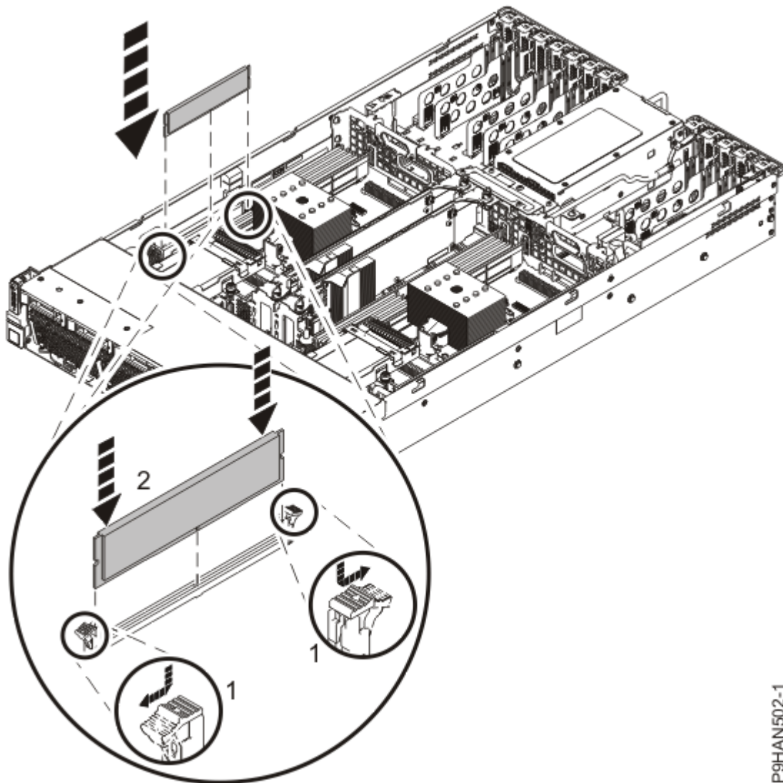
Figura 9. Instalación de un módulo de memoria
