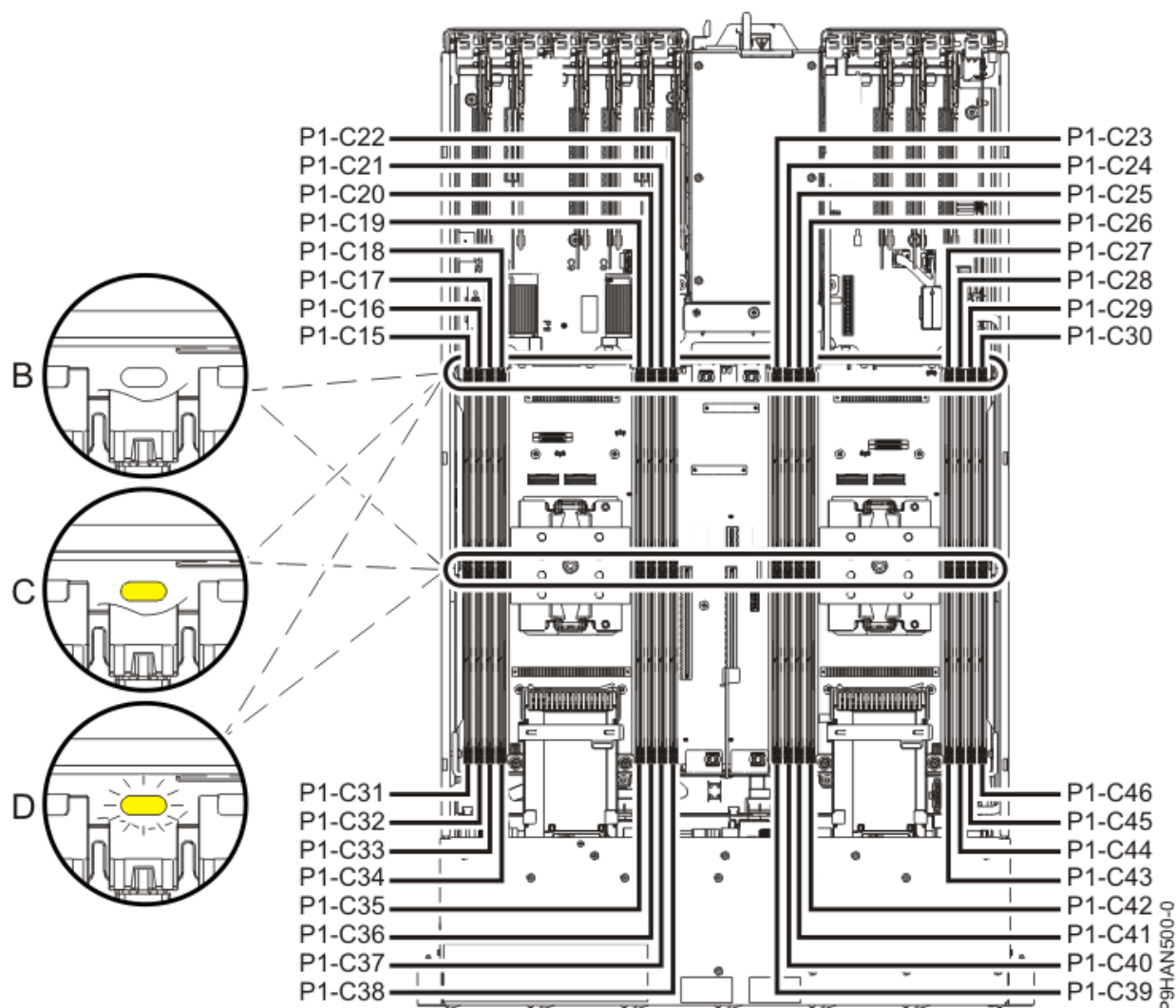
Figura 19. Indicadores LED para un módulo de memoria funcional y anómalo
