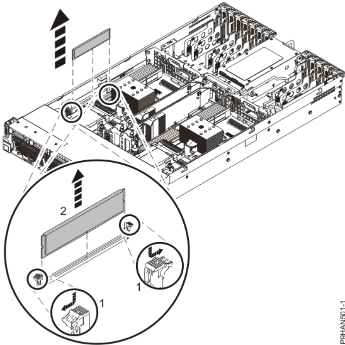
Figura 35. Extracción de un módulo de memoria
