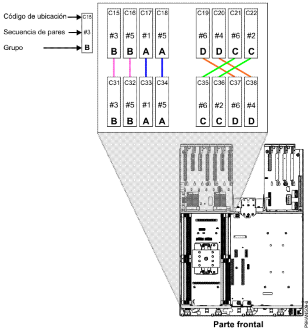
Figura 27. Secuencia de conexión, un procesador del sistema, sistema montado en bastidor
