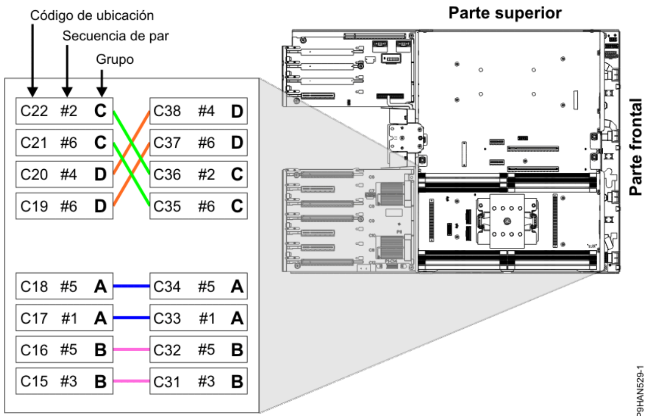
Figura 28. Secuencia de conexión, un procesador del sistema, sistema autónomo
