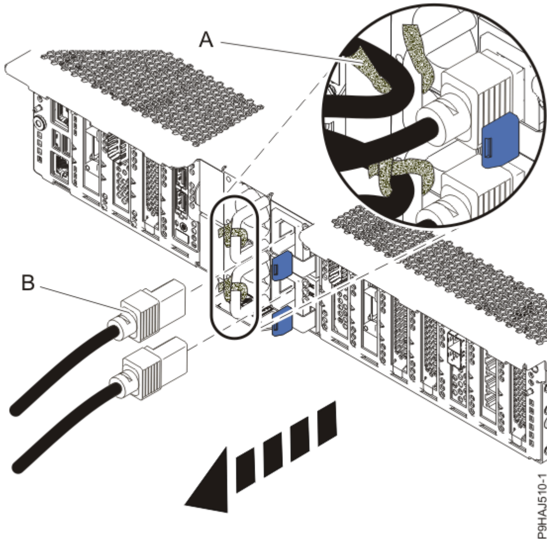
Figura 4. Extracción de los cables de alimentación
