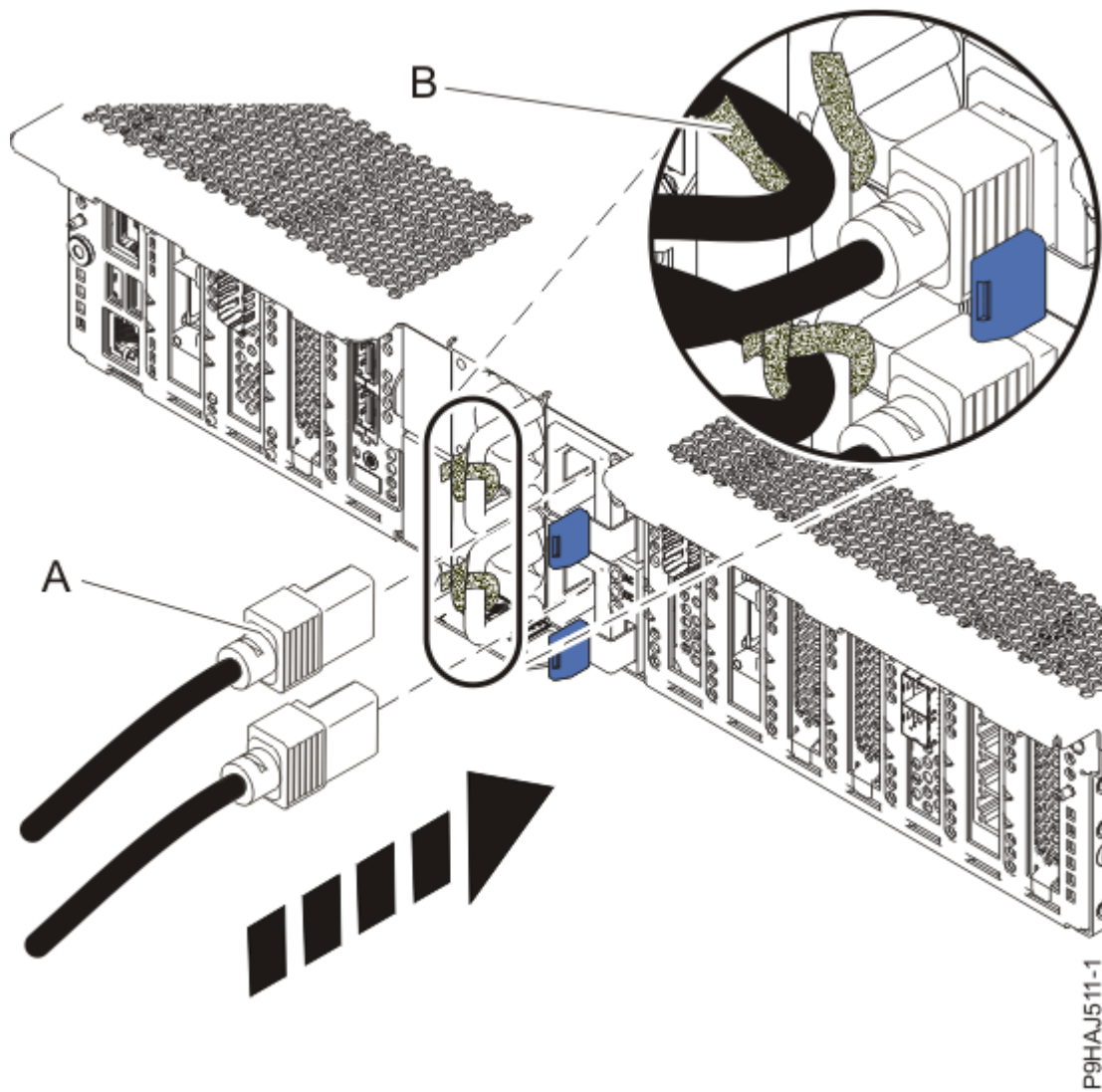
Figura 39. Conexión de los cables de alimentación
