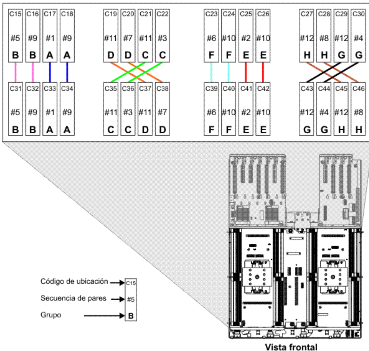
Figura 29. Secuencia de conexión, dos procesadores del sistema
