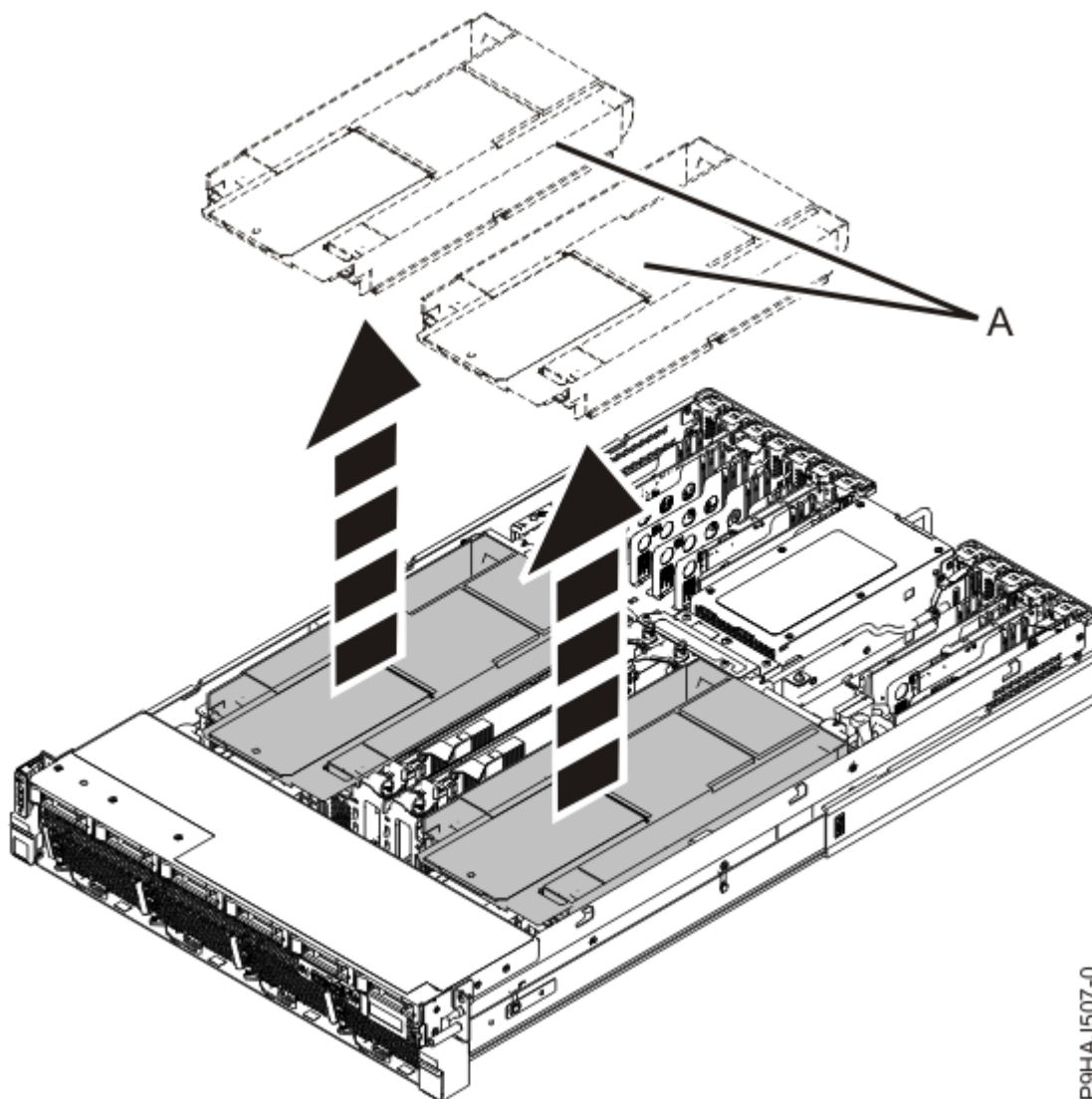
Figura 34. Extracción del deflector de aire
