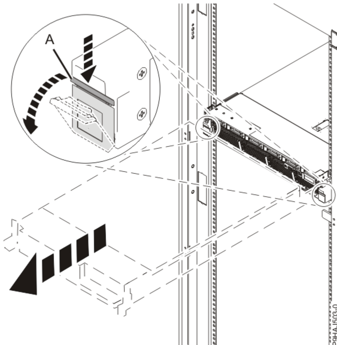
Figura 31. Cómo abrir los pestillos laterales
