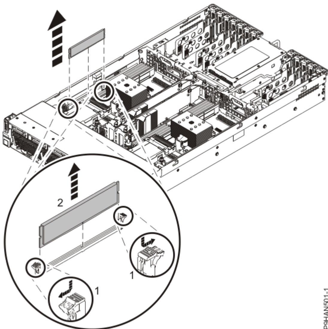
Figura 21. Extracción de un módulo de memoria
