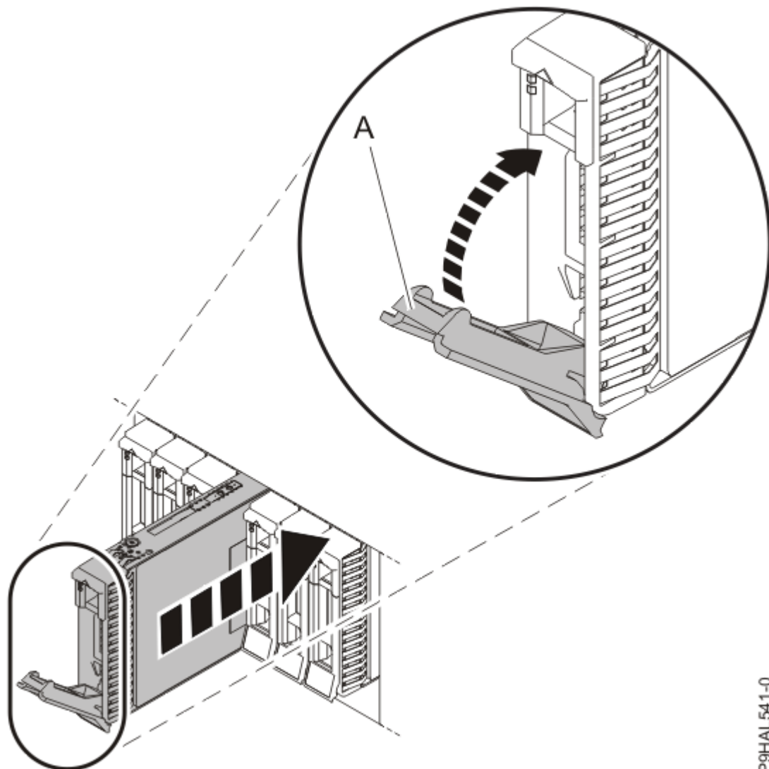
Figura 18. Sustitución de una unidad en un alojamiento
