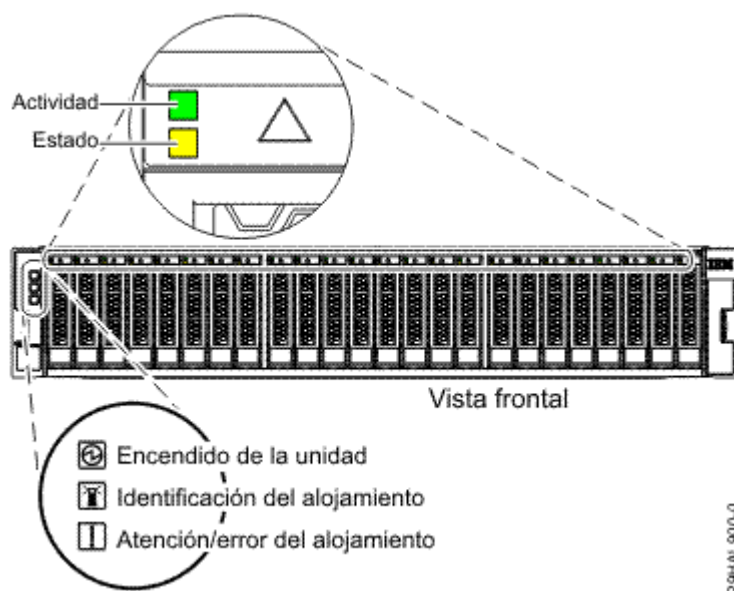
Figura 12. Vista frontal del alojamiento de almacenamiento que muestra los indicadores de servicio
