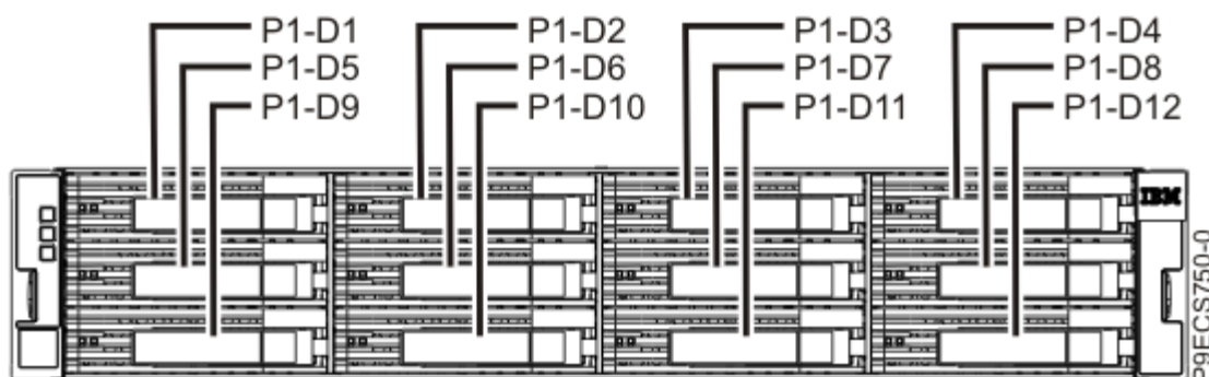
Figura 1. Vista frontal del alojamiento de almacenamiento ESLL que muestra las ubicaciones de las unidades
