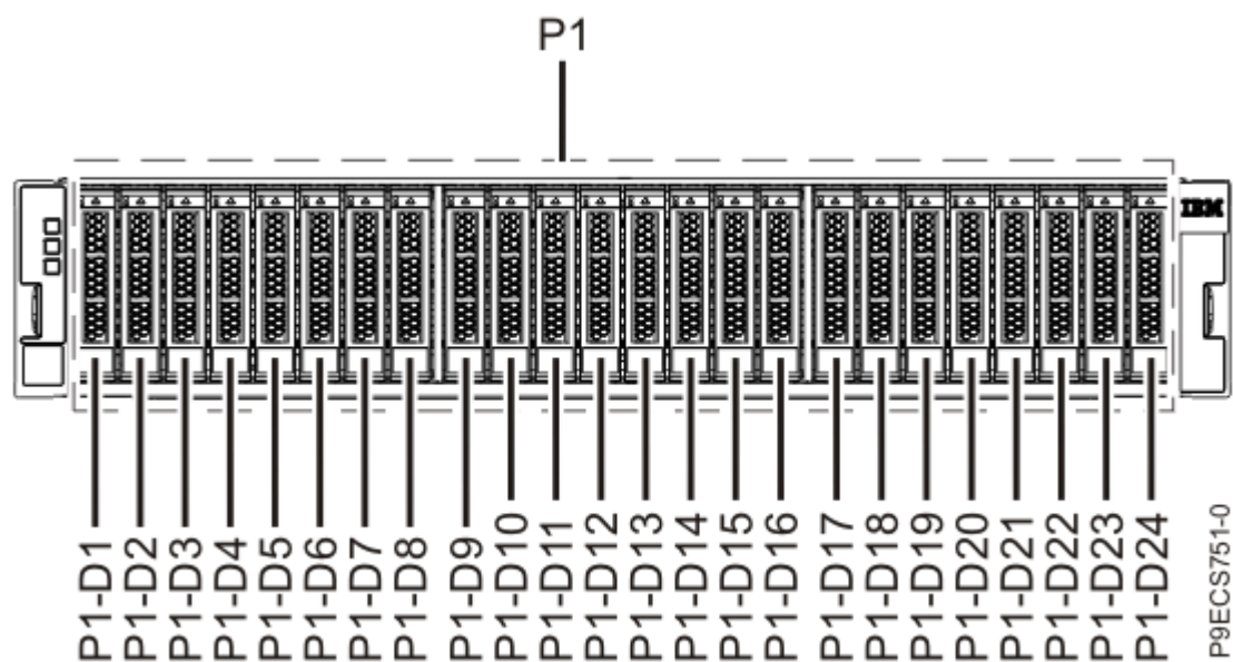
Figura 10. Vista frontal del alojamiento de almacenamiento ESLS que muestra las ubicaciones de las unidades
