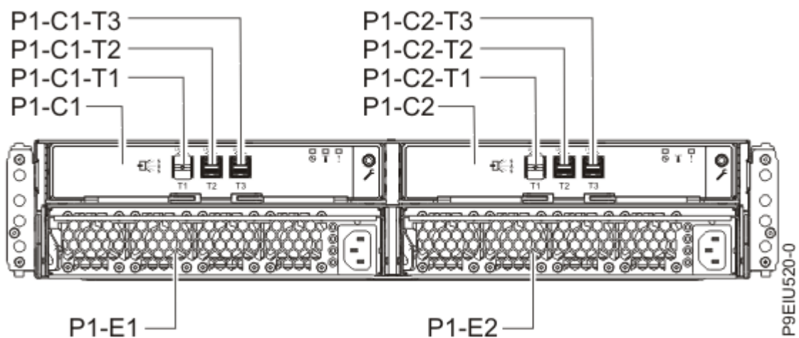
Figura 3. Vista posterior de los alojamientos de almacenamiento
