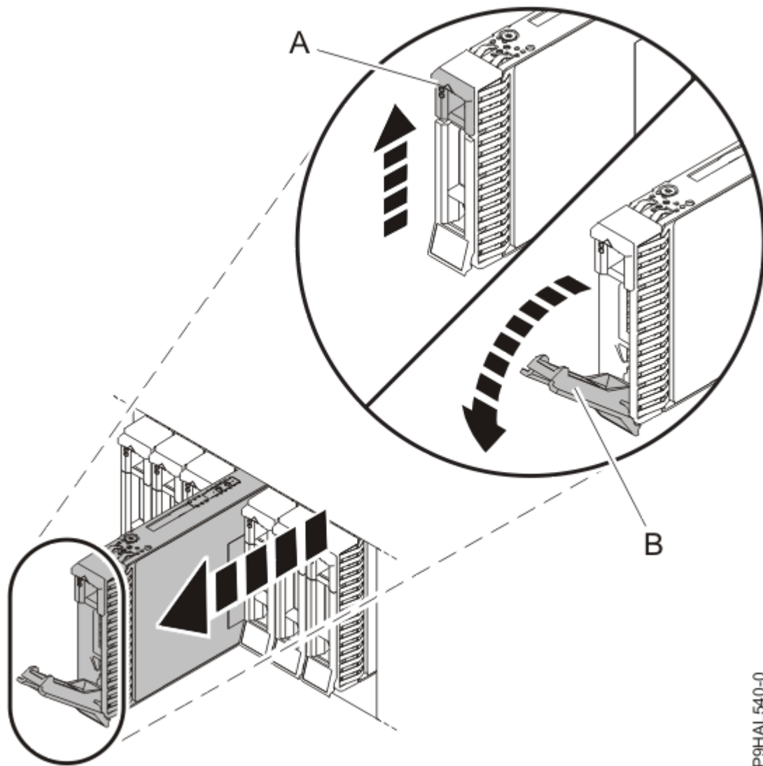
Figura 17. Desbloqueo y extracción de la unidad
