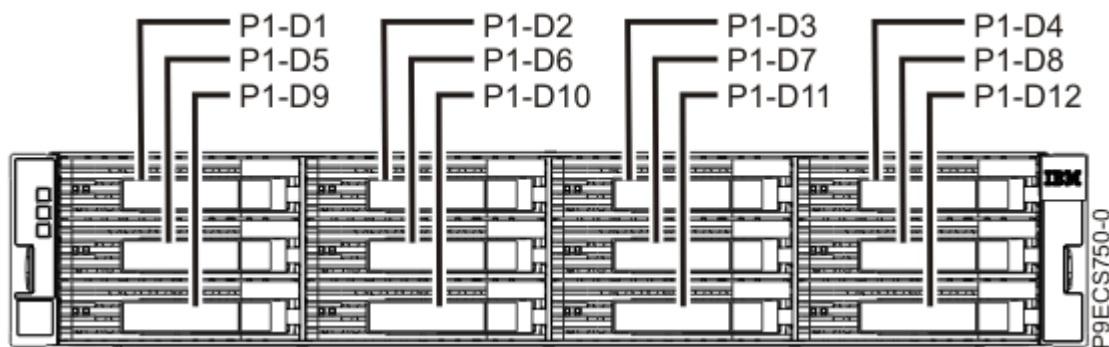
Figura 9. Vista frontal del alojamiento de almacenamiento ESLL que muestra las ubicaciones de las unidades
