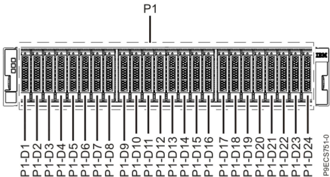
Figura 2. Vista frontal del alojamiento de almacenamiento ESLS que muestra las ubicaciones de las unidades
