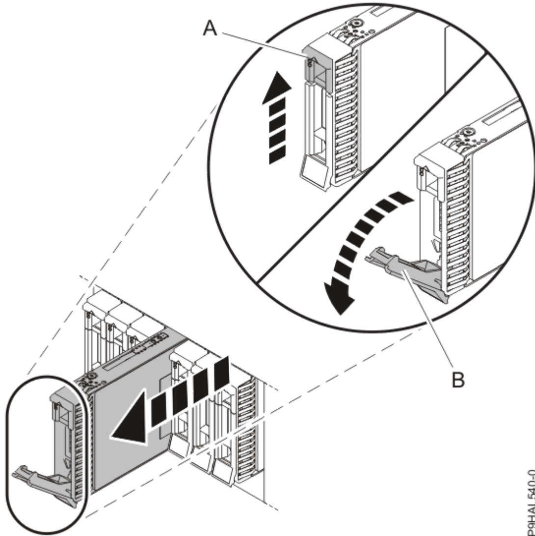
Figura 15. Desbloqueo y extracción de la unidad
