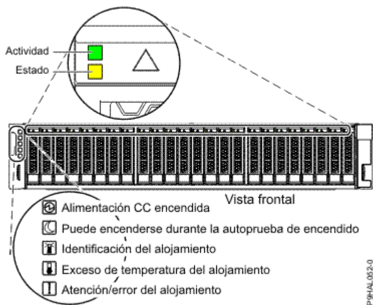
Figura 3. Vista frontal de 5887 que muestra los indicadores de servicio
