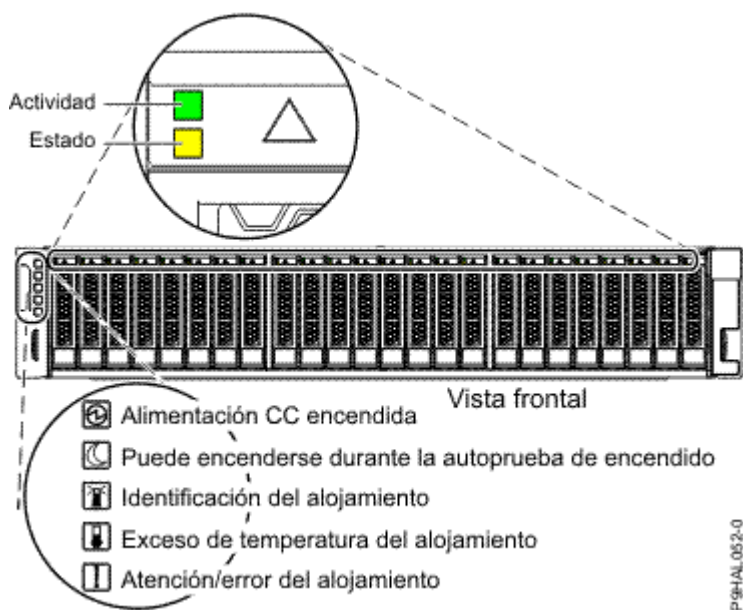
Figura 11. Vista frontal de 5887 que muestra los indicadores de servicio
