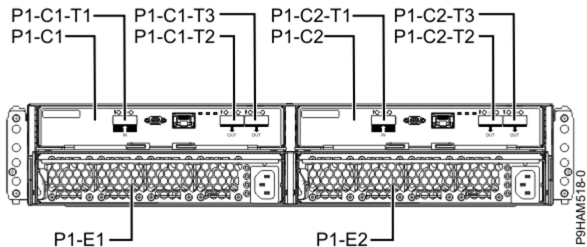
Figura 10. Vista posterior de 5887
