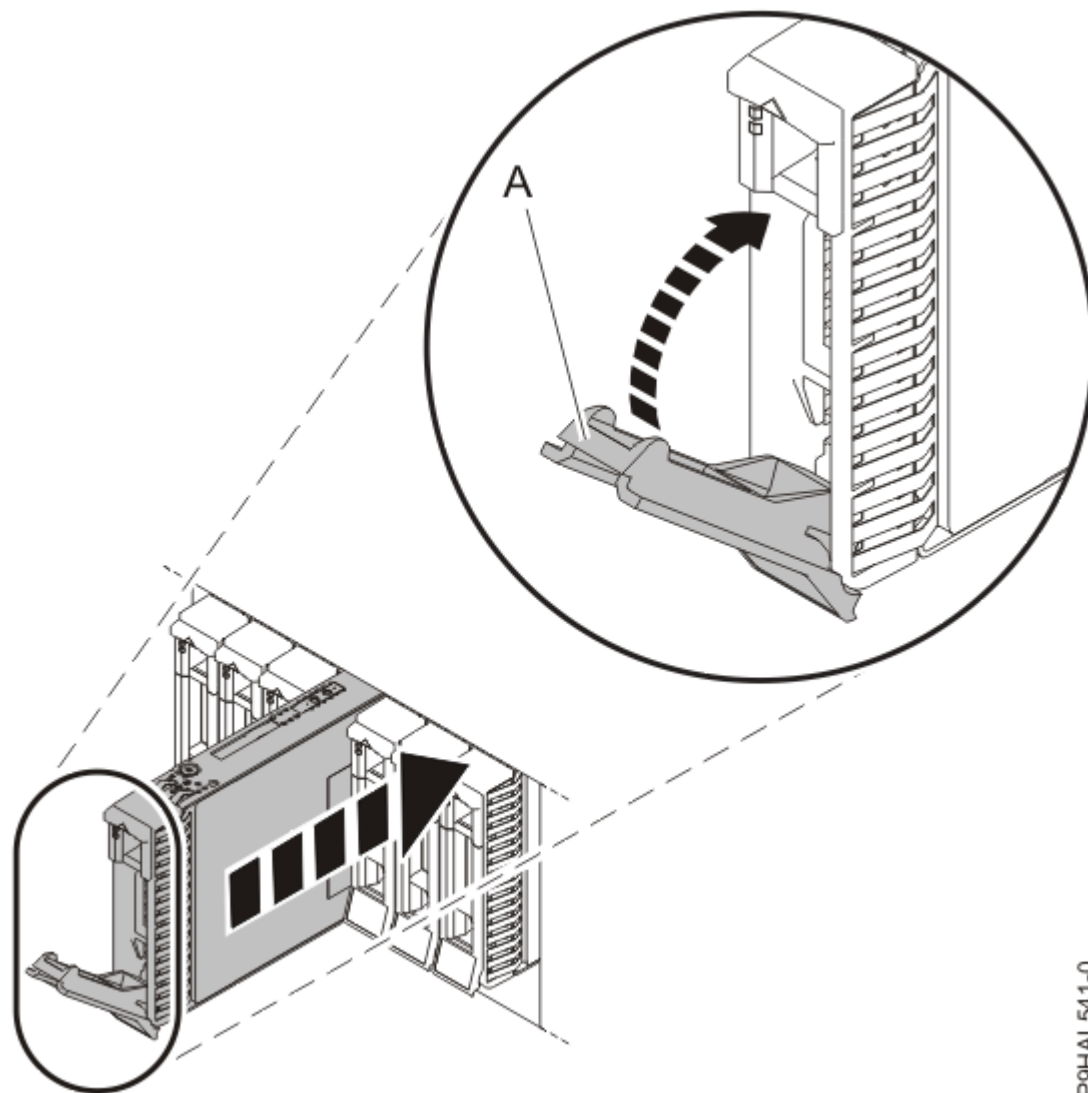
Figura 19. Instalación de una unidad en un sistema
