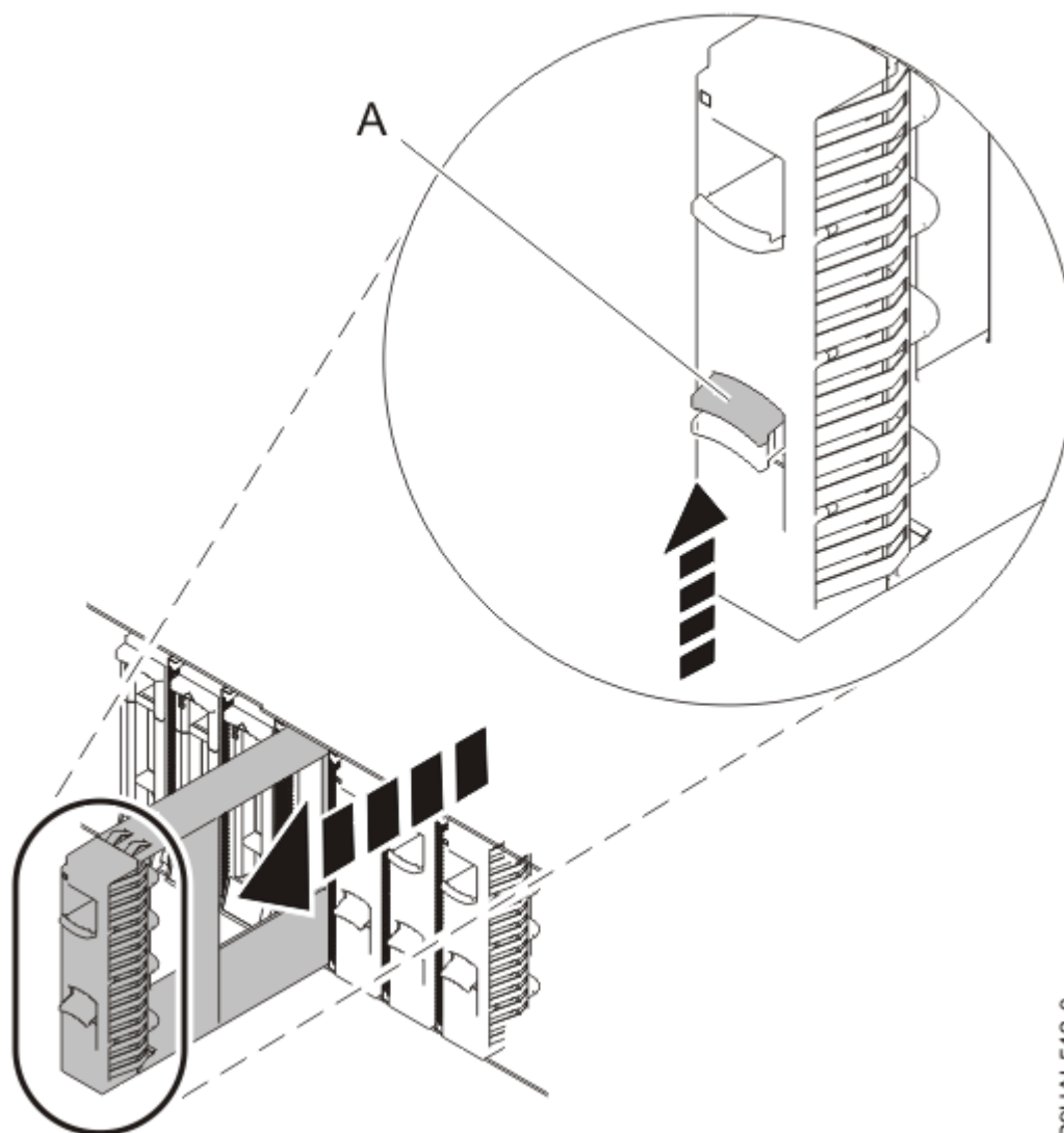
Figura 5. Extracción de un panel de relleno de la unidad
