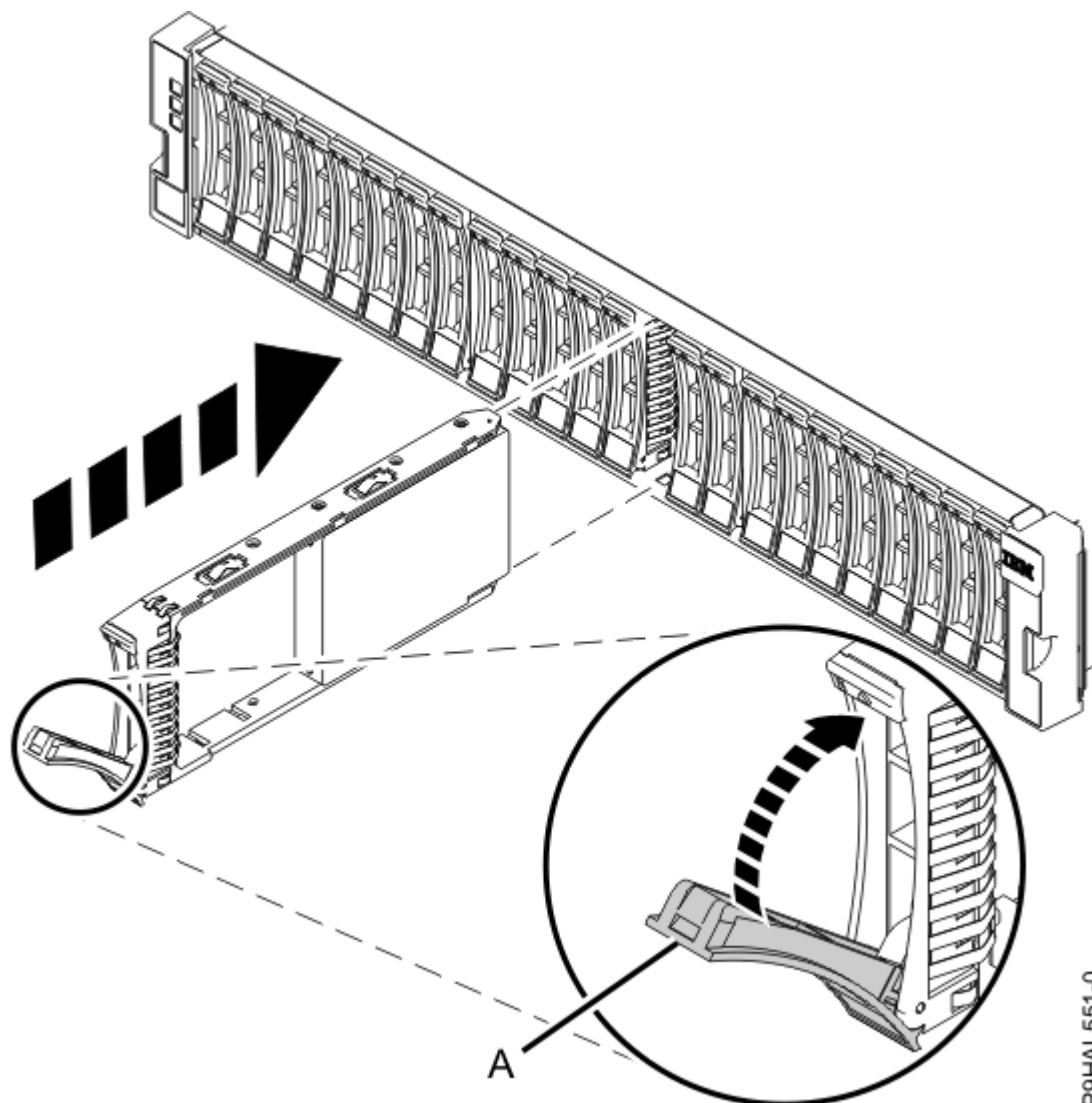
Figura 6. Instalación o sustitución de una unidad en un alojamiento
