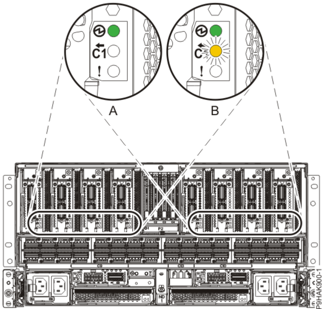
Figura 2. Ubicaciones de los LED de adaptador en un sistema 9080-M9S
