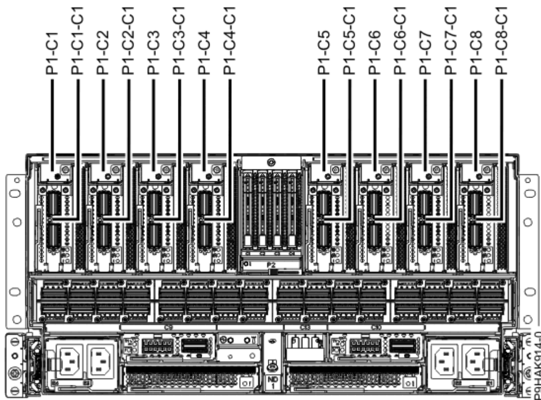
Figura 1. Ubicaciones de los adaptadores y de las casetes en el sistema 9080-M9S
