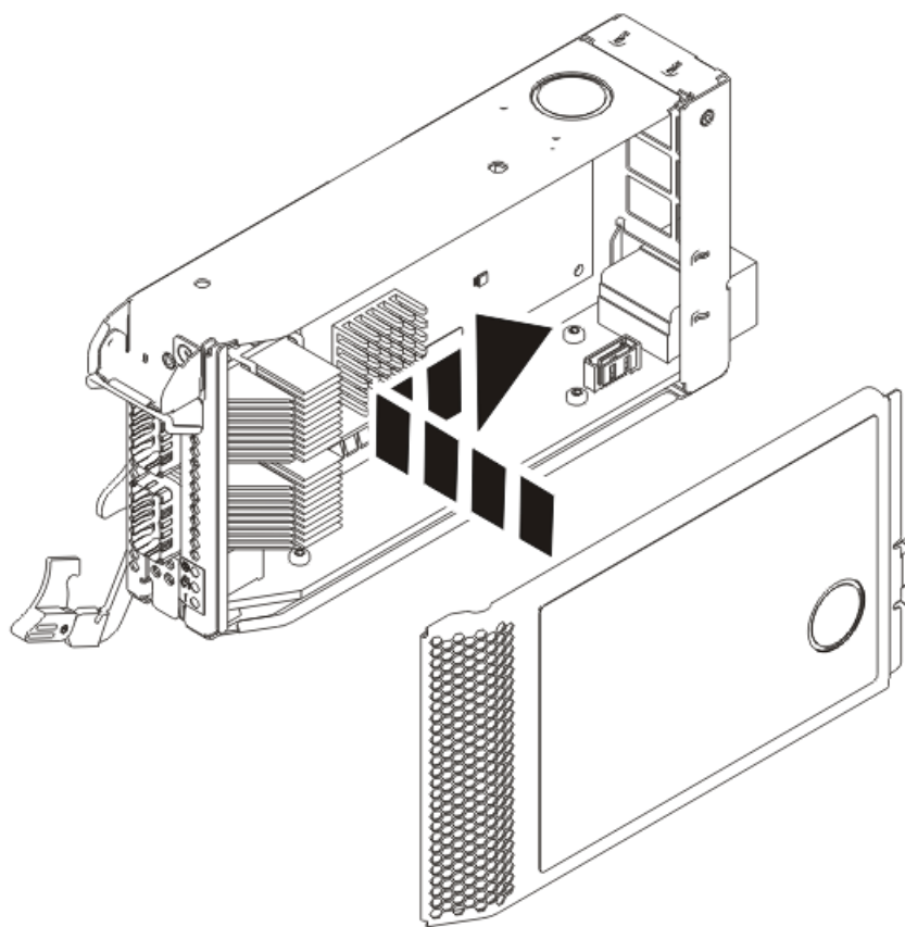
Figura 13. Sustitución de la cubierta lateral en la casete del adaptador para el sistema 9080-M9S
