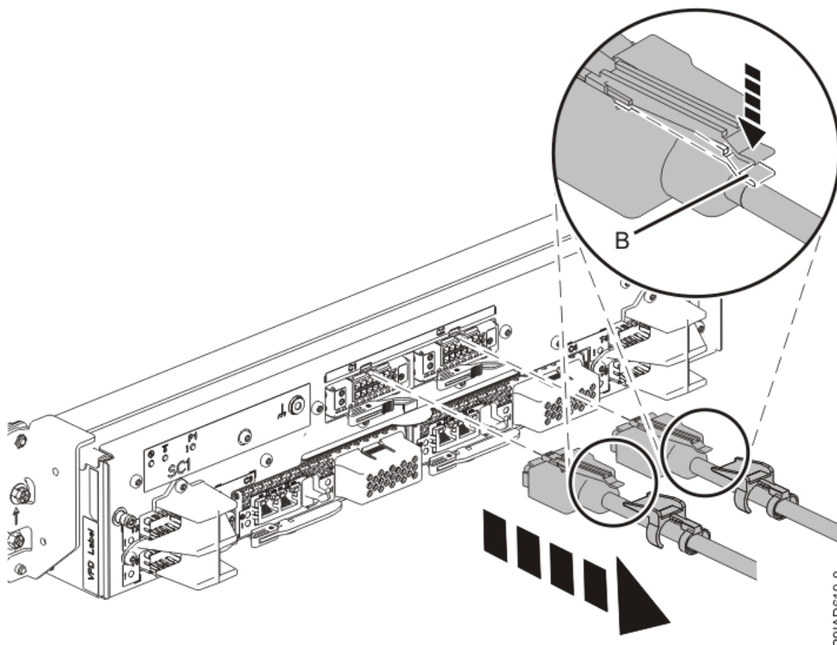
Figura 4. Extracción del cable UPIC de la unidad de control del sistema
