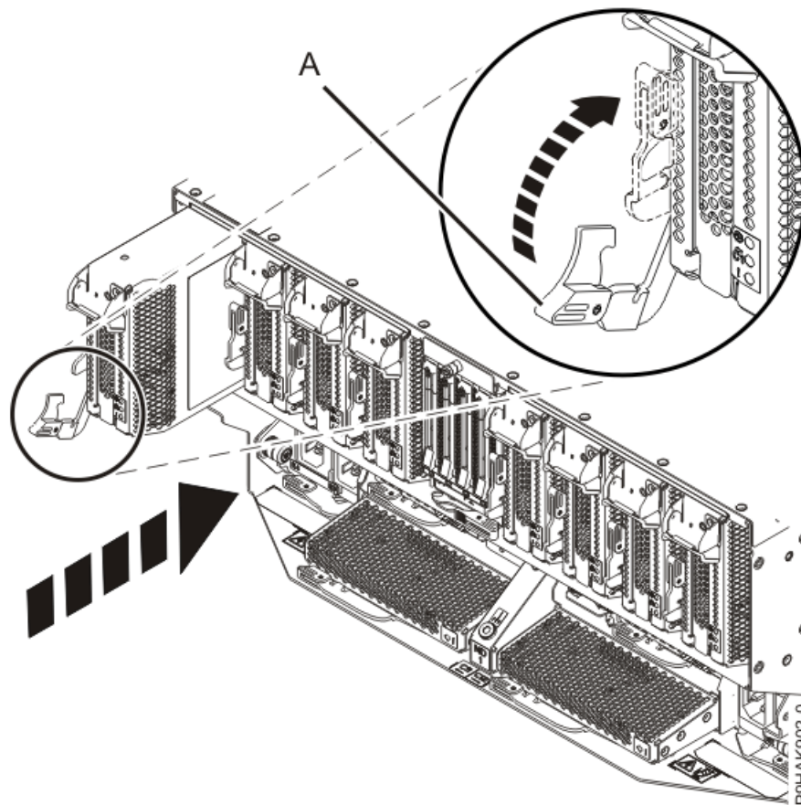
Figura 14. Instalación de una casete en el sistema 9080-M9S
