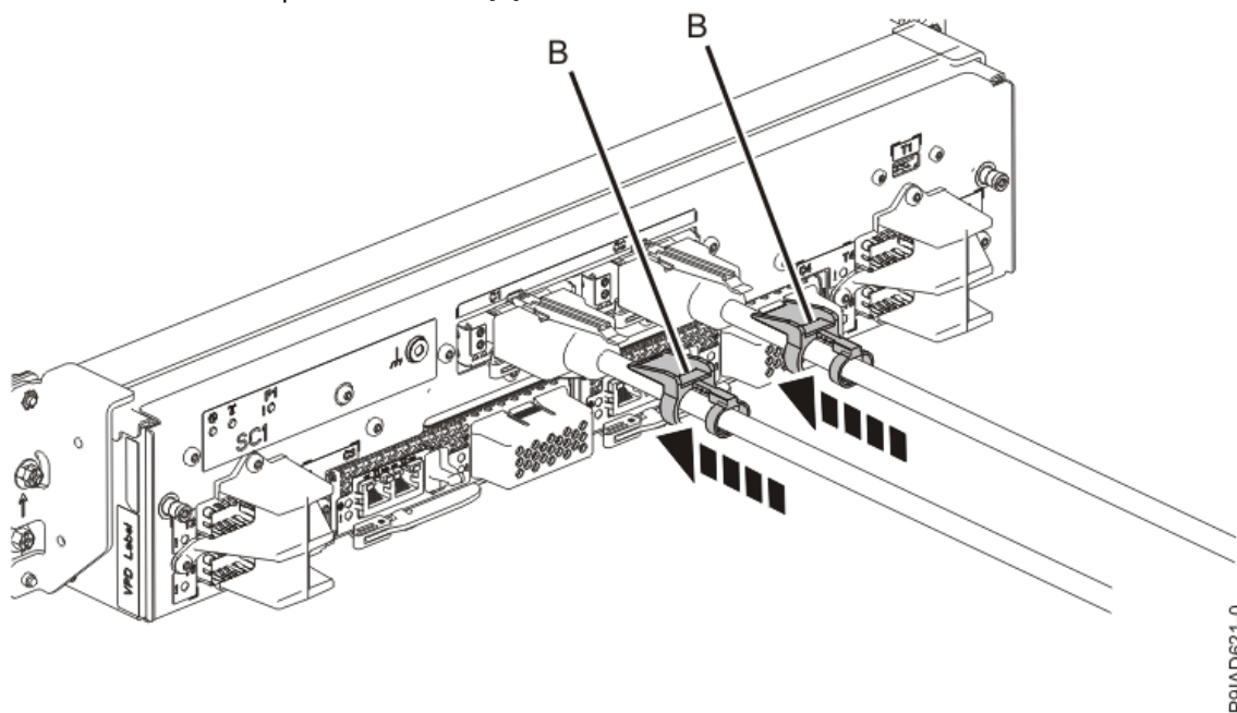
Figura 17. Sustitución del cable UPIC en la unidad de control del sistema
