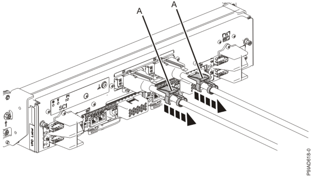
Figura 3. Extracción del cierre de cable UPIC
