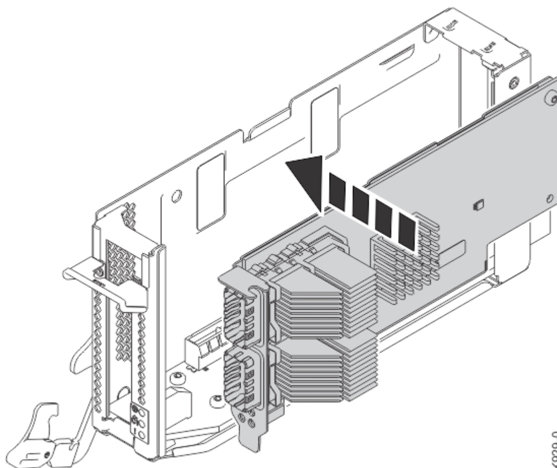
Figura 11. Instalación de un adaptador en una casete para el sistema 9080-M9S
