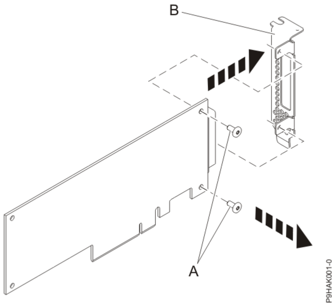
Figura 18. Extracción de la contrapunta de altura reducida de un adaptador
