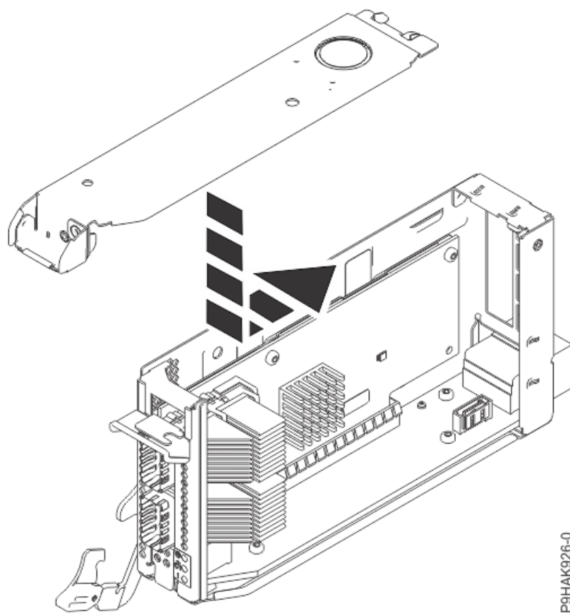
Figura 12. Sustitución de la cubierta superior en la casete del adaptador para el sistema 9080-M9S
