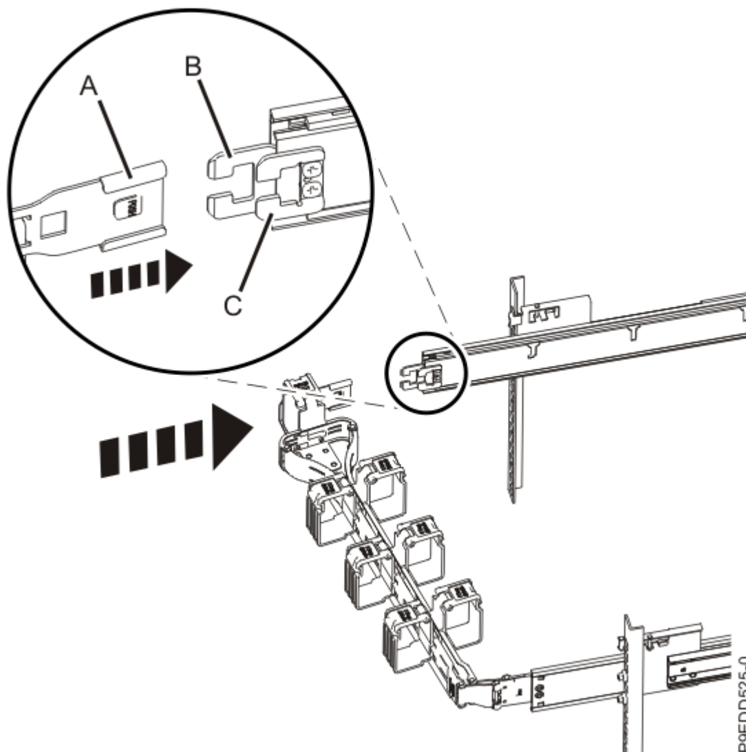
Figura 7. Cierre del brazo portacables
