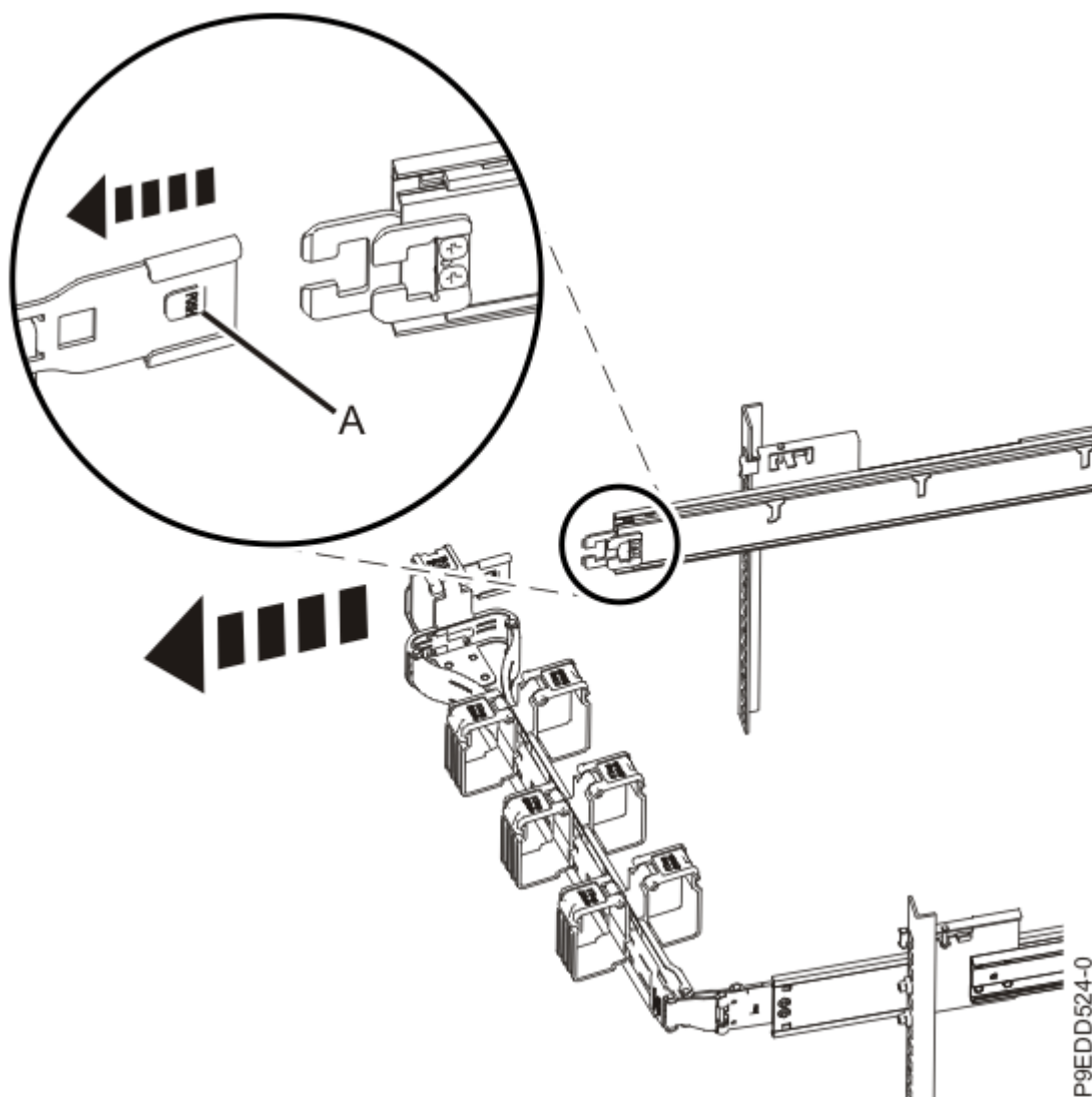
Figura 20. Liberación de la abrazadera de montaje
