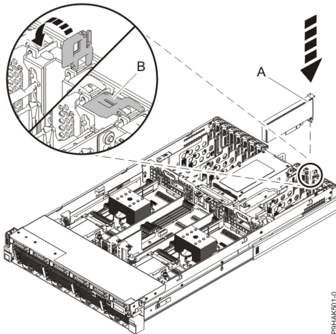
Figura 11. Instalación o sustitución de un adaptador en un 5105-22E, 9008-22L, 9009-22A, 9009-22G, 9223-22H o 9223-22S
