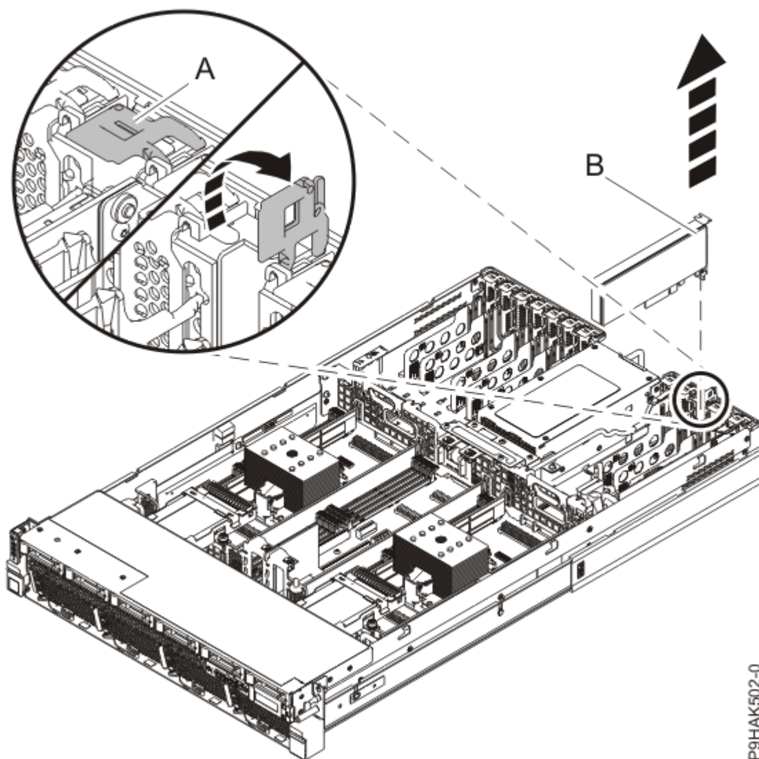
Figura 38. Extracción de un adaptador del sistema 5105-22E, 9008-22L, 9009-22A, 9009-22G, 9223-22H o 9223-22S
