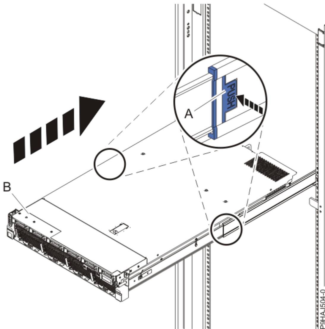
Figura 41. Colocación del sistema en la posición operativa
