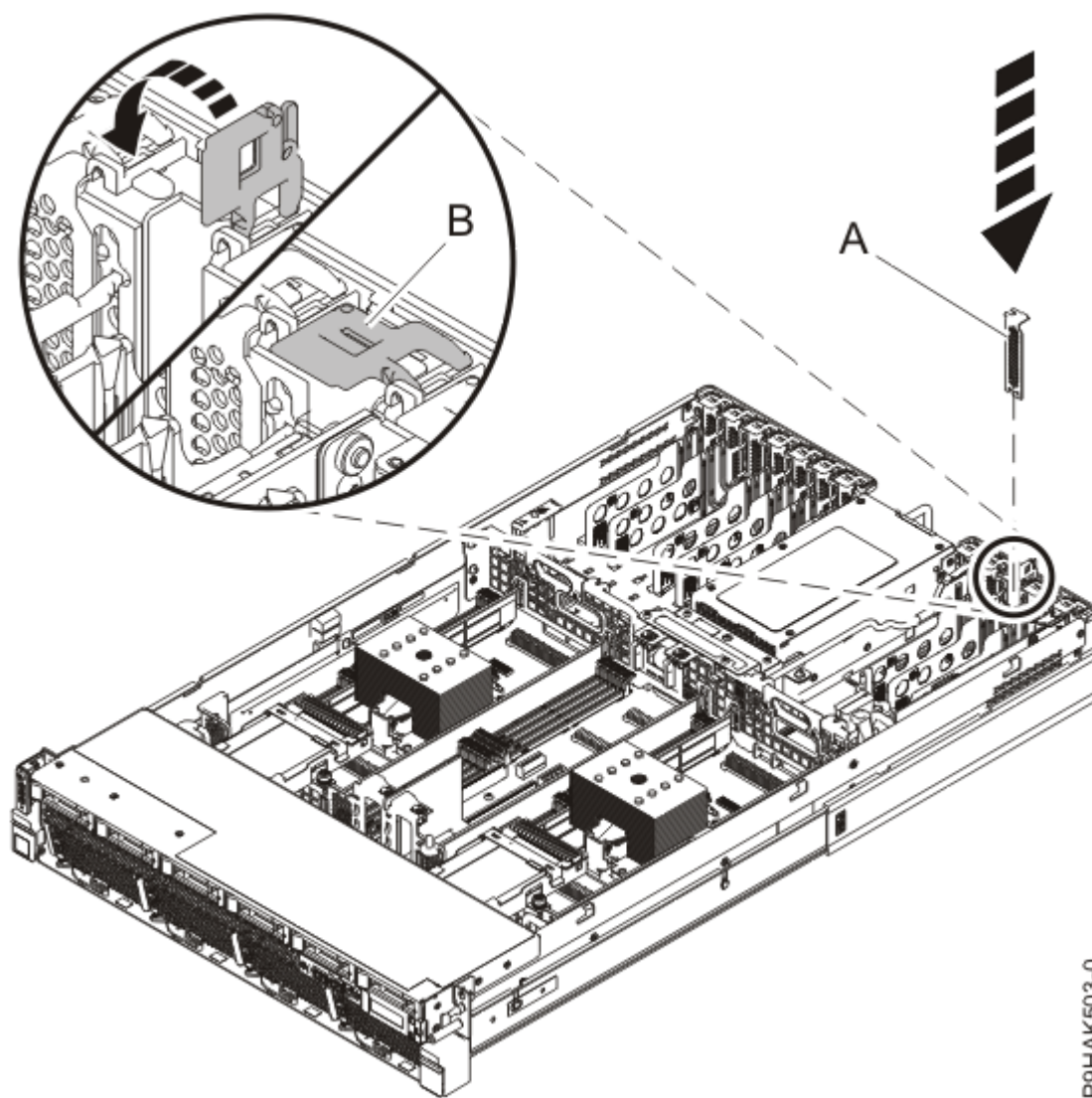
Figura 39. Instalación de un panel de relleno en una ranura en un sistema 5105-22E, 9008-22L, 9009-22A, 9009-22G, 9223-22H o 9223-22S
