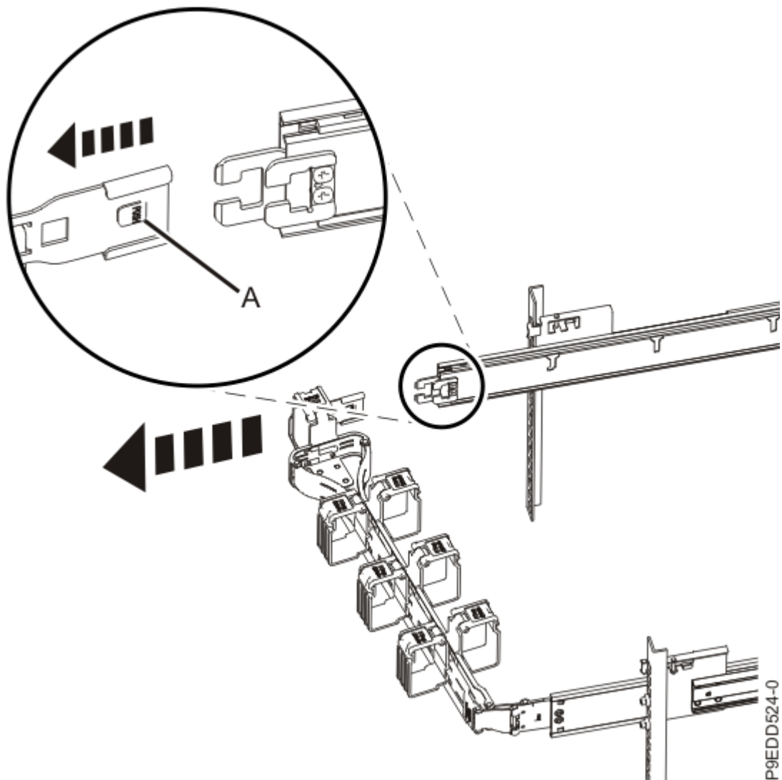
Figura 2. Liberación de la abrazadera de montaje
