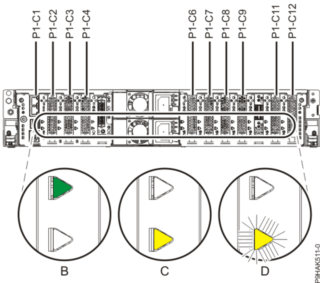
Figura 1. Ubicación de las ranuras del adaptador y de los LED en el sistema 5105-22E, 9008-22L, 9009-22A, 9009-22G, 9223-22H o 9223-22S
