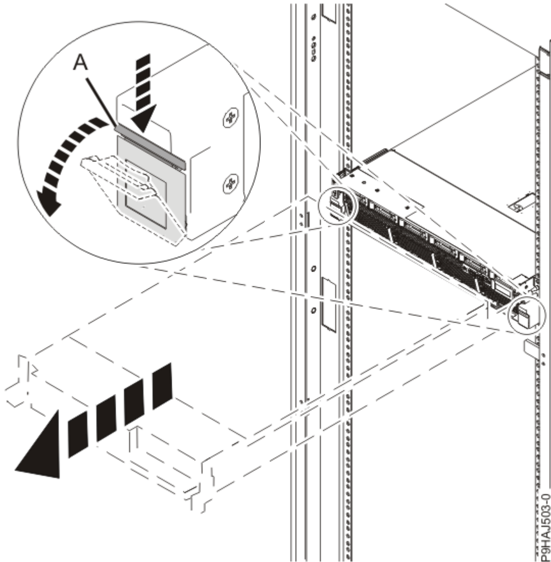
Figura 36. Cómo abrir los pestillos laterales
