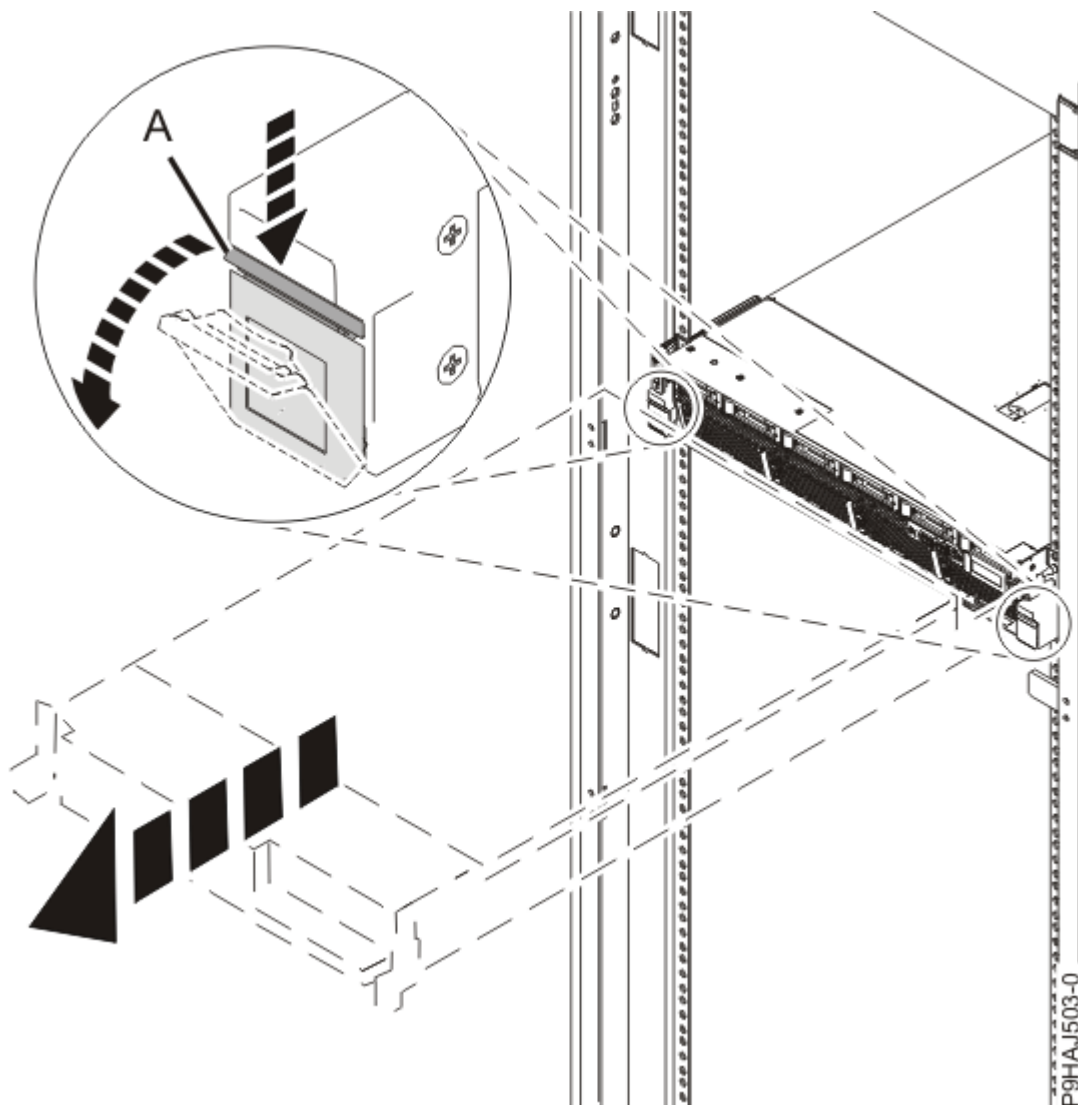
Figura 8. Cómo abrir los pestillos laterales
