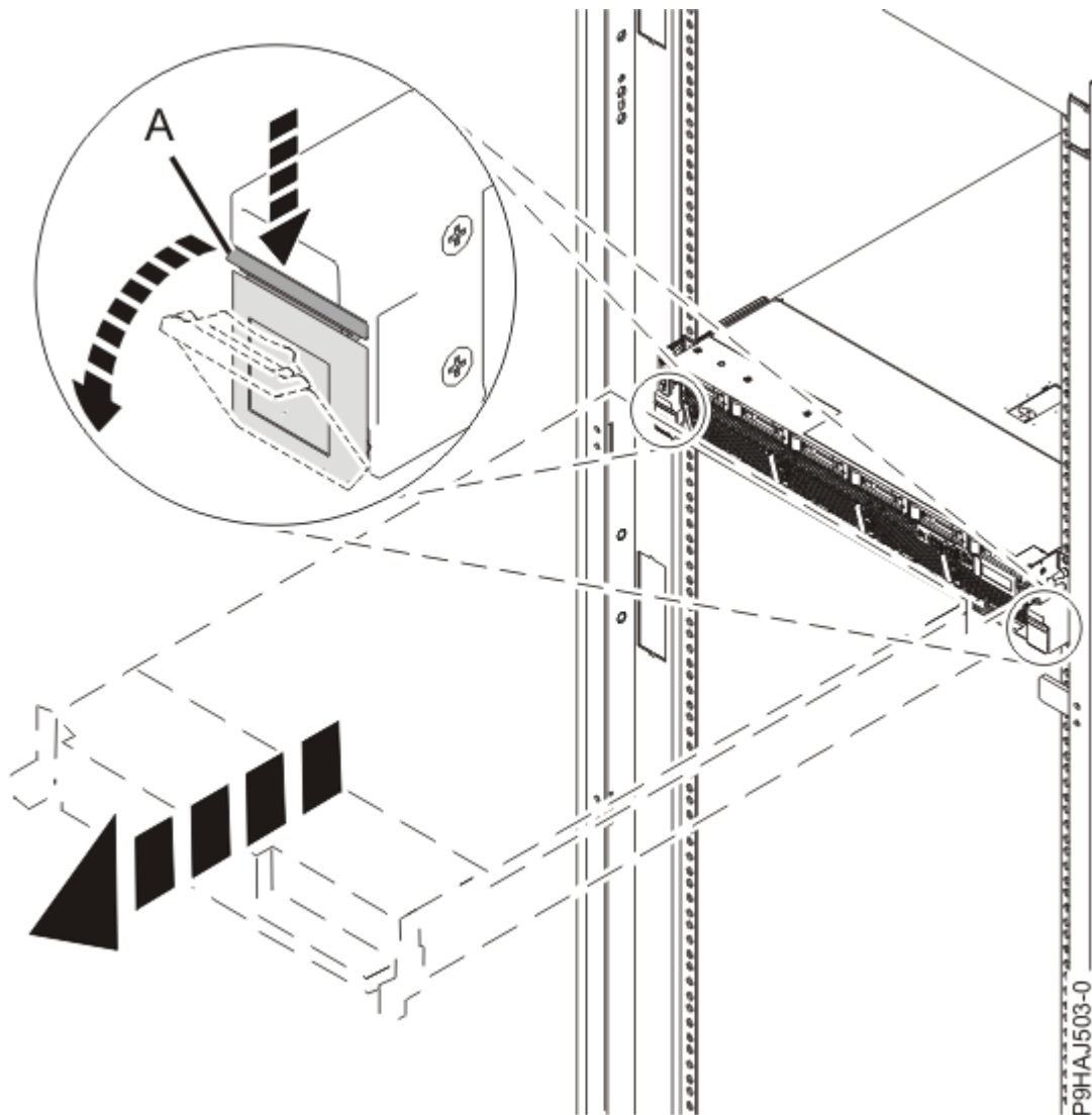
Figura 9. Cómo abrir los pestillos laterales
