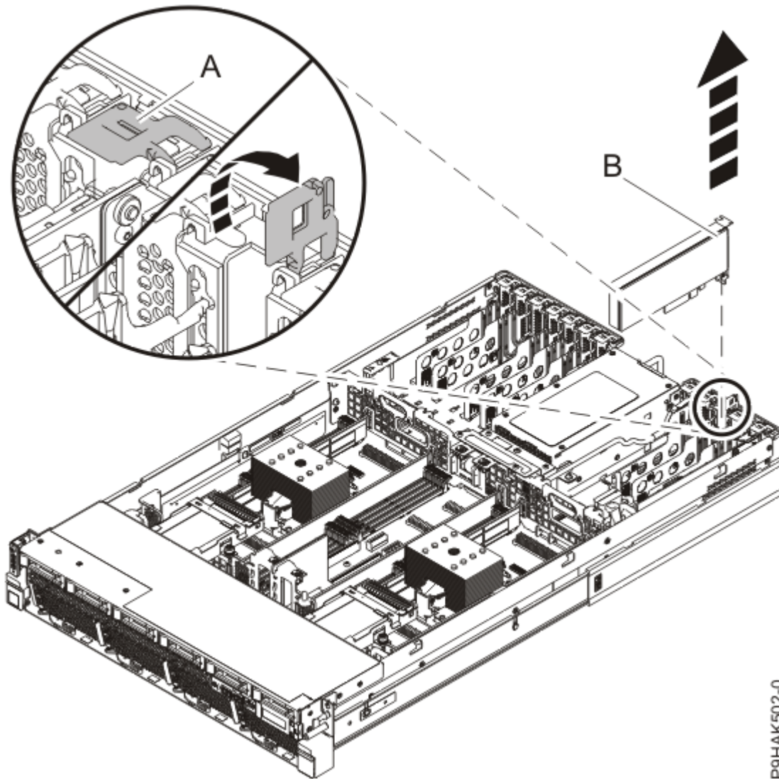
Figura 25. Extracción de un adaptador del sistema 5105-22E, 9008-22L, 9009-22A, 9009-22G, 9223-22H o 9223-22S
