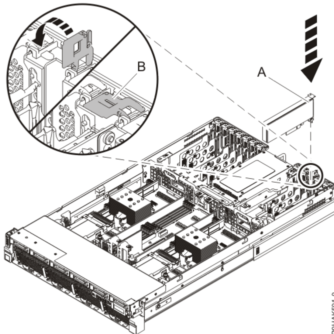
Figura 26. Instalación o sustitución de un adaptador en un 5105-22E, 9008-22L, 9009-22A, 9009-22G, 9223-22H o 9223-22S
