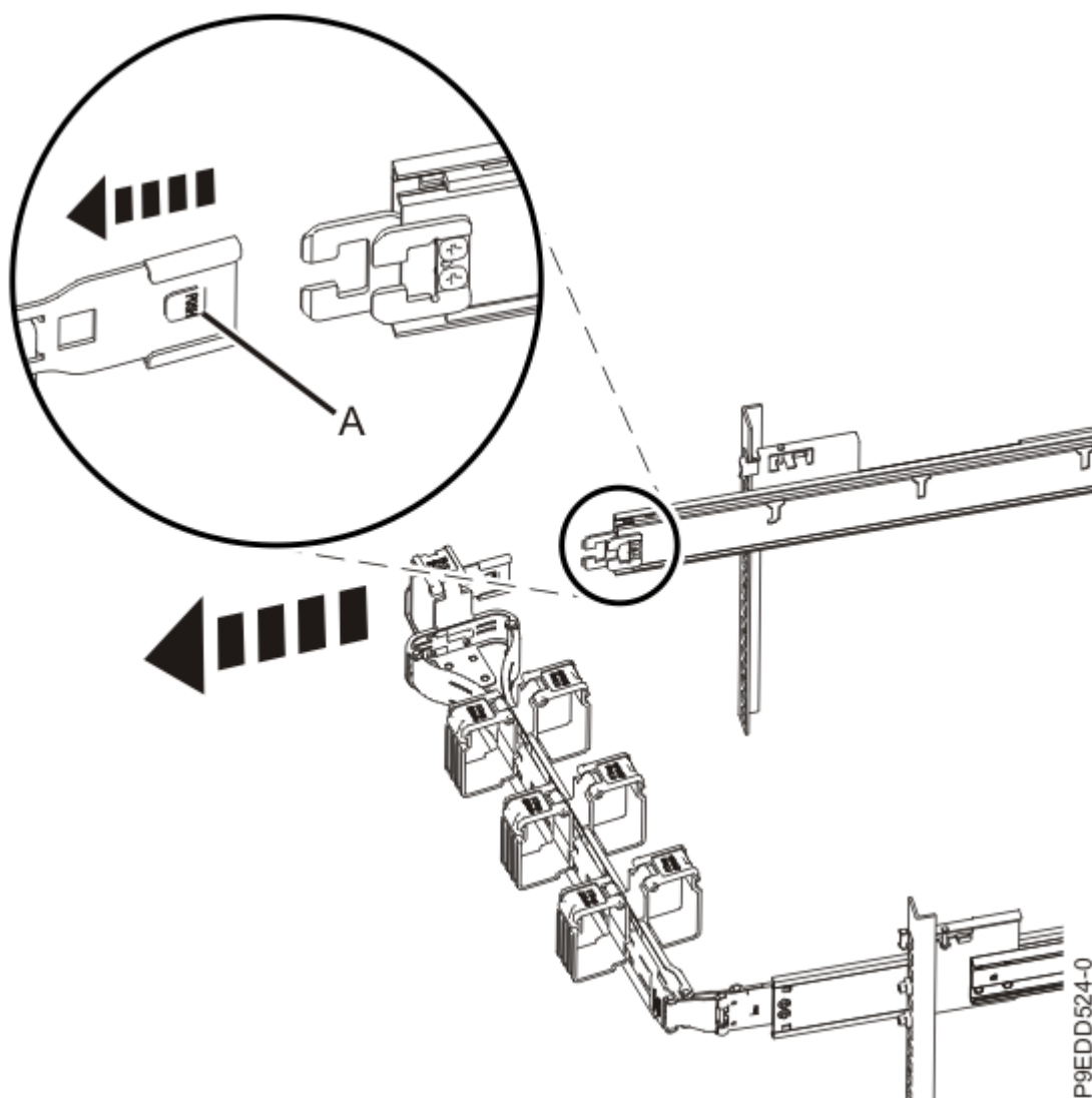
Figura 19. Liberación de la abrazadera de montaje
