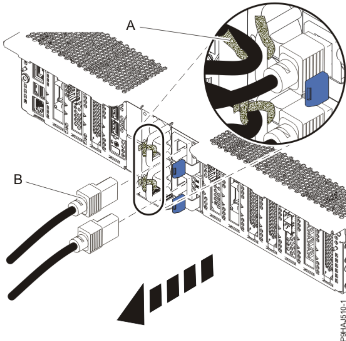
Figura 18. Extracción de los cables de alimentación
