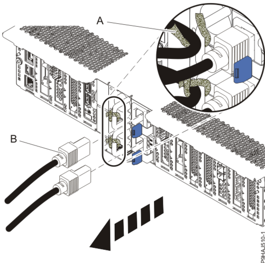
Figura 34. Extracción de los cables de alimentación
