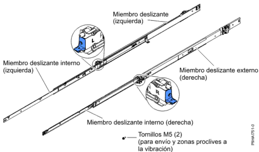
Figura 10. Contenido de la caja del riel
