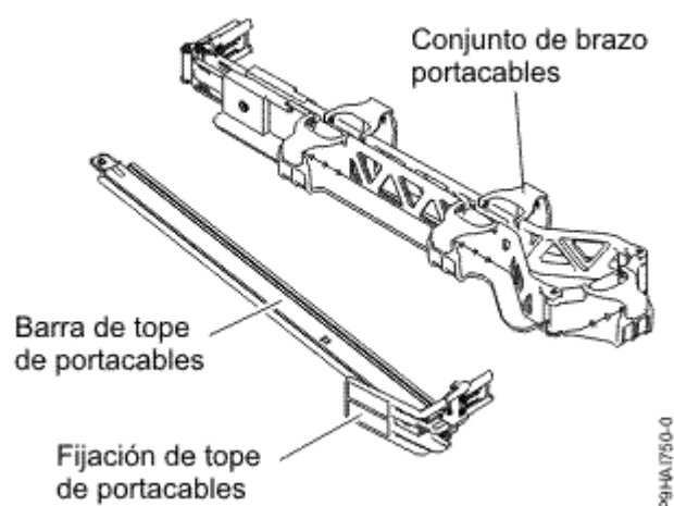
Figura 9. Contenido de la caja del brazo portacables
