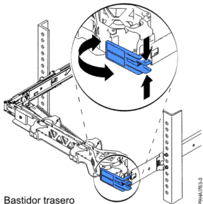
Figura 21. Soporte de fijación de tope de portacables
