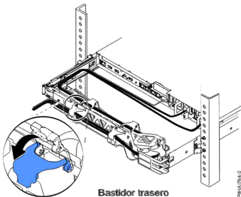
Figura 22. Conexión y direccionamiento del cable de alimentación
