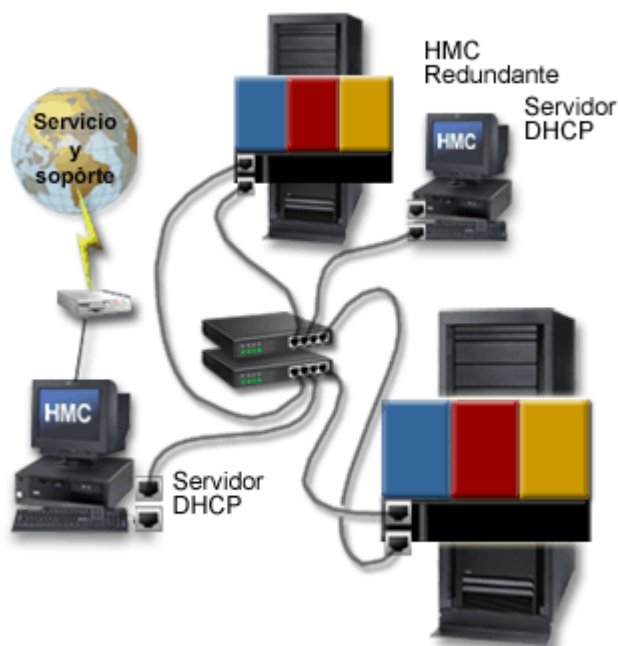
Figura 25. Red privada con una HMC como servidor DHCP
