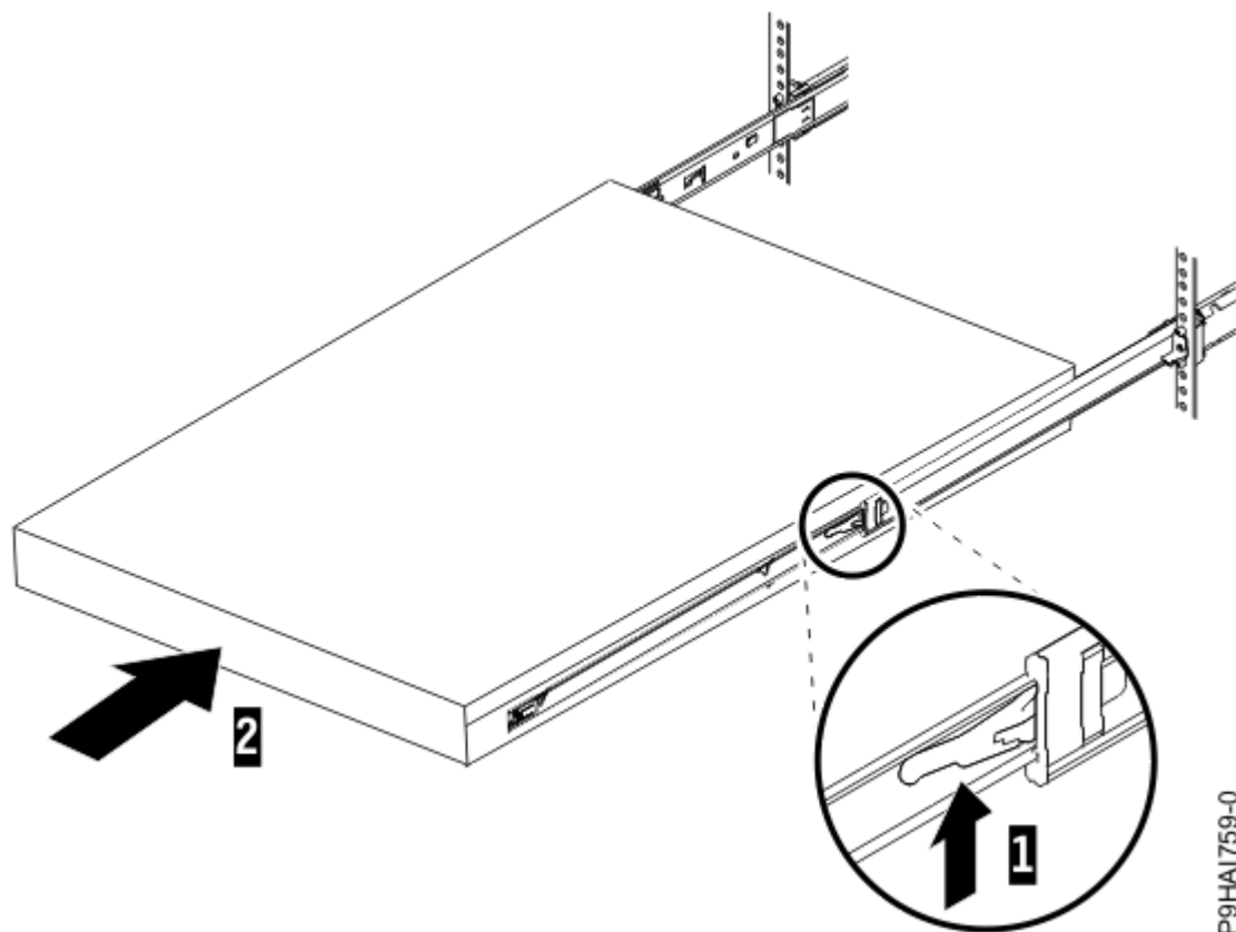
Figura 17. Pestillos de desenganche y servidor
