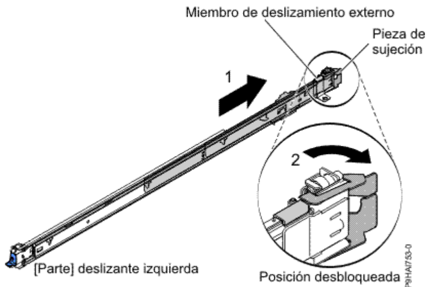
Figura 12. Riel deslizante y miembro deslizante externo
