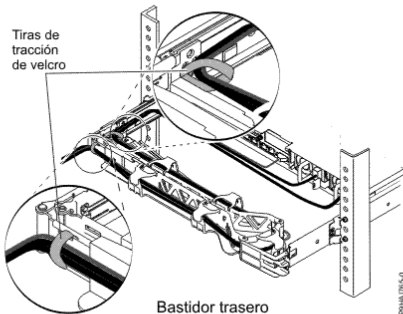
Figura 23. Cierres velcro
