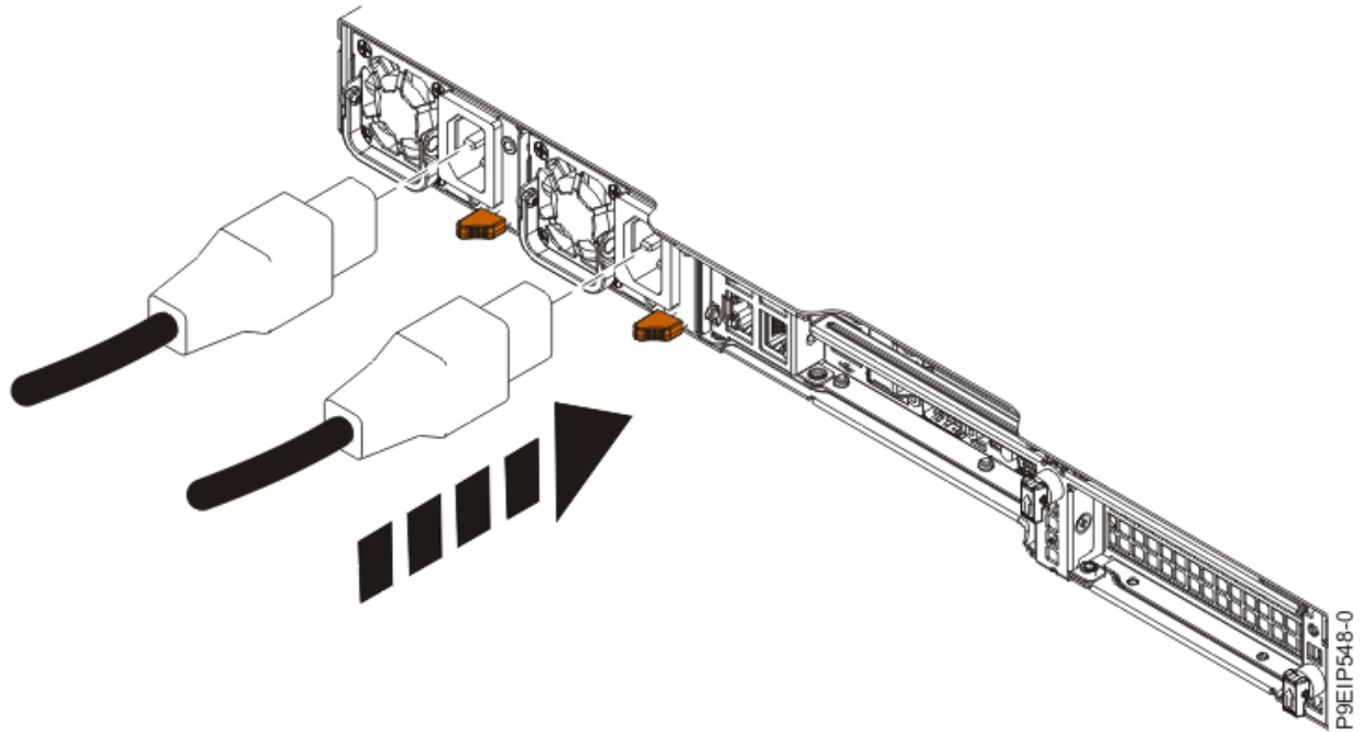
Figura 6. Conexión de los cables de alimentación a las fuentes de alimentación
