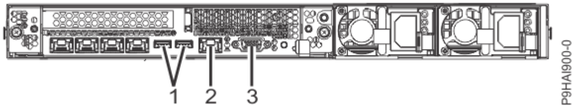
Figura 3. Puertos posteriores
