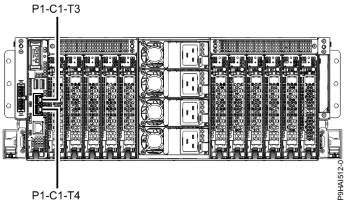
Figura 28. Ubicaciones de puertos de HMC de 9040-MR9
