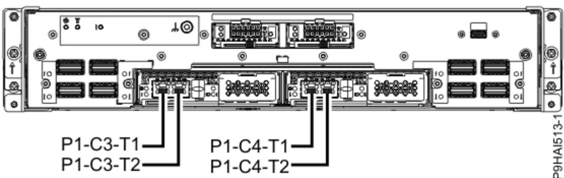
Figura 29. Ubicaciones de puertos de HMC de 9080-M9S
