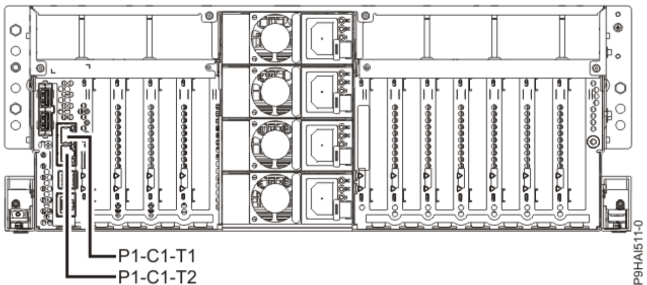
Figura 27. Ubicaciones de los puertos de la HMC en el modelo 9009-41A, 9009-41G, 9009-42A, 9009-42G, 9223-42H y 9223-42S
