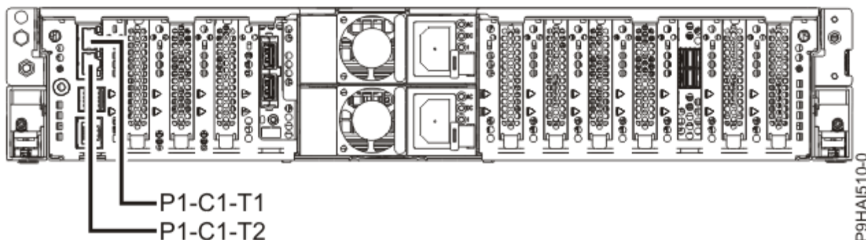
Figura 26. Ubicaciones de los puertos de la HMC en el modelo 5105-22E, 9008-22L, 9009-22A, 9009-22G, 9223-22H y 9223-22S
