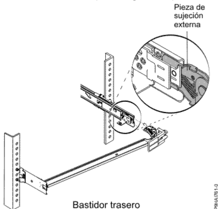
Figura 19. Conexión de la pieza de sujeción de tope al riel deslizante
