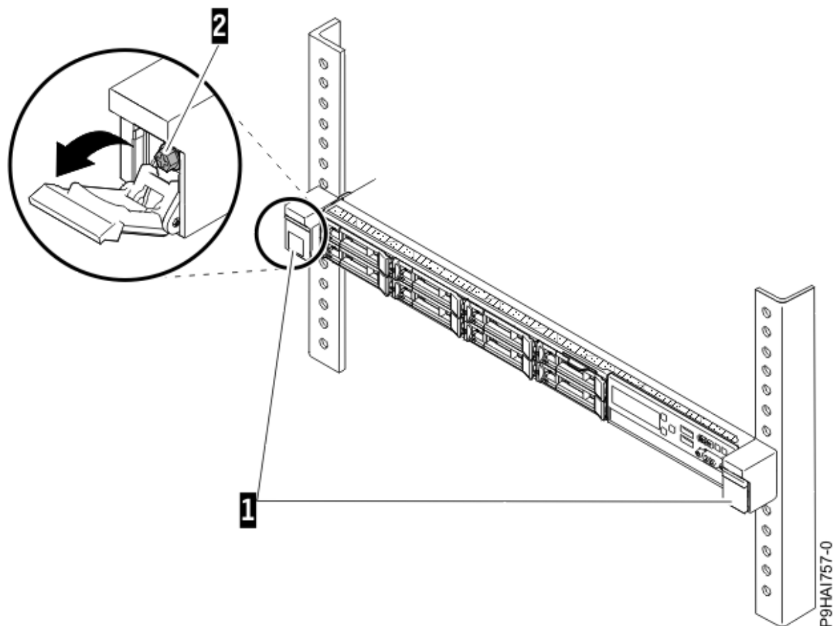
Figura 15. Riel frontal del bastidor y patillas
