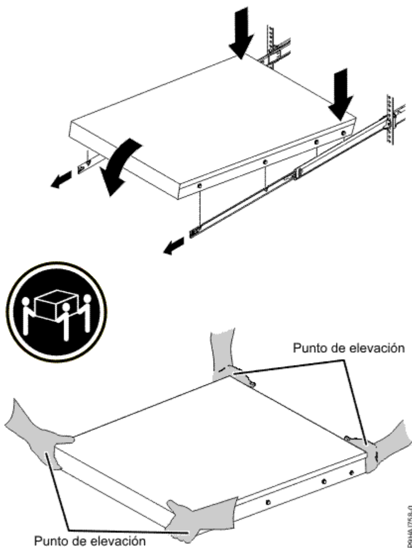
Figura 16. Rieles deslizantes extendidos, cabezas de clavo de servidor alineadas con ranuras en el riel y puntos de elevación
