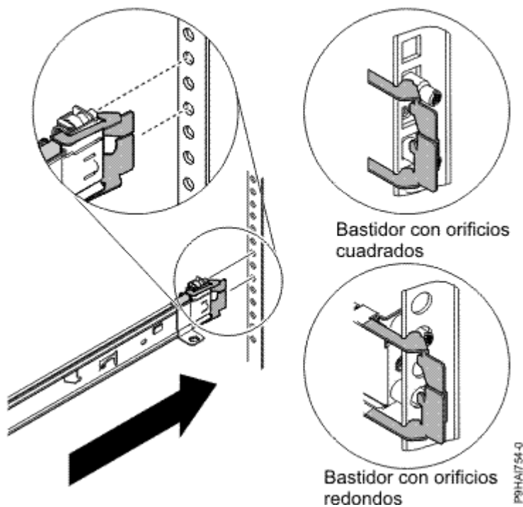
Figura 13. Alinear las patillas con los orificios de la parte posterior del bastidor
