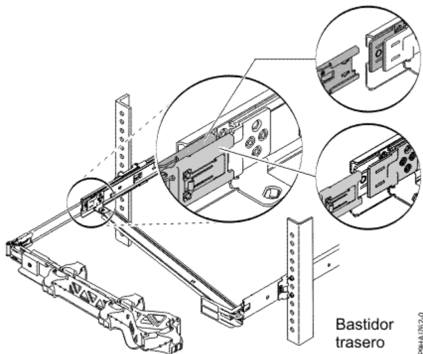
Figura 20. Conexión de brazo portacables
