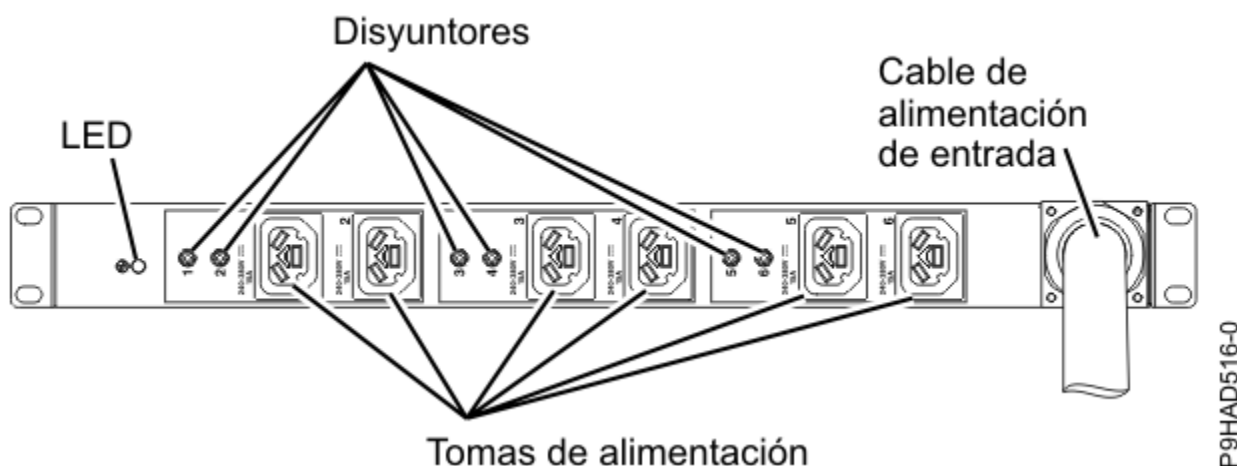
Figura 42. PDU HVDC
