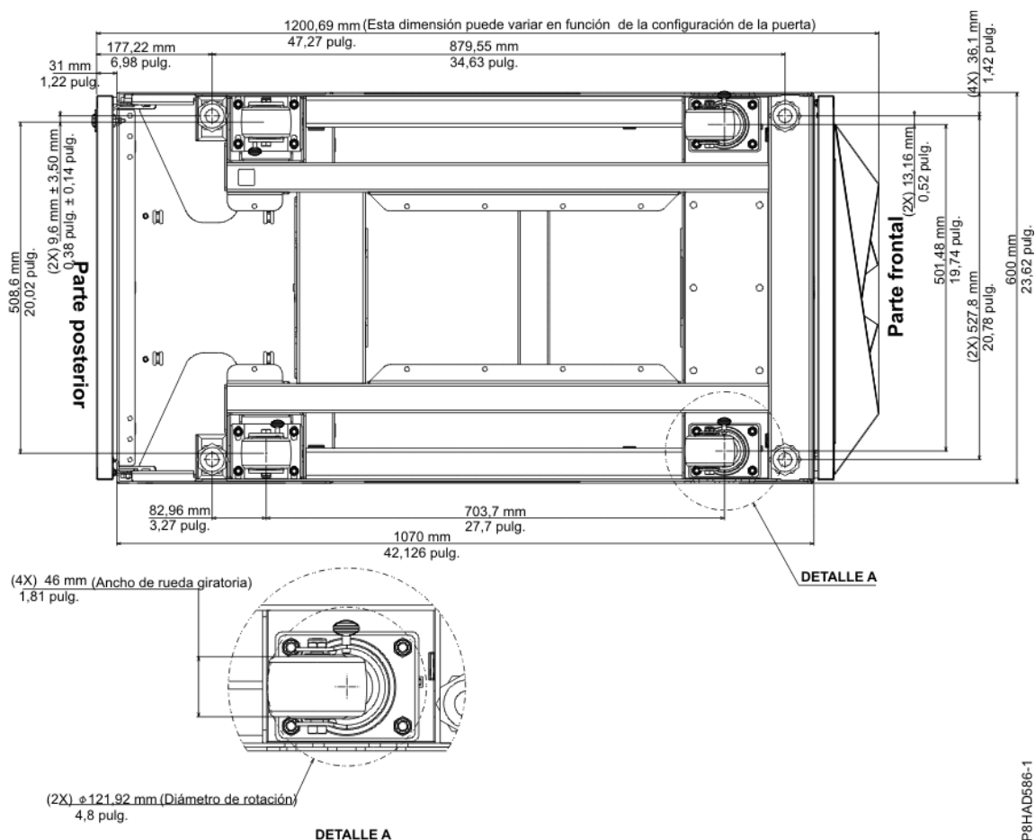
Figura 14. Ubicaciones de ruedas giratorias y niveladores
