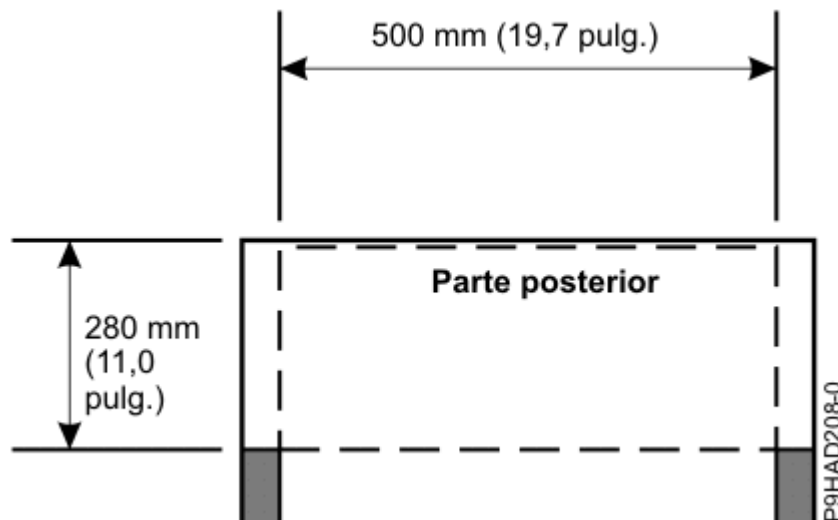
Figura 36. Espacio libre posterior del bastidor del modelo 9080-M9S (instalación de pieza de sujeción de bastidor estrecha)
