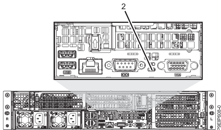
Figura 64. LED en la parte posterior del sistema
