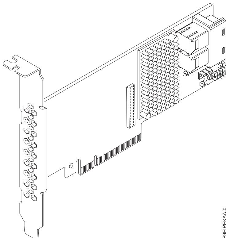
Figura 42. Controlador SAS3 Broadcom (LSI) MegaRAID 9361-8i con 8 puertos internos (1 GB de memoria caché) PCIe3.0 x8 LP con cables
