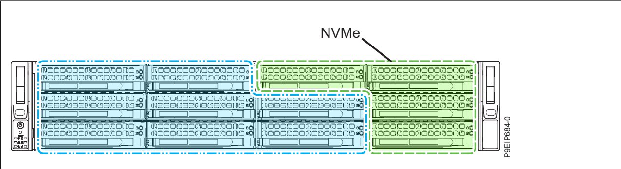
Figura 4. Hasta 8 unidades SAS o SATA, o una combinación de HDD SAS y HDD SATA (ocho unidades en total), cuatro unidades NVMe conectadas a un adaptador NVMe, y hasta dos DOM
