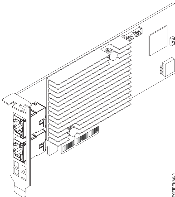
Figura 25. Adaptador de red convergido PCIe3 x4 Intel x550 10GBase-T con puertos duales RJ45
