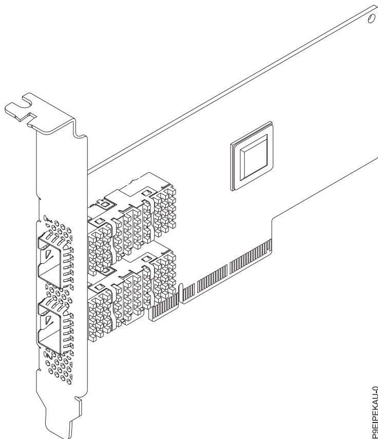
Figura 39. Adaptador Adaptador SFP28 PCIe3.0 x8 LP de puerto dual y 25 GbE Mellanox MCX4121A-ACAT ConnectX-4 Lx EN
