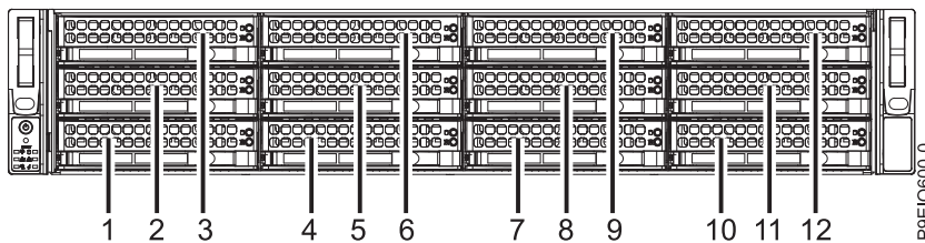
Figura 10. Unidades NVMe en las ubicaciones de 9 a 12
