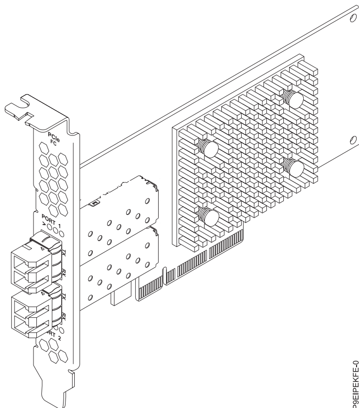
Figura 46. Adaptador de canal de fibra PCIe3 x8 LP QLogic QLE2742 de 2 puertos y 32 Gb
