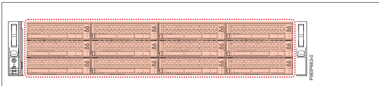
Figura 6. Hasta 12 unidades SAS o SATA, o una combinación de HDD SAS y SSD SATA (12 unidades en total), adaptador SAS/SATA y hasta dos DOM
