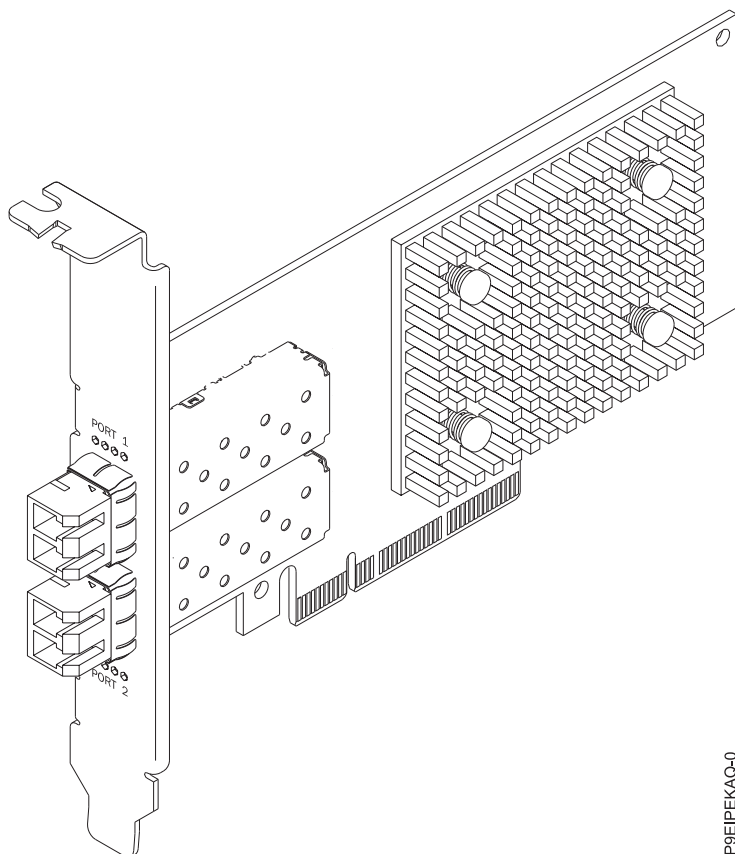
Figura 37. Adaptador de canal de fibra PCIe3 x8 LP Qlogic QLE2692OP de puerto dual y 16 Gb
