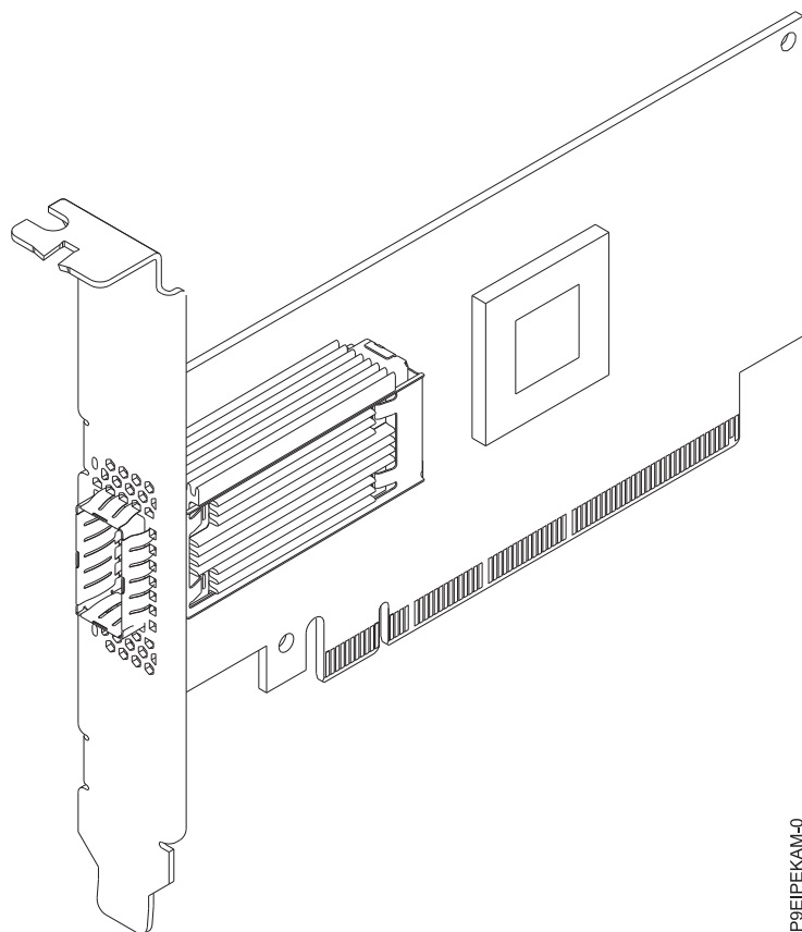
Figura 35. Adaptador QSFP28 PCIe3.0 x16 LP de un puerto y 100 GbE Mellanox MCX415A-CCAT ConnectX-4 EN
