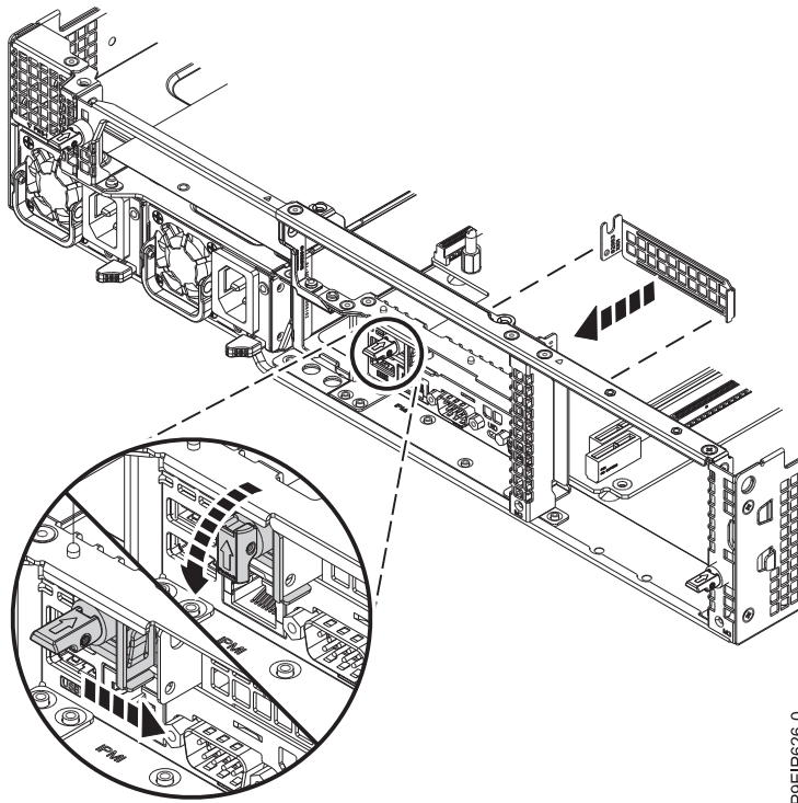
Figura 59. Deslizamiento del retén de contrapunta a la posición de cerrado
