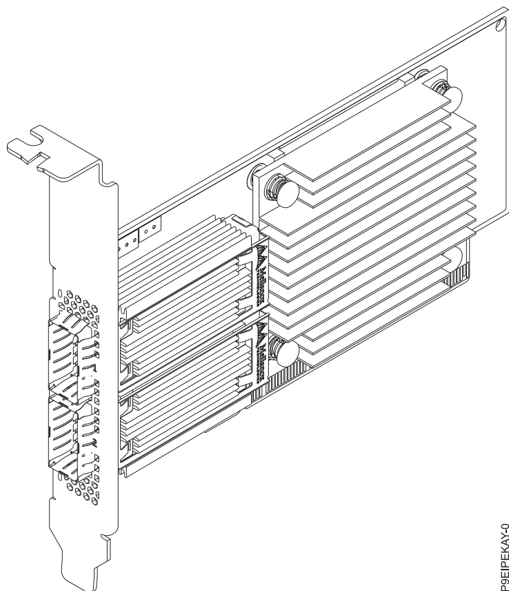
Figura 41. Adaptador Adaptador QSFP28 PCIe4.0 x16 LP de puerto dual y VPI EDR InfiniBand 100 Gb/s y 100 GbE Mellanox MCX556A-EDAT ConnectX-5
