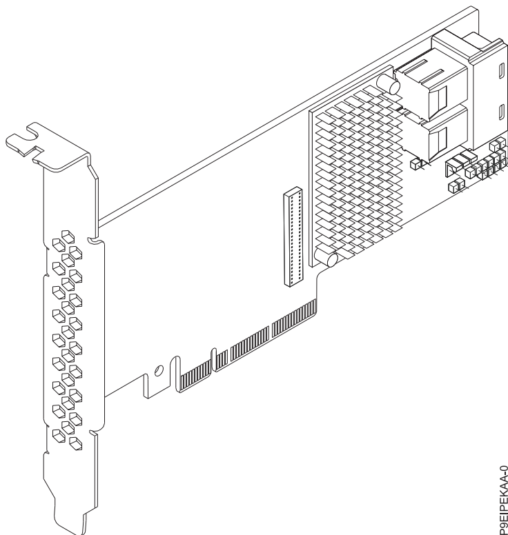
Figura 29. Controlador SAS3 Broadcom (LSI) MegaRAID 9361-8i con 8 puertos internos (1 GB de memoria caché) PCIe3.0 x8 LP con cables
