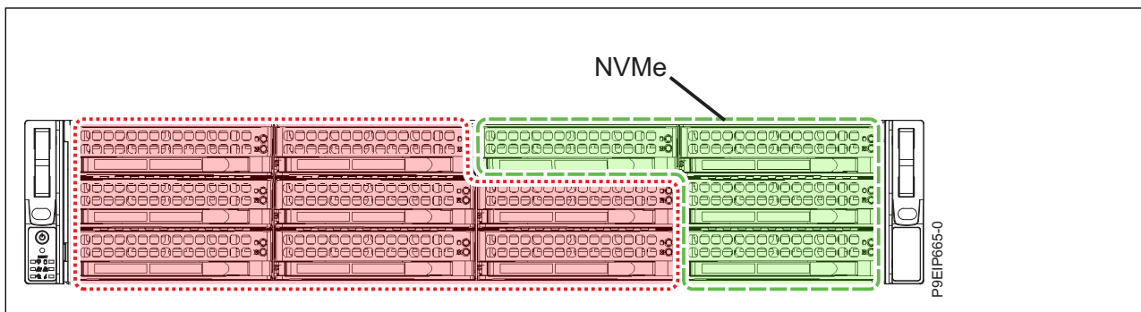
Figura 8. Hasta ocho unidades SAS o SATA, o una combinación de HDD SAS y SSD SATA (ocho unidades en total), adaptador SAS/SATA, cuatro unidades NVMe conectadas a un adaptador NVMe, y hasta dos DOM
