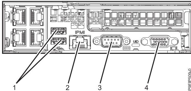
Figura 2. Puertos posteriores
