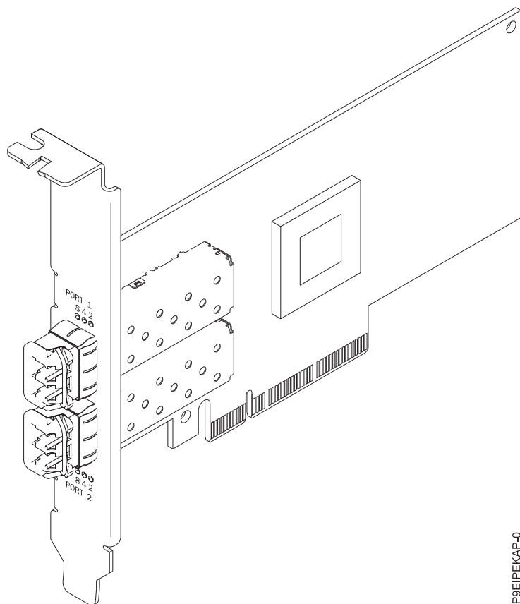
Figura 36. Adaptador Adaptador QSFP28 PCIe3.0 x16 LP de un puerto y 100 GbE Mellanox MCX415A-CCAT ConnectX-4 EN
