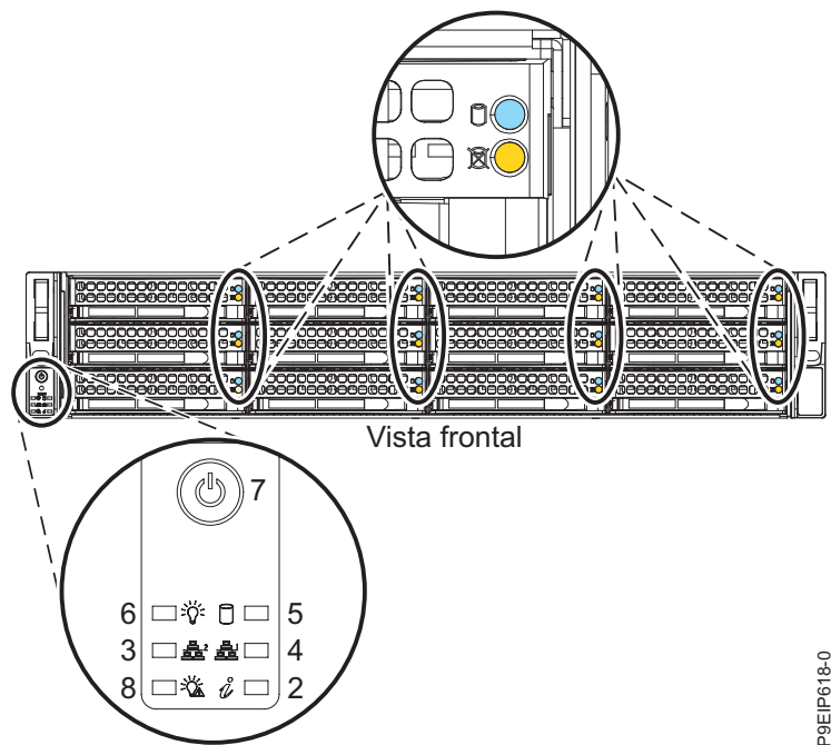
Figura 63. LED en la parte frontal del sistema
