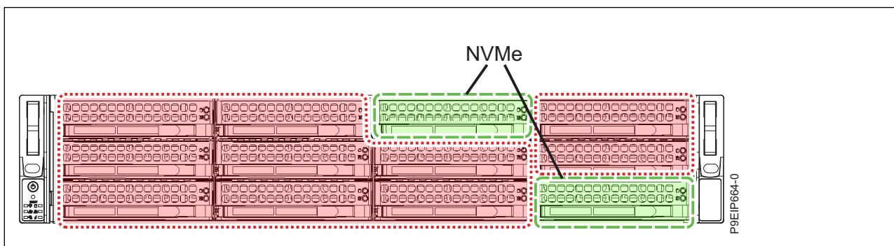
Figura 7. Hasta 10 unidades SAS o SATA, o una combinación de HDD SAS y SSD SATA (10 unidades en total), adaptador SAS/SATA, dos unidades NVMe conectadas a un adaptador NVMe, y hasta dos DOM
