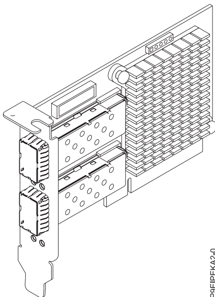
Figura 27. Intel 82599ES Ethernet x520-DA2 con puerto dual y 10G/1G SFP+
