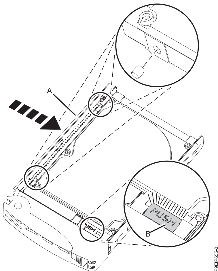
Figura 18. Cierre de la bandeja de la unidad posterior
