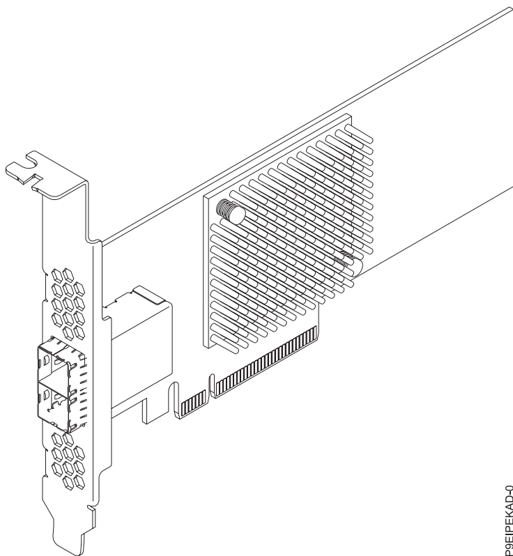
Figura 44. Adaptador SAS3 HBA PCIe3.0 x8 LP Broadcom (LSI) 9300-8E
