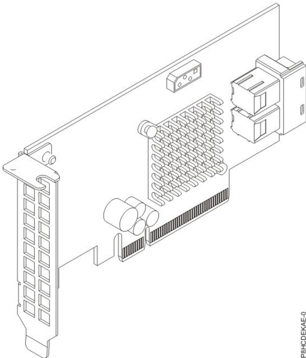
Figura 33. Controlador SAS3 Broadcom (LSI) MegaRAID 9361-8i SAS3 con 8 puertos internos (2 GB de memoria caché) PCIe3.0 x8 con cables
