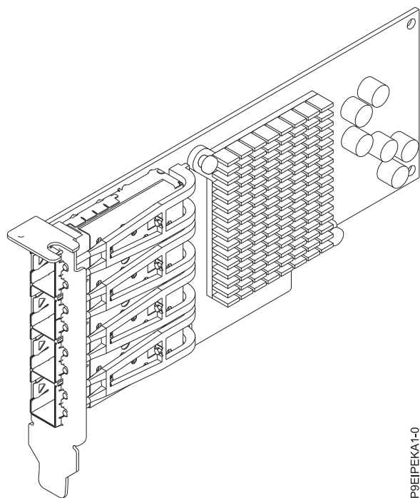
Figura 26. Adaptador Ethernet Cavium (Qlogic) BCM57840 PCIe3.0 x8 LP de m4 puertos SFP+ y 10 Gb
