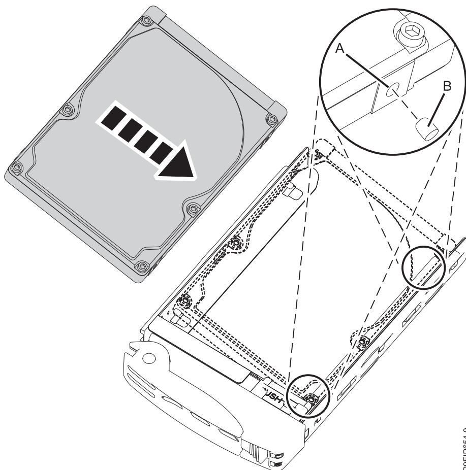
Figura 17. Inserción de la unidad posterior en la bandeja
