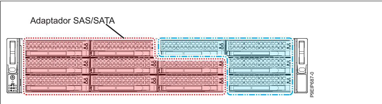
Figura 5. Hasta ocho unidades SAS o SATA conectadas a un adaptador SAS/SATA, hasta cuatro unidades SAS o SATA conectadas a un controlador integrado y hasta dos DOM
