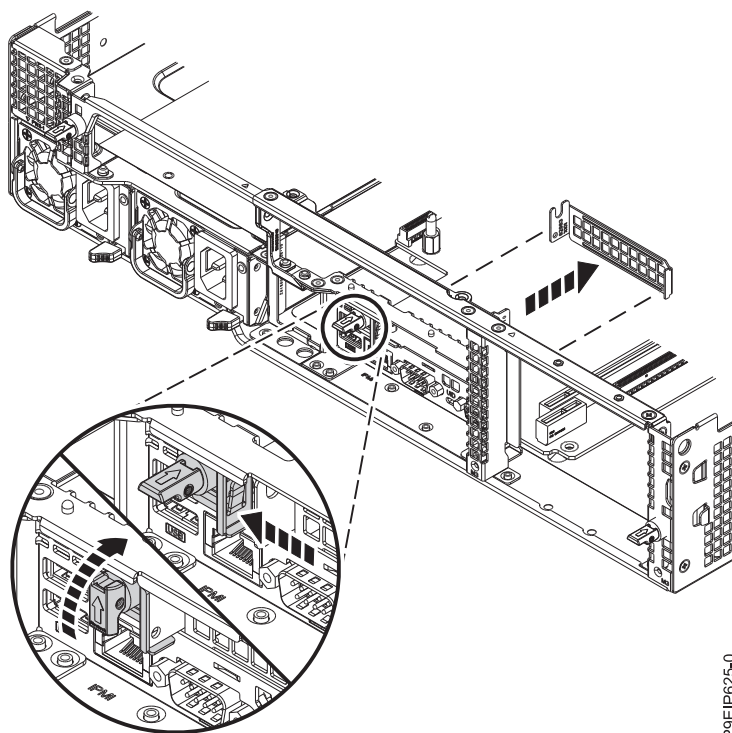
Figura 58. Liberación de la contrapunta
