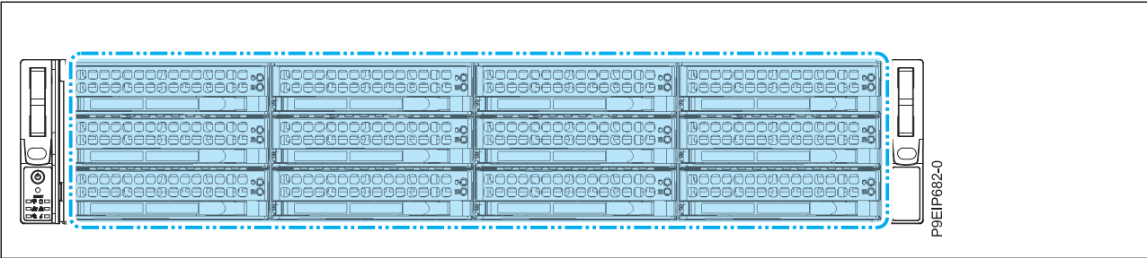
Figura 3. Hasta 12 unidades SAS o SATA y hasta dos DOM
