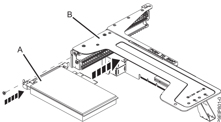
Figura 56. Inserción de un adaptador en la posición 2 de la tarjeta de expansión PCIe
