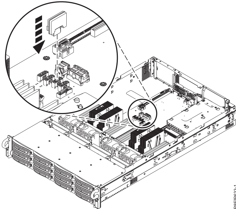
Figura 20. Instalación de una DOM
