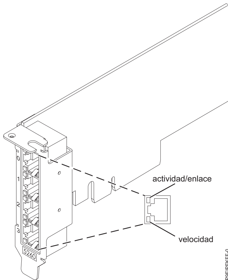
Figura 47. PCIe x4 LP de tarjeta de interfaz de red de Broadcom 5719 QP 1G (1G/100M/10M)
