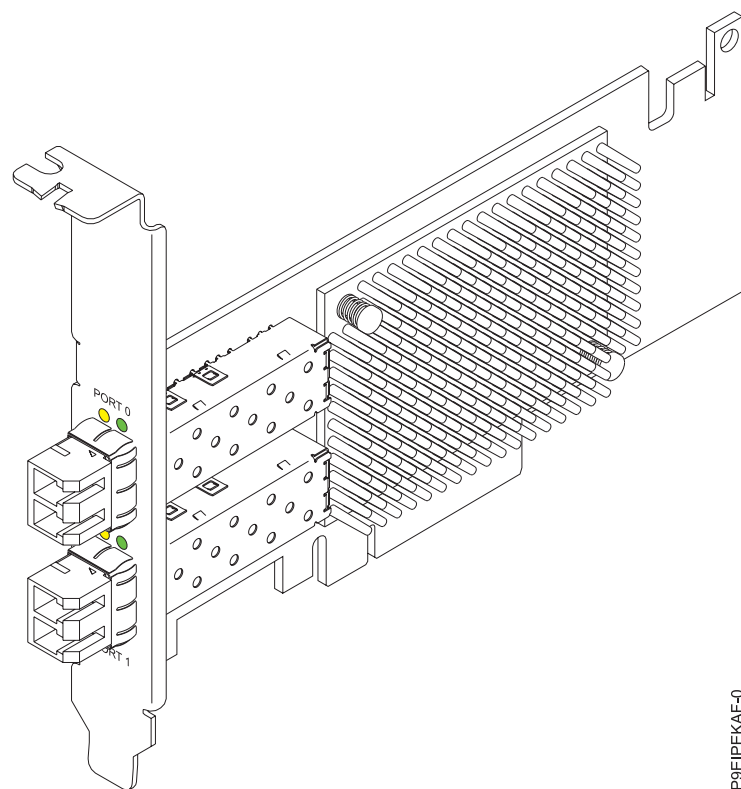
Figura 31. Tarjeta de canal de fibra PCIe3.0 x8 LP Emulex LPE16002B-M6-O de puerto dual y 16 Gb
