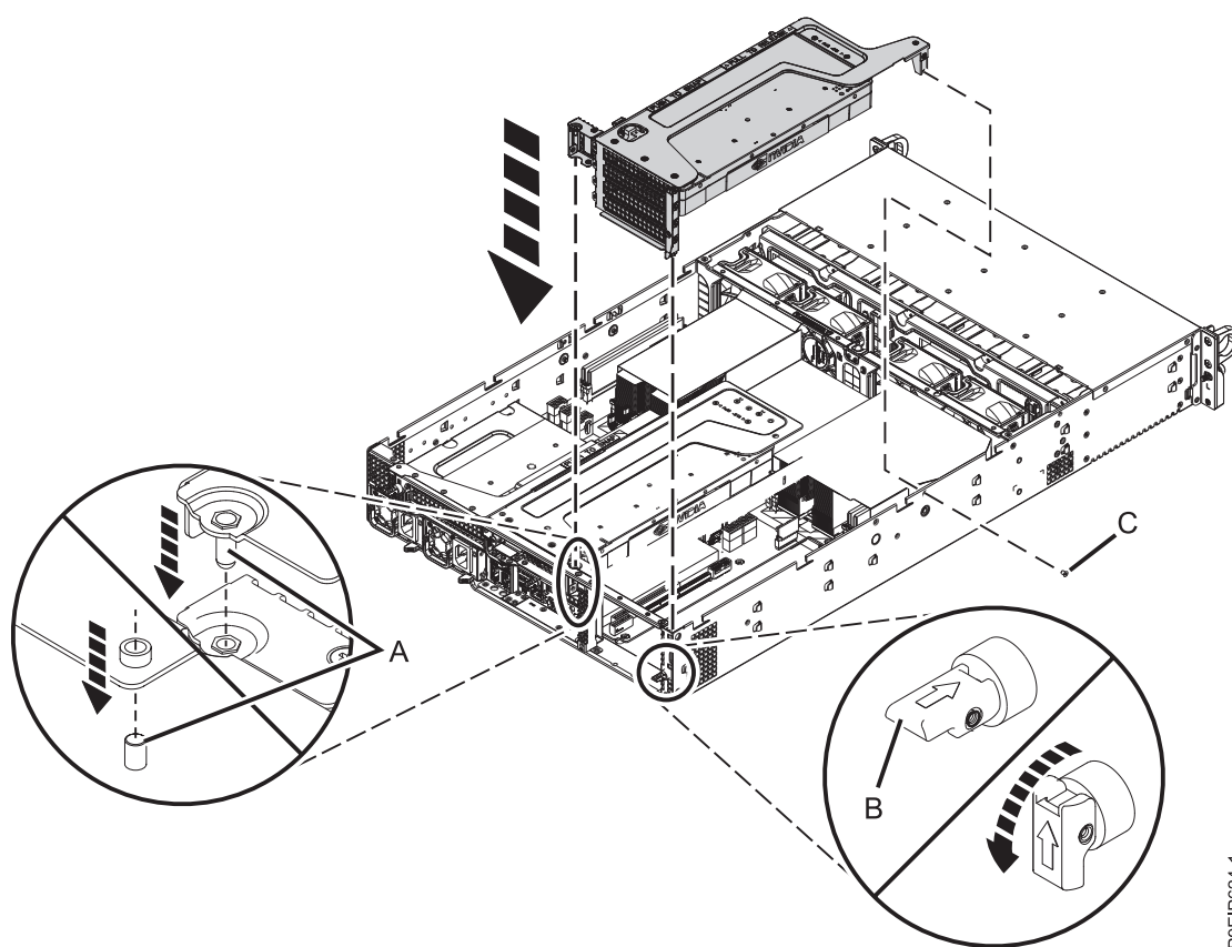
Figura 62. Inserción de la tarjeta de expansión del adaptador PCIe
