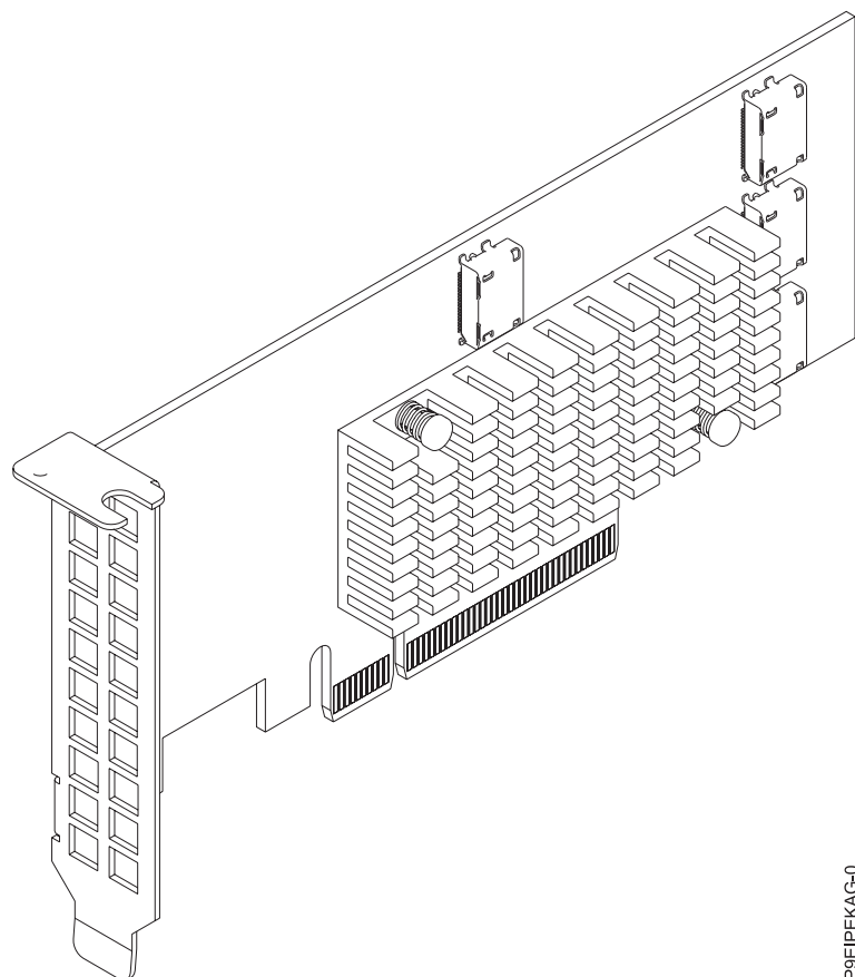
Figura 32. Adaptador de bus de host NVMe cuatripuerto SMC (PEX9733) PCIe3.0 x8 LP con cables
