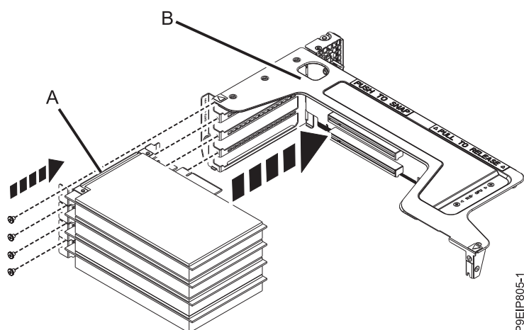
Figura 61. Inserción de un adaptador PCIe en la tarjeta de expansión
