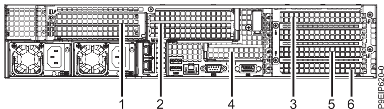
Figura 24. Vista posterior de un sistema 9006-22P con las ranuras PCIe indicadas
