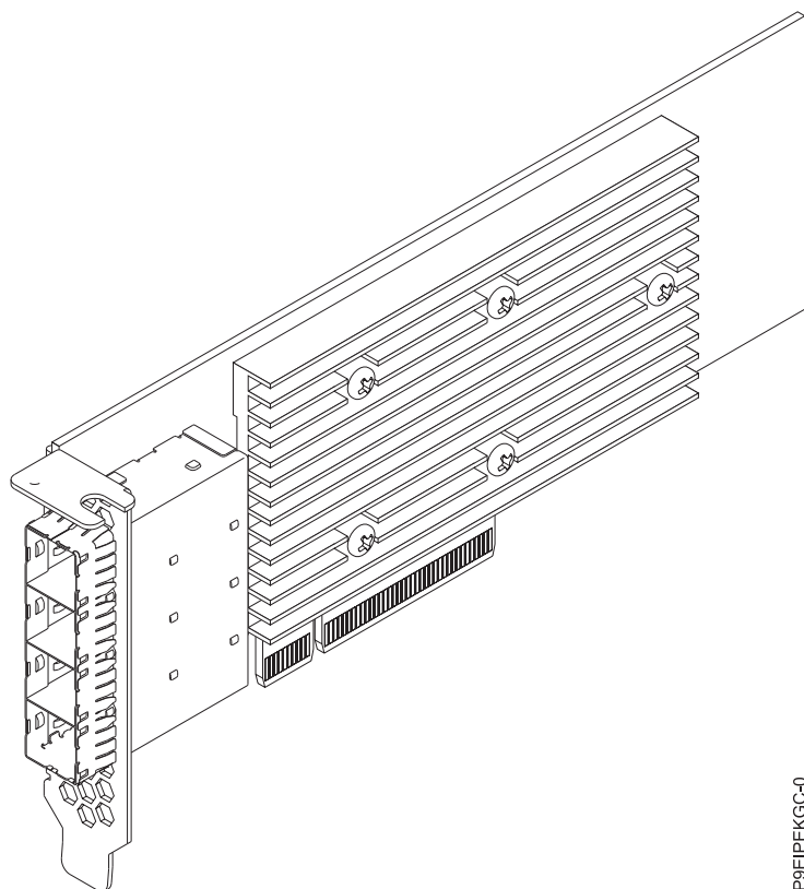
Figura 50. Adaptador PCIe3.0 x8 LP Broadcom (LSI) 9305-16E SAS3 HBA
