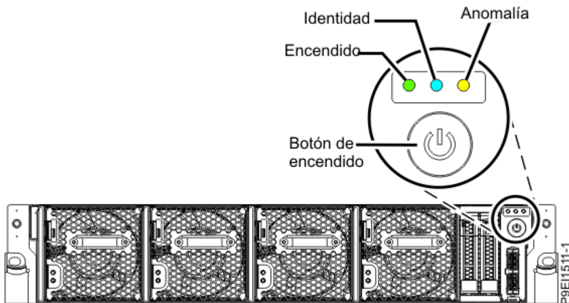
Figura 40. Botón de encendido
