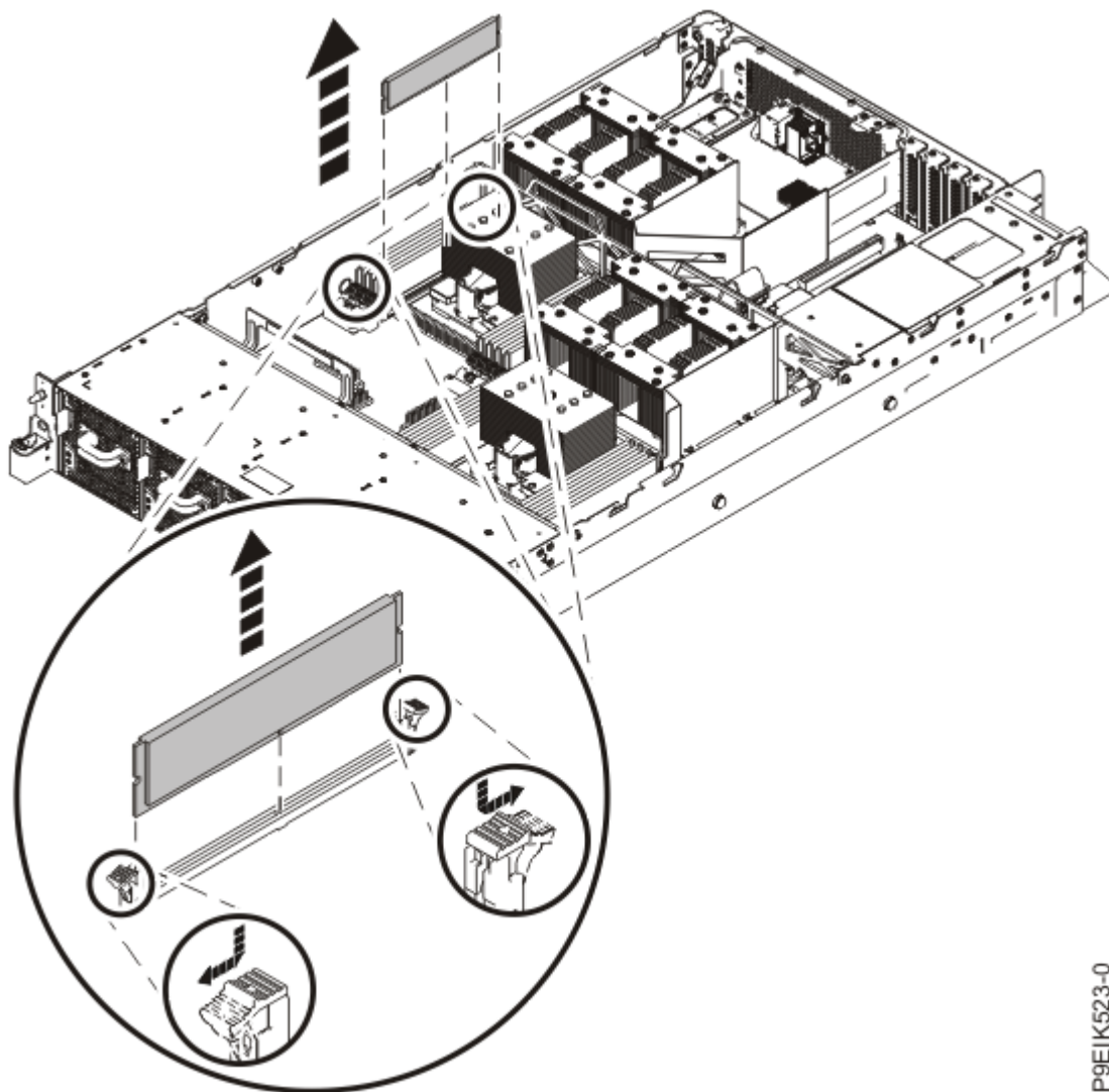
Figura 9. Extracción de los módulos de memoria
