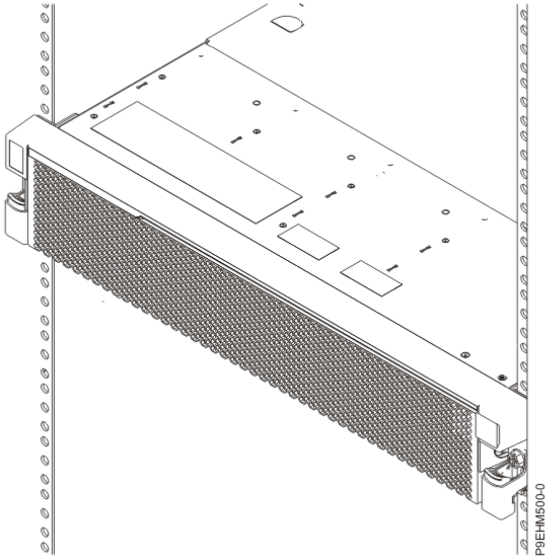
Figura 2. Instalación del servidor en el bastidor
