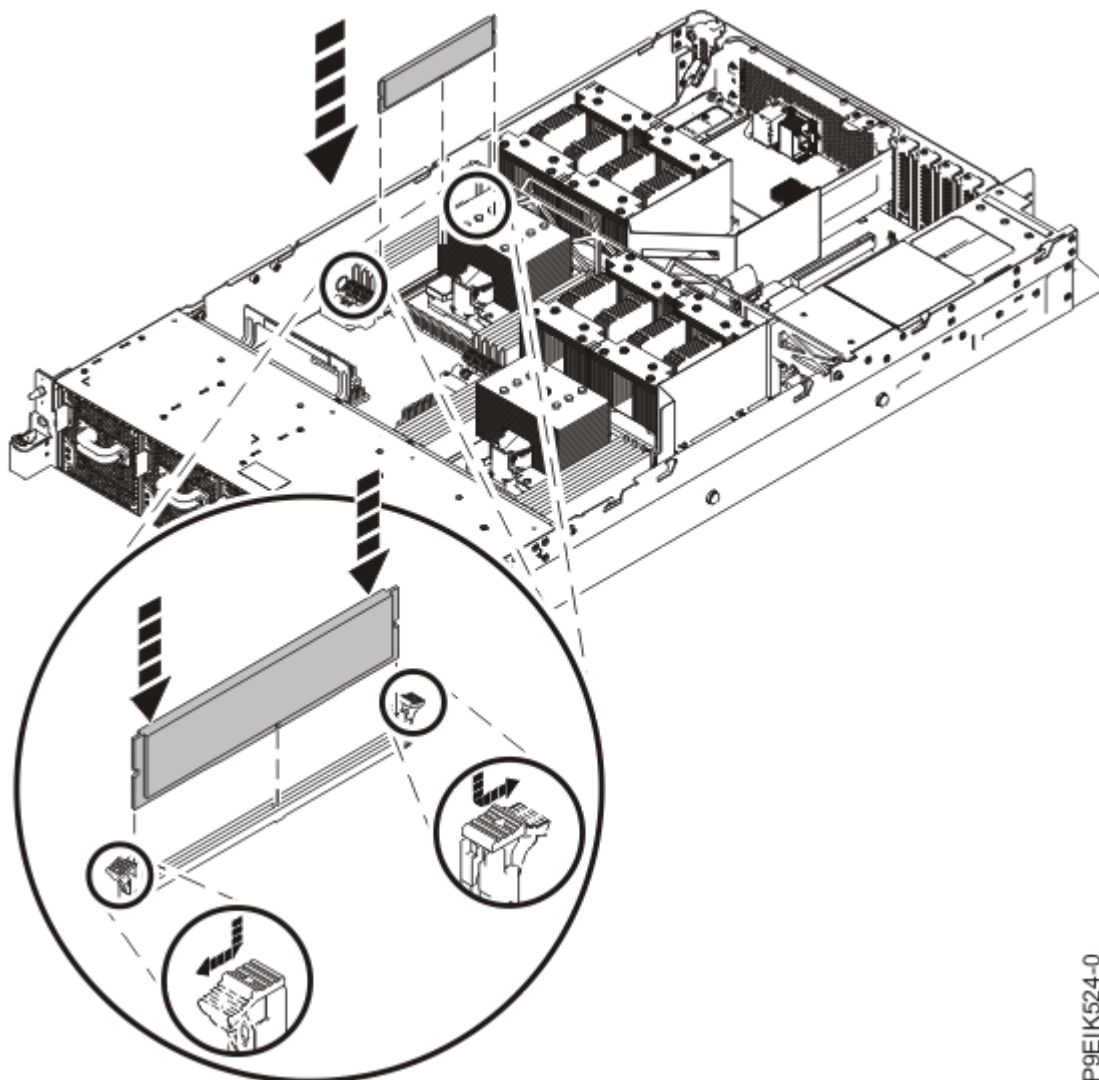
Figura 10. Instalación de módulos de memoria
