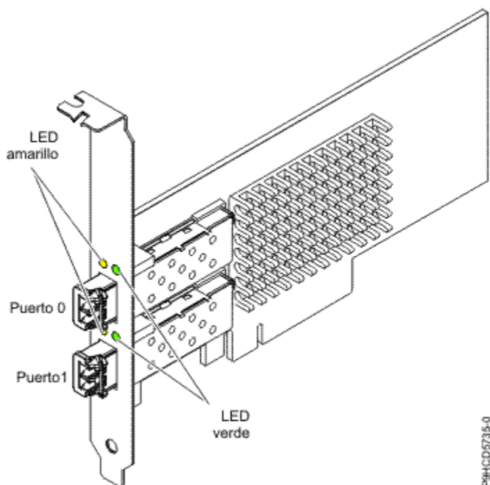
Figura 25. Adaptador de canal de fibra PCIe3 LP 16 Gb de 2 puertos
