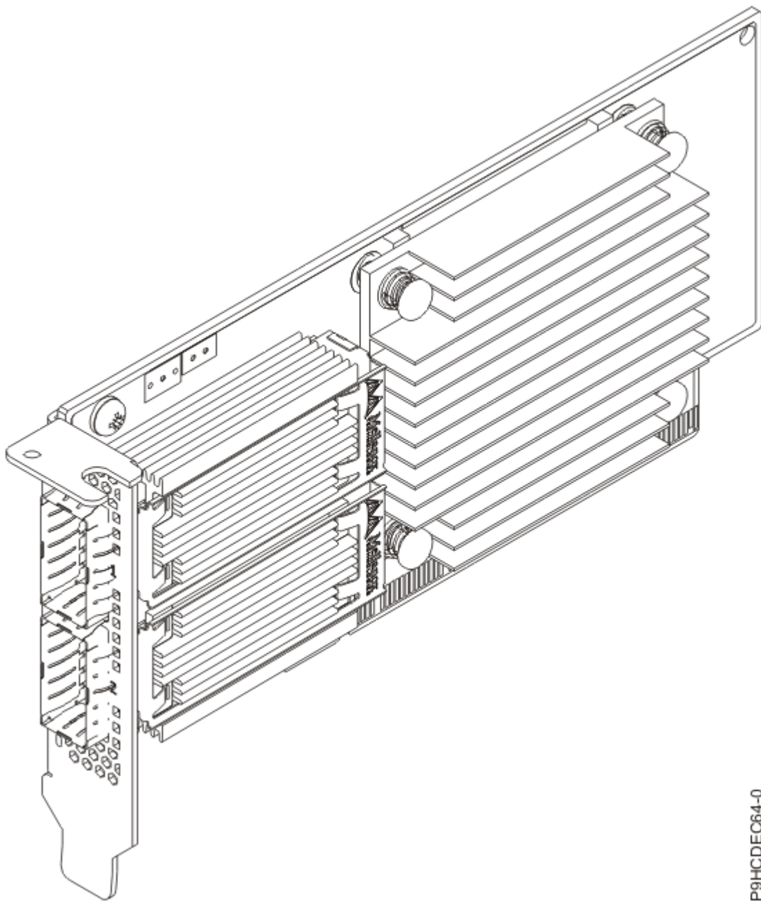
Figura 22. Adaptador PCIe4 x16 de 2 puertos EDR 100 GB IB ConnectX-5 compatible con CAPI
