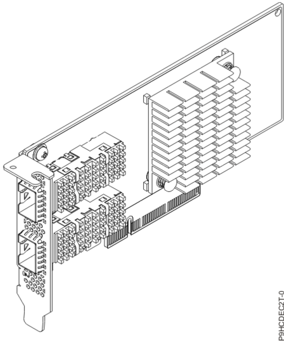
Figura 15. Adaptador PCIe3 LP de 2 puertos 25/10 Gb NIC y ROCE SFP28 (FC EC2T)
