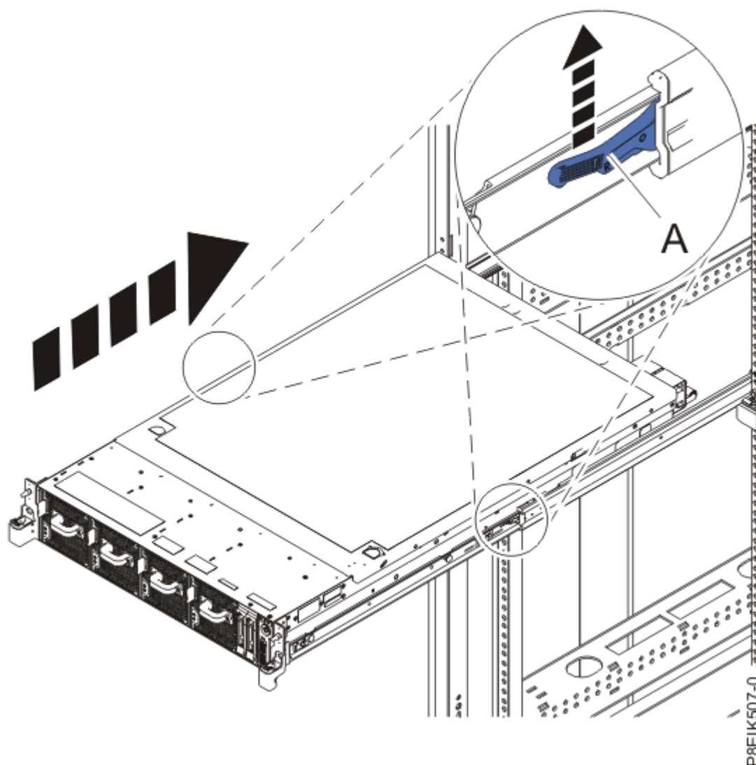
Figura 45. Colocación del sistema en la posición operativa
