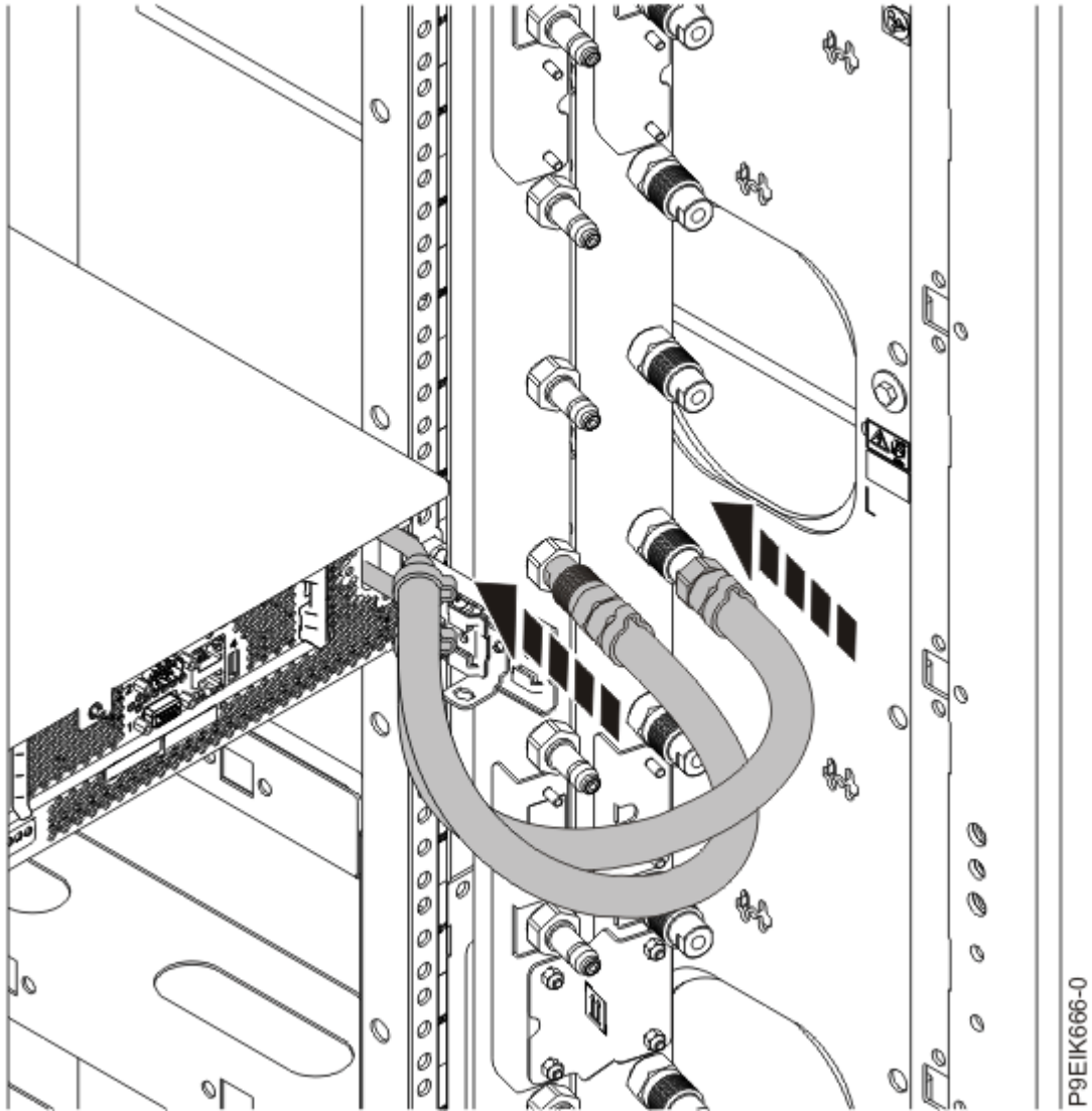
Figura 3. Conexión de las mangueras de agua
