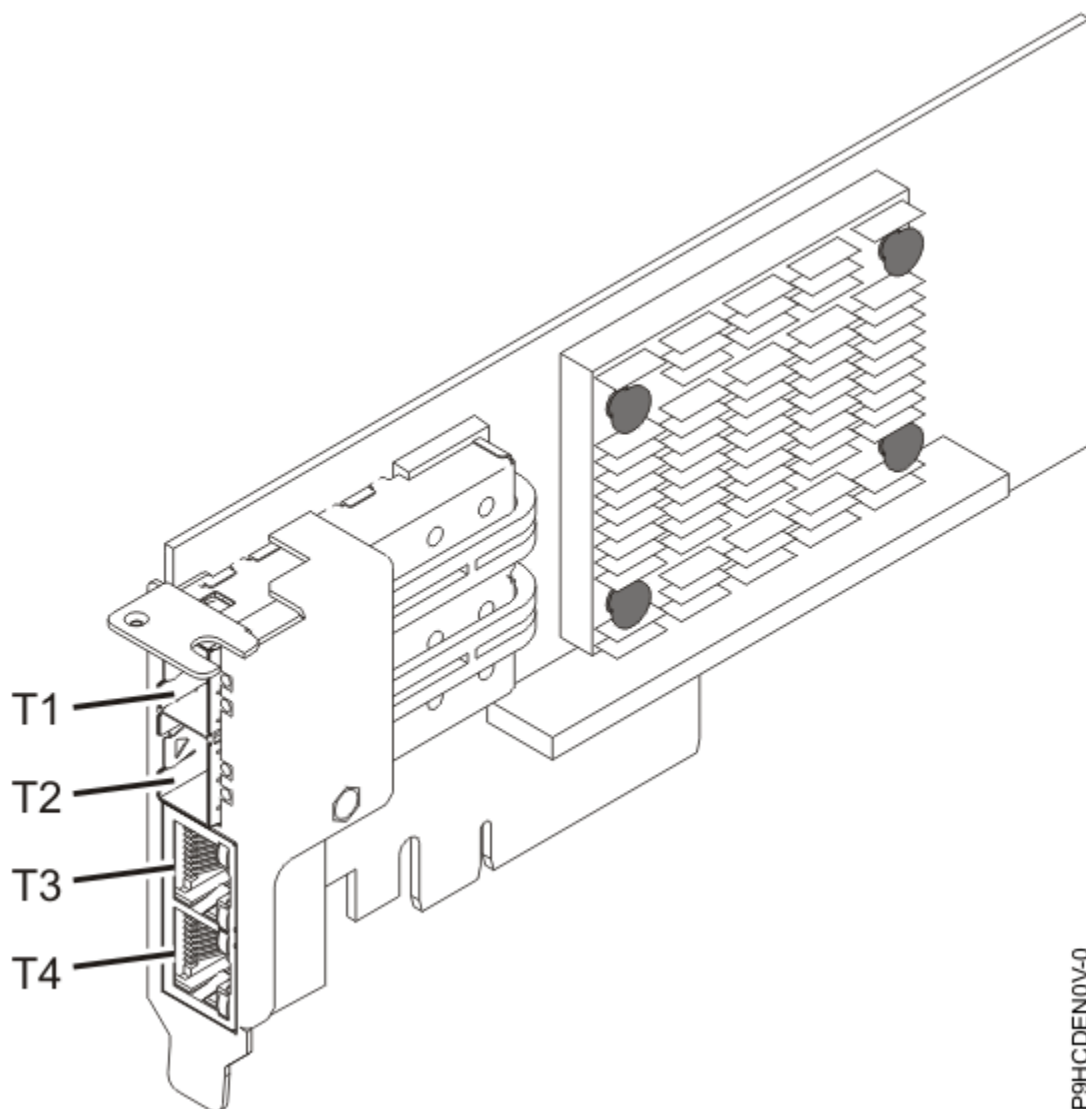
Figura 30. Adaptador de cobre SFP+RJ45 PCIe2 LP de 4 puertos (10 Gb + 1 GbE)
