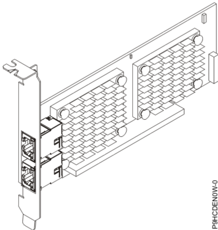
Figura 23. Adaptador PCIe2 de 2 puertos y 10 GbE BaseT RJ45 (FC EL55 o FC EN0W)
