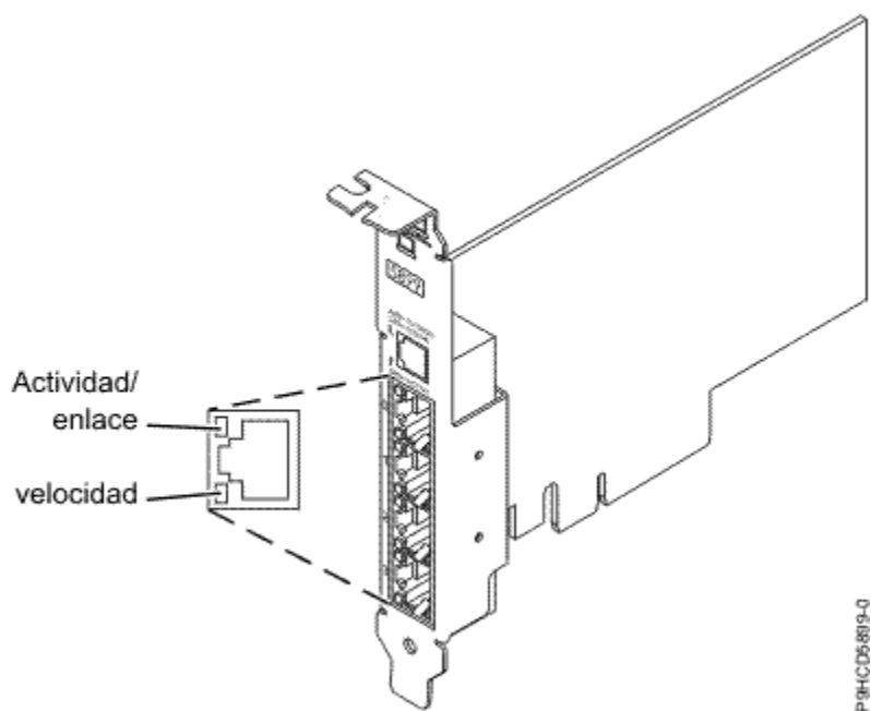
Figura 27. Adaptador PCIe2 de 4 puertos y 1 GbE FC 5899 y FC EL4L
