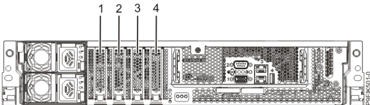
Figura 12. Vista posterior de un sistema con las ranuras PCIe indicadas
