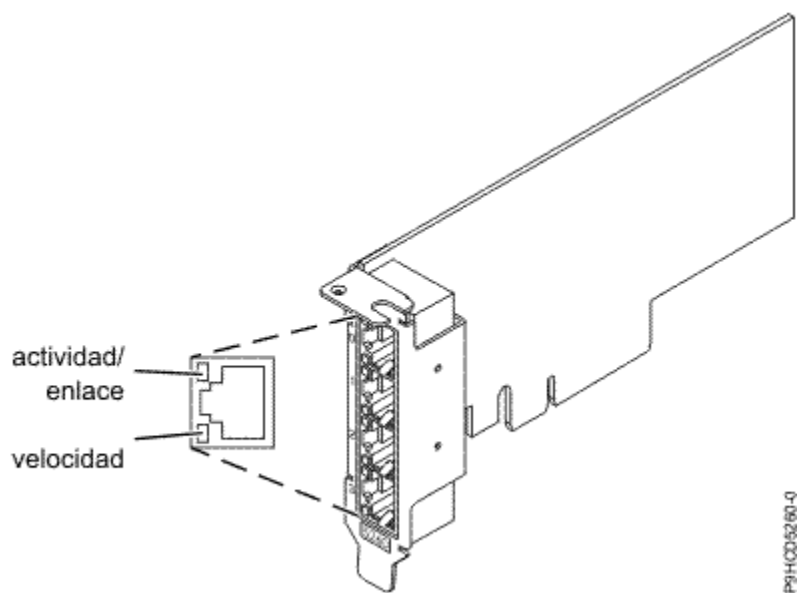
Figura 26. Adaptador PCIe2 de 4 puertos y 1 GbE FC 5260 y FC EL4M
