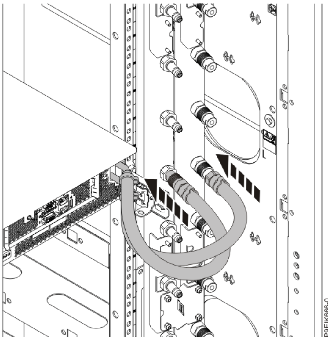
Figura 46. Conexión de las mangueras de agua
