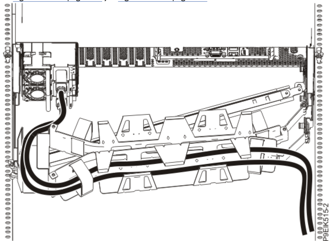
Figura 47. Enrollado del cable de alimentación en el brazo portacables
