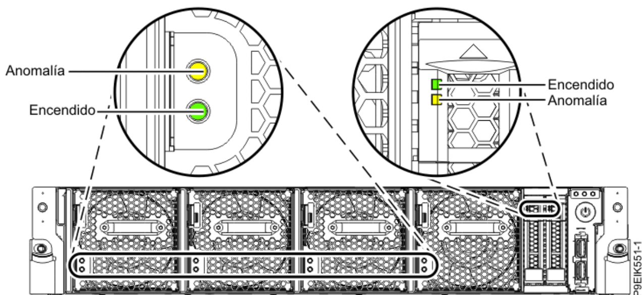
Figura 35. LED frontales con bisel apagado
