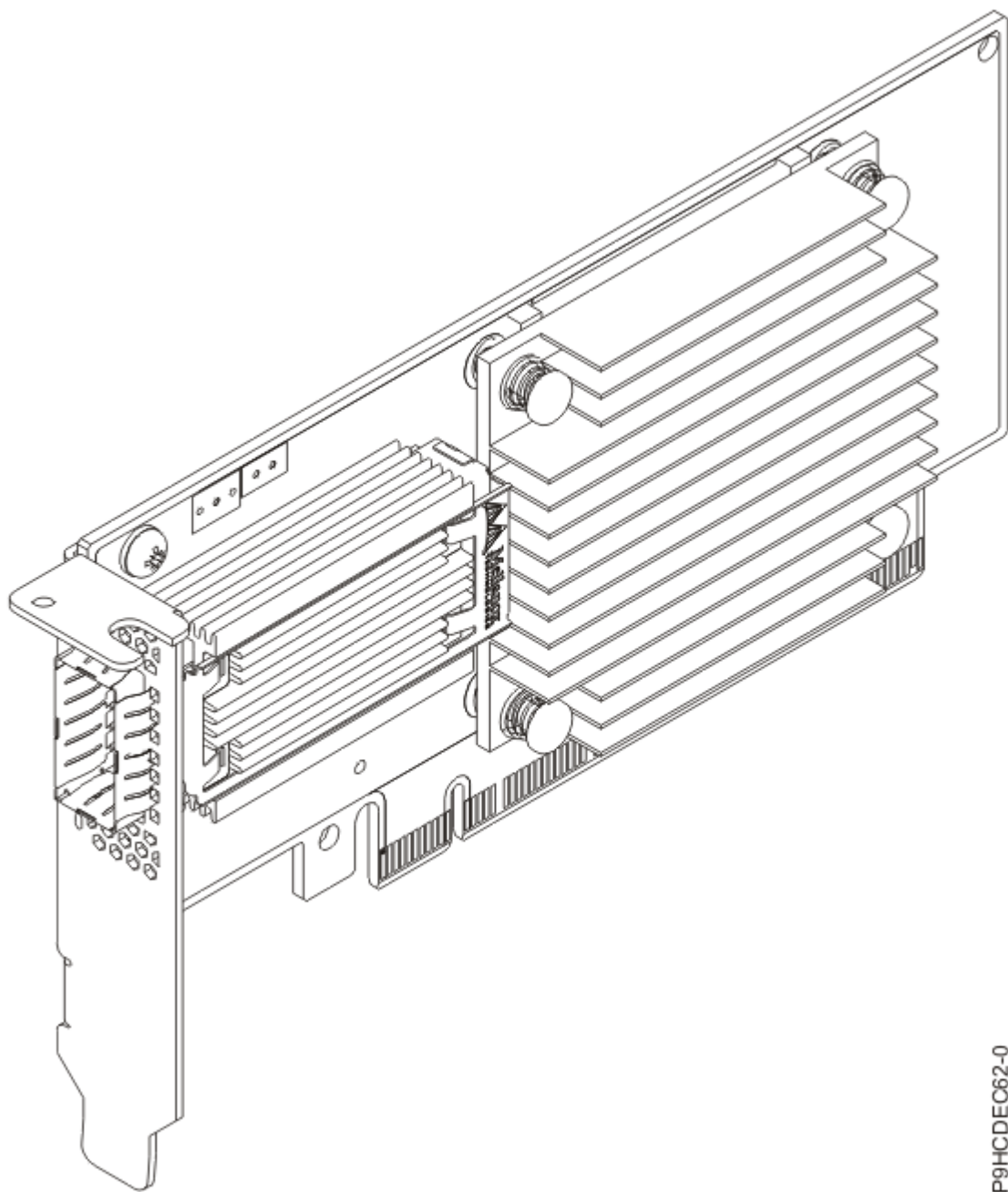
Figura 21. Adaptador PCIe4 x16 de 1 puerto EDR 100 GB IB ConnectX-5 compatible con CAPI
