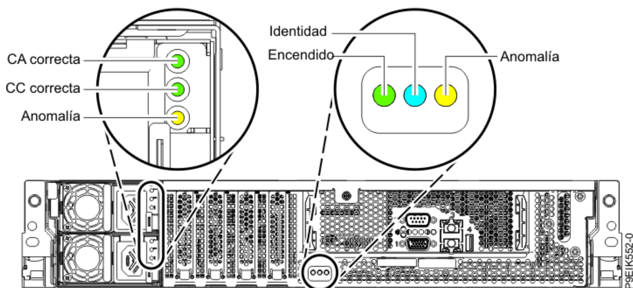
Figura 36. LED posteriores
