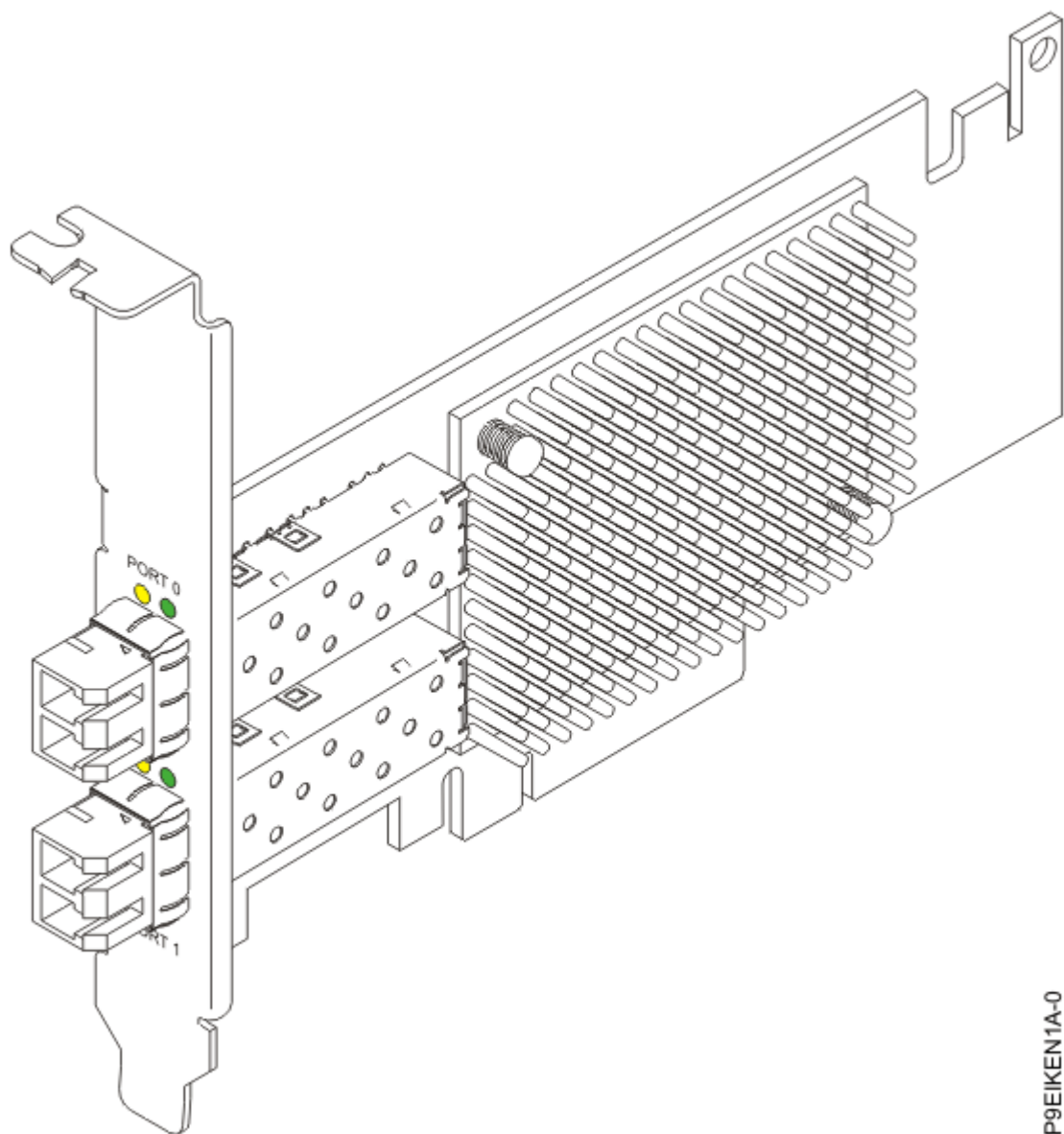
Figura 28. Adaptador de canal de fibra PCIe3 x8 de 2 puertos (32 Gb/s)
