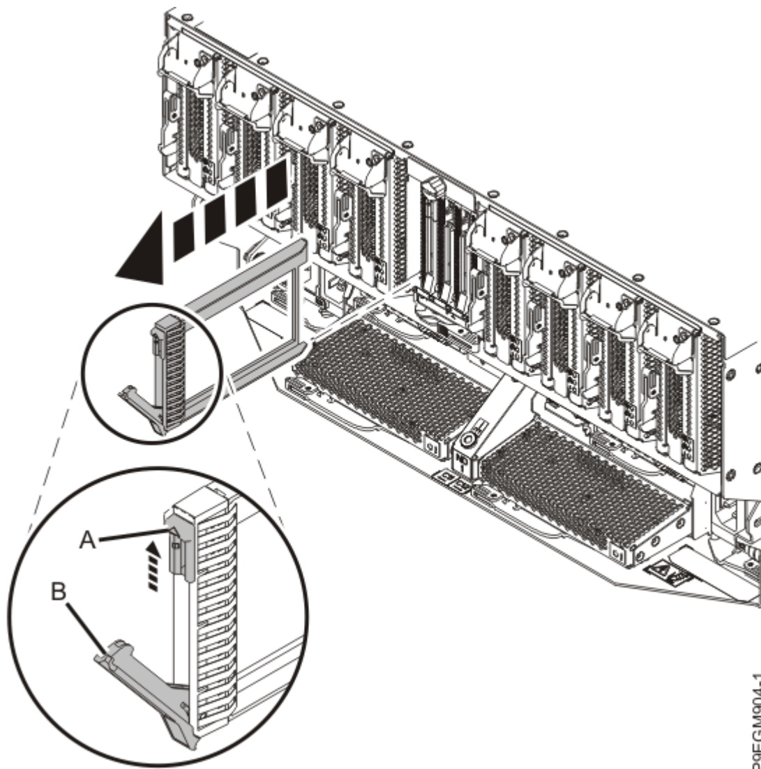
Figura 6. Extracción de una placa de relleno de la unidad NVMe del sistema 9080-M9S
