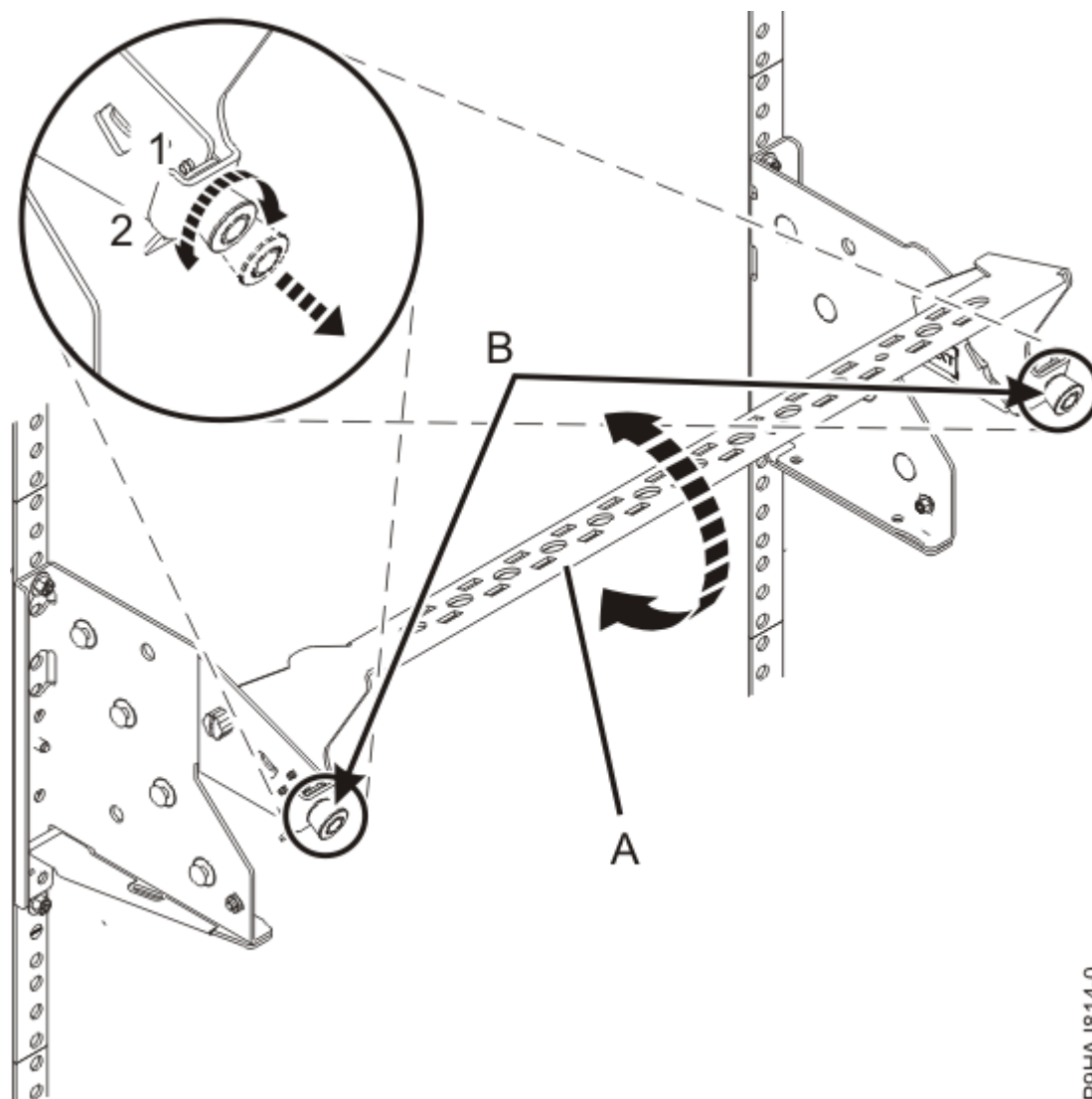
Figura 5. Colocación de la abrazadera portacables en la posición de servicio elevada
