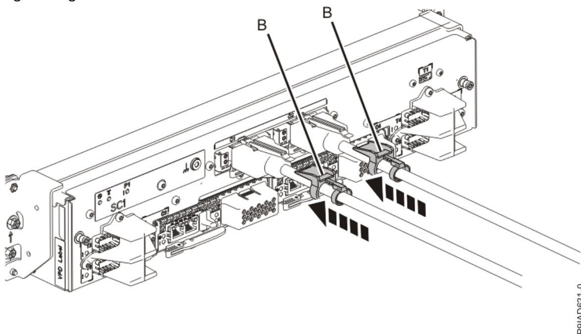
Figura 10. Sustitución del cable UPIC en la unidad de control del sistema
