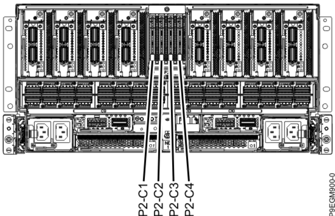
Figura 1. Ubicación de las unidades NVMe U.2 en el sistema 9080-M9S
