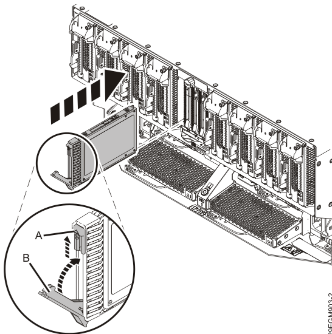
Figura 7. Instalación o colocación de una unidad NVMe U.2 en el sistema 9080-M9S
