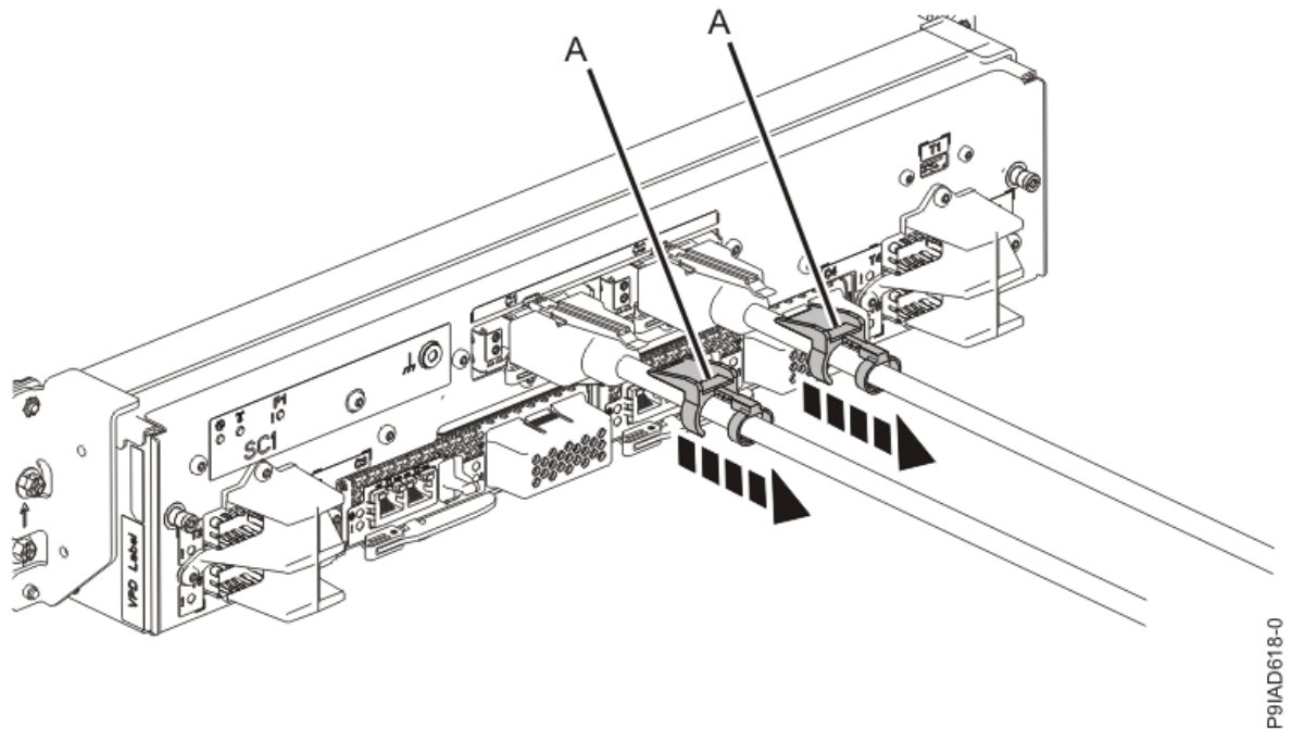
Figura 3. Extracción del cierre de cable UPIC
