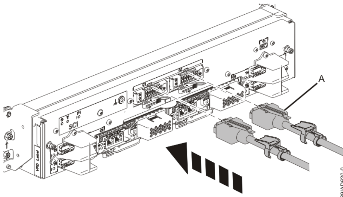
Figura 9. Sustitución del cable UPIC en la unidad de control del sistema
