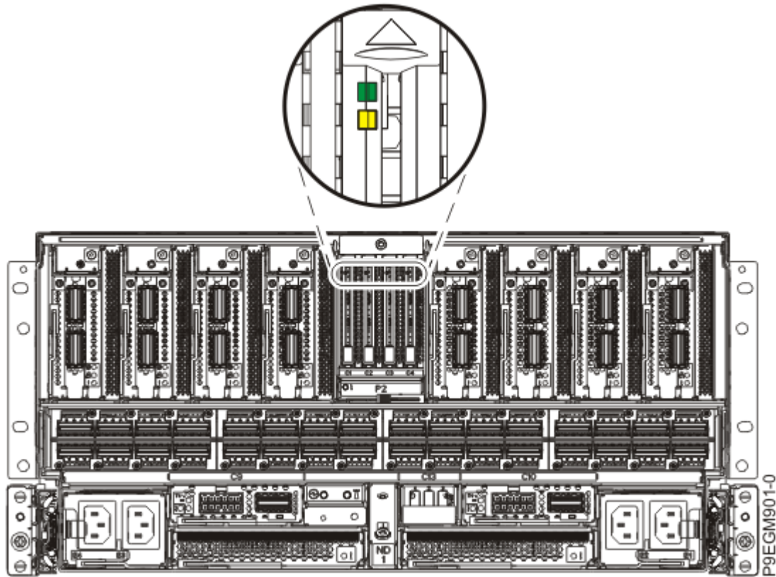
Figura 2. Ubicaciones de los LED de la unidad NVMe U.2 en el sistema 9080-M9S
