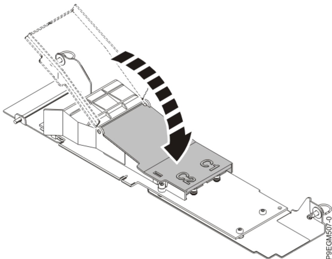
Figura 7. Cierre de la cubierta negra de la tarjeta portadora NVMe M.2
