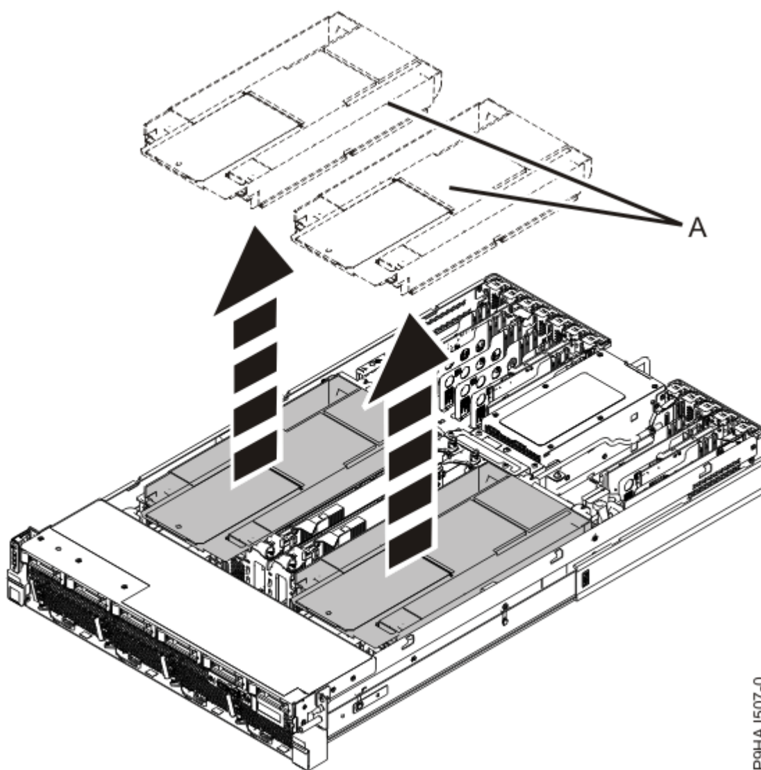
Figura 13. Extracción del deflector de aire
