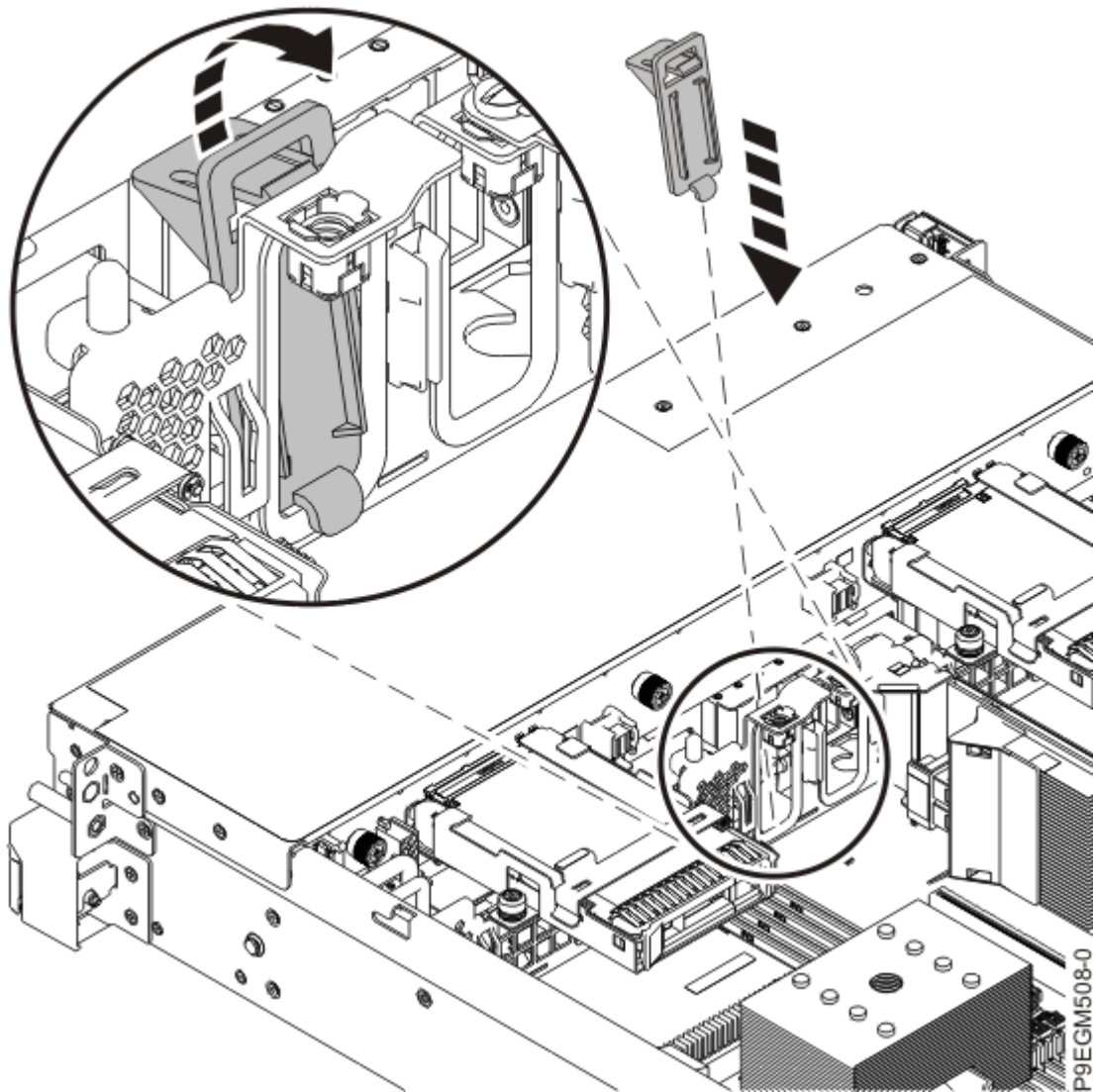
Figura 18. Instalación del relleno de fijación
