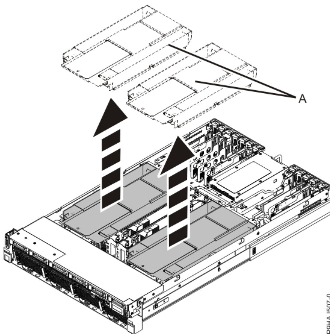
Figura 4. Extracción del deflector de aire
