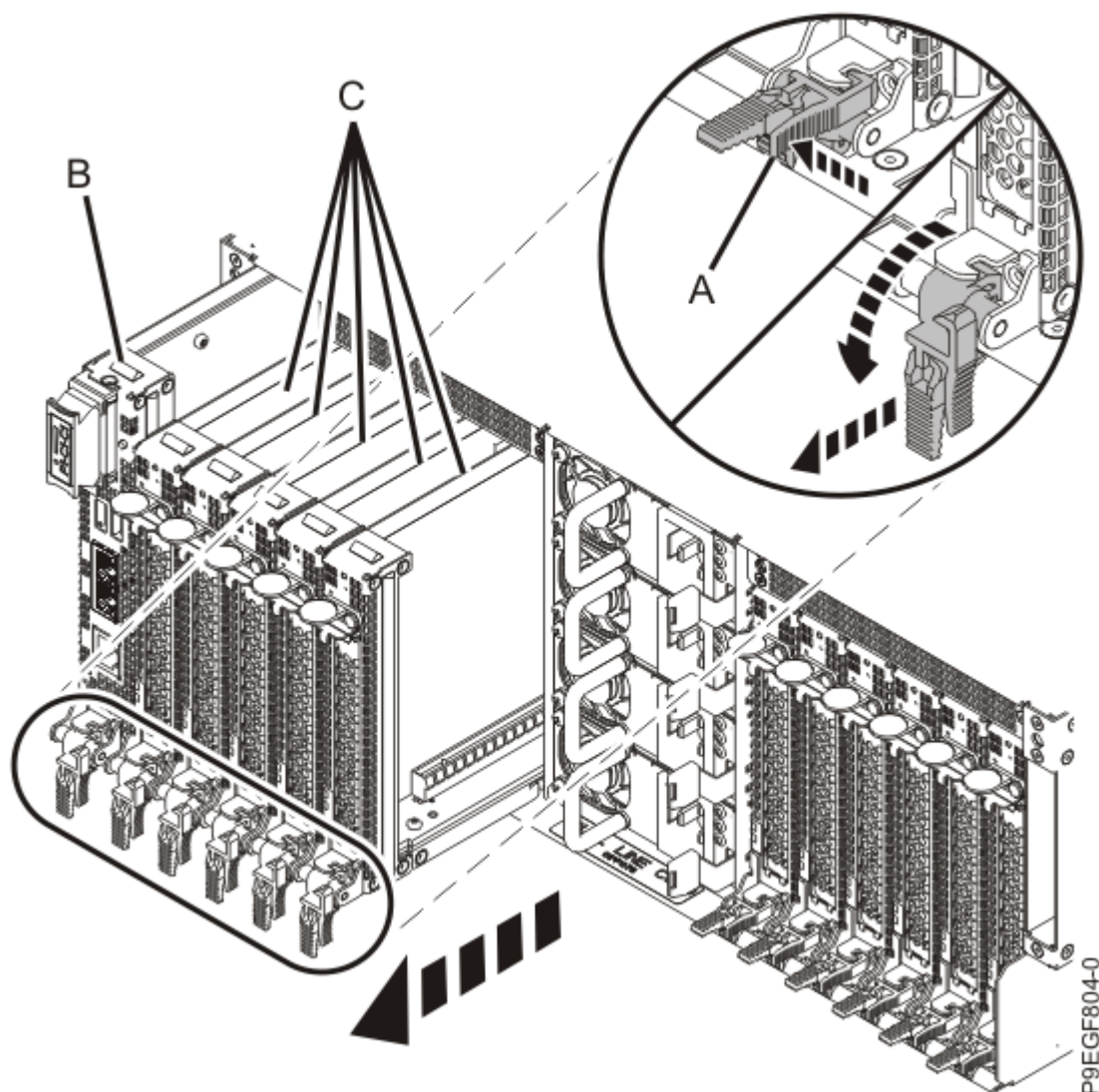
Figura 2. Extracción de la tarjeta del procesador de servicio y los casetes PCIe
