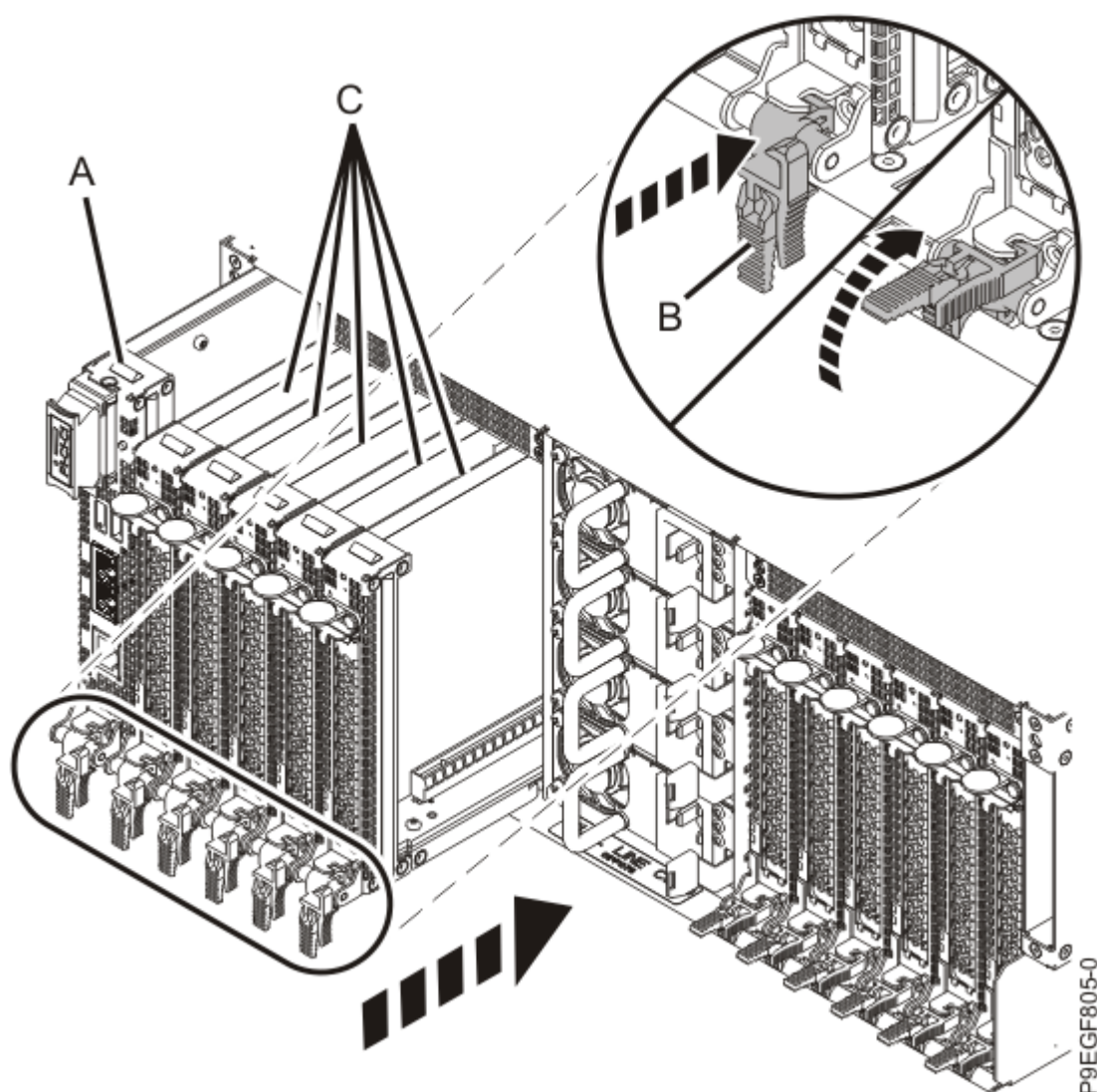
Figura 15. Sustitución de la tarjeta del procesador de servicio y las casetes PCIe
