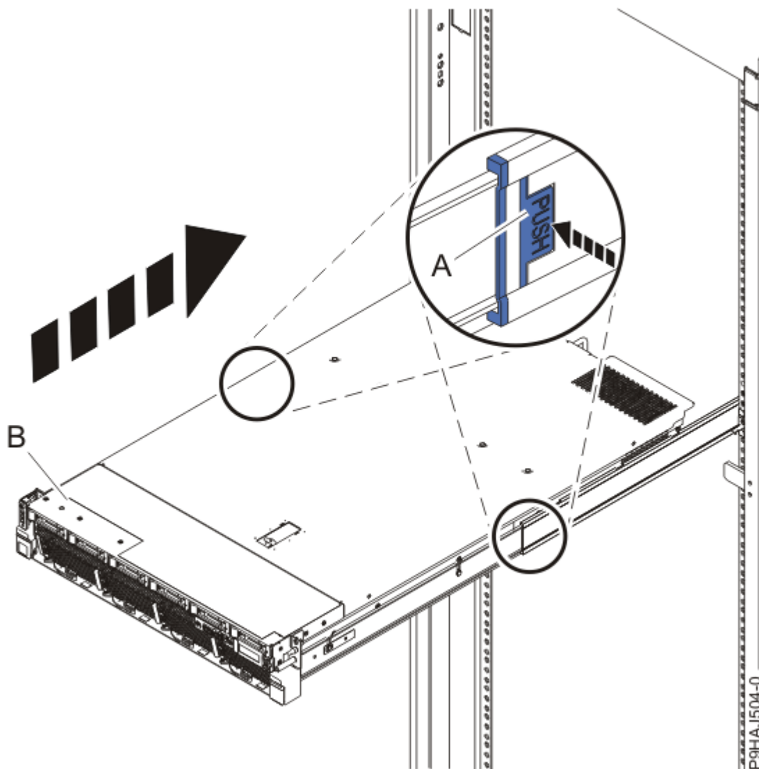
Figura 8. Colocación del sistema en la posición operativa
