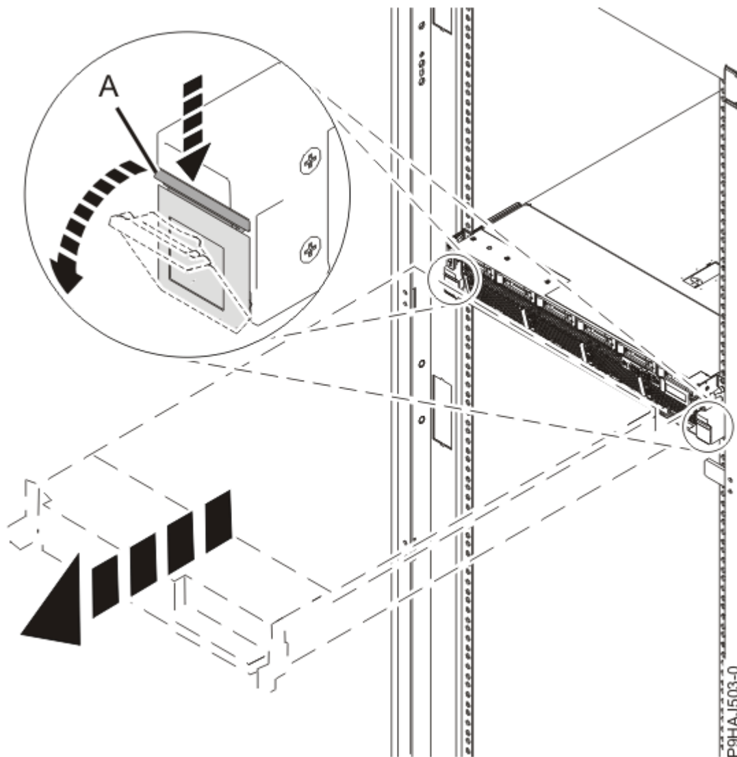
Figura 2. Cómo abrir los pestillos laterales
