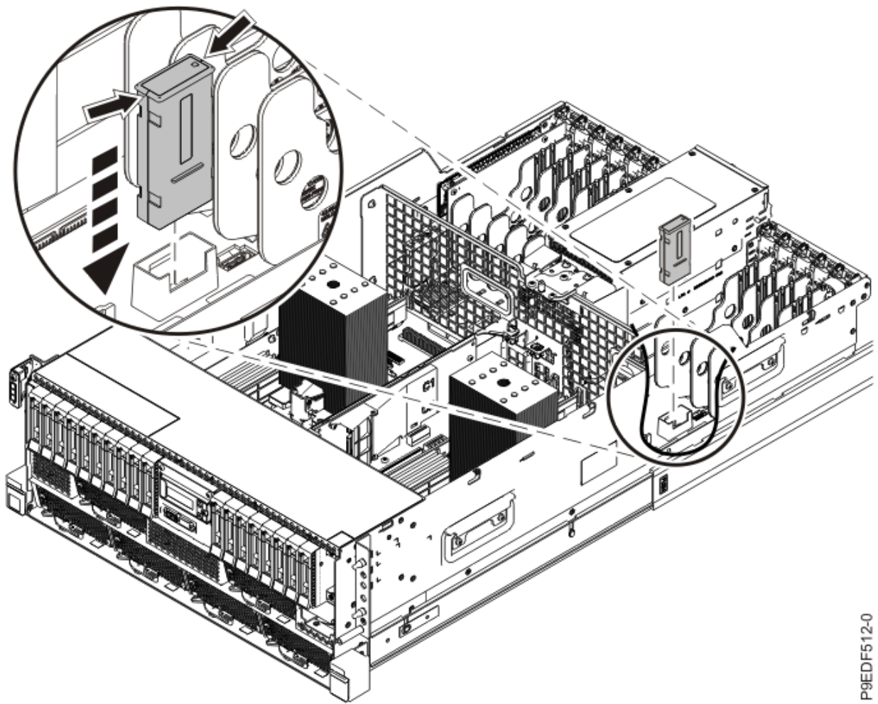
Figura 14. Sustitución de la tarjeta de VPD
