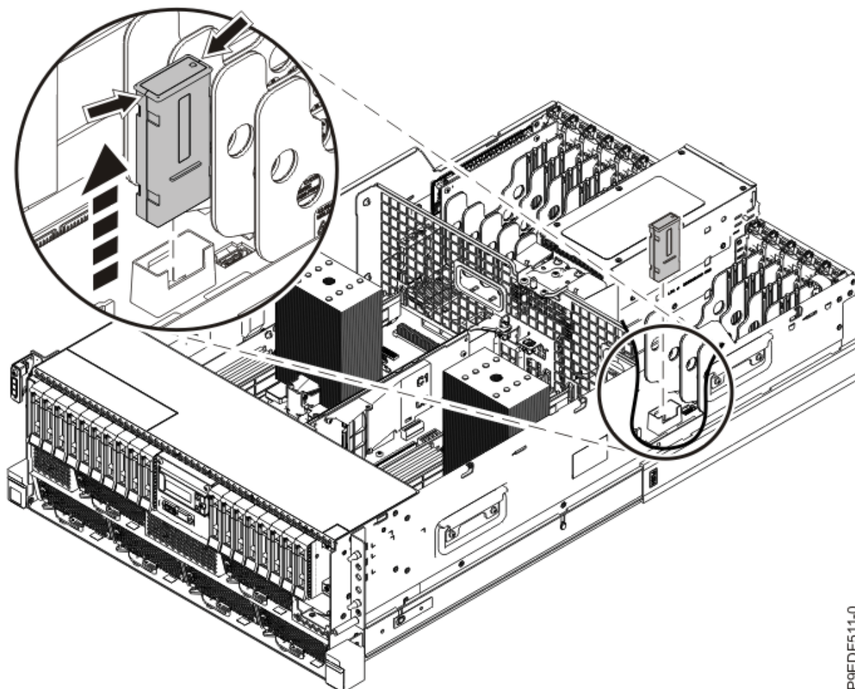
Figura 7. Extracción de la tarjeta de VPD
