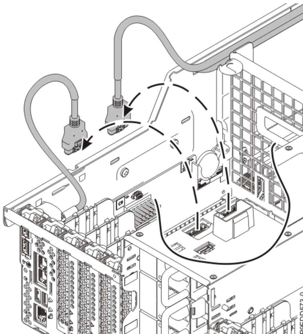
Figura 8. Cómo mover los cables USB frontal y posterior
