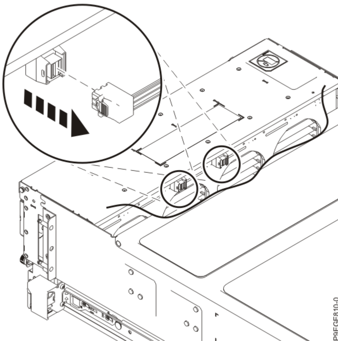
Figura 6. Desconexión de los cables SAS de la placa posterior base de la unidad de disco
