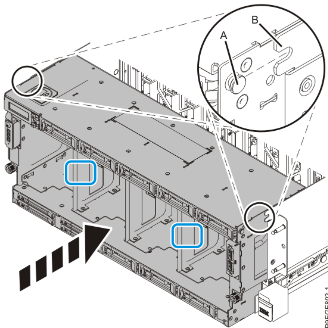
Figura 11. Colocación parcial de la placa posterior de la unidad de disco
