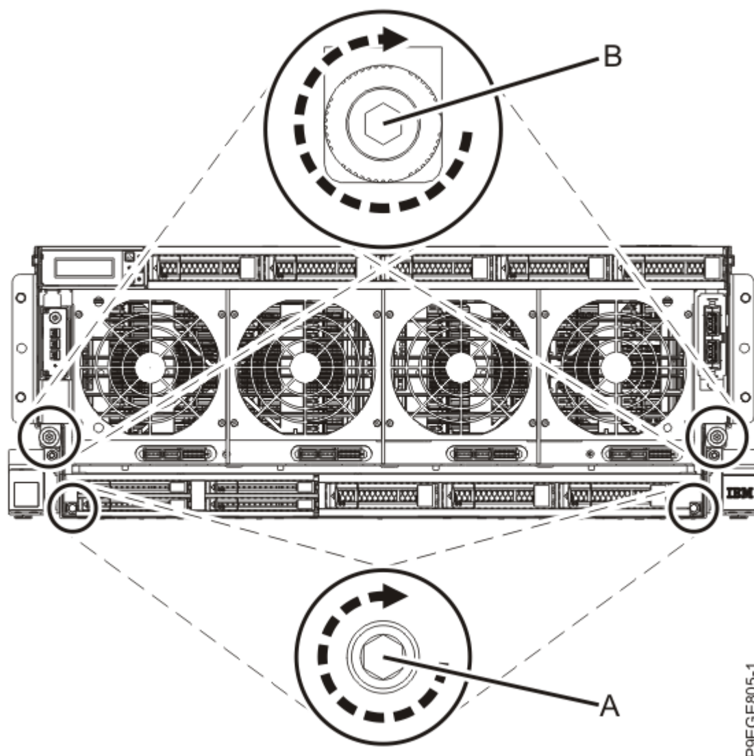
Figura 17. Fijación de los tornillos para la placa posterior de la unidad de disco
