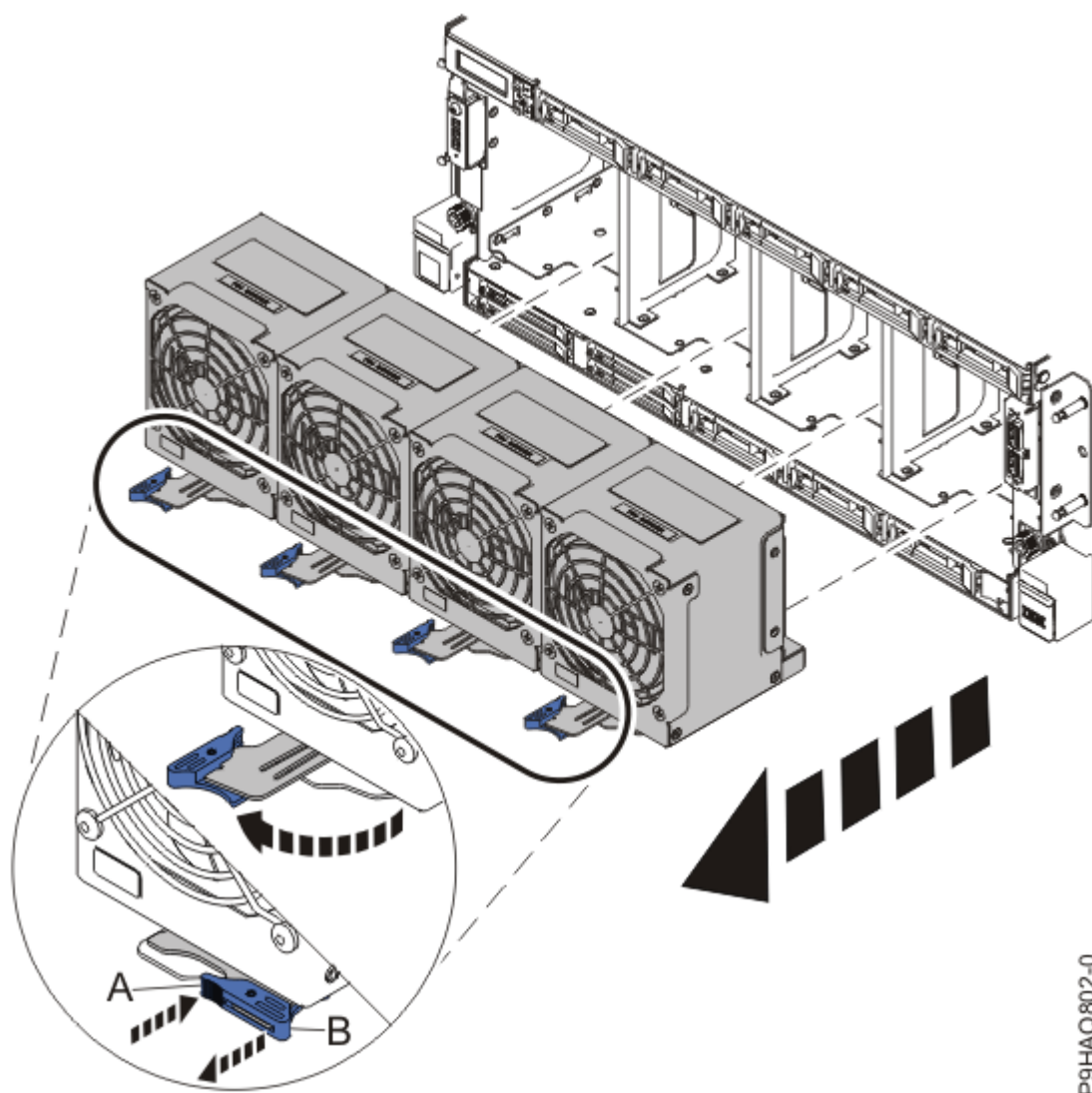
Figura 2. Extracción de los ventiladores
