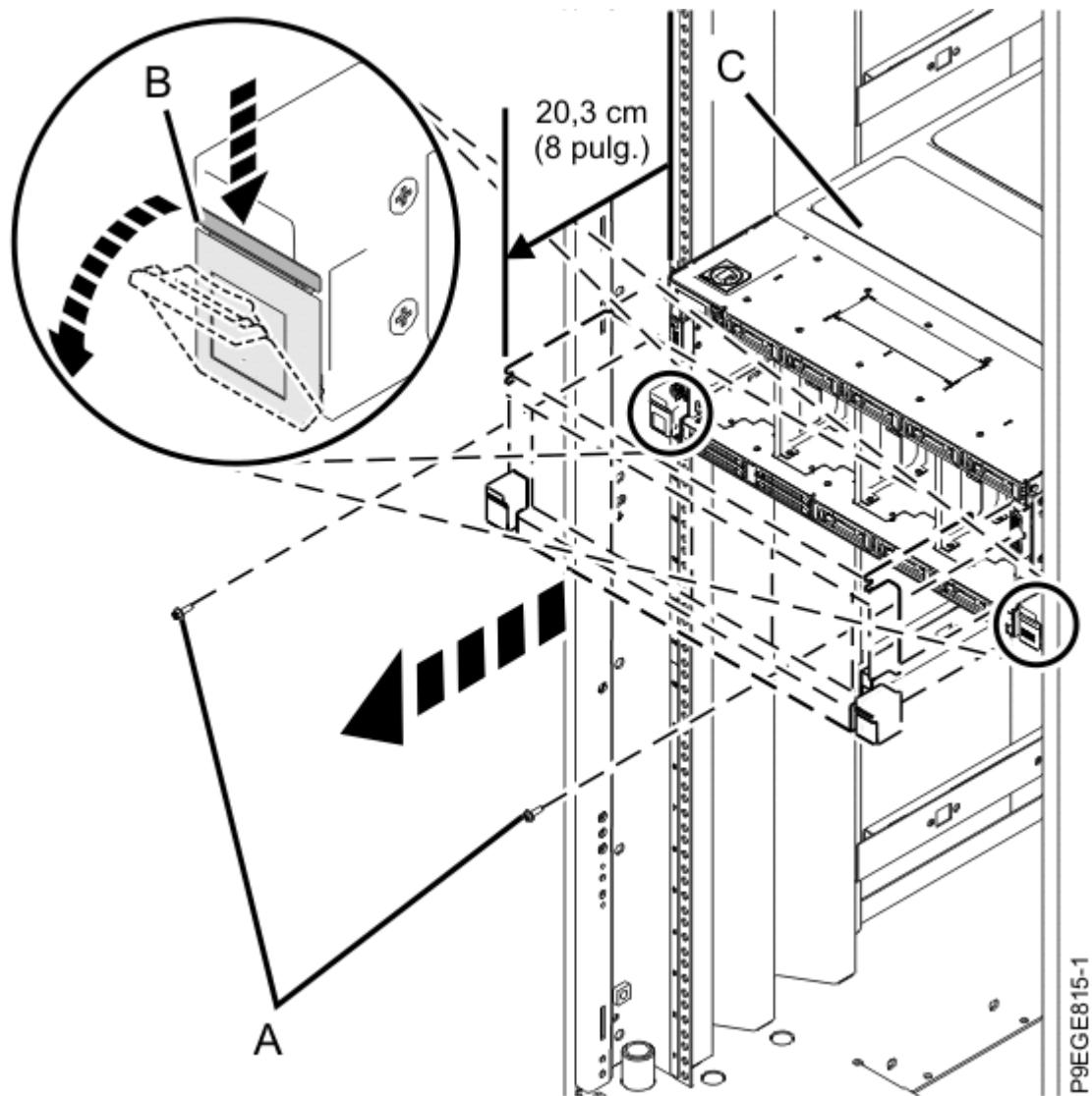
Figura 5. Deslizamiento parcial del sistema desde el bastidor
