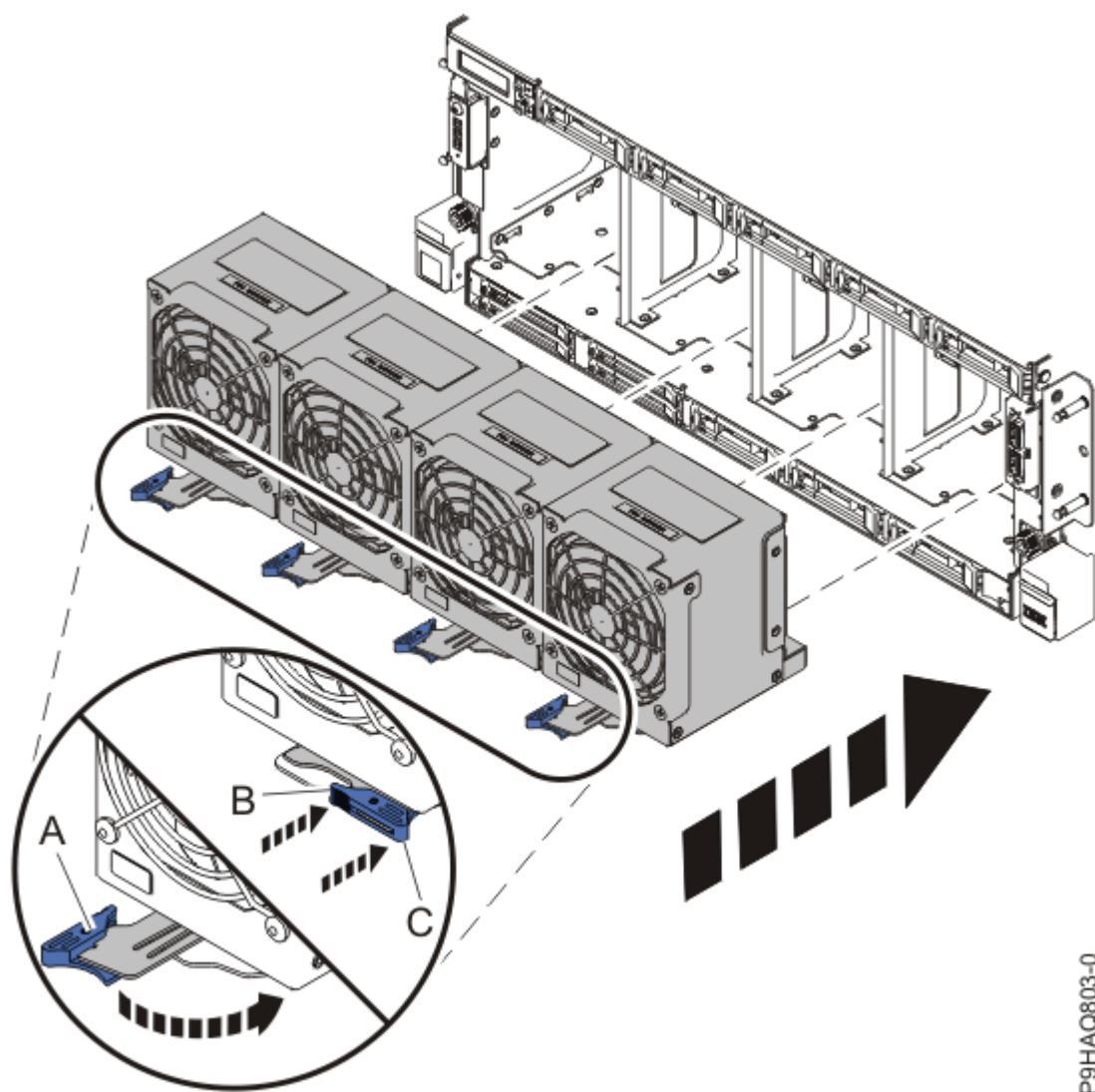
Figura 18. Sustitución de los ventiladores
