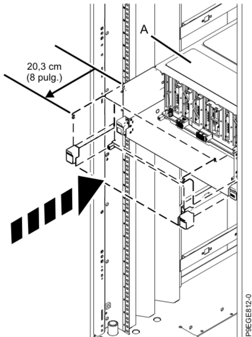
Figura 12. Deslizamiento parcial del sistema en el bastidor
