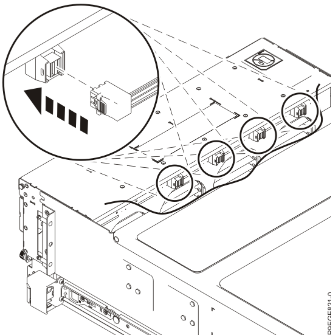
Figura 14. Conexión de los cables SAS a la placa posterior de la unidad de disco de función expandida
