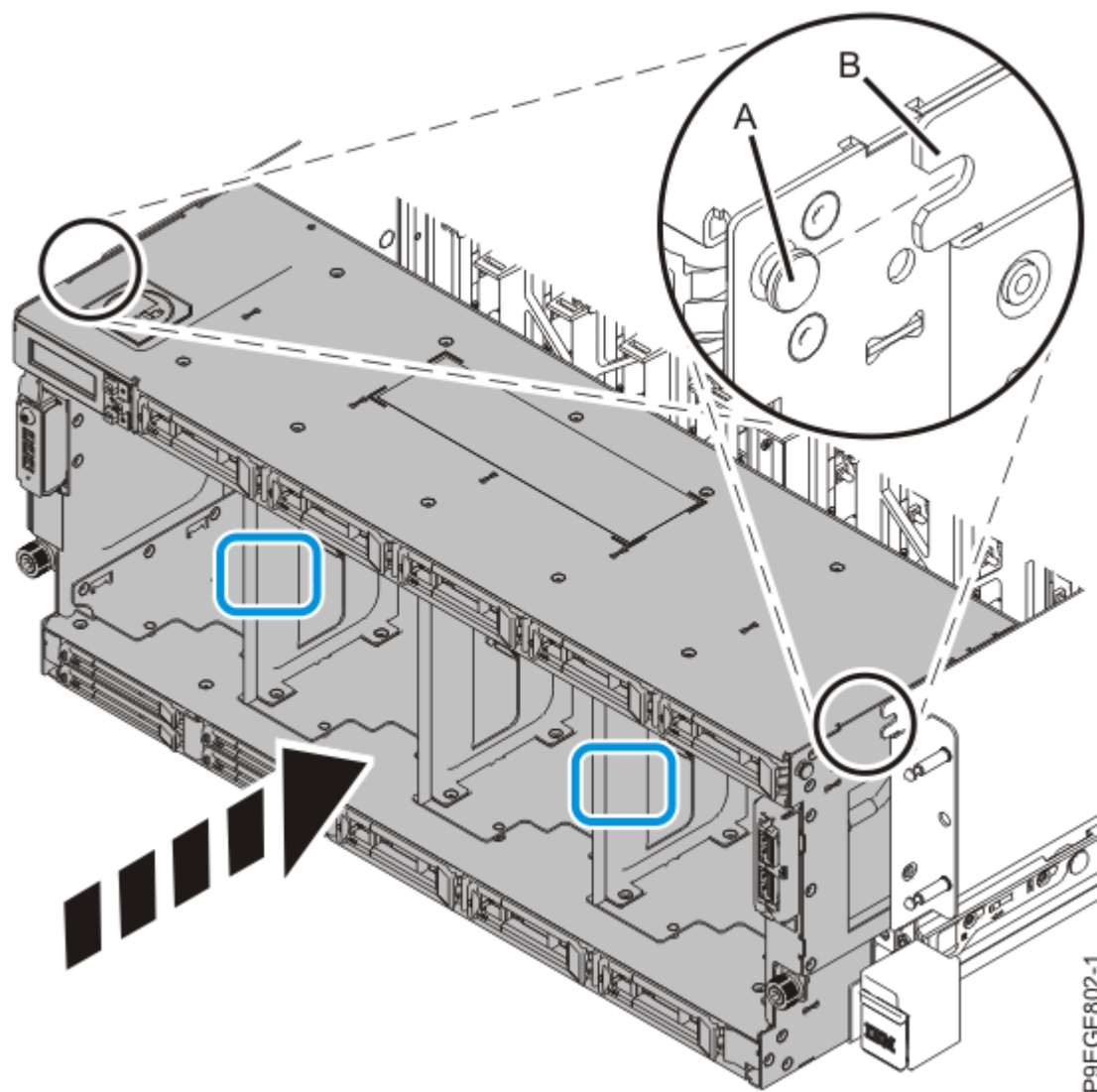
Figura 15. Colocación de la placa posterior de la unidad de disco
