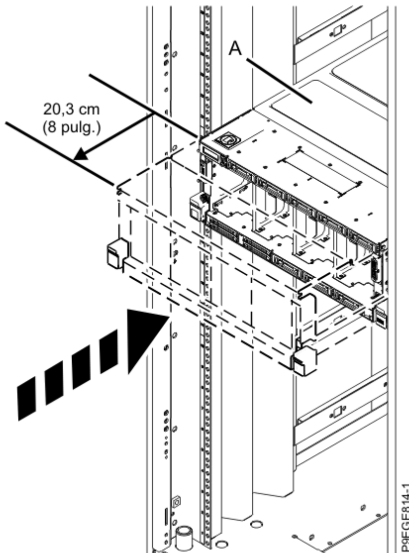
Figura 16. Colocación del sistema en la posición operativa
