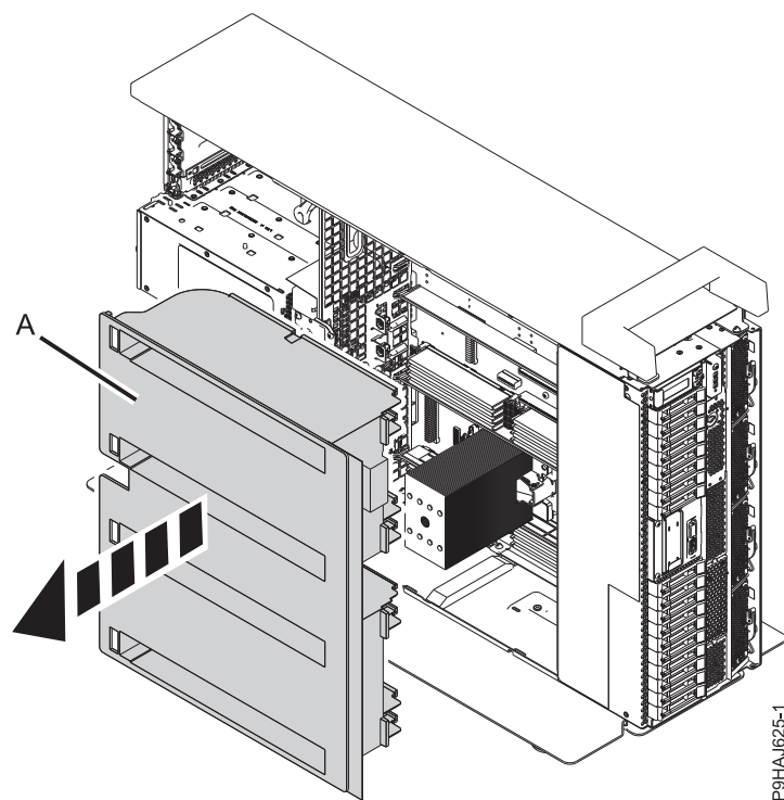
Figura 35. Extracción del deflector de aire de un sistema autónomo
