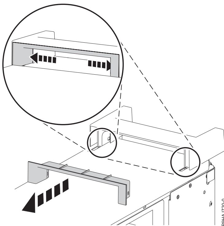
Figura 18. Extracción de la pieza de plástico de la tapa de asa
