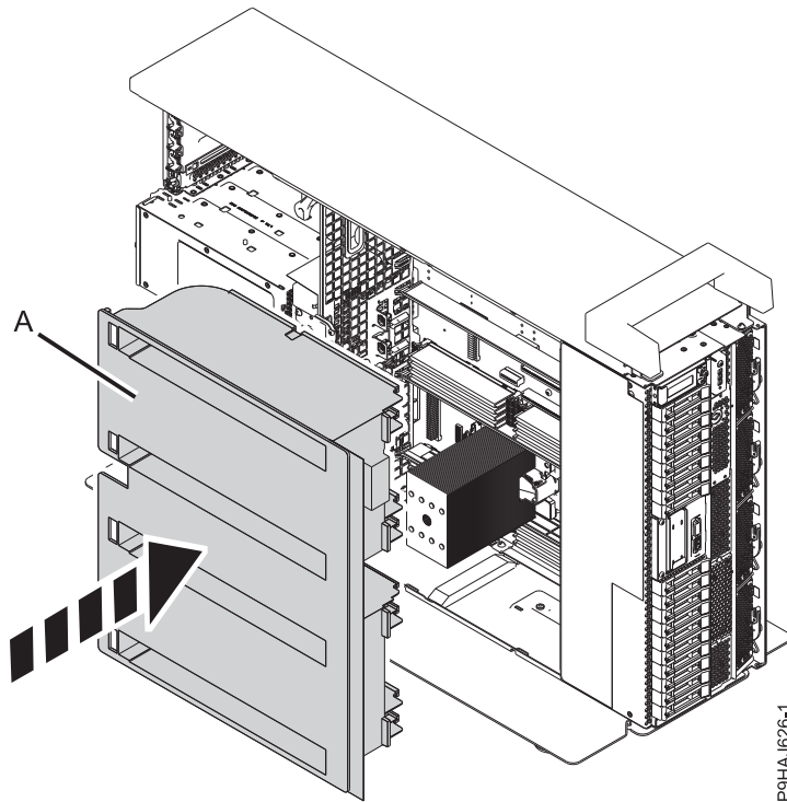
Figura 37. Sustitución del deflector de aire en un sistema autónomo
