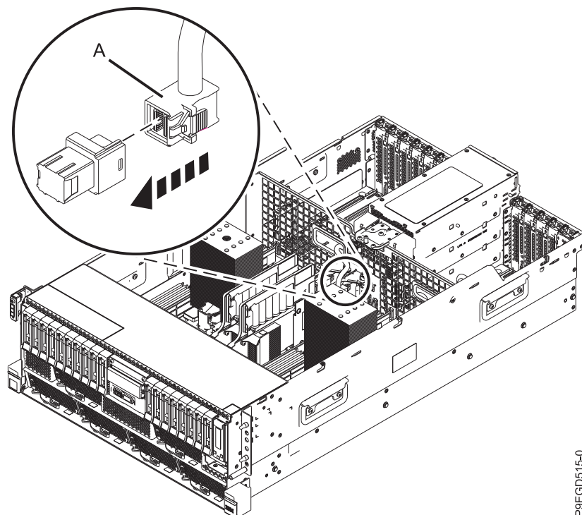
Figura 8. Instalación del cable SAS posterior
