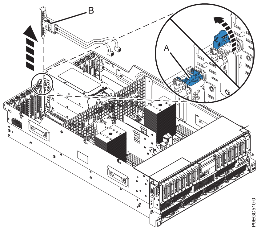
Figura 5. Extracción del adaptador de cable SAS posterior
