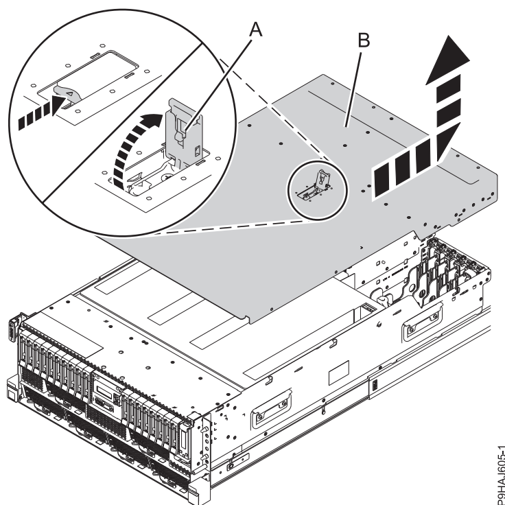
Figura 30. Extracción de la cubierta de acceso de servicio de un sistema montado en bastidor
