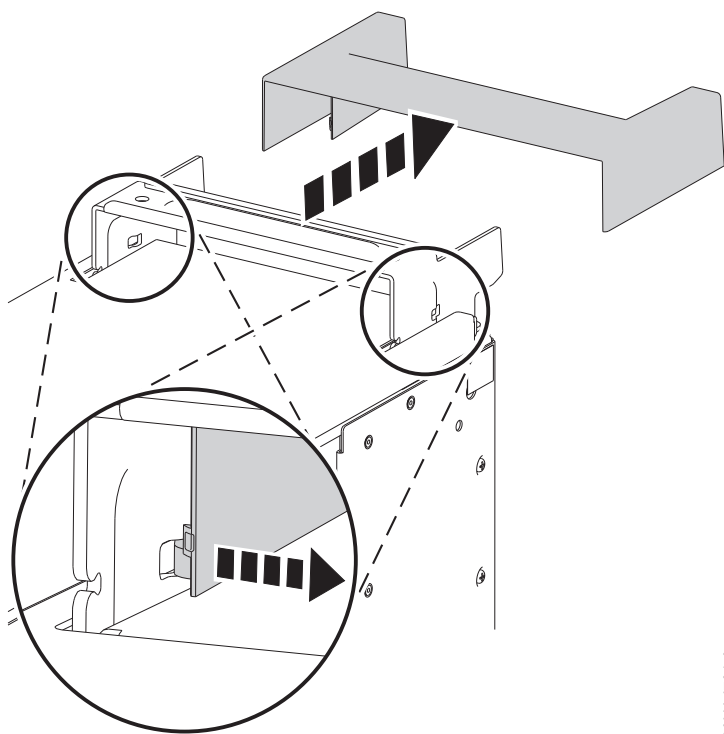
Figura 19. Extracción de la tapa de asa
