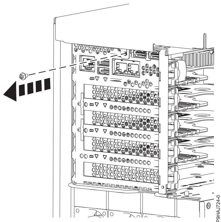
Figura 20. Extracción del tornillo de la cubierta lateral
