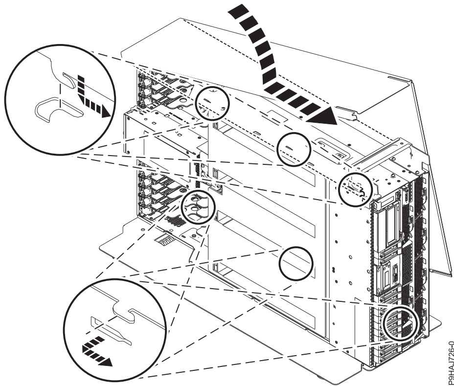
Figura 26. Instalación de la cubierta lateral
