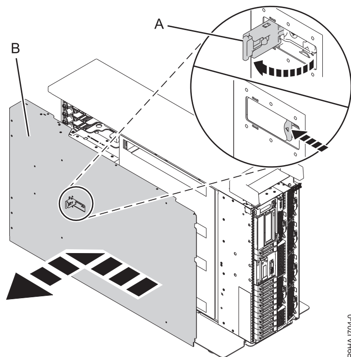
Figura 31. Extracción de la cubierta de acceso de servicio
