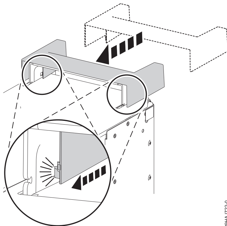
Figura 28. Fijación de la tapa de asa
