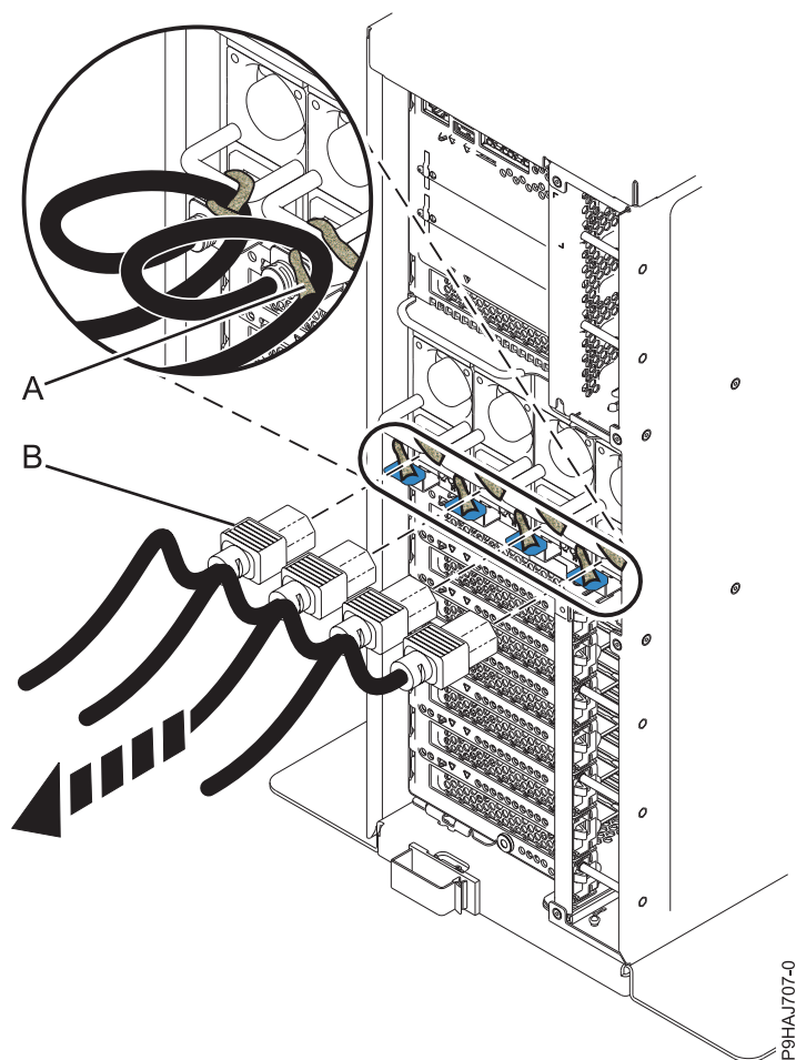
Figura 43. Extracción de los cables de alimentación de un servidor autónomo
