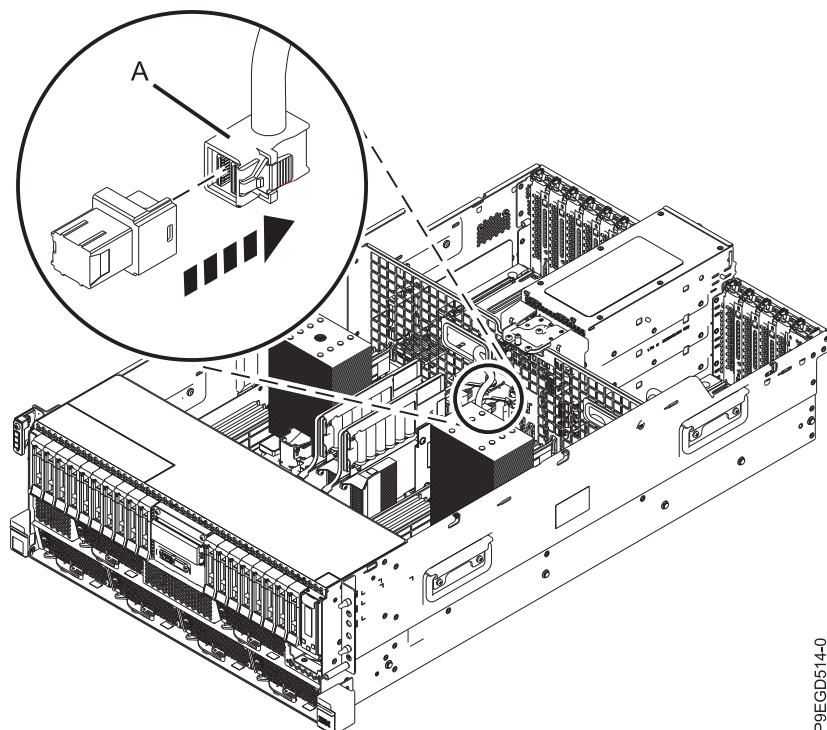
Figura 4. Desconexión de los cables SAS posteriores del adaptador SAS RAID interno en la ubicación de ranura P1-C49 y P-C50
