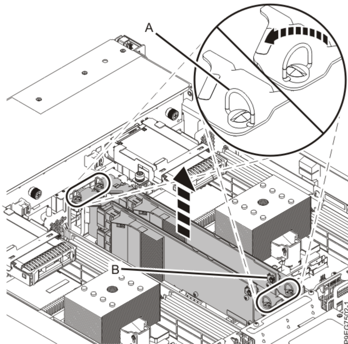
Figura 7. Extracción del adaptador SAS RAID
