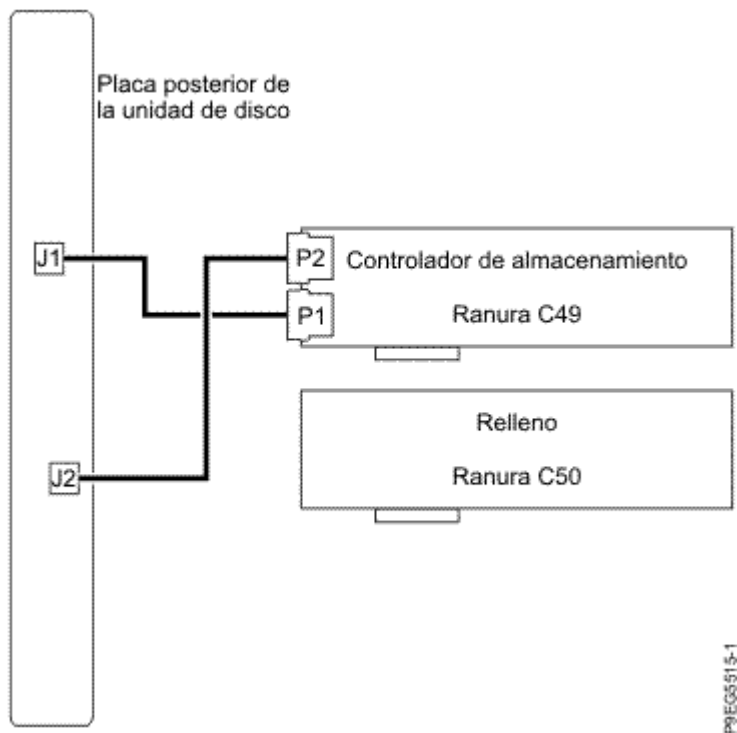
Figura 9. Reconexión del cable SAS en una configuración de almacenamiento base
