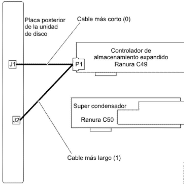
Figura 11. Reconexión del cable SAS "Y" en una configuración de controlador de almacenamiento de alto rendimiento
