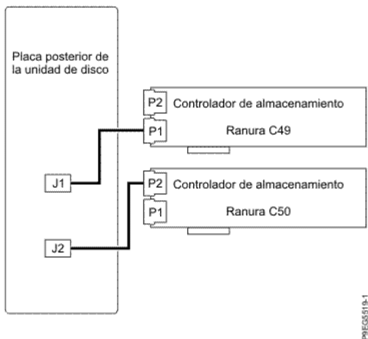
Figura 14. Reconexión del cable SAS en una configuración de discos divididos
