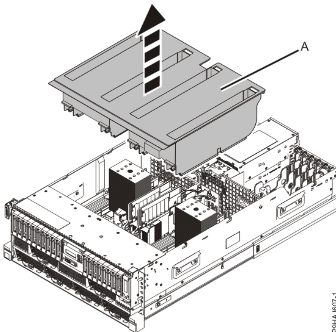
Figura 7. Extracción del deflector de aire de un sistema montado en bastidor
