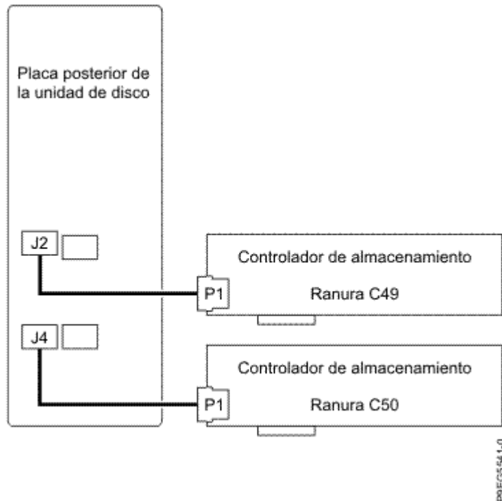
Figura 15. Reconexión del cable SAS en la configuración de la función ampliada de 12 unidades
