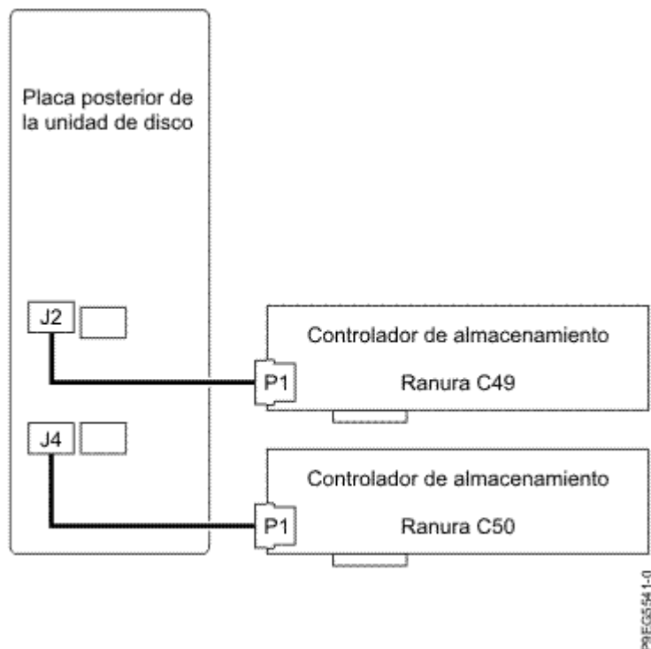
Figura 16. Reconexión del cable SAS en la configuración de la función ampliada de 18 unidades
