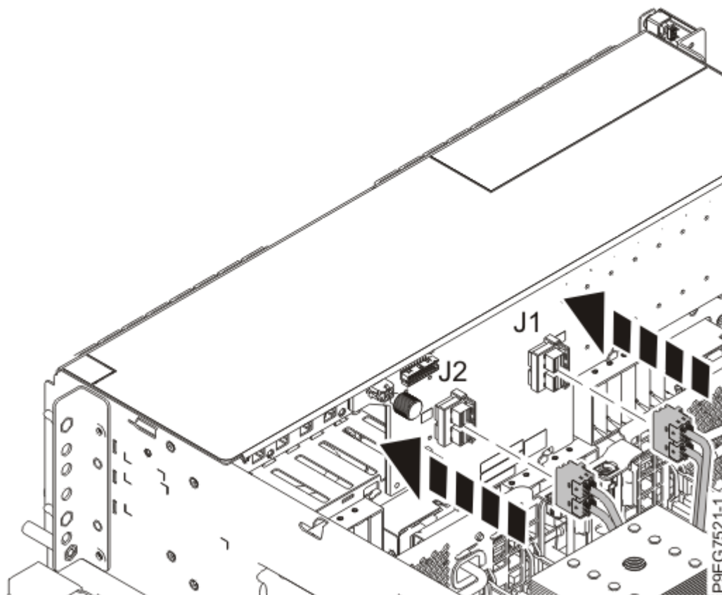
Figura 11. Reconexión de los cable SAS frontales en la placa posterior de la unidad de disco de función base
