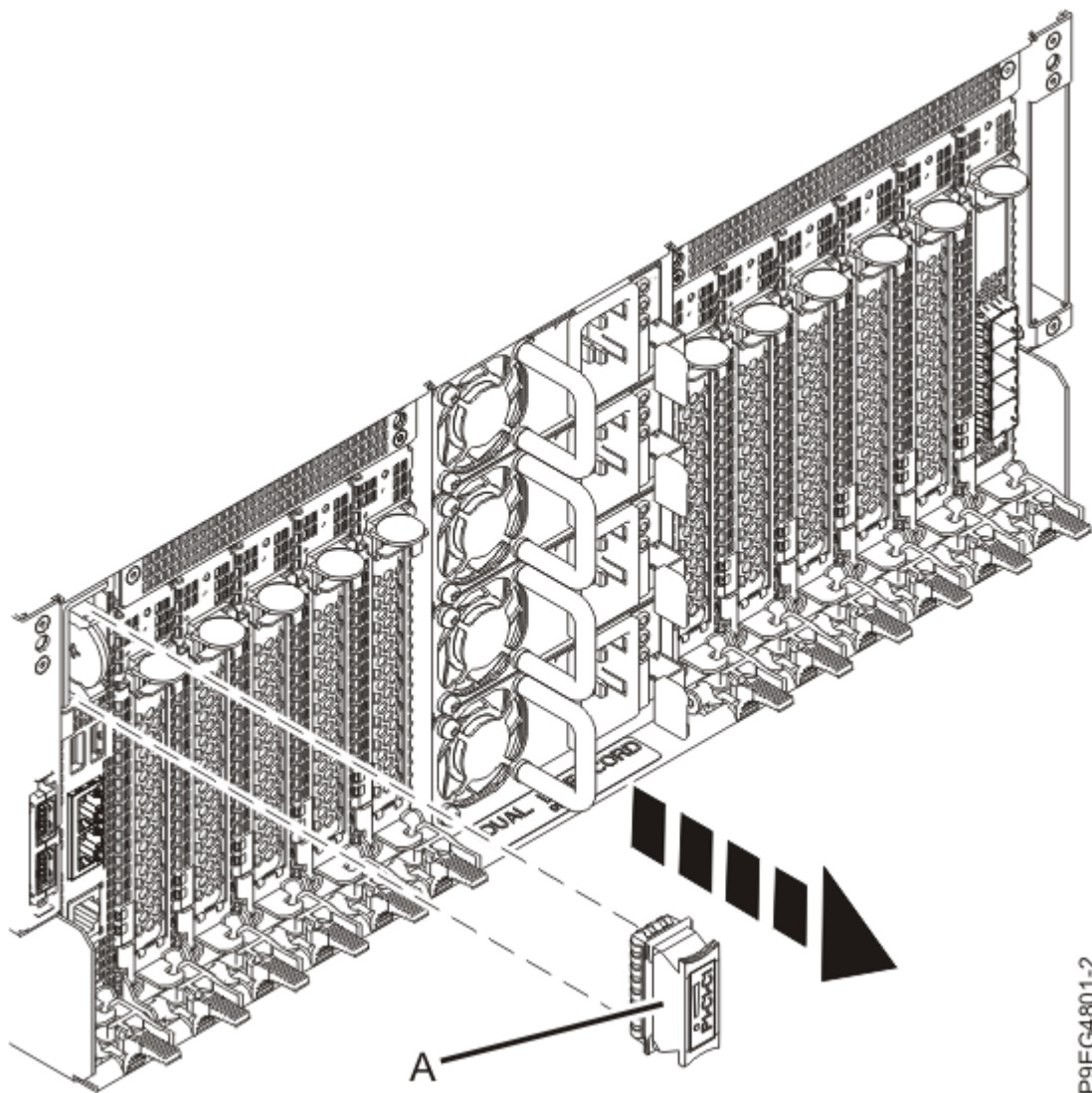
Figura 1. Extracción de la cubierta de la batería de hora del día
