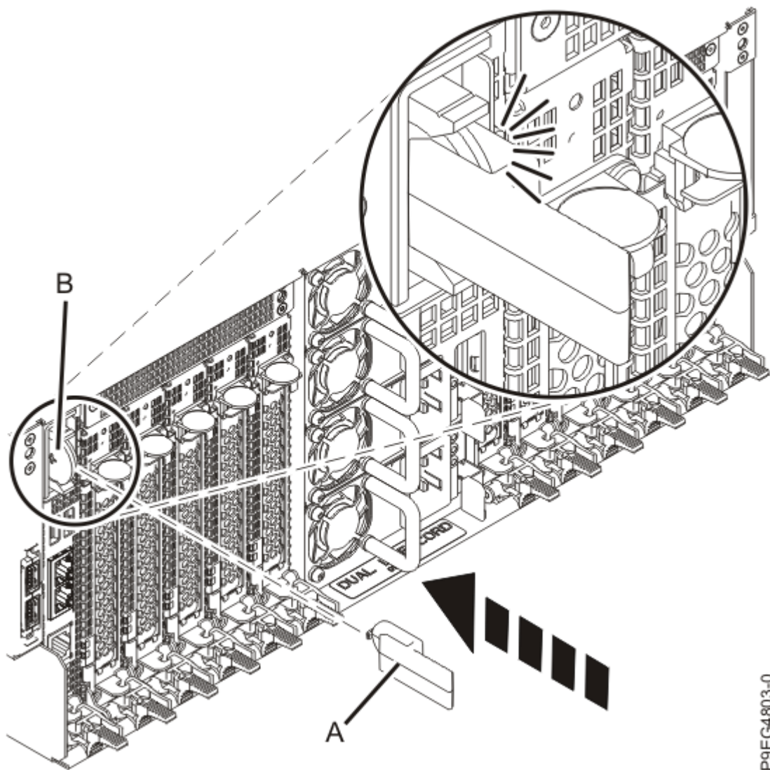
Figura 2. Conexión de la herramienta de extracción de la batería a la batería de hora del día c) Tire de la herramienta y la batería de hora del día ( A ) en la tarjeta de servicio.
