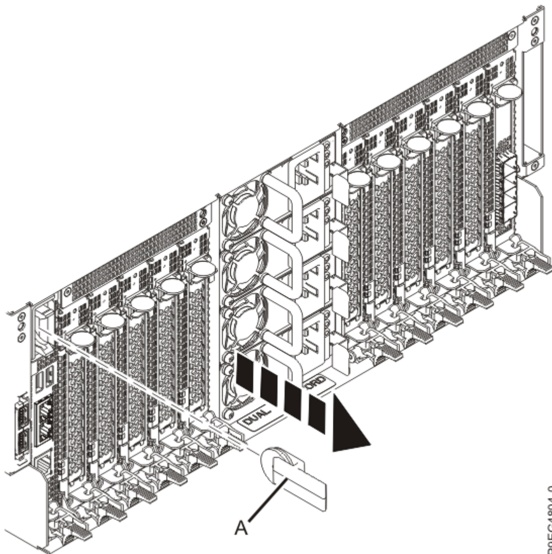
Figura 3. Extracción de la batería de hora del día
