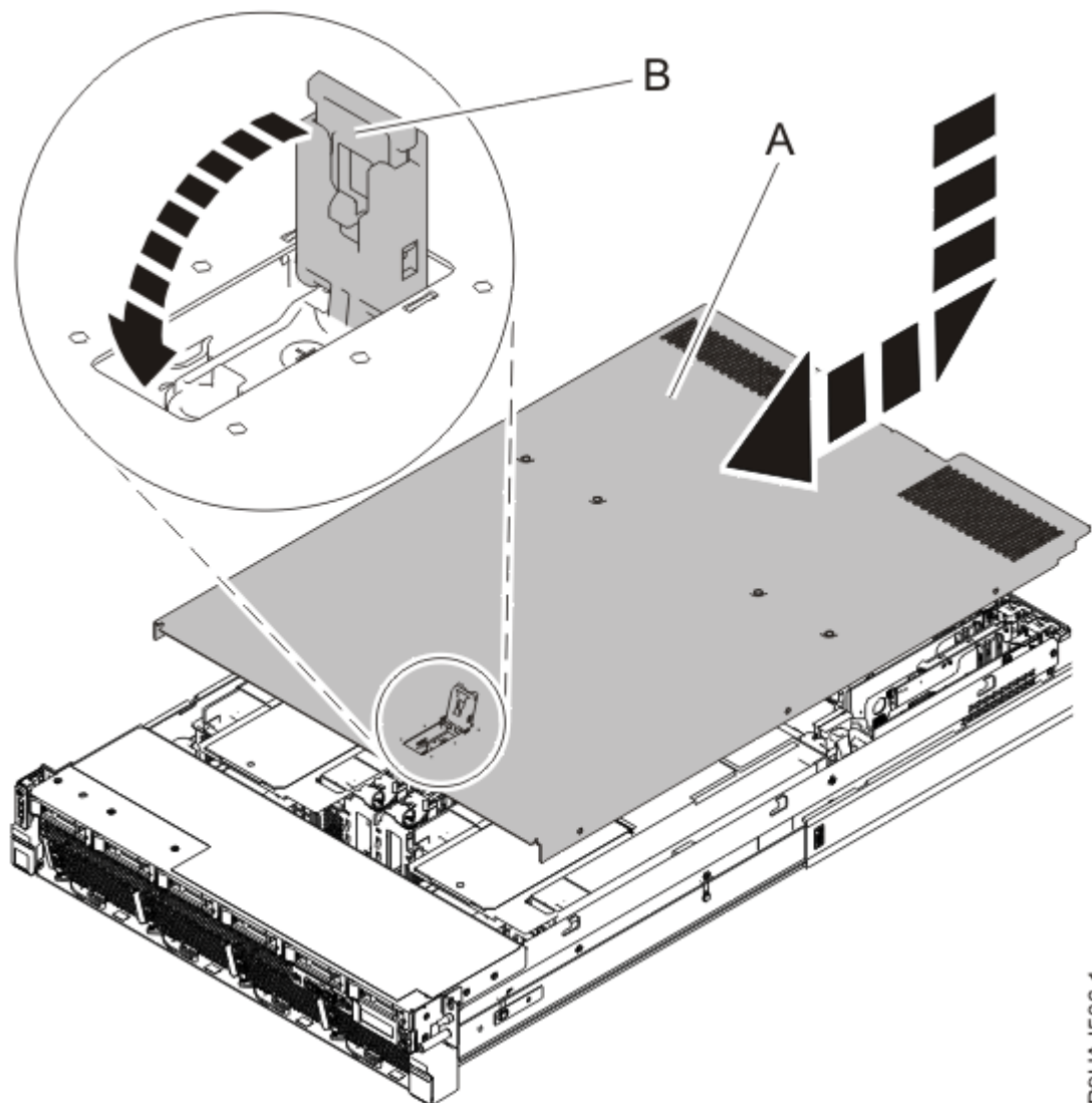
Figura 7. Instalación de la cubierta de acceso de servicio
