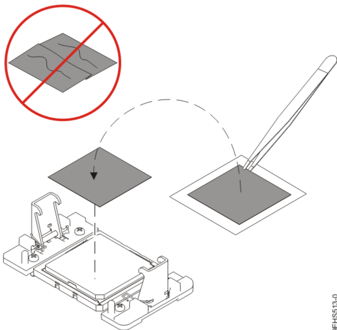
Figura 23. Cómo desplazar el TIM en el módulo del procesador del sistema
