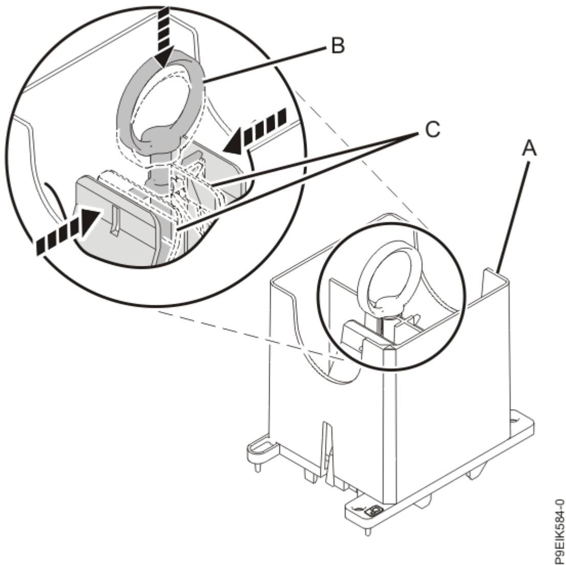
Figura 14. Cómo asegurarse de que la herramienta de extracción esté en posición abierta
