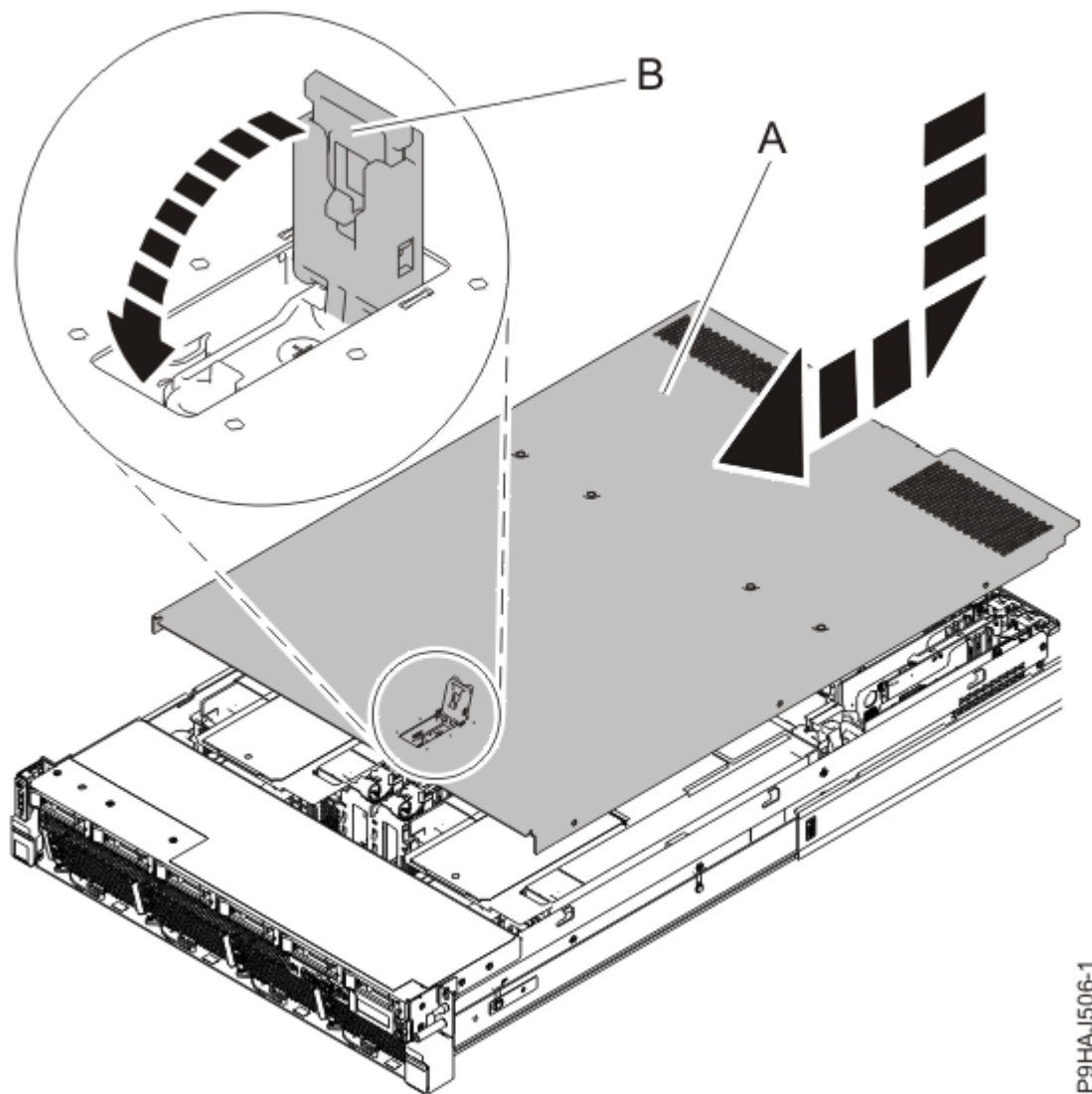
Figura 28. Instalación de la cubierta de acceso de servicio
