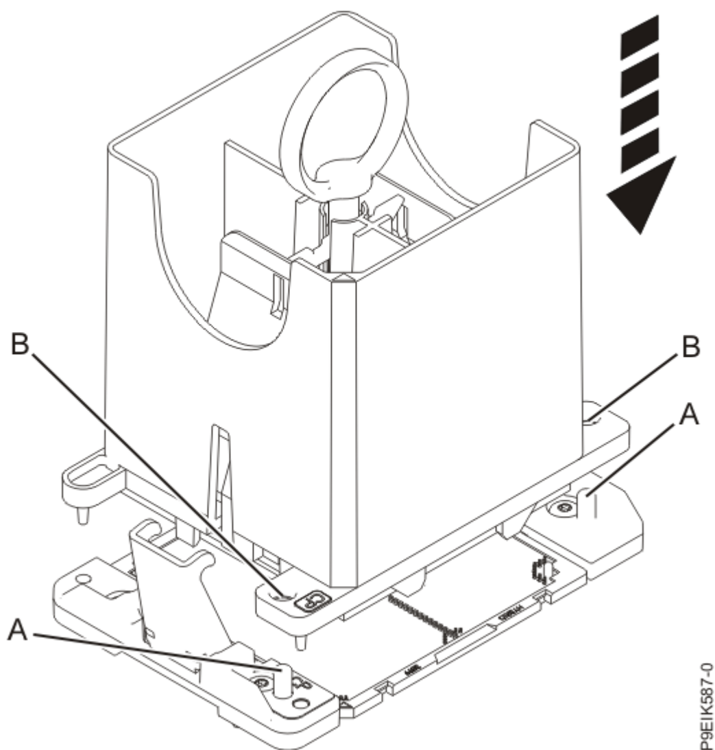
Figura 18. Instalación del módulo del procesador del sistema
