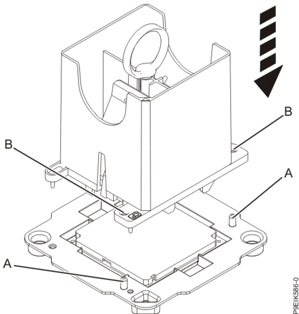
Figura 15. Cómo bajar la herramienta de extracción en el módulo del procesador del sistema
