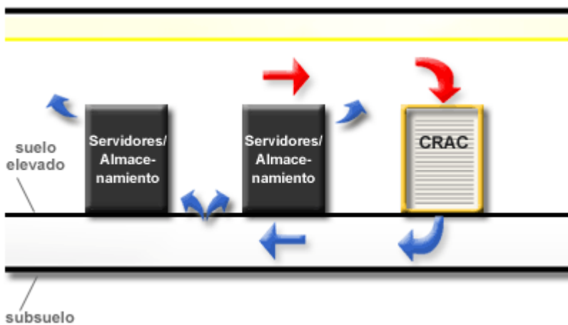
Figura 42. Distribución de aire subterráneo
