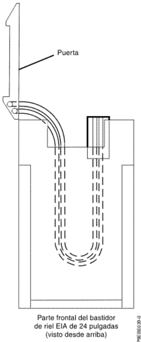
Figura 30. Ejemplo 2 de manejo de mangueras en suelo elevado y suelo no elevado; bucle bajo el bastidor de riel EIA de 24 pulgadas con la puerta abierta
