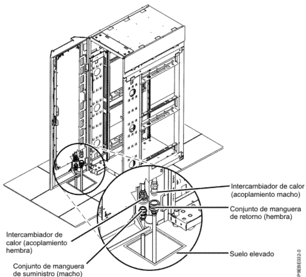
Figura 23. Ejemplo 1 de manejo de mangueras en suelo elevado; tamaño y posición de la abertura de entarimado para bastidores de riel EIA de 19 pulgadas
