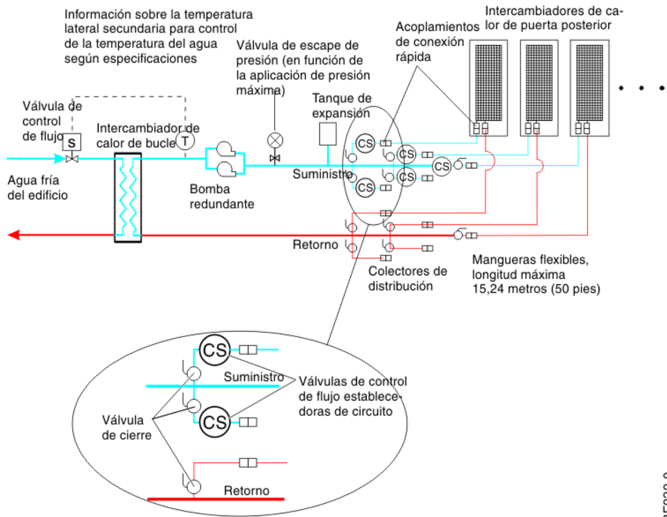
Figura 16. Distribución de refrigerante utilizando una solución fabricada
