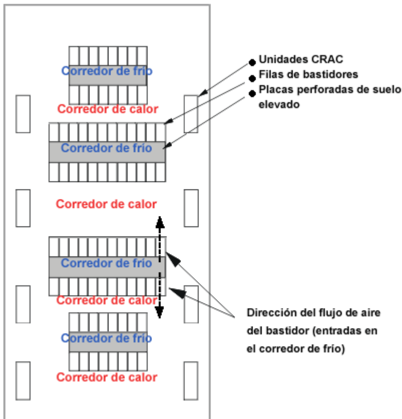
Figura 2. Organización en corredor de calor y corredor de frío
