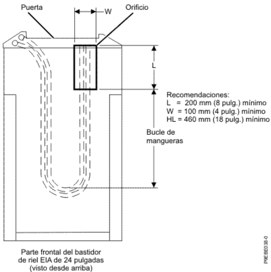
Figura 28. Ejemplo 2 de manejo de mangueras en suelo elevado y suelo no elevado; bucle bajo el bastidor de riel EIA de 24 pulgadas con la puerta cerrada
