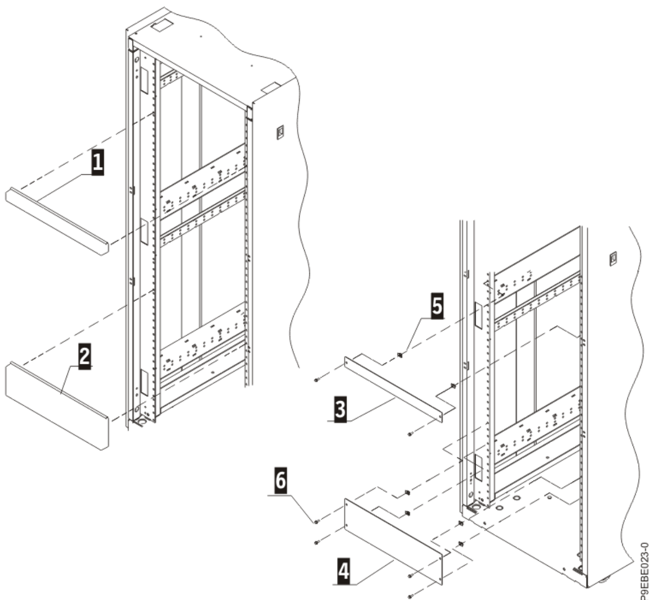
Figura 1. Imagen de los paneles de relleno 1U y 3U y números de pieza
