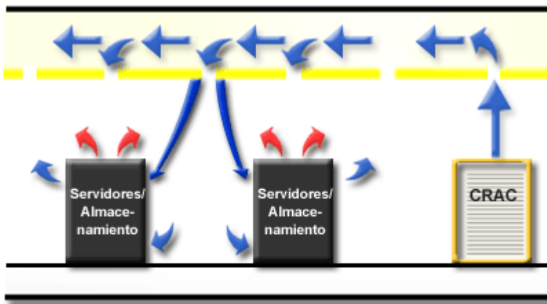
Figura 44. Sistema de distribución de aire global
