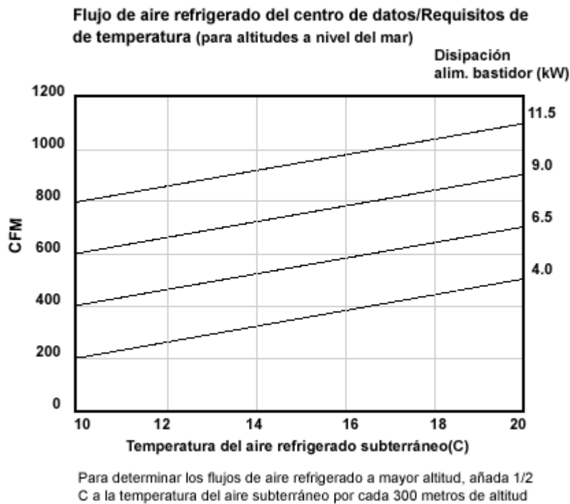
Figura 4. Requisitos de corriente de aire refrigerado y temperatura en equipos de gama alta
