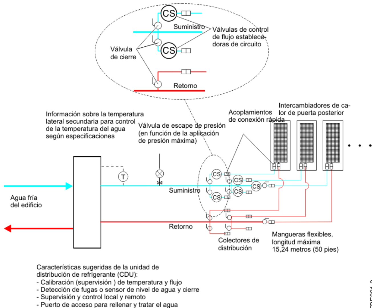
Figura 17. Distribución de refrigerante utilizando soluciones de proveedor genéricas
