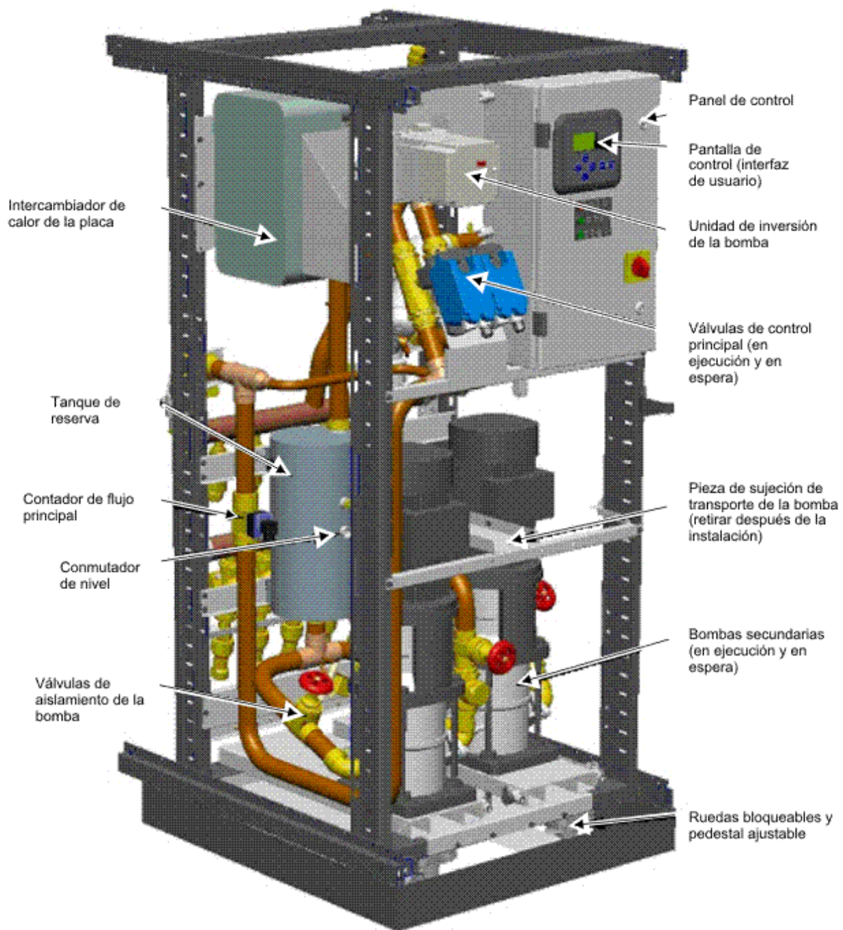
Figura 33. Unidad de distribución de refrigeración
