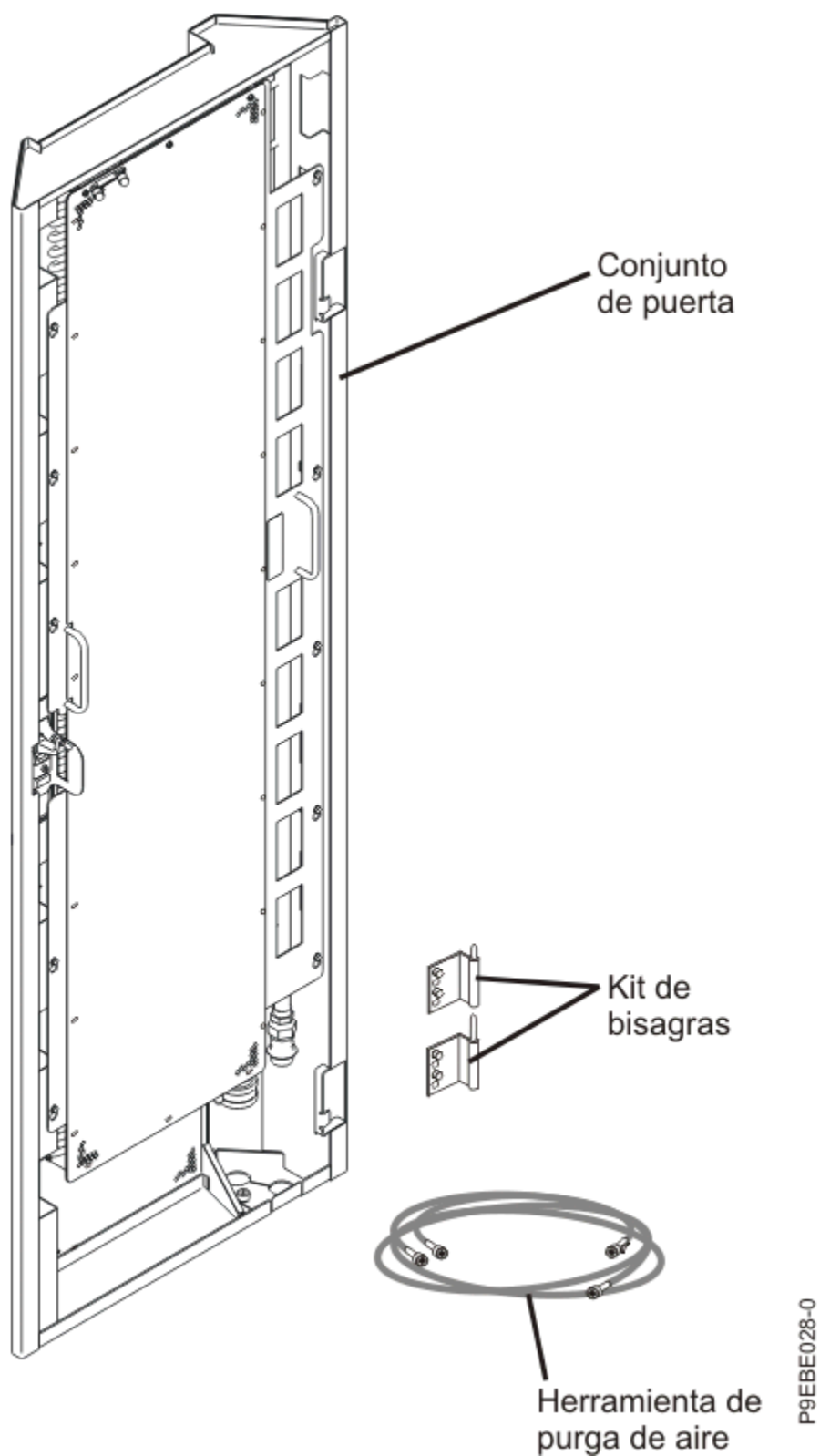
Figura 12. Componentes del kit de intercambiador de calor para bastidores de riel EIA de 19 pulgadas
