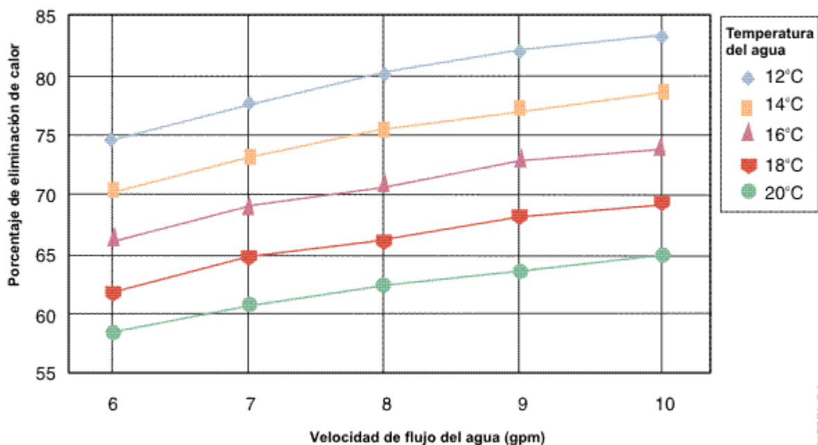
Figura 15. Rendimiento típico de un intercambiador de calor de la puerta posterior, carga de calor de 20 kW
