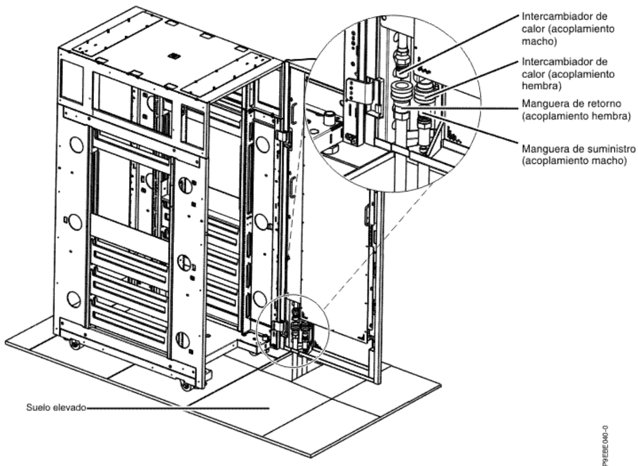
Figura 24. Ejemplo 1 de manejo de mangueras en suelo elevado; tamaño y posición de la abertura de entarimado para bastidores de riel EIA de 24 pulgadas
