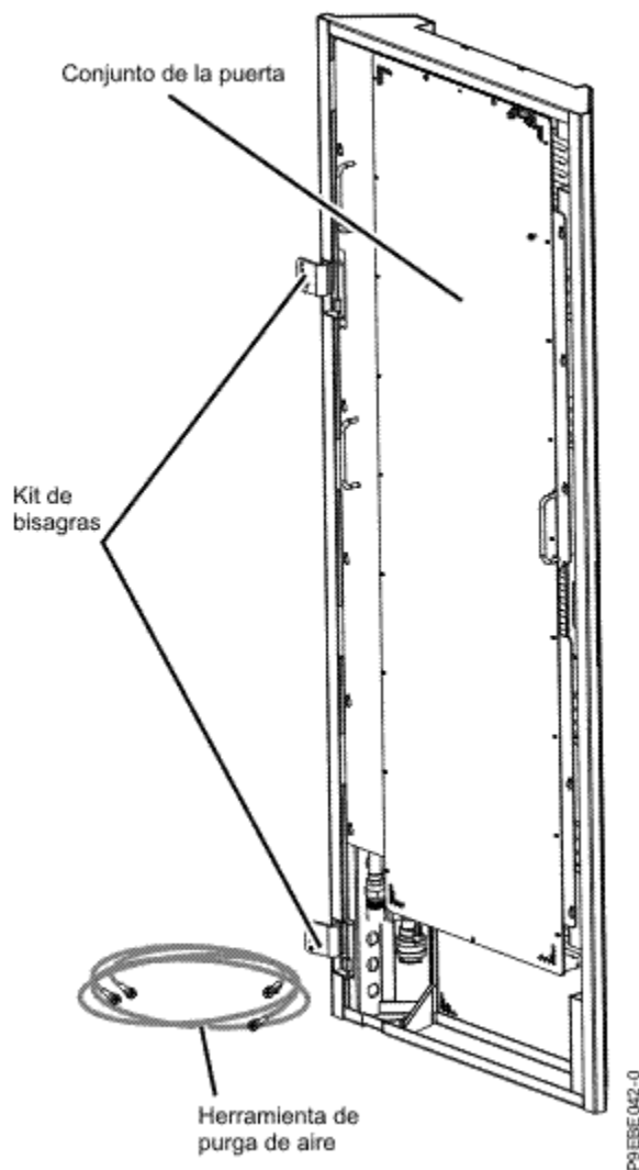
Figura 13. Componentes del kit de intercambiador de calor para bastidores de riel EIA de 24 pulgadas
