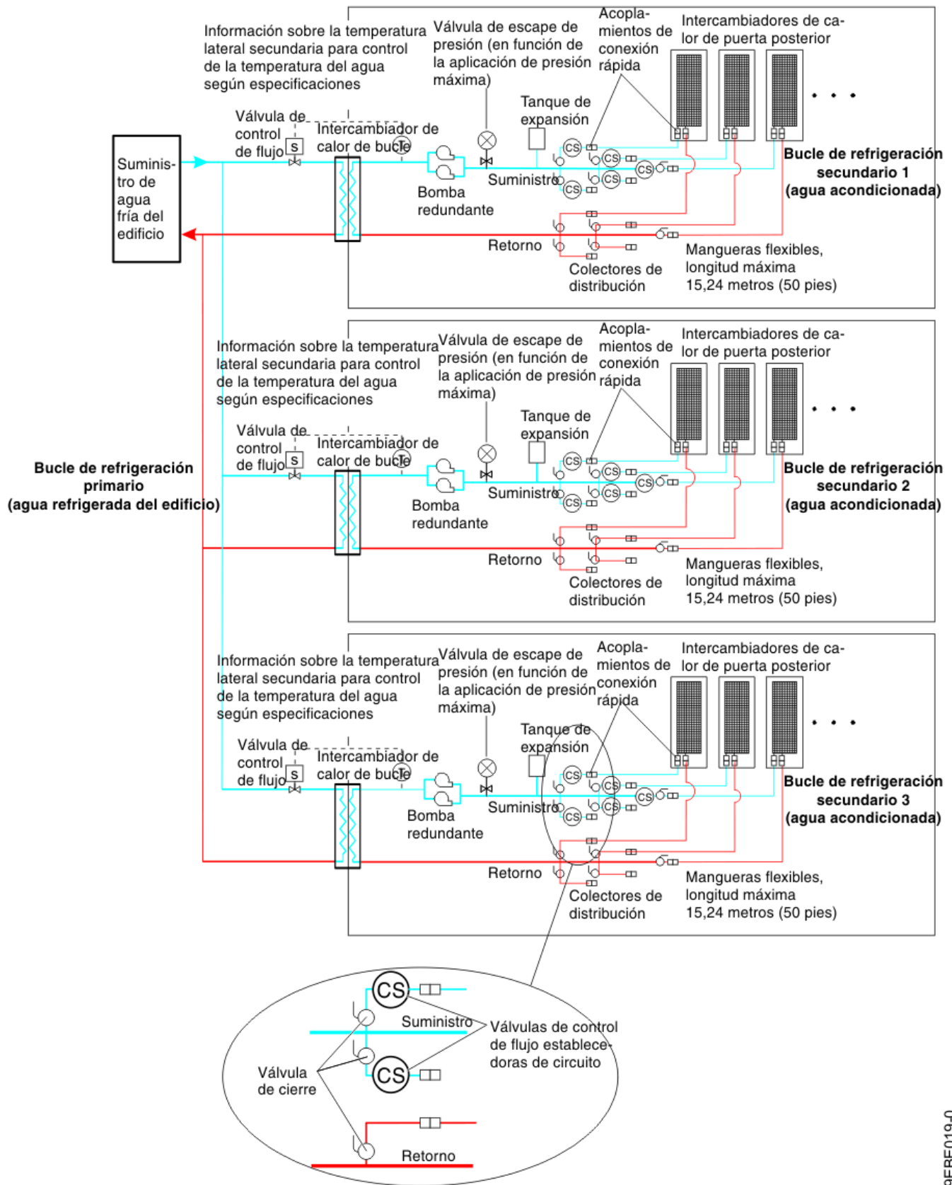
Figura 19. Bucles de refrigeración primario y secundario
