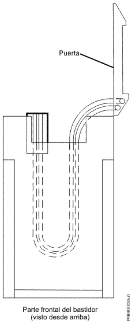
Figura 29. Ejemplo 2 de manejo de mangueras en suelo elevado y suelo no elevado; bucle bajo el bastidor de riel EIA de 19 pulgadas con la puerta abierta
