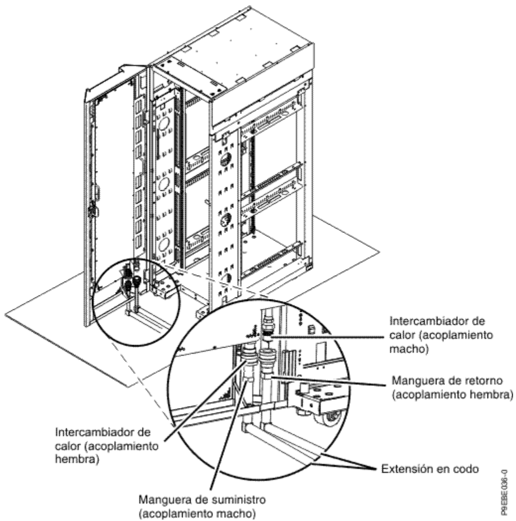
Figura 31. Requisitos de mangueras en suelos no elevados para el bastidor de riel EIA de 19 pulgadas
