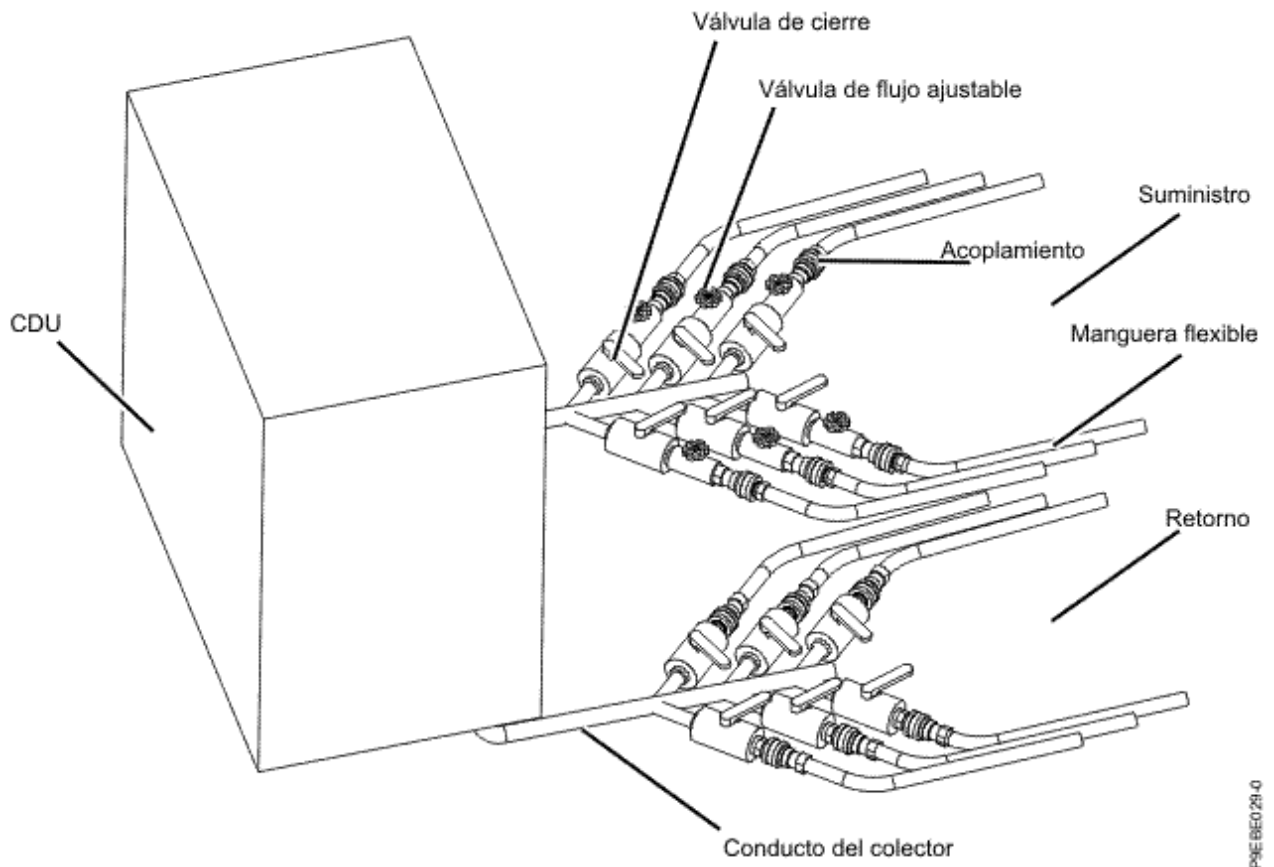
Figura 20. Disposición de colector de distribución central típica en una ubicación central
