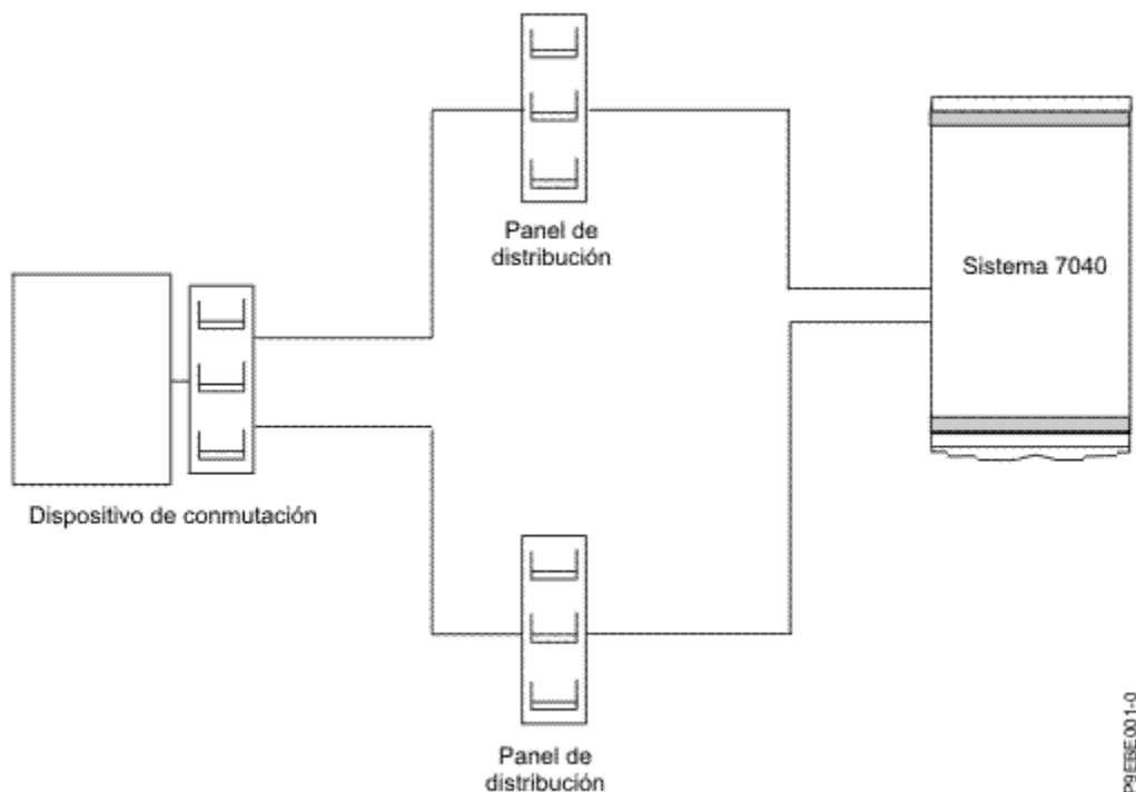
Figura 9. Instalación de alimentación dual - Panel de distribución redundante
