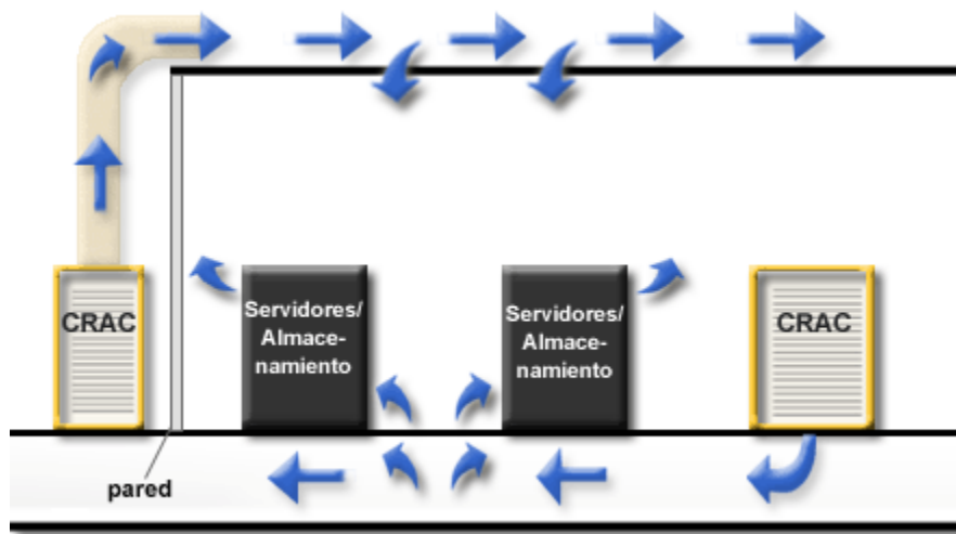
Figura 43. Combinación de sistemas de aire acondicionado global y subterráneo
