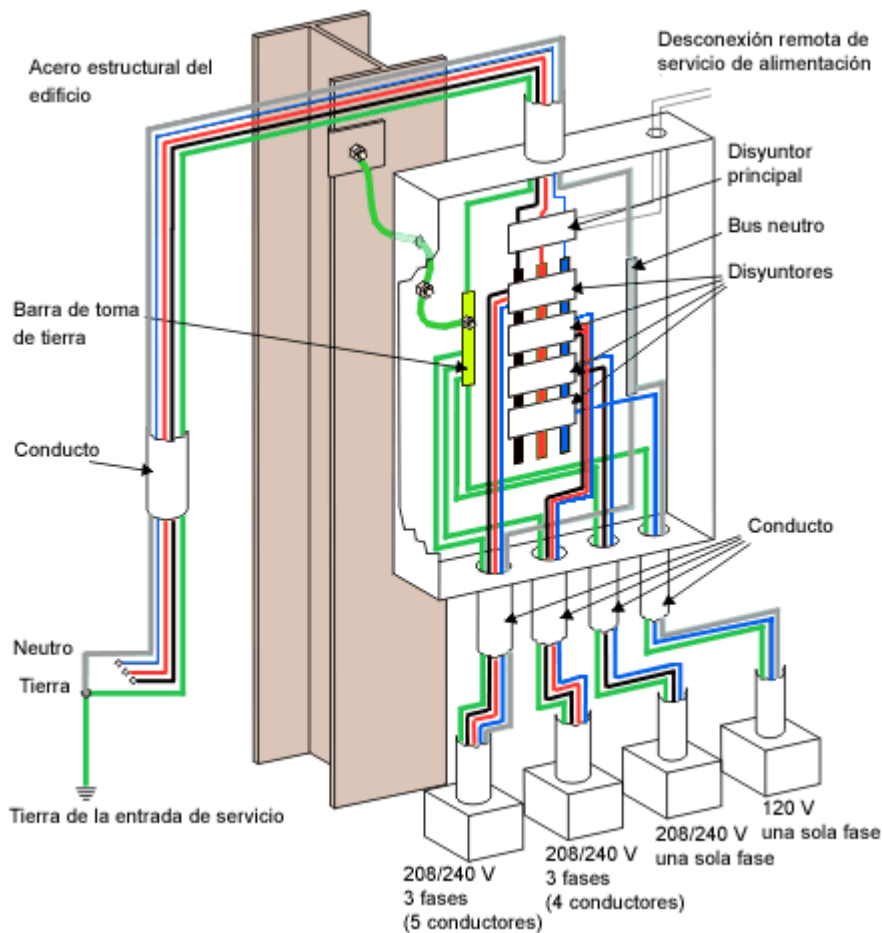
Figura 34. Placa de toma de tierra para fluctuaciones transitorias
