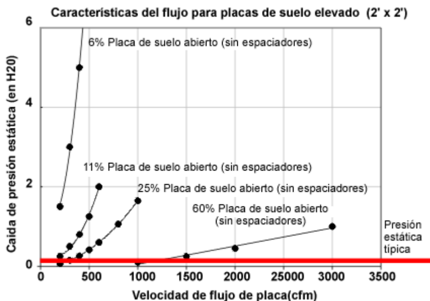
Figura 5. Capacidades de flujo volumétrico de las diversas placas del entarimado
