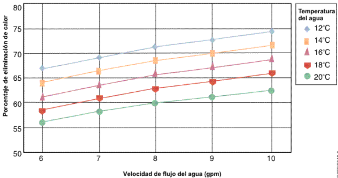
Figura 14. Rendimiento típico de un intercambiador de calor de la puerta posterior, carga de calor de 32 kW
