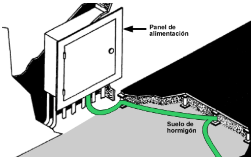
Figura 36. Toma de tierra temporal utilizando la estructura de soporte del pavimento elevado
