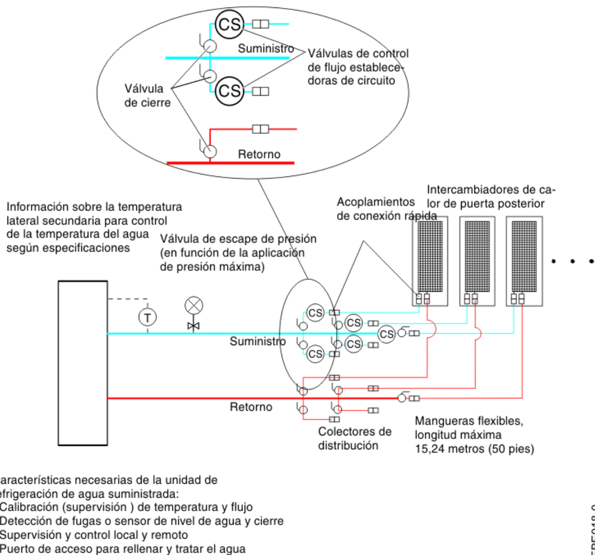
Figura 18. Unidad de distribución de refrigeración que utiliza una unidad de refrigeración de agua para proporcionar agua acondicionada
