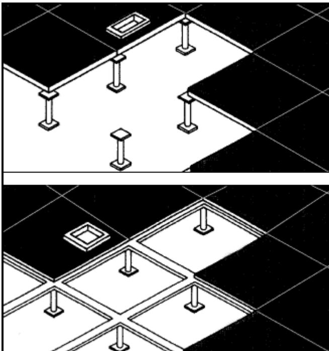
Figura 38. Tipos de suelos elevados
