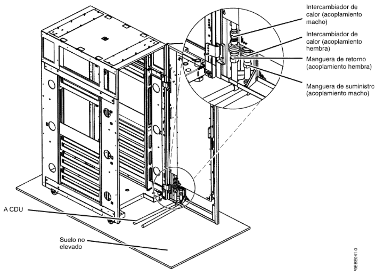
Figura 32. Requisitos de mangueras en suelos no elevados para el bastidor de riel EIA de 24 pulgadas
