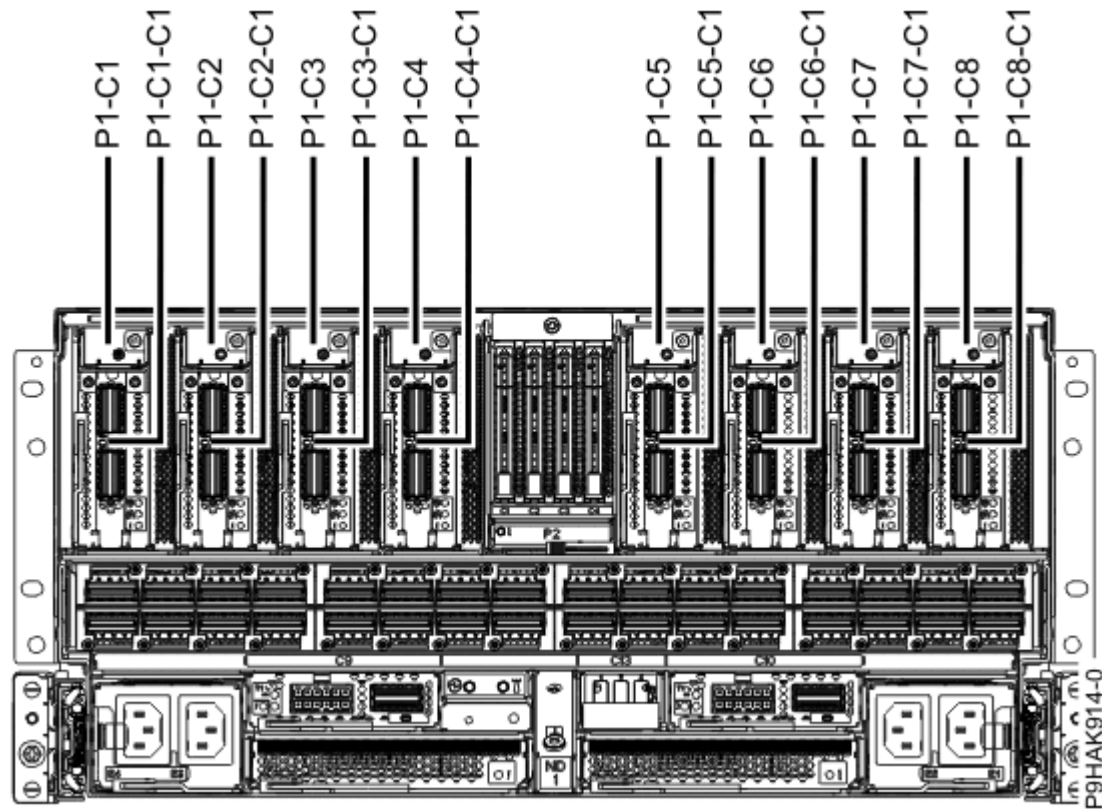
Figura 1. Vista posterior de un sistema 9080-M9S montado en bastidor con los códigos de ubicación de ranuras PCIe
