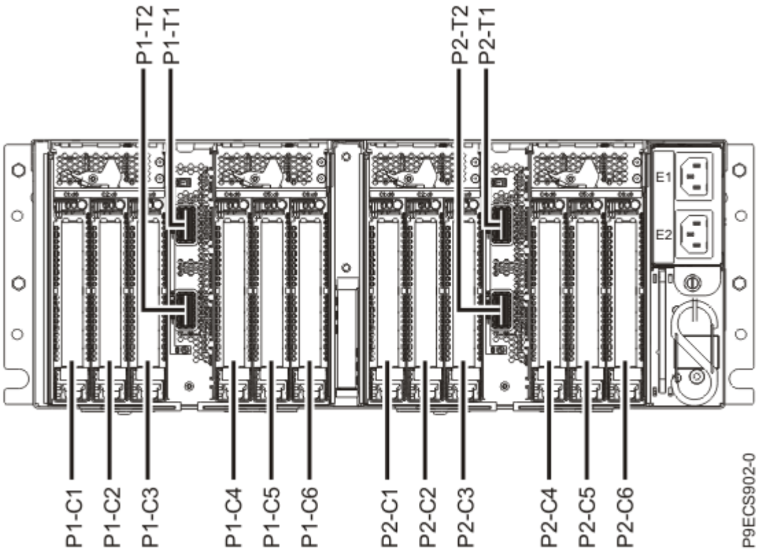
Figura 2. Vista posterior de un cajón de expansión PCIe3 EMX0 con los códigos de ubicación de ranuras PCIe
