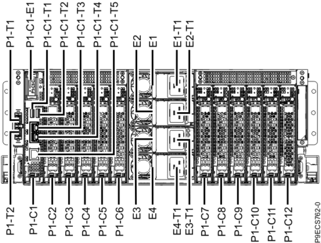
Figura 1. Vista posterior de un sistema 9040-MR9 montado en bastidor con los códigos de ubicación de ranuras PCIe
