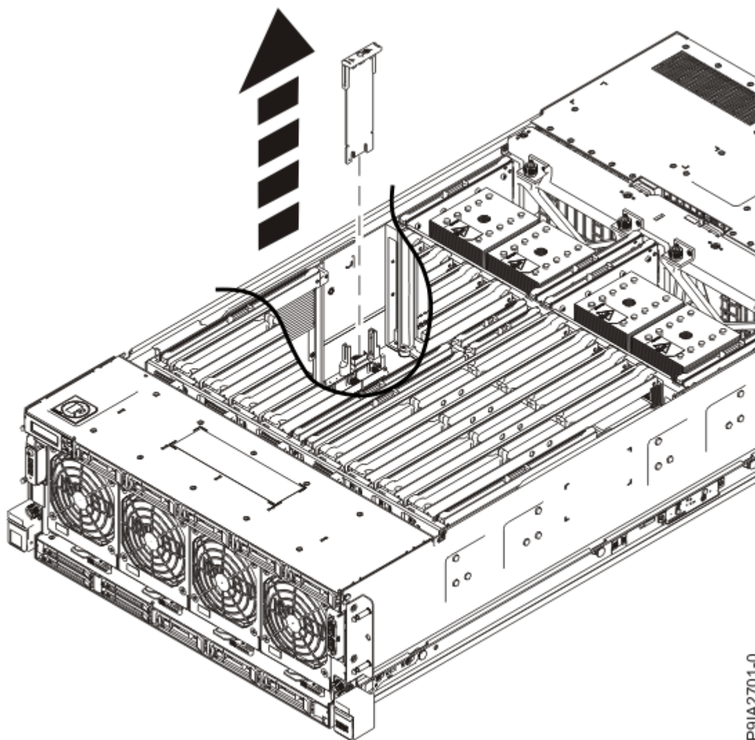
Abbildung 7. TPM-Karte entfernen
