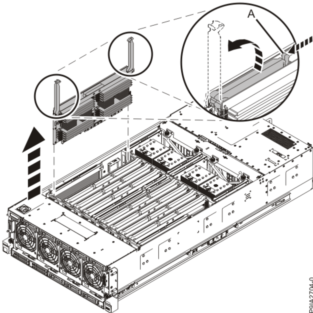
Abbildung 6. Speicherriserkarte an Position P1-C26 entfernen
