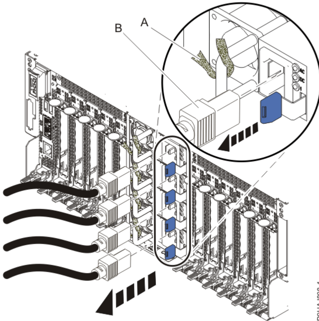
Abbildung 1. Netzkabel abziehen
