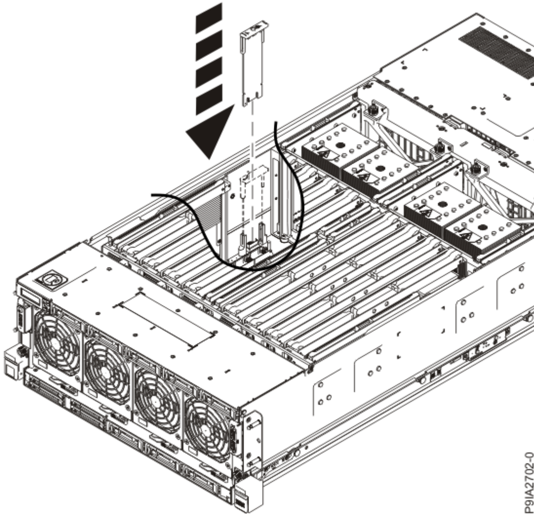
Abbildung 8. TPM-Karte austauschen
