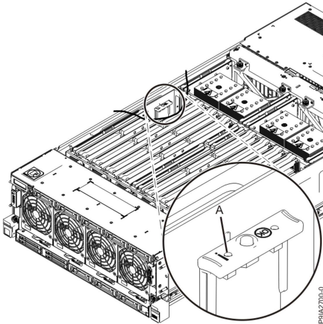
Abbildung 5. Position der Serviceindikator-LED der Trusted Platform Module-Karte
