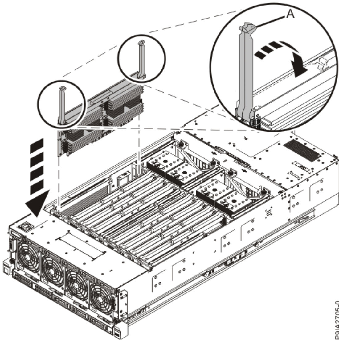
Abbildung 9. Speicherriserkarte an Position P1-C26 austauschen
