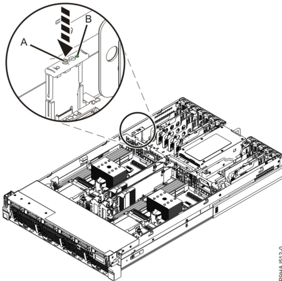
Abbildung 4. Kennzeichnungs-LED aktivieren
