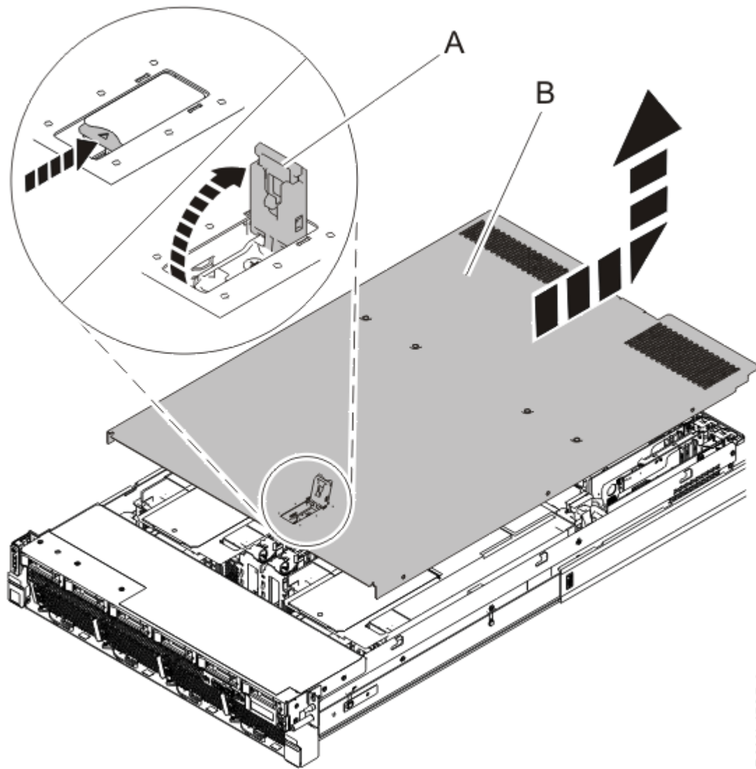
Abbildung 3. Serviceabdeckung ausbauen
