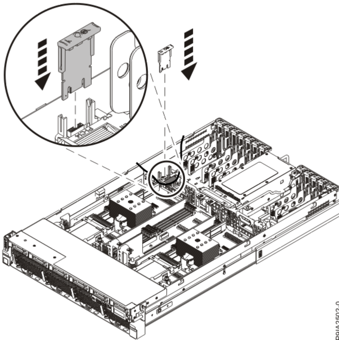
Abbildung 7. TPM-Karte austauschen
