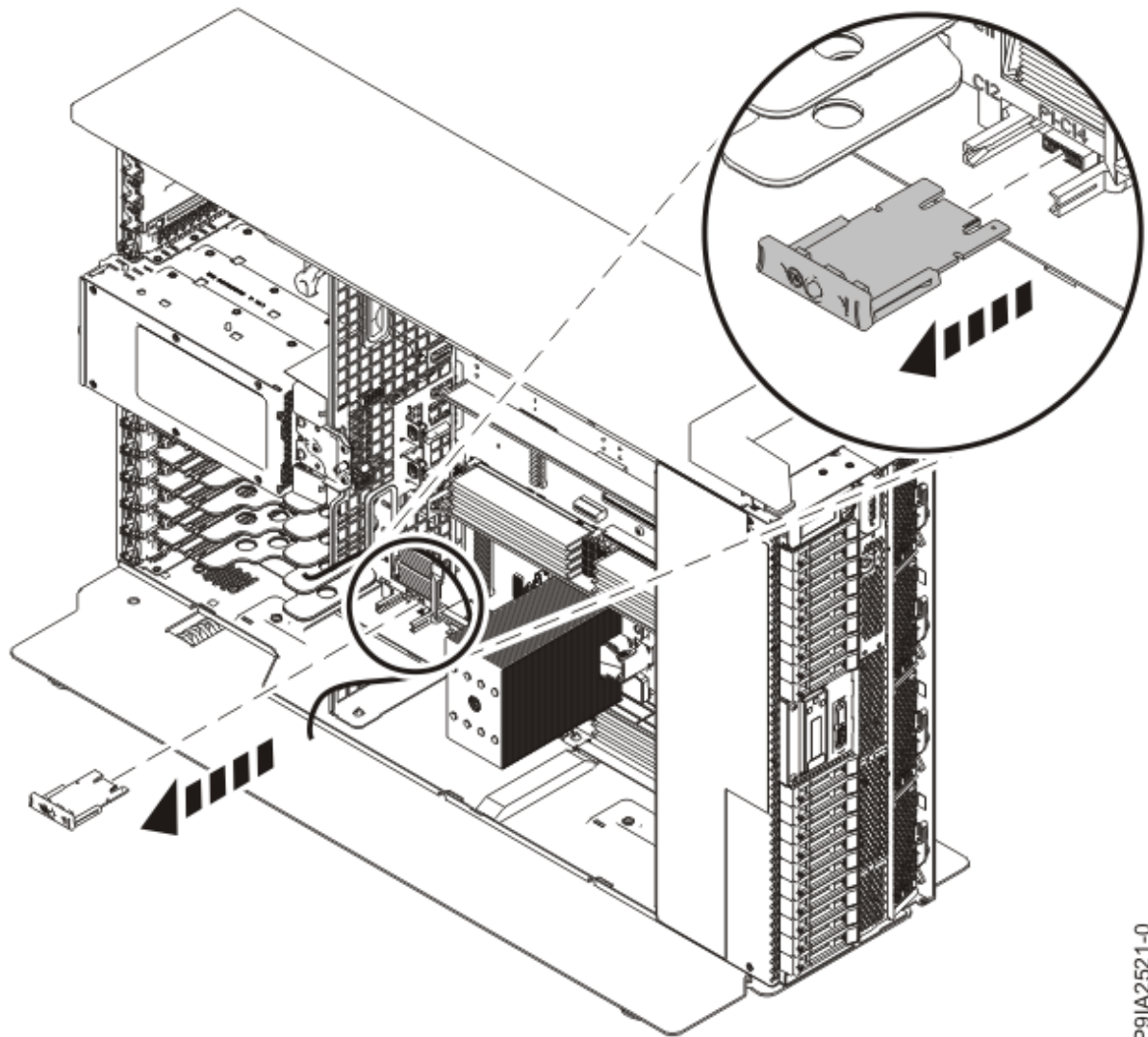
Abbildung 11. TPM-Karte aus einem Standalone-System entfernen
