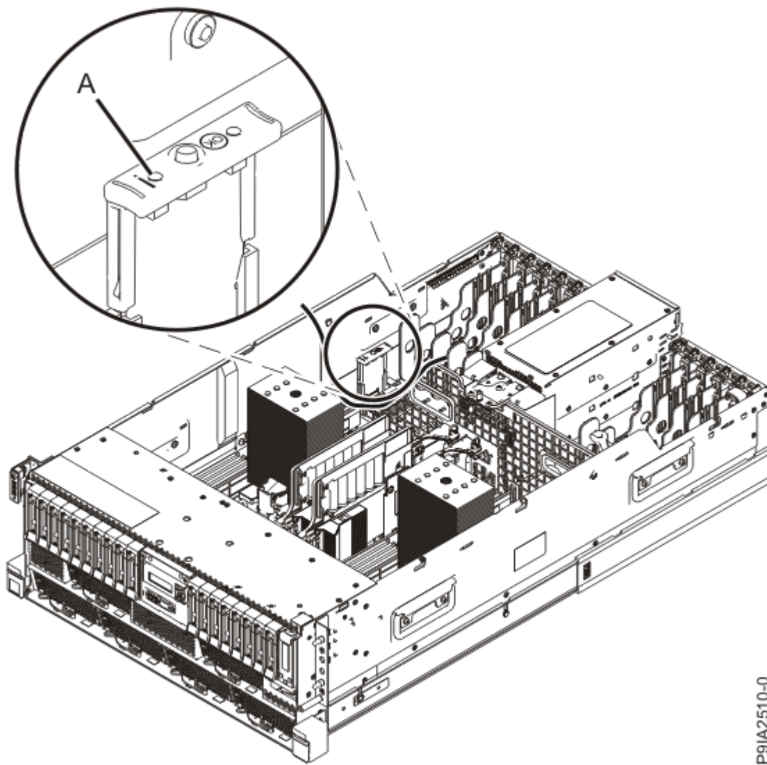
Abbildung 8. Position der Serviceindikator-LED der Trusted Platform Module-Karte bei einem Einschubserver
