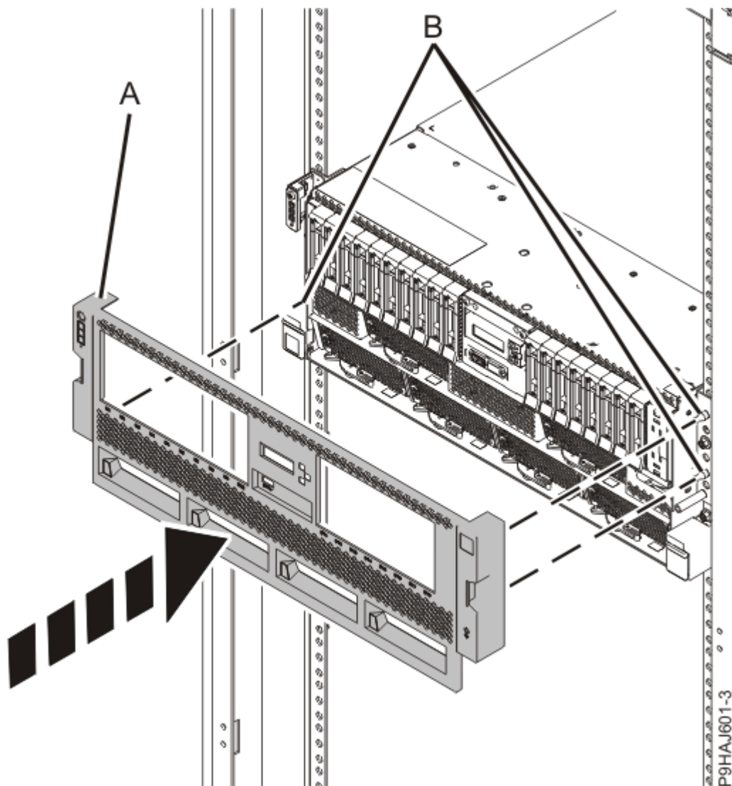
Abbildung 17. Vordere Abdeckung installieren
