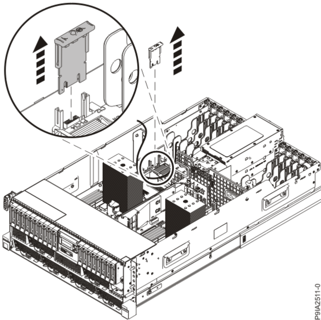
Abbildung 10. TPM-Karte aus einem Einschubsystem entfernen
