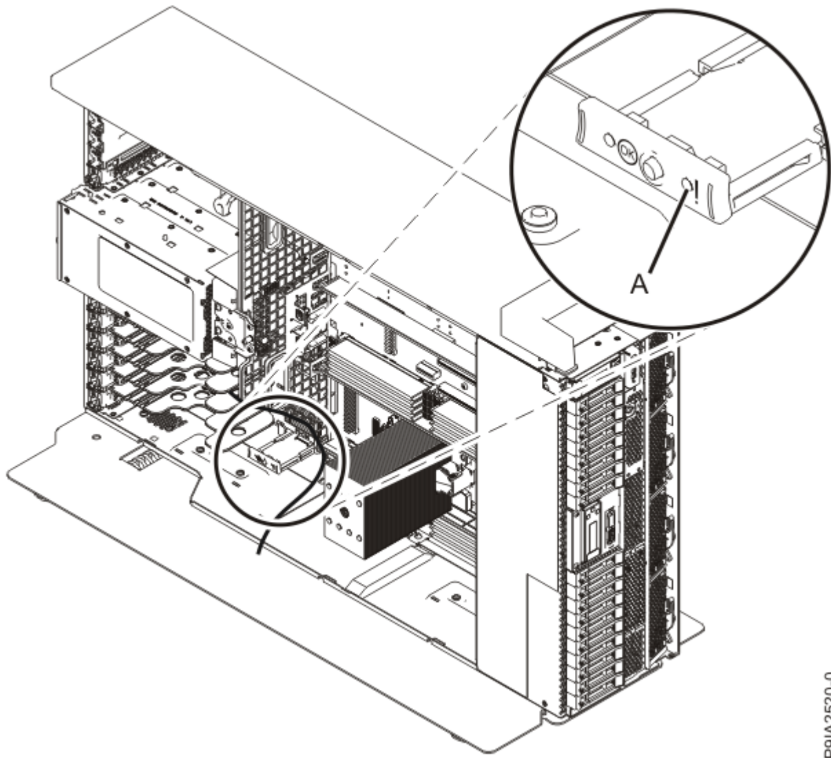
Abbildung 9. Position der Serviceindikator-LED der Trusted Platform Module-Karte bei einem Standalone-Server
