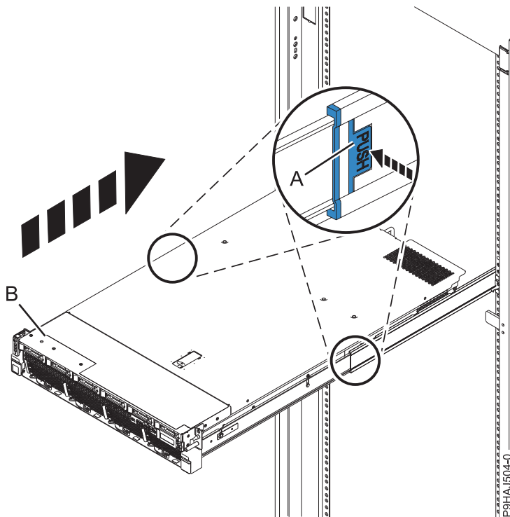
Abbildung 38. System in die Betriebsposition bringen
