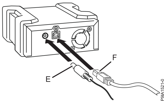
Abbildung 3. Rückansicht einer externen RDX-Andockstation und der zugehörigen Kabel
