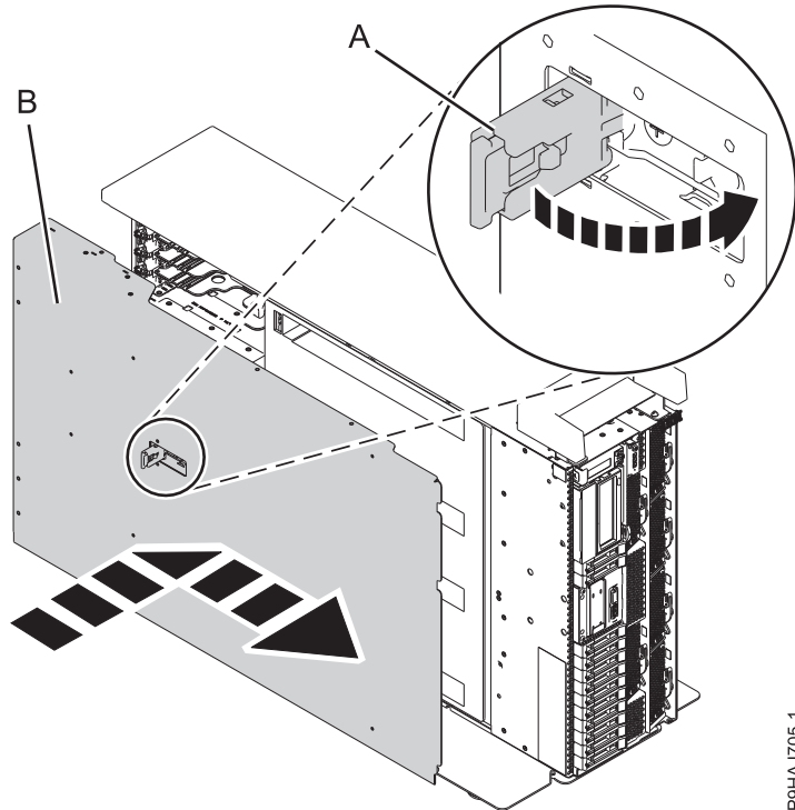
Abbildung 30. Serviceabdeckung installieren
