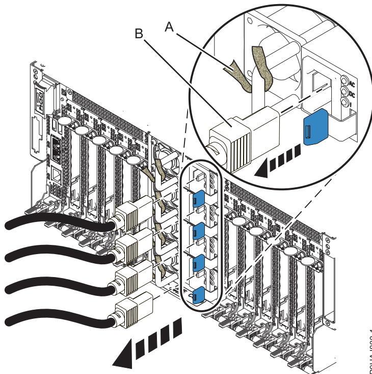
Abbildung 42. Netzkabel abziehen
