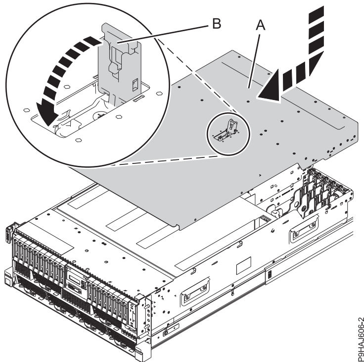
Abbildung 29. Serviceabdeckung installieren
