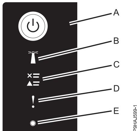
Abbildung 4. Anzeigen der Steuerkonsole
