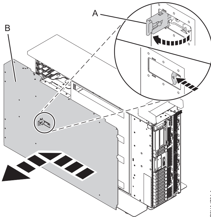
Abbildung 27. Serviceabdeckung ausbauen
