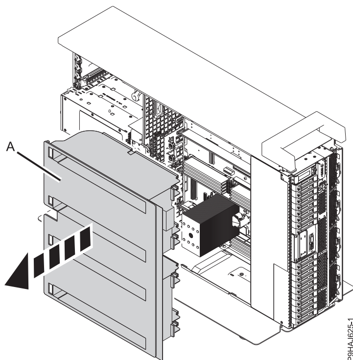
Abbildung 34. Luftführung aus einem Standalone-System ausbauen
