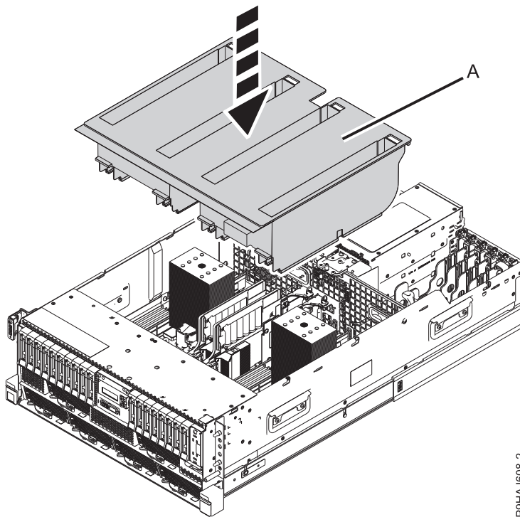
Abbildung 35. Luftführung bei einem Einschubsystem wiedereinbauen
