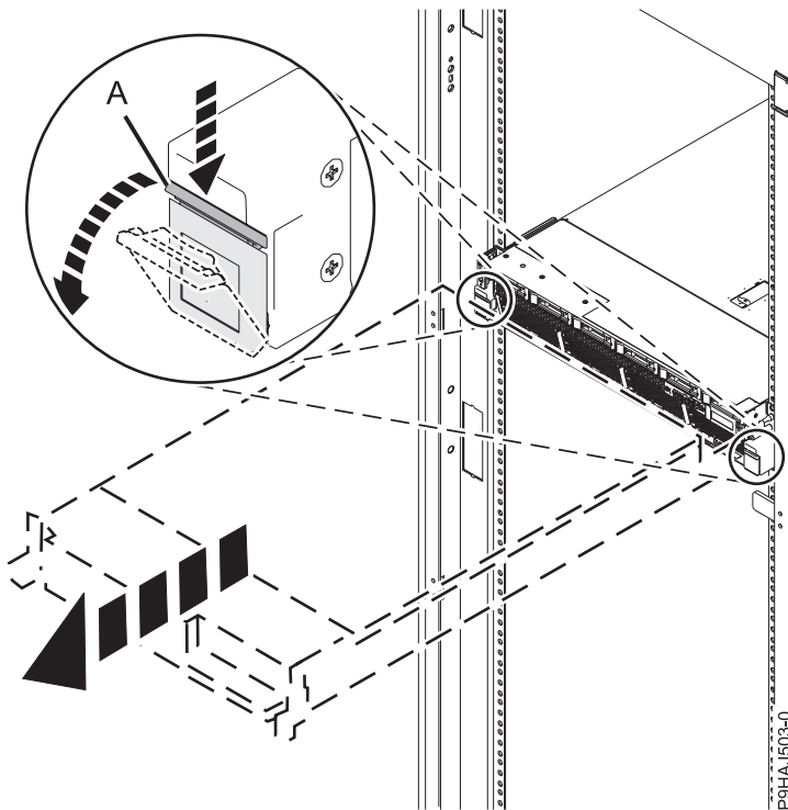
Abbildung 37. Seitliche Verriegelungen entriegeln
