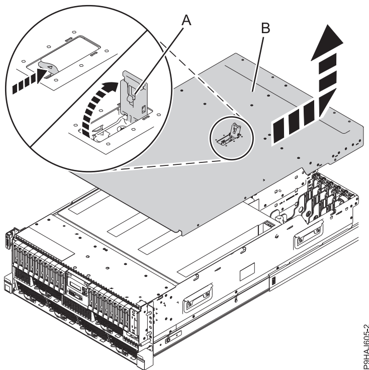
Abbildung 26. Serviceabdeckung eines Einschubsystems ausbauen
