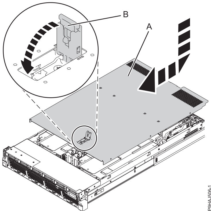
Abbildung 28. Serviceabdeckung installieren
