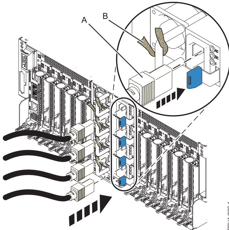
Abbildung 46. Netzkabel anschließen
