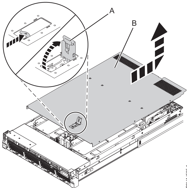
Abbildung 25. Serviceabdeckung ausbauen
