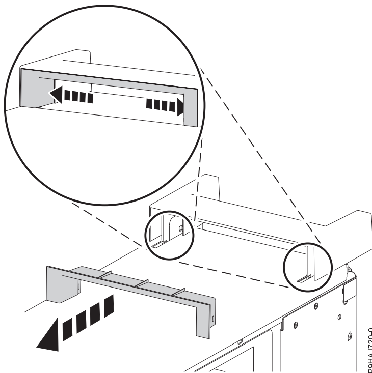
Abbildung 12. Plastikelement von der Griffabdeckung entfernen
