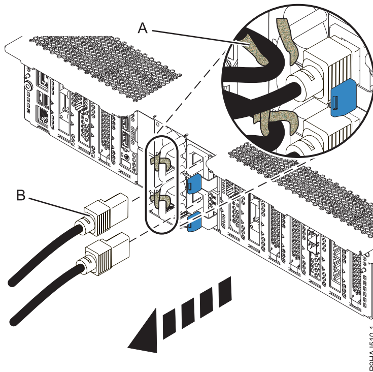
Abbildung 39. Netzkabel abziehen
