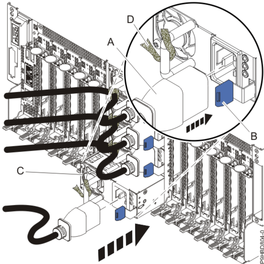
Abbildung 5. Netzteil austauschen
