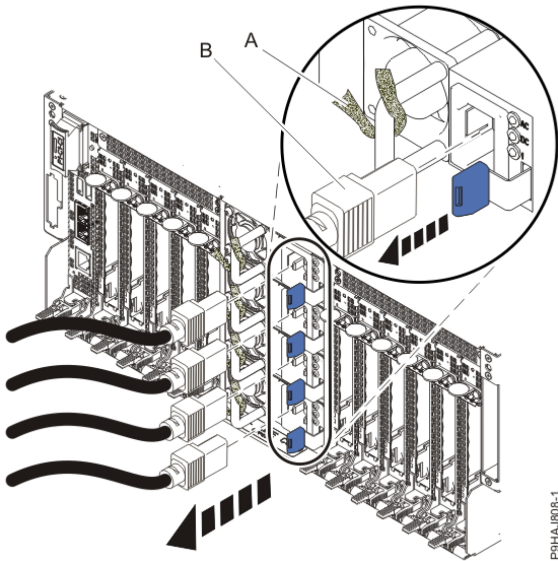
Abbildung 3. Netzkabel abziehen
