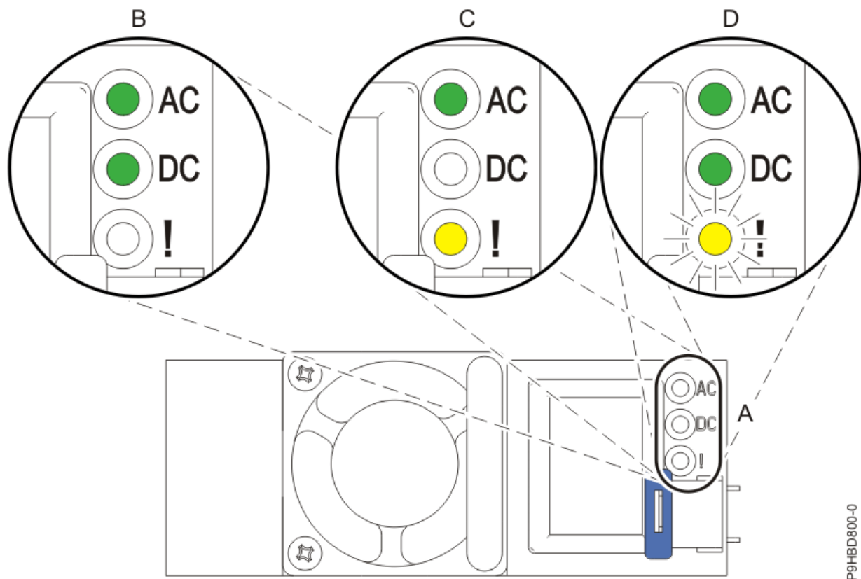
Abbildung 2. LEDs für ein funktionierendes (B) und ein fehlerhaftes (C, D) Netzteil in einem Einschubsystem
