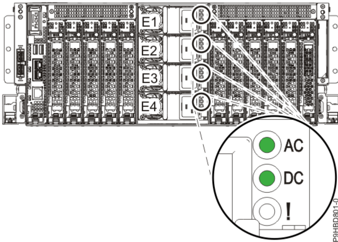
Abbildung 6. LEDs für ein funktionierendes Netzteil
