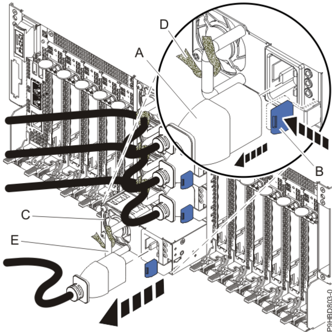
Abbildung 4. Netzteil entfernen
