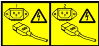
Abbildung 3. Netzkabel abziehen
