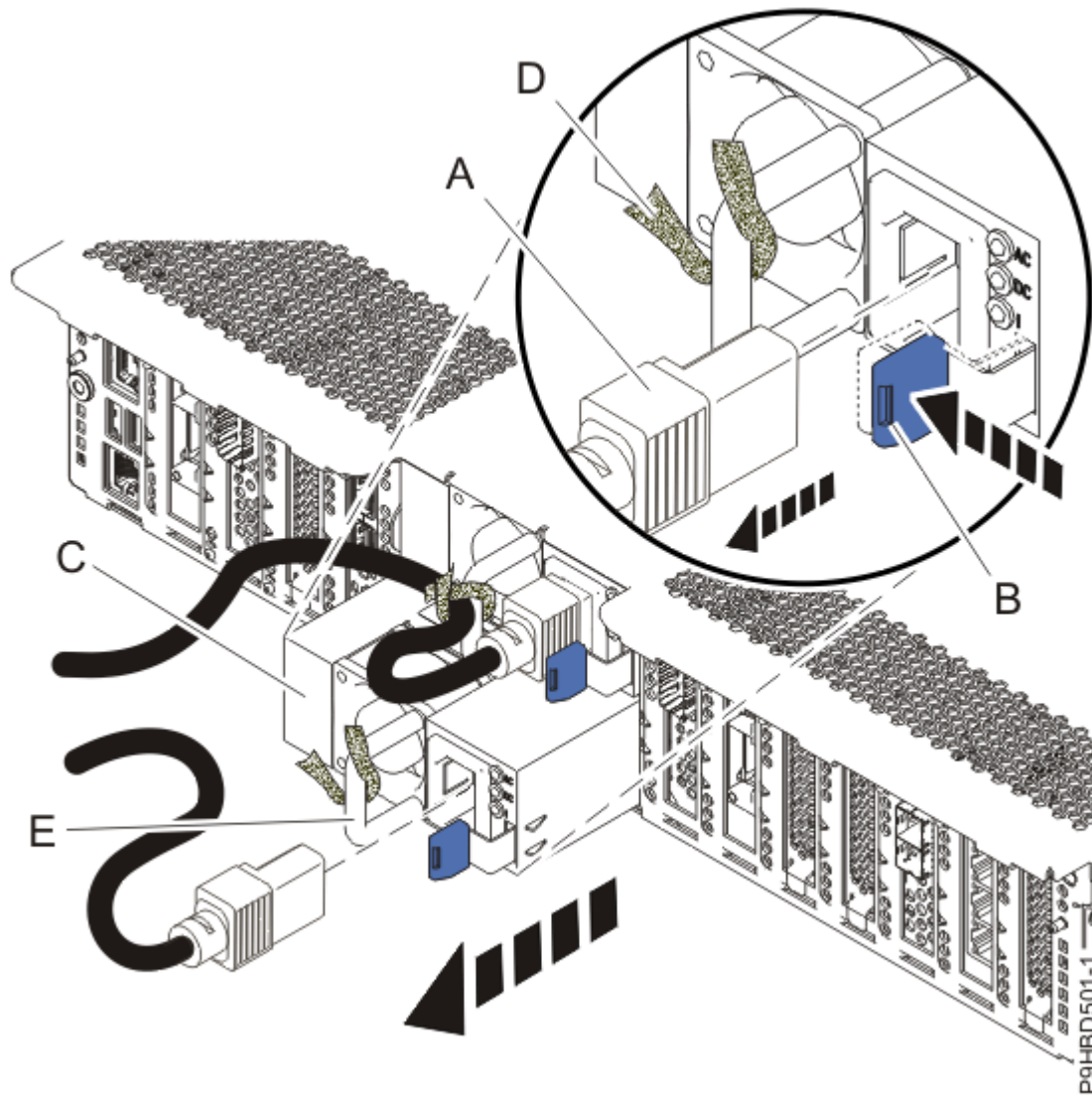
Abbildung 5. Netzteil ausbauen
