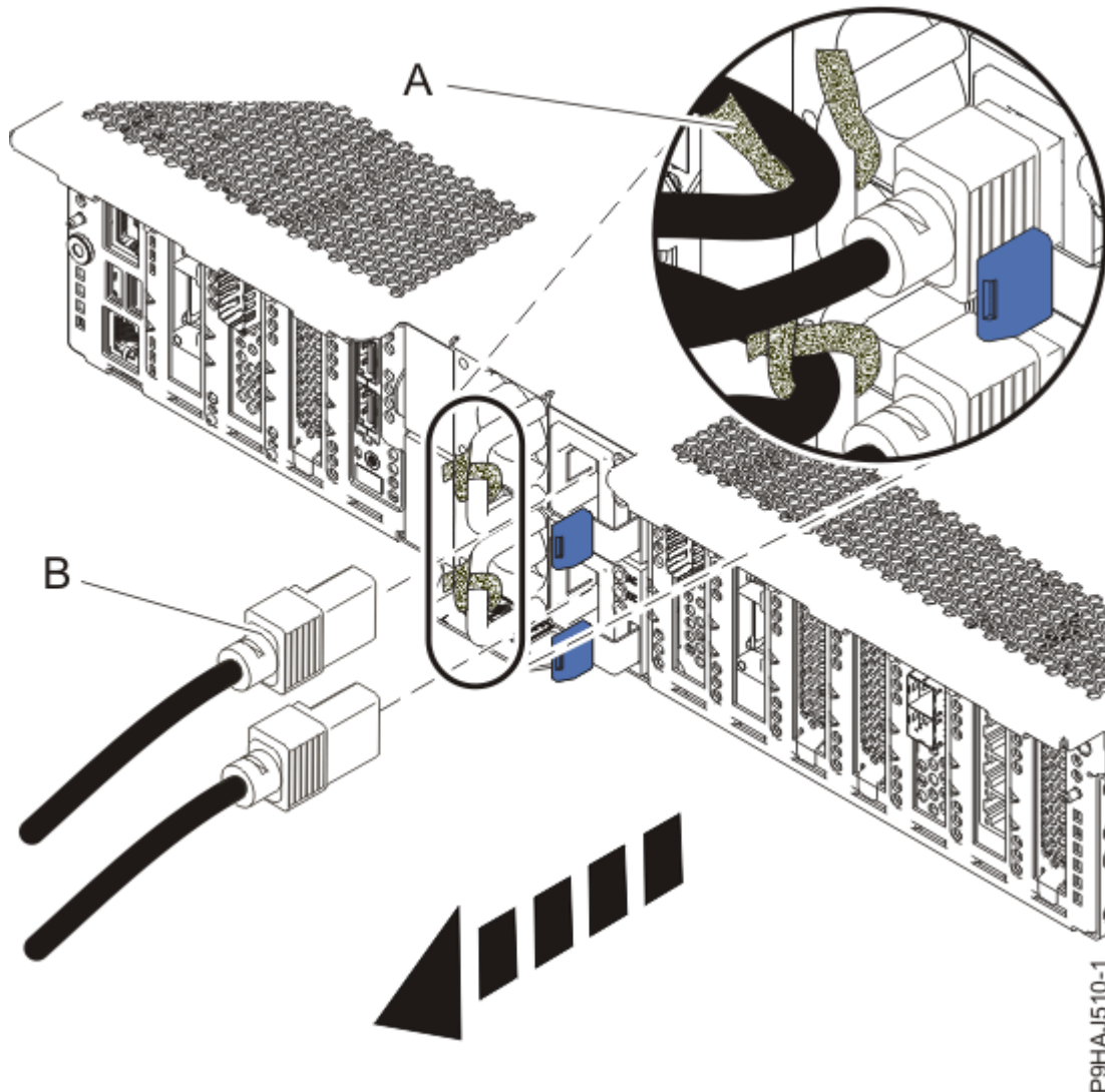
Abbildung 3. Netzkabel abziehen
