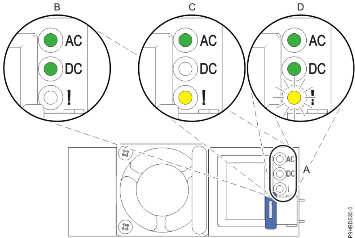
Abbildung 2. LEDs für ein funktionierendes (B) und ein fehlerhaftes (C, D) Netzteil
