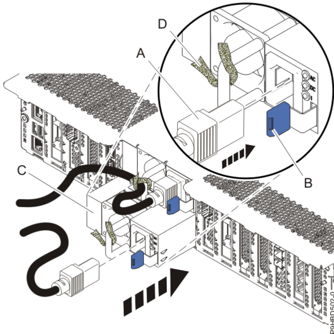
Abbildung 6. Netzteil austauschen
