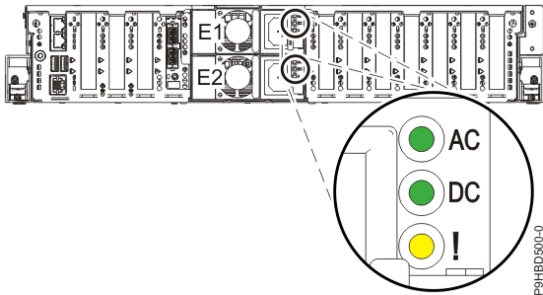
Abbildung 1. Position der Netzteile und LEDs im System
