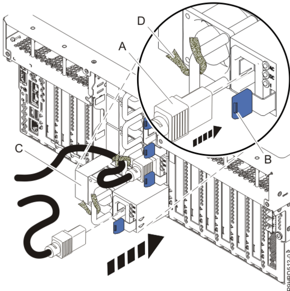
Abbildung 9. Netzteil austauschen
