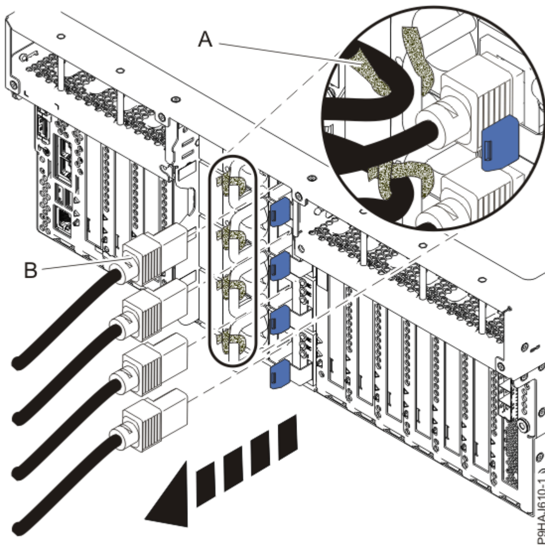
Abbildung 5. Netzkabel von einem Einschubserver abziehen
