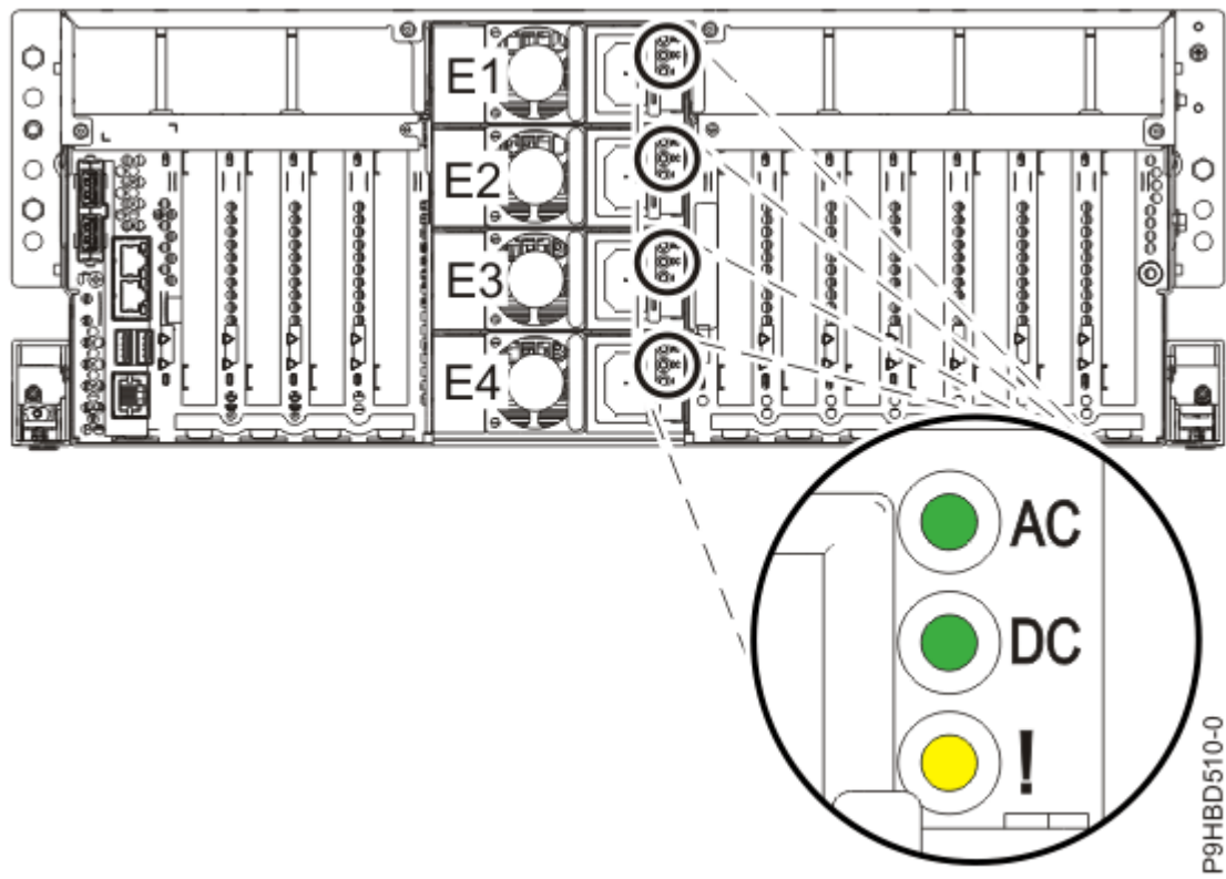
Abbildung 1. Position der Netzteile und LEDs im Einschubsystem
