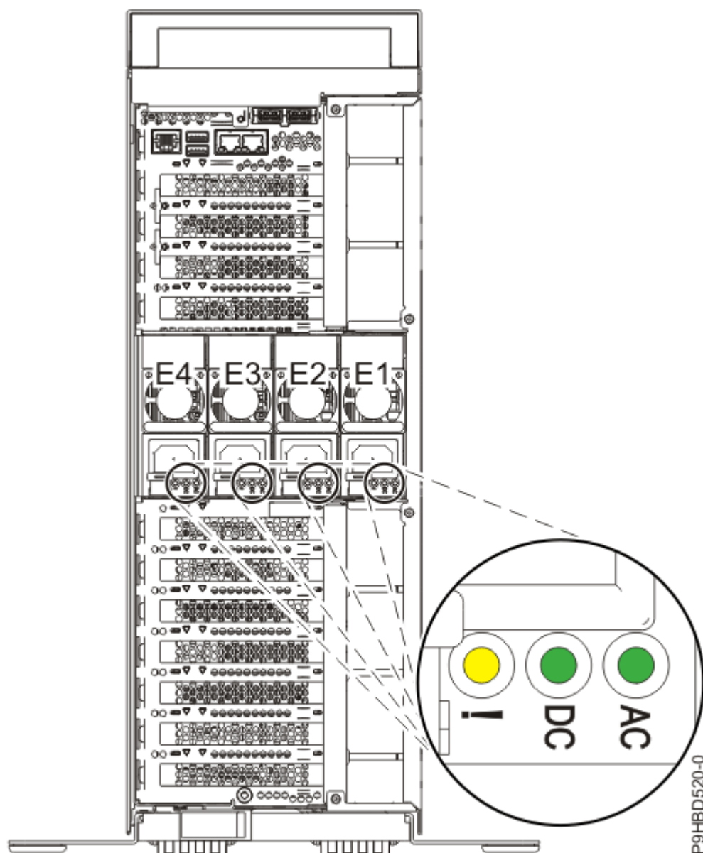
Abbildung 2. Position der Netzteile und LEDs im Standalone-System
