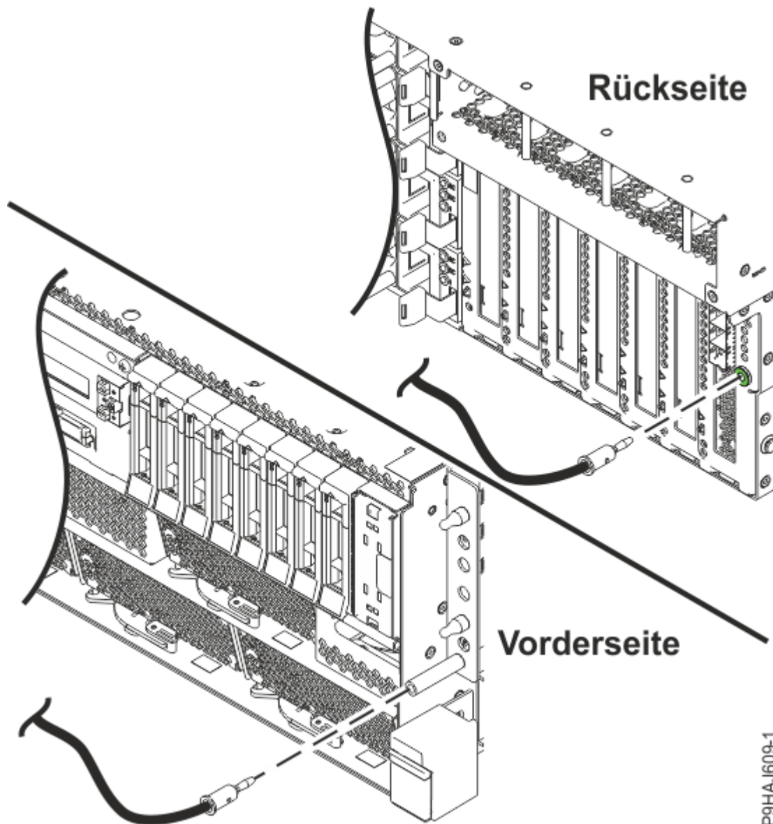
Abbildung 7. Position der ESD-Stecker
