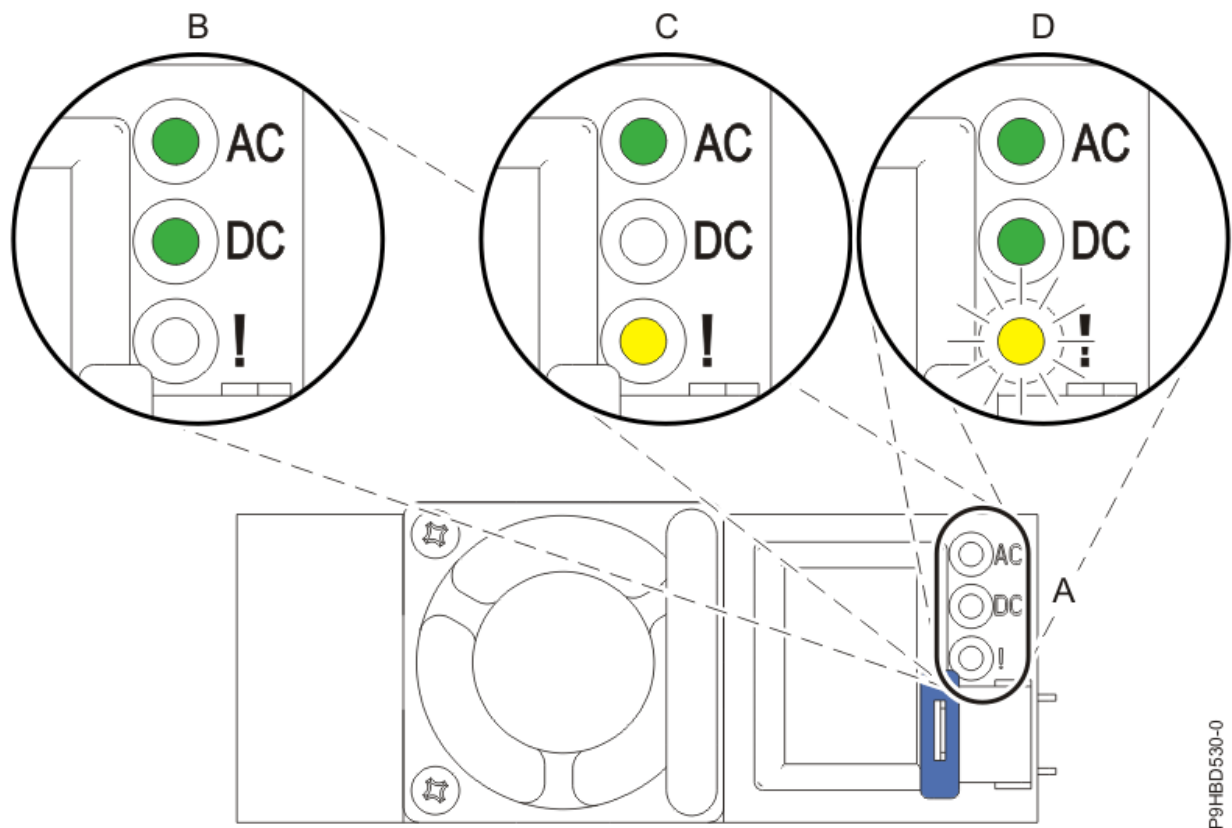
Abbildung 3. LEDs für ein funktionierendes (B) und ein fehlerhaftes (C, D) Netzteil in einem Einschubsystem
