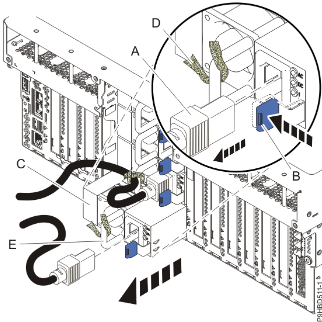
Abbildung 8. Netzteil ausbauen
