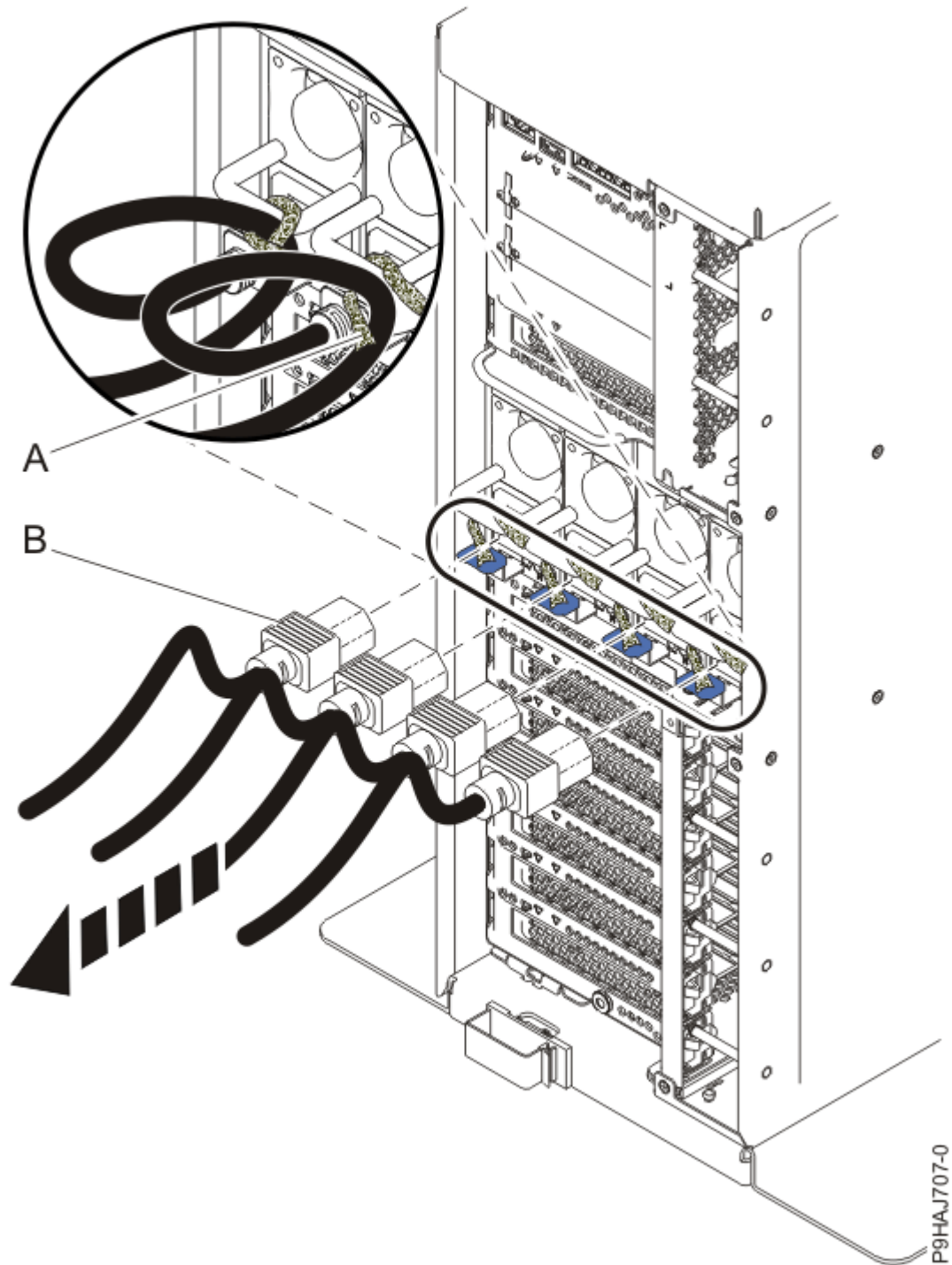
Abbildung 6. Netzkabel von einem Standalone-Server abziehen
