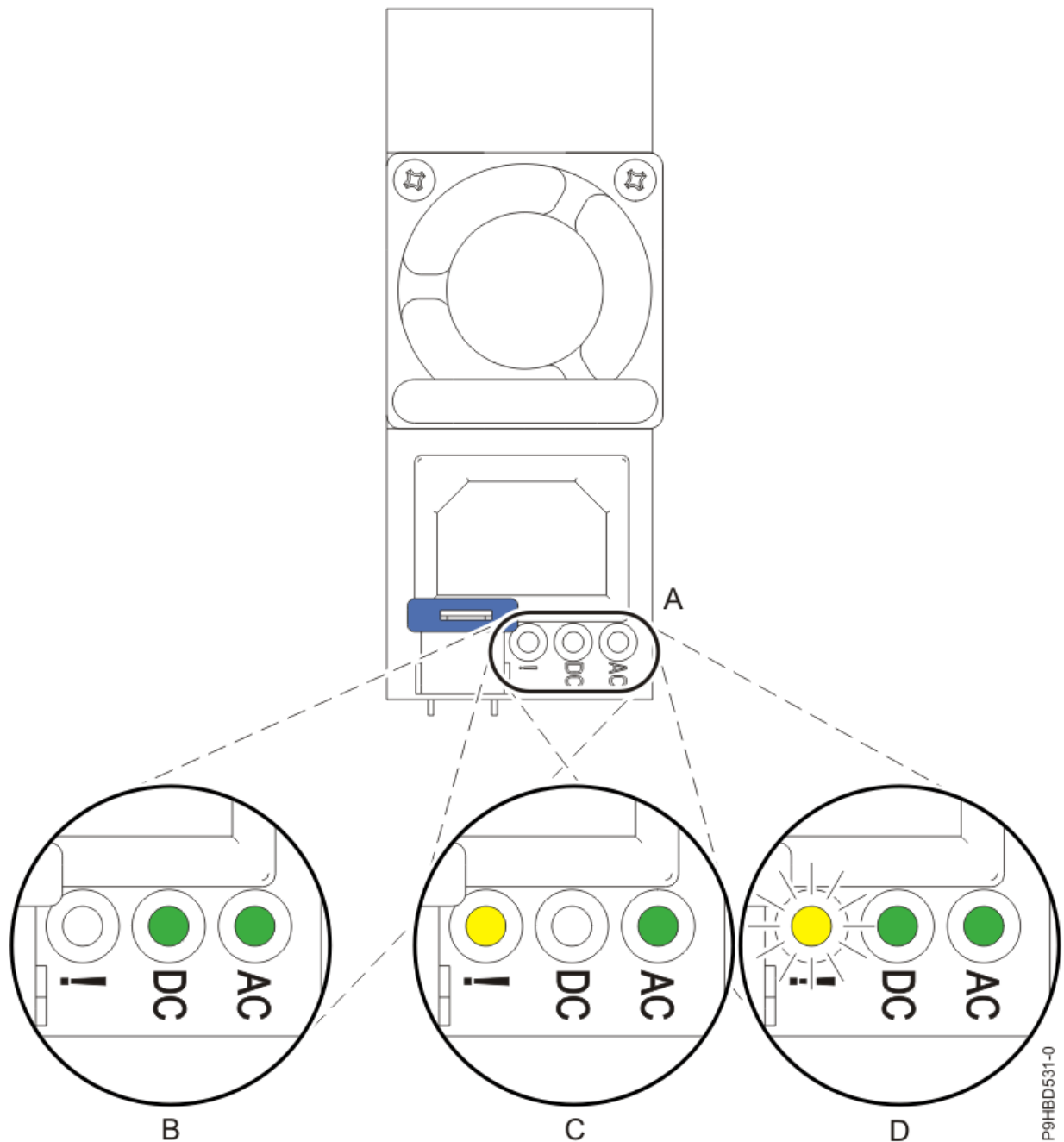
Abbildung 4. LEDs für ein funktionierendes ( B ) und ein fehlerhaftes ( C, D ) Netzteil in einem Standalone-System
