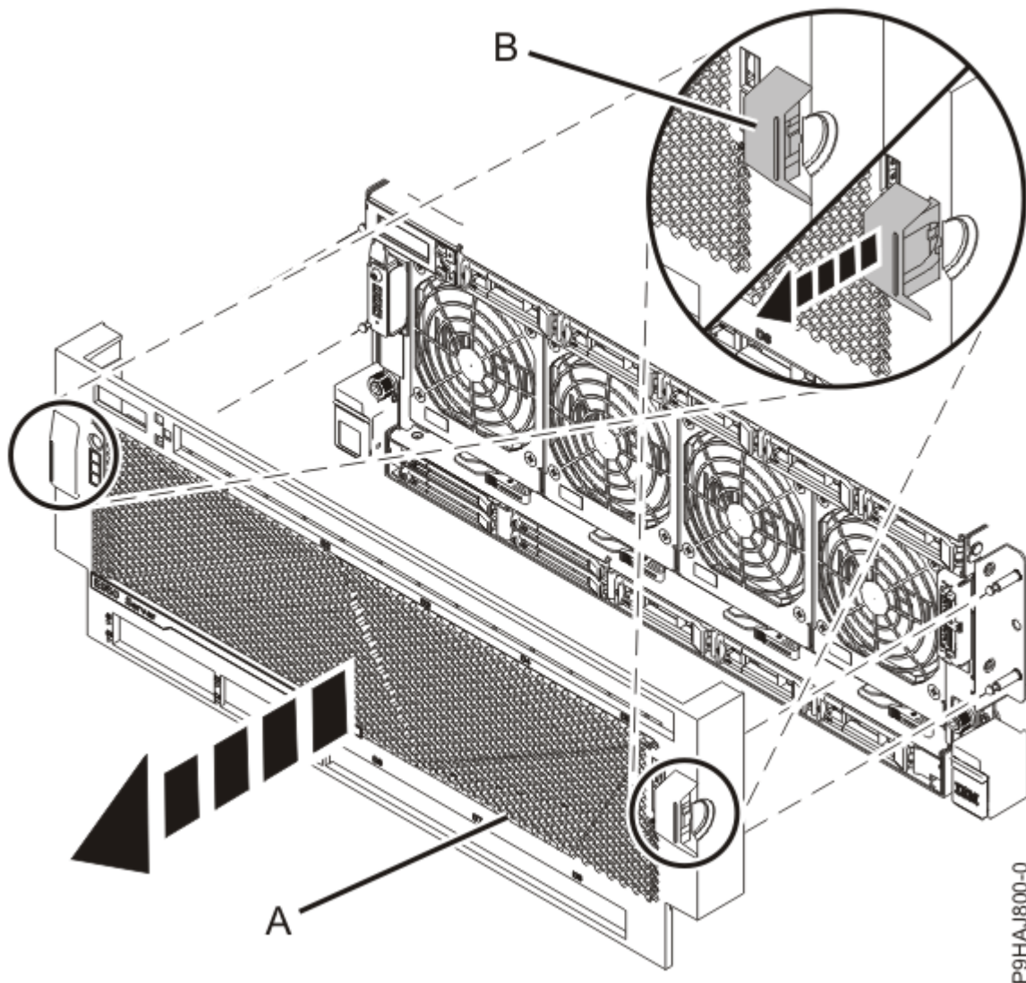
Abbildung 7. Vordere Abdeckung ausbauen
