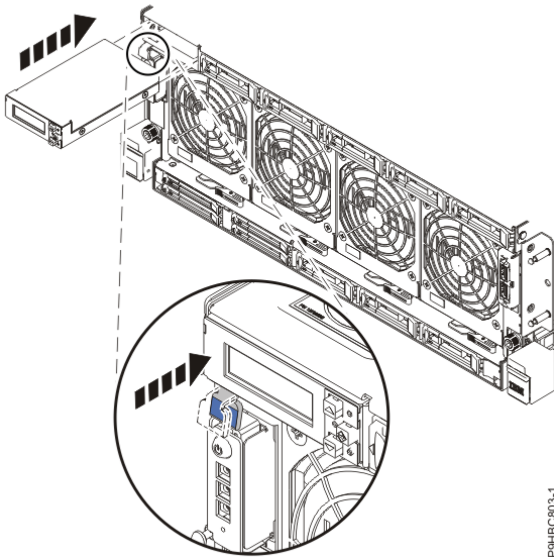
Abbildung 9. Steuerkonsolenanzeige austauschen
