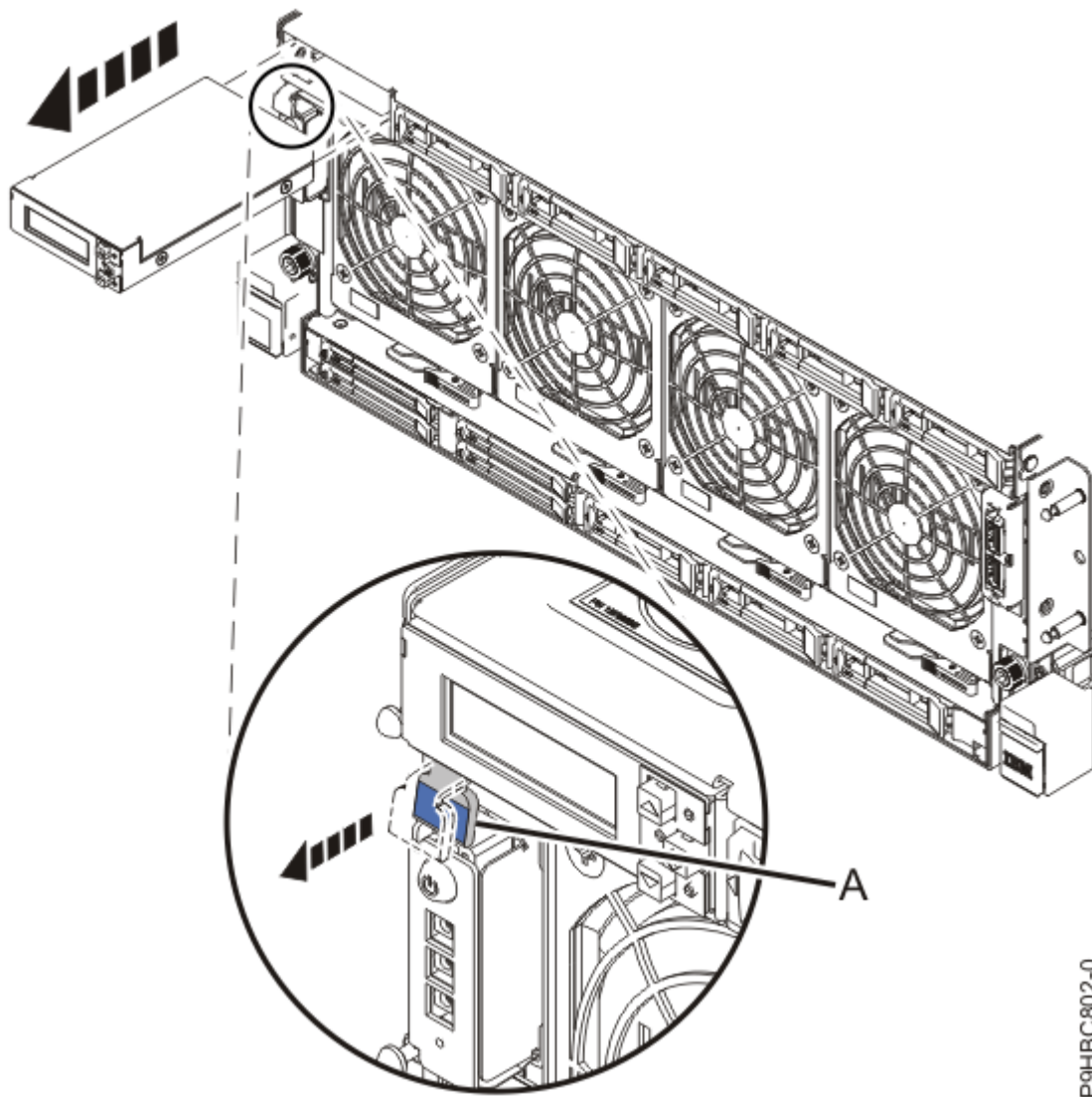
Abbildung 8. Steuerkonsolenanzeige ausbauen
