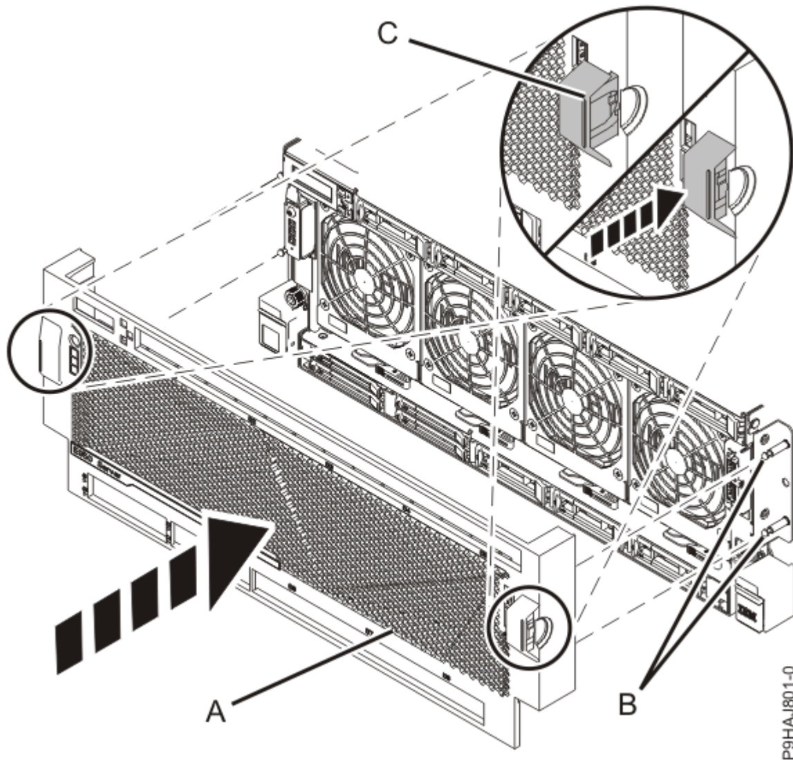
Abbildung 5. Vordere Abdeckung installieren
