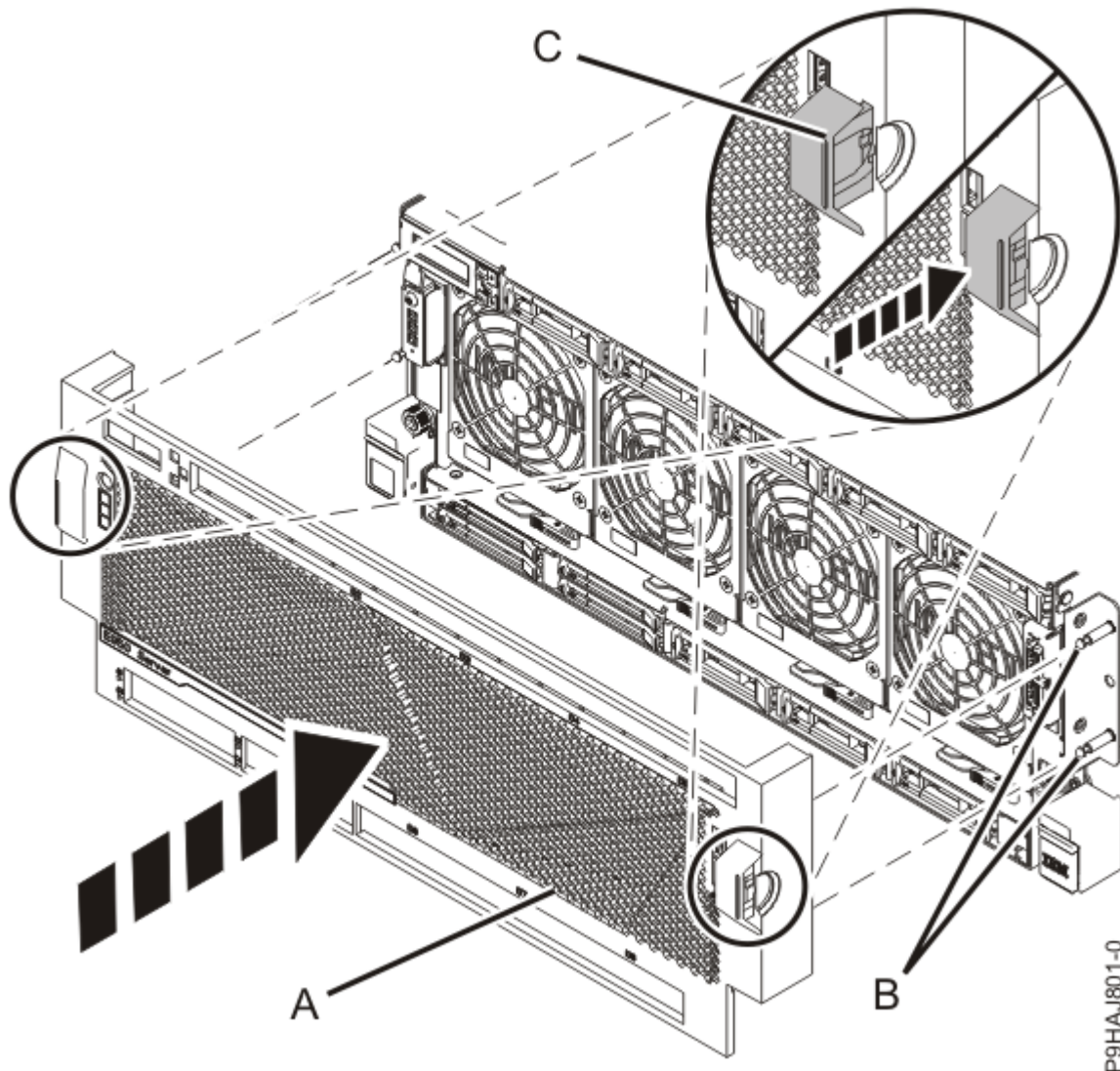
Abbildung 10. Vordere Abdeckung installieren
