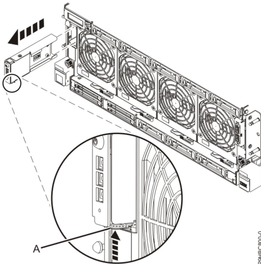
Abbildung 3. Steuerkonsole ausbauen
