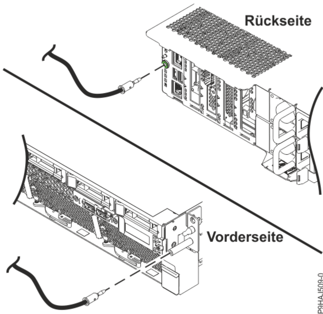
Abbildung 19. Position der ESD-Stecker
