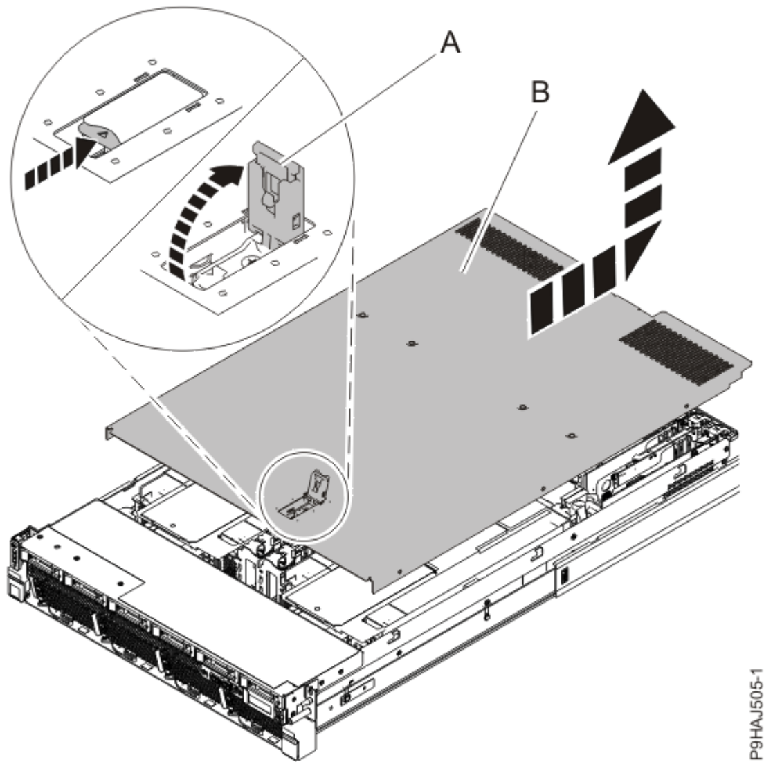
Abbildung 6. Serviceabdeckung ausbauen
