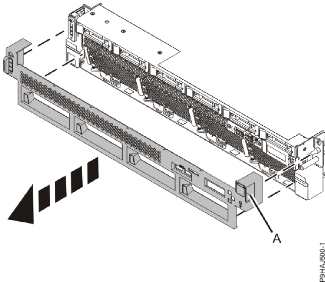
Abbildung 18. Vordere Abdeckungen ausbauen
