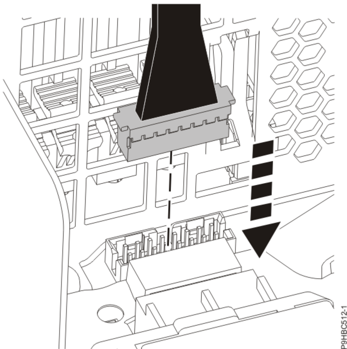
Abbildung 41. Steuerkonsolenkabel an der Systemrückwandplatine anschließen
