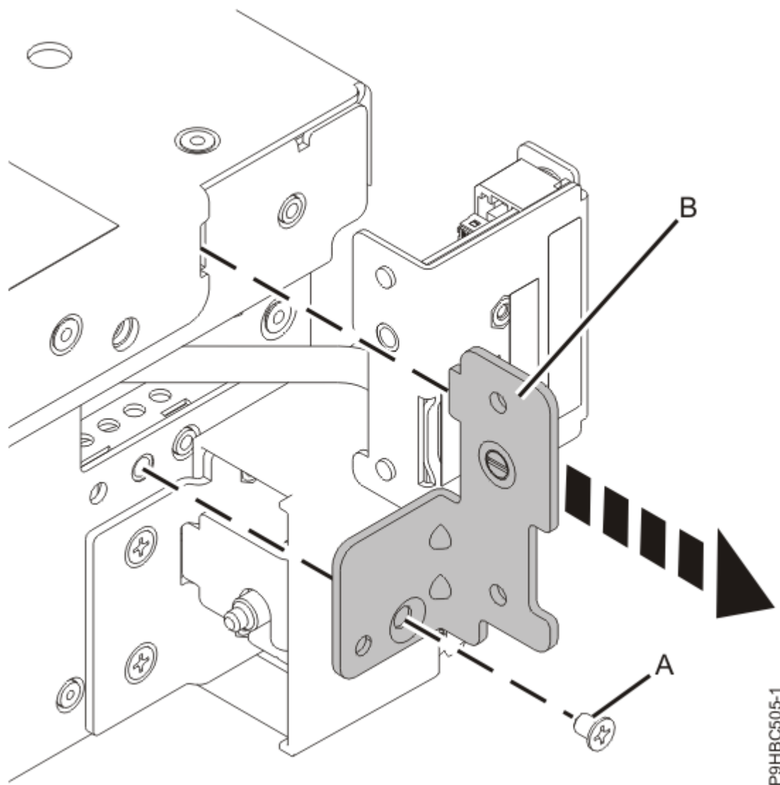
Abbildung 33. Steuerkonsolenhalterung ausbauen
