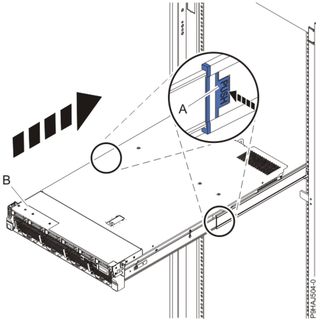
Abbildung 65. System in die Betriebsposition bringen
