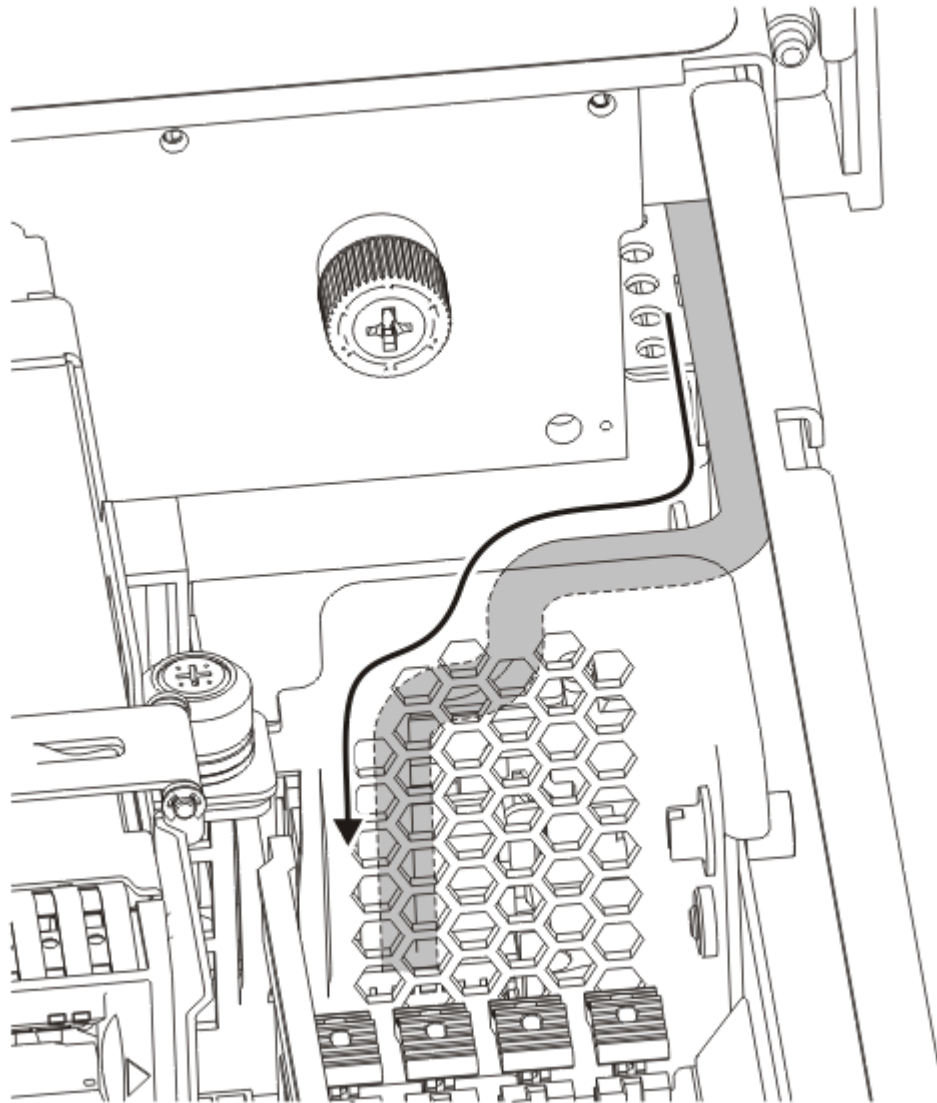
Abbildung 38. Steuerkonsolenkabelpfad
