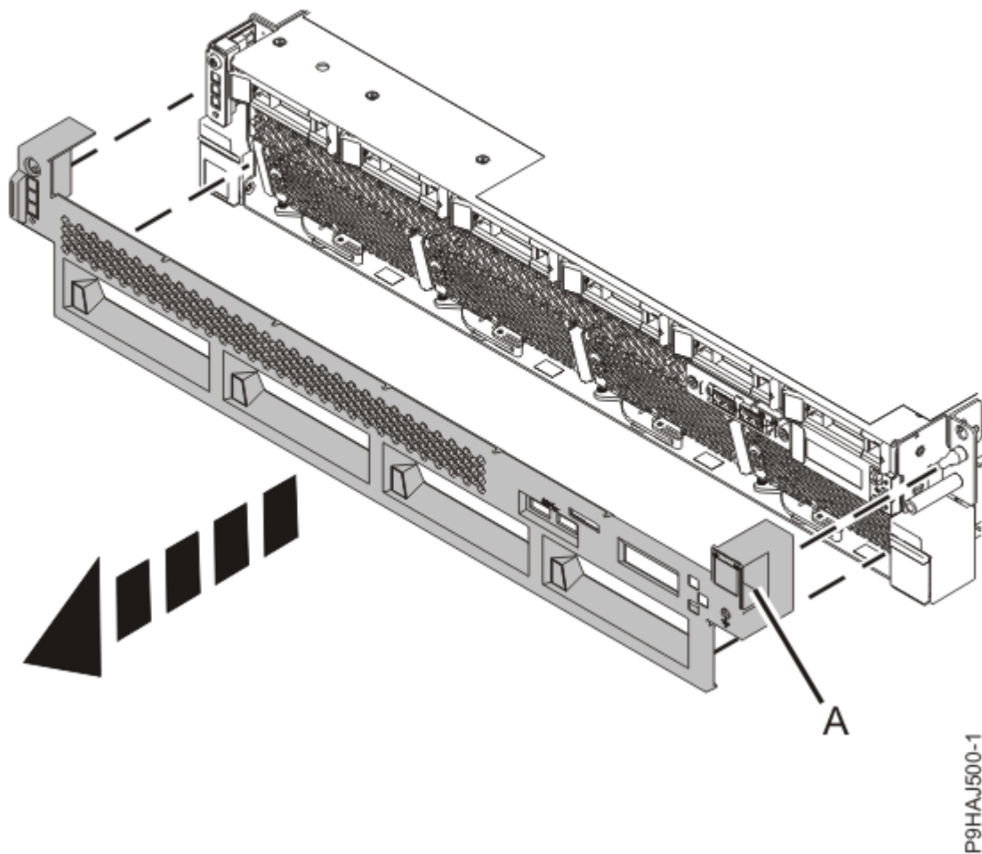
Abbildung 3. Vordere Abdeckungen ausbauen
