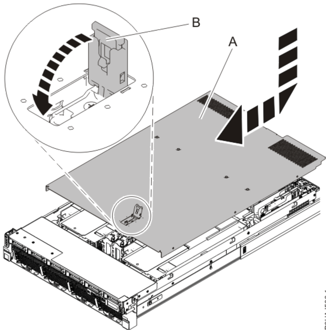
Abbildung 43. Serviceabdeckung installieren
