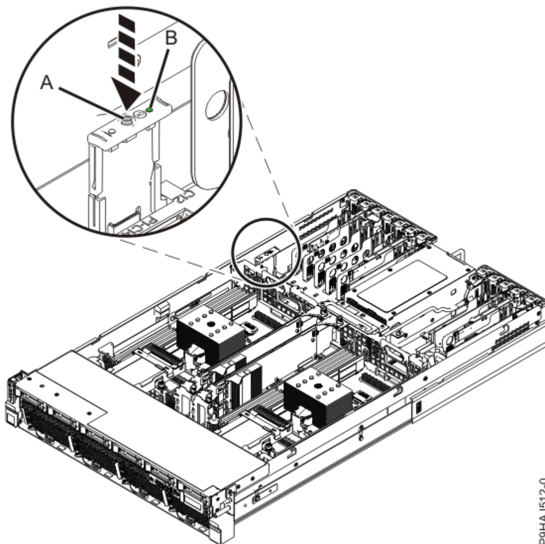
Abbildung 7. Kennzeichnungs-LED aktivieren
