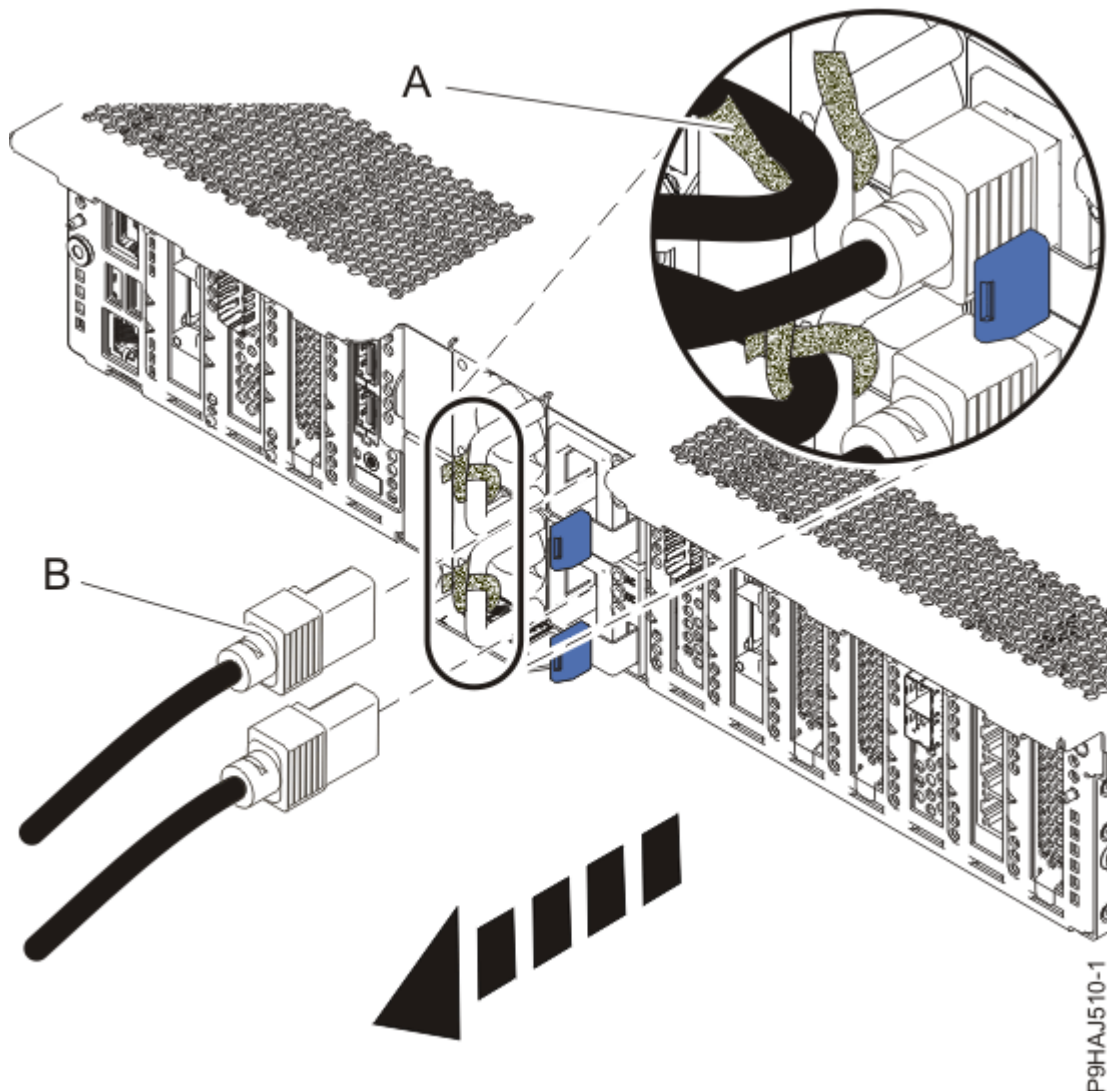
Abbildung 2. Netzkabel abziehen
