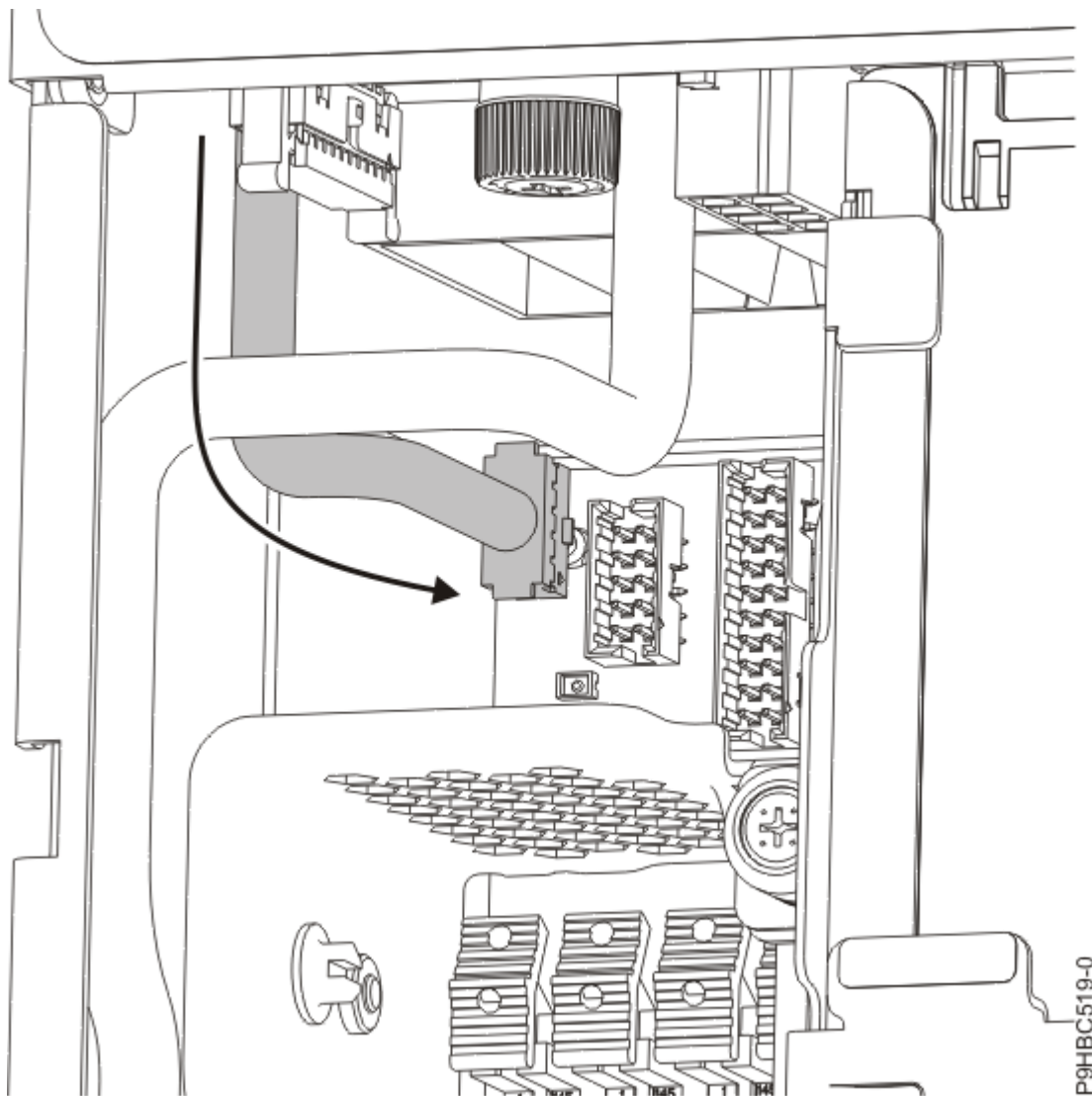
Abbildung 59. Steuerkonsolenanzeigekabelpfad
