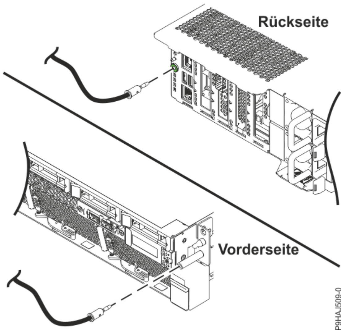
Abbildung 5. Position der ESD-Stecker
