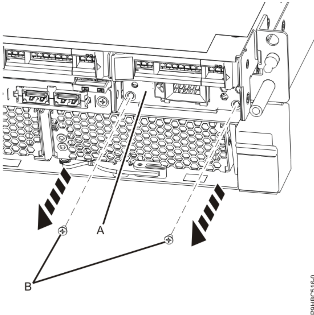
Abbildung 56. Steuerkonsolenanzeigehalter an der Halterung ausbauen
