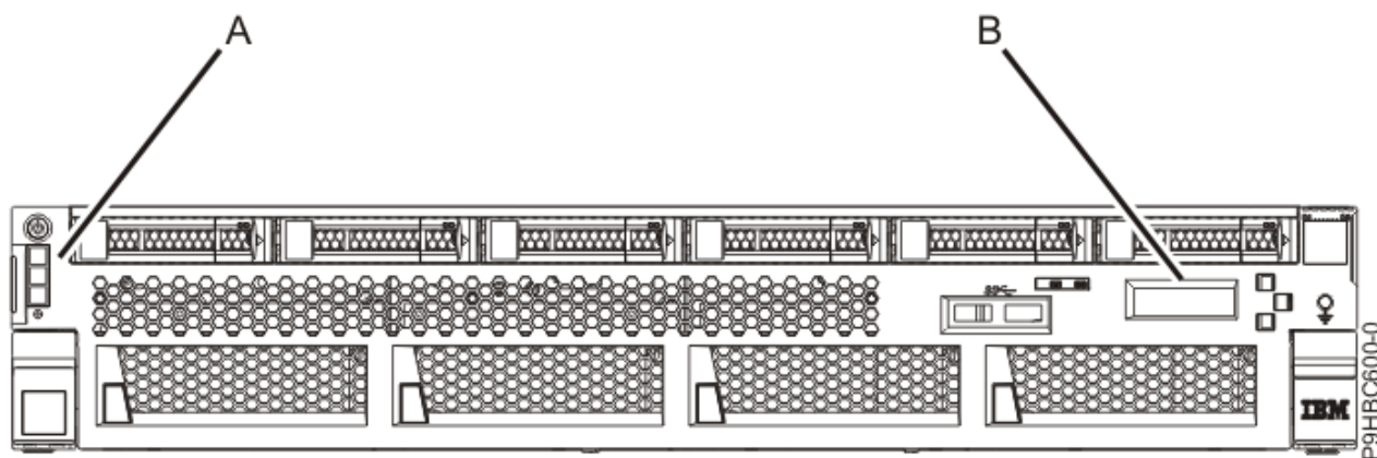
Abbildung 1. Steuerkonsolen
