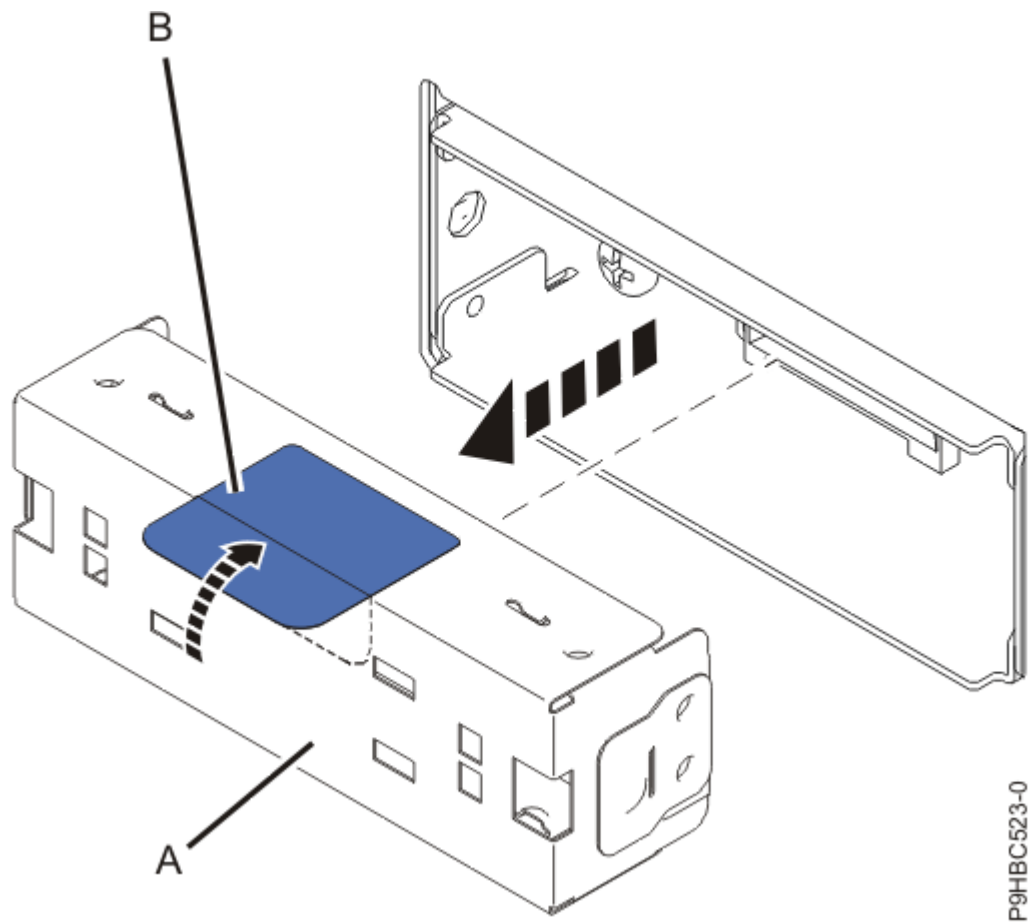
Abbildung 22. Anzeigen-Platzhalterelement ausbauen
