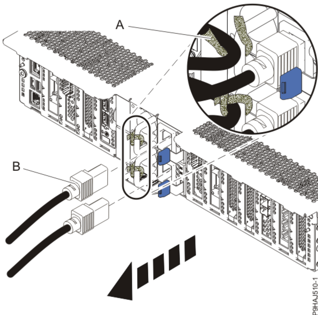
Abbildung 25. Netzkabel abziehen
