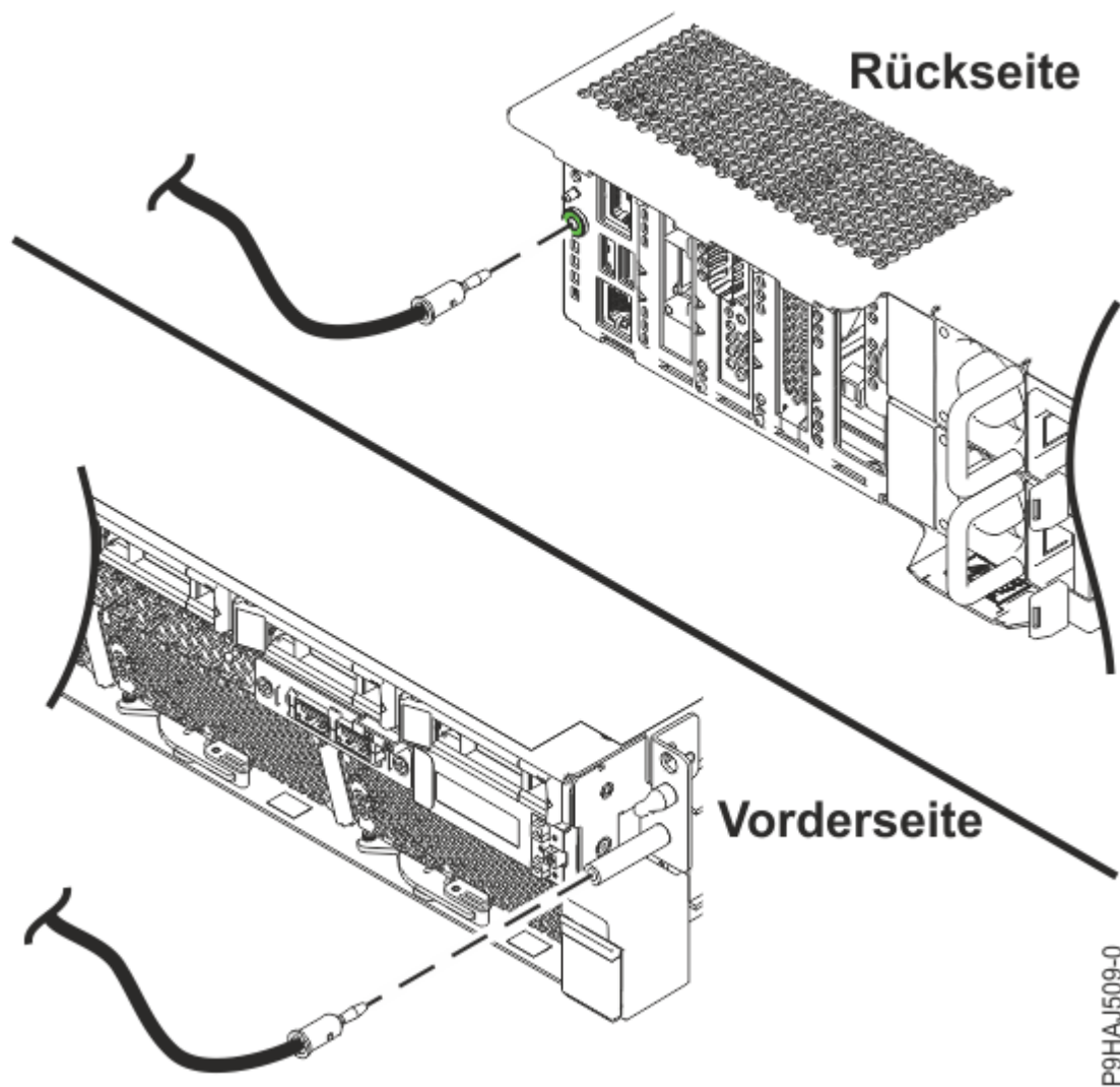
Abbildung 28. Position der ESD-Stecker
