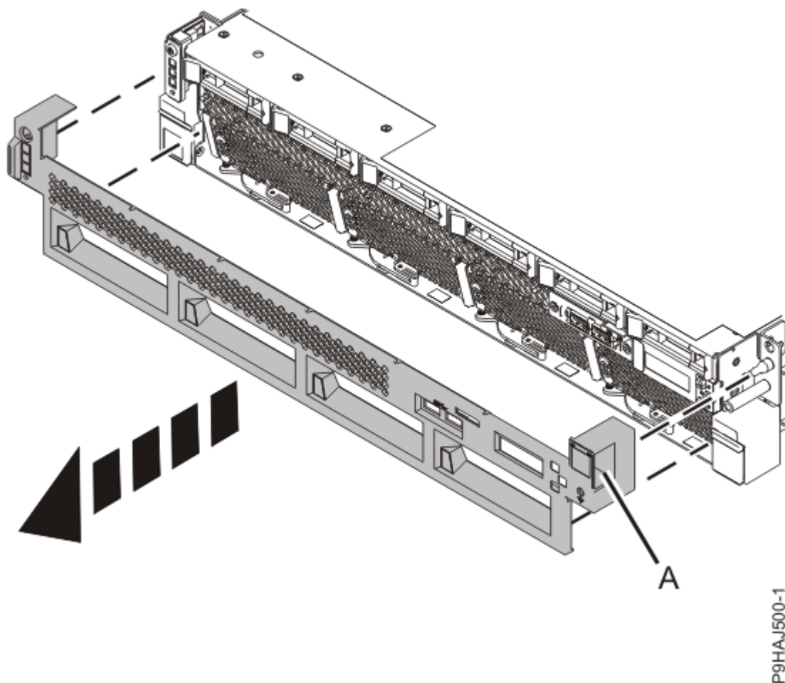
Abbildung 49. Vordere Abdeckungen ausbauen
