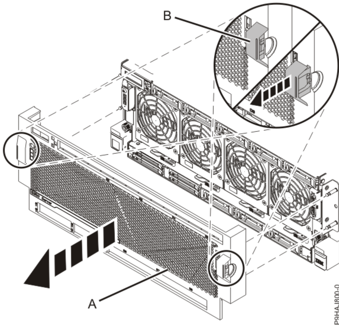
Abbildung 1. Vordere Abdeckung ausbauen
