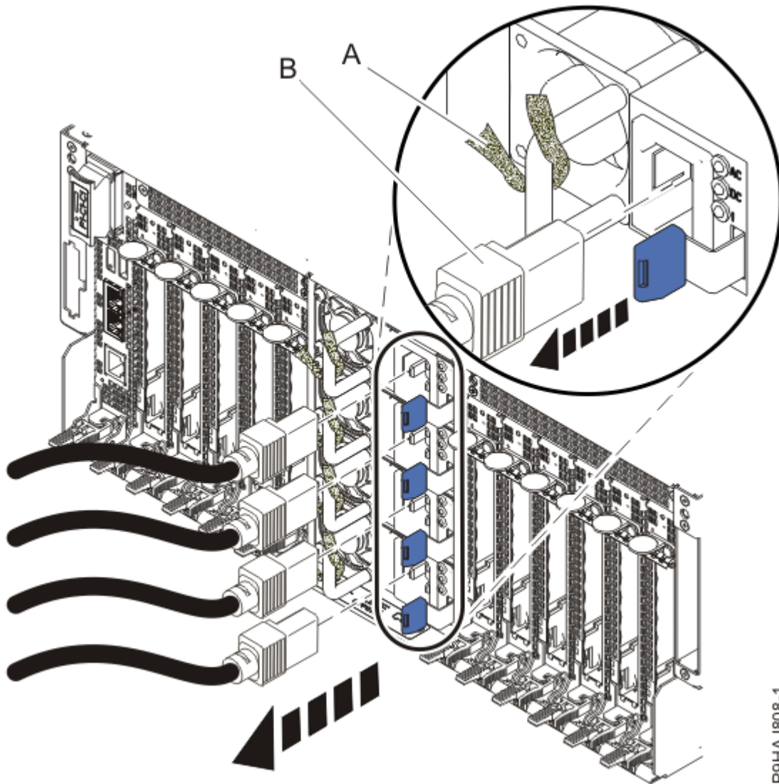
Abbildung 3. Netzkabel abziehen
