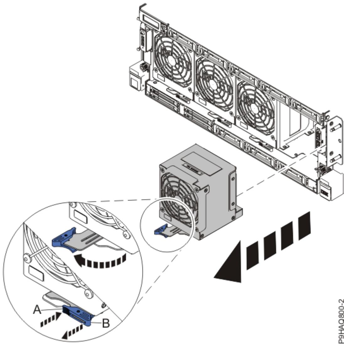
Abbildung 4. Lüfter aus dem System ausbauen
