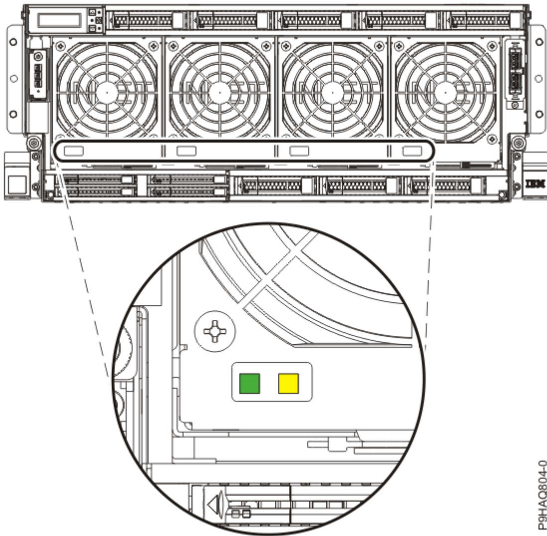
Abbildung 2. Lüfter-LEDs im System
