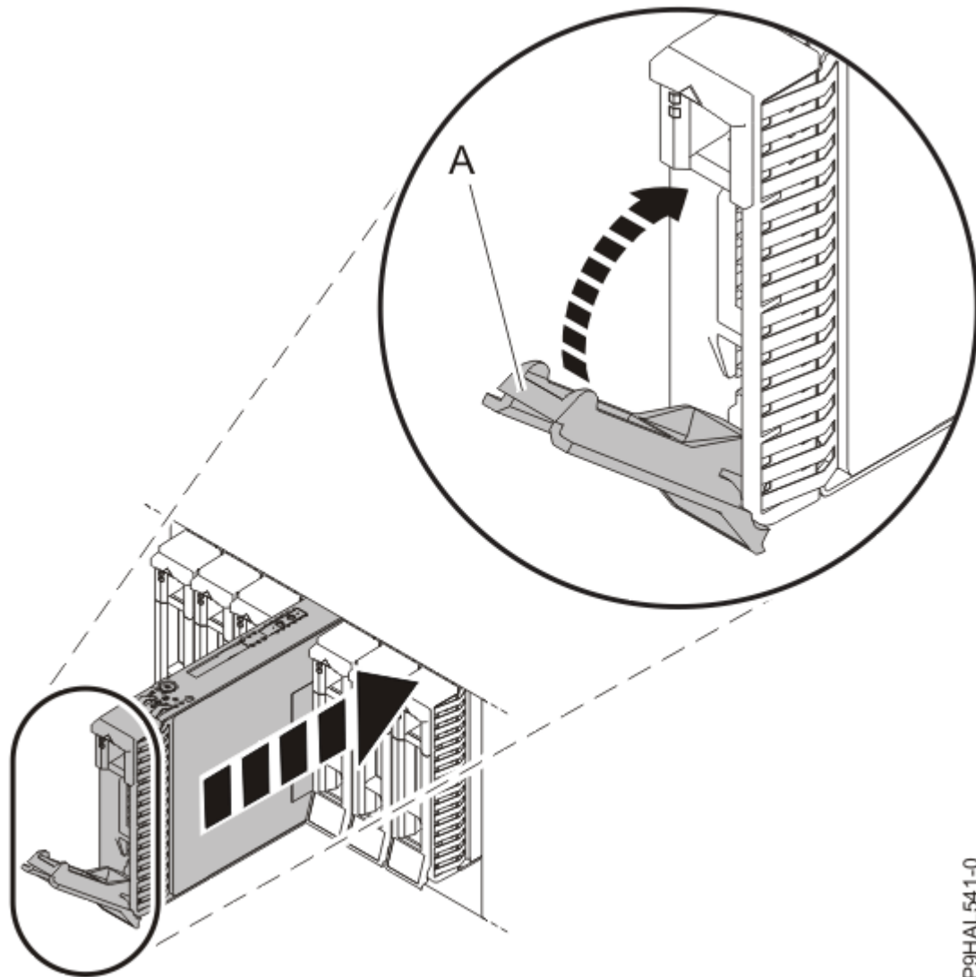
Abbildung 20. Laufwerk in einem System installieren
