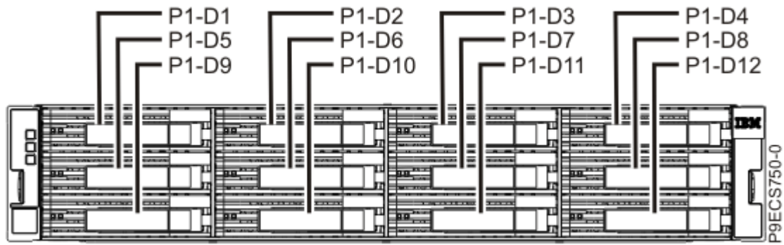
Abbildung 1. Vorderansicht der ESLL-Speichereinheit mit den Positionen der Laufwerke
