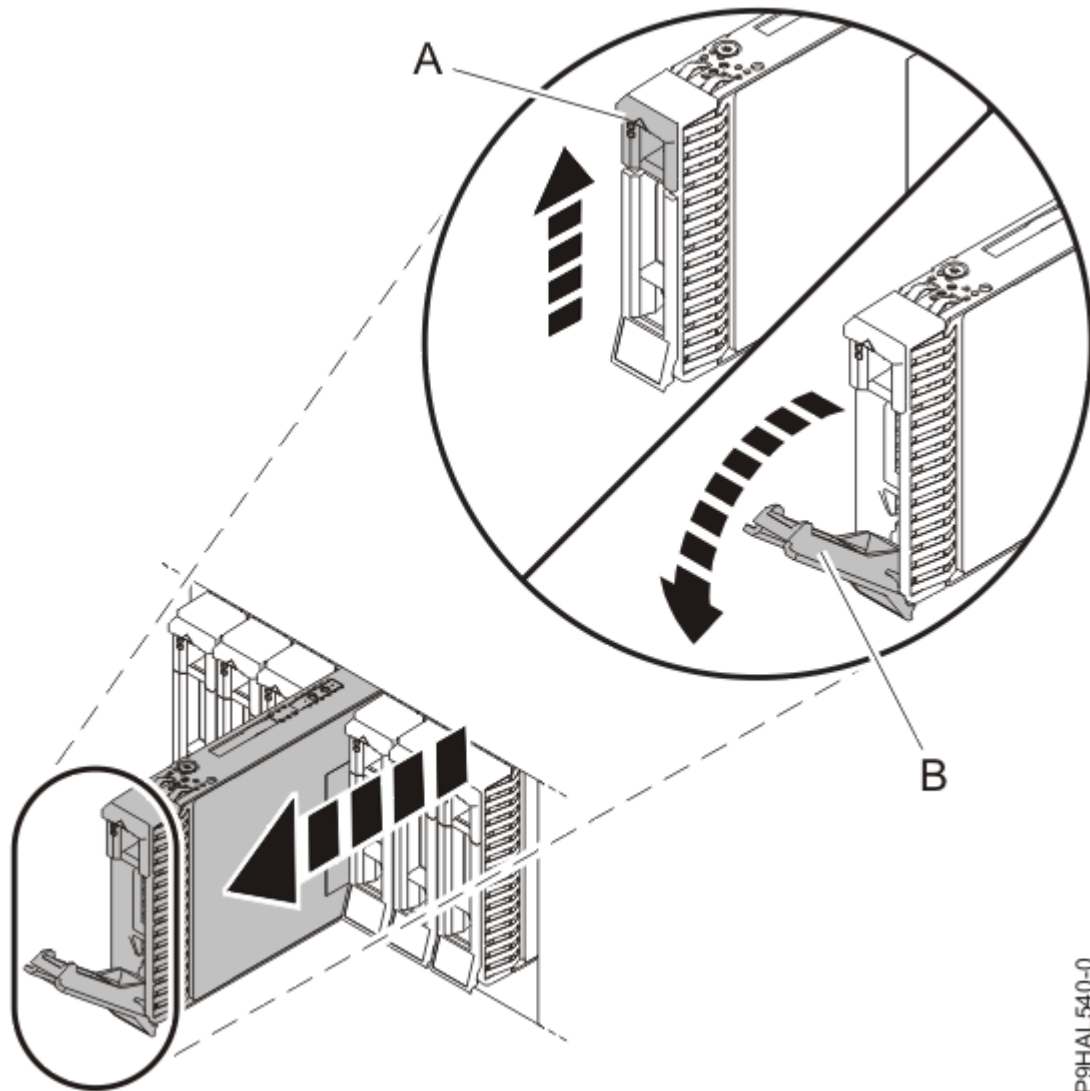
Abbildung 17. Laufwerk entriegeln und ausbauen
