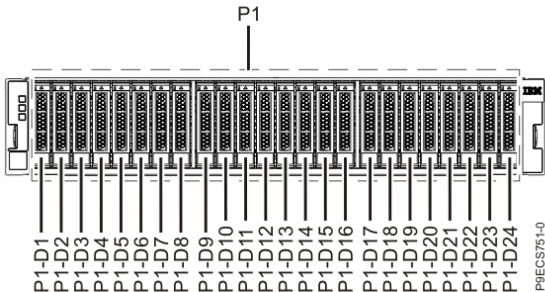
Abbildung 10. Vorderansicht der ESLS-Speichereinheit mit den Positionen der Laufwerke
