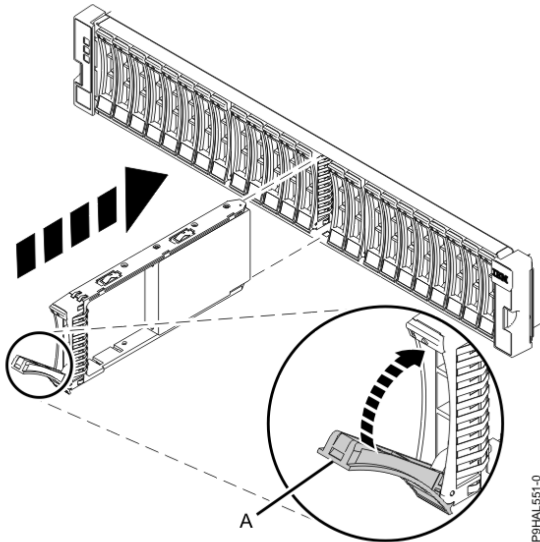
Abbildung 6. Laufwerk in einem Gehäuse installieren oder wiedereinbauen
