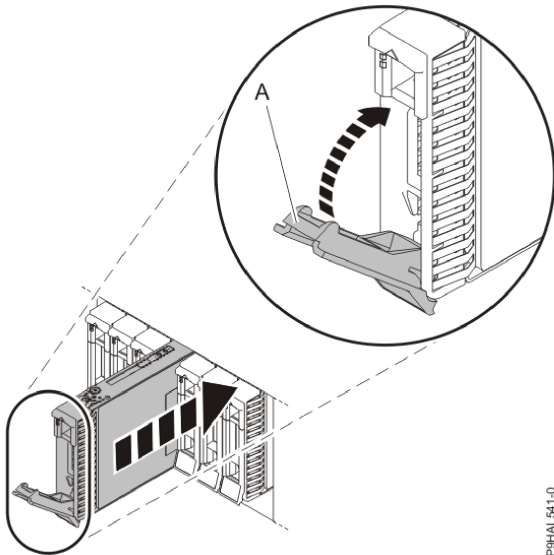
Abbildung 18. Laufwerk in einem Gehäuse wiedereinbauen
