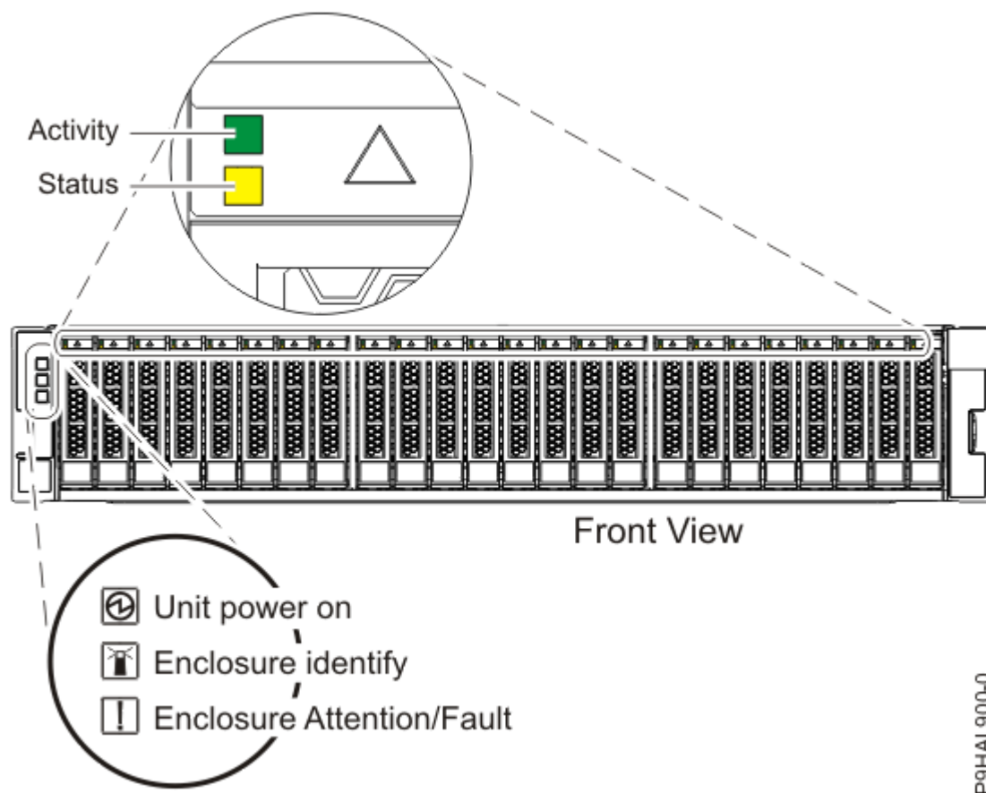
Abbildung 12. Vorderansicht der Speichereinheit mit den Serviceindikatoren
