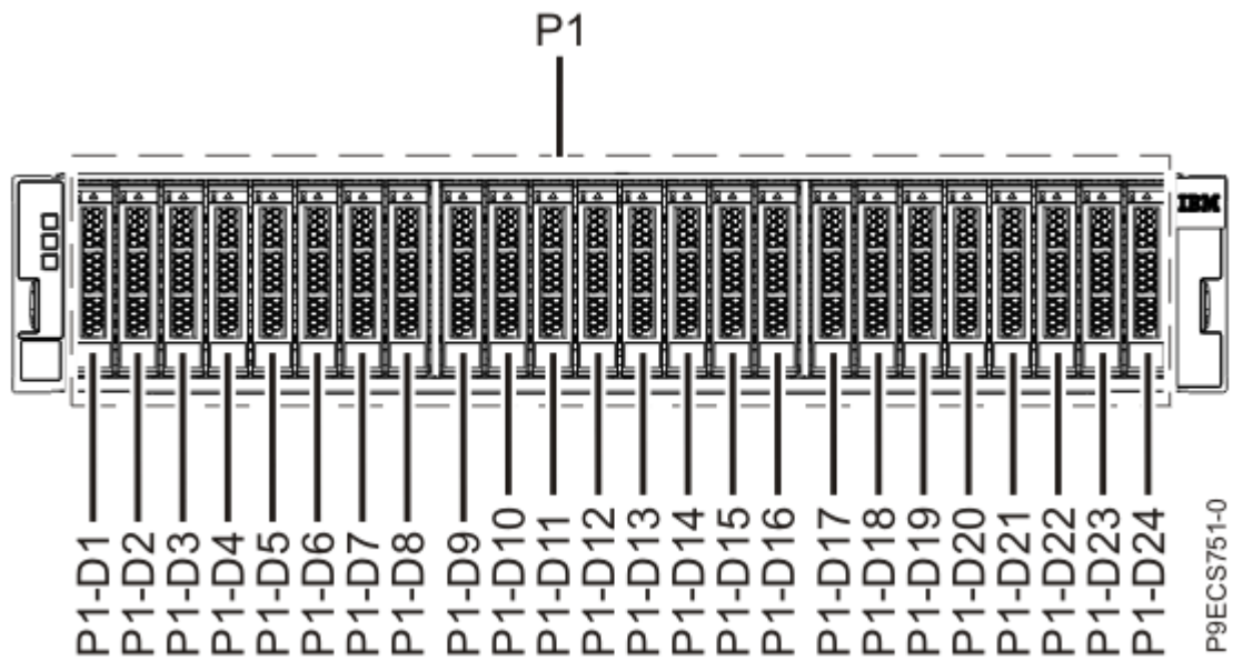
Abbildung 2. Vorderansicht der ESLS-Speichereinheit mit den Positionen der Laufwerke
