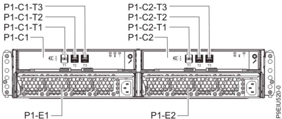
Abbildung 3. Rückansicht der Speichereinheiten
