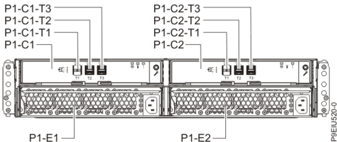
Abbildung 11. Rückansicht der Speichereinheiten
