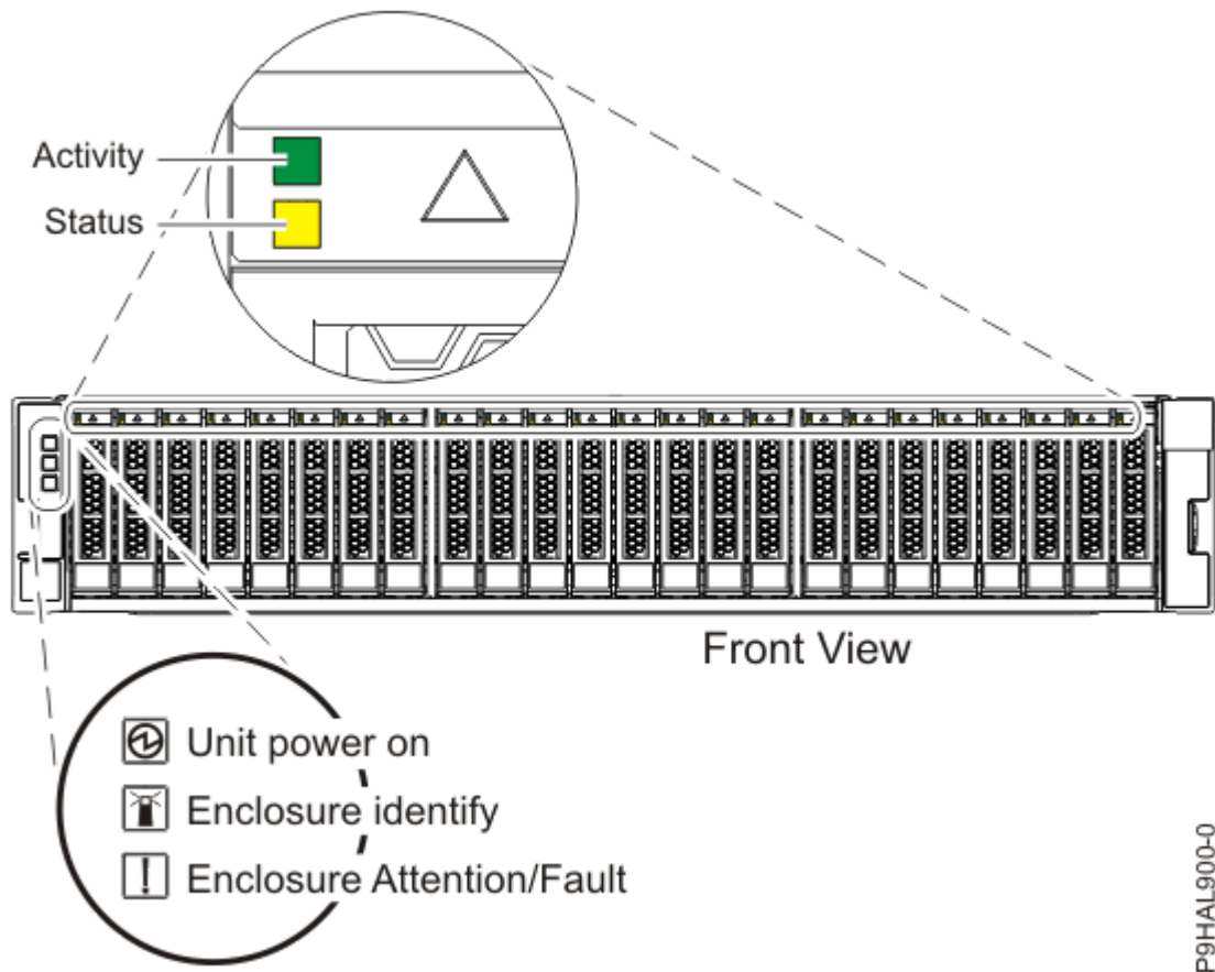
Abbildung 4. Vorderansicht der Speichereinheit mit den Serviceindikatoren
