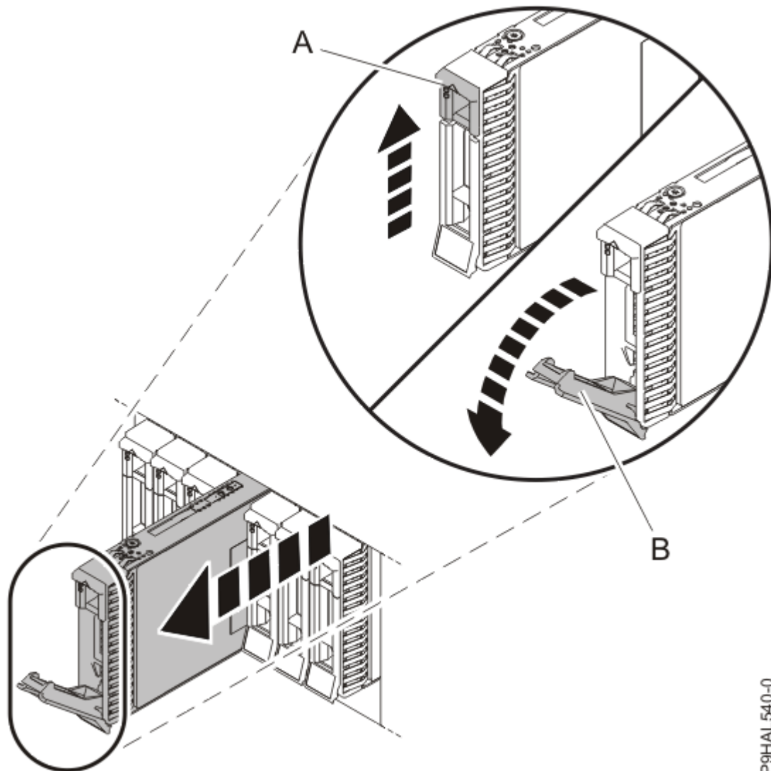
Abbildung 16. Laufwerk entriegeln und ausbauen
