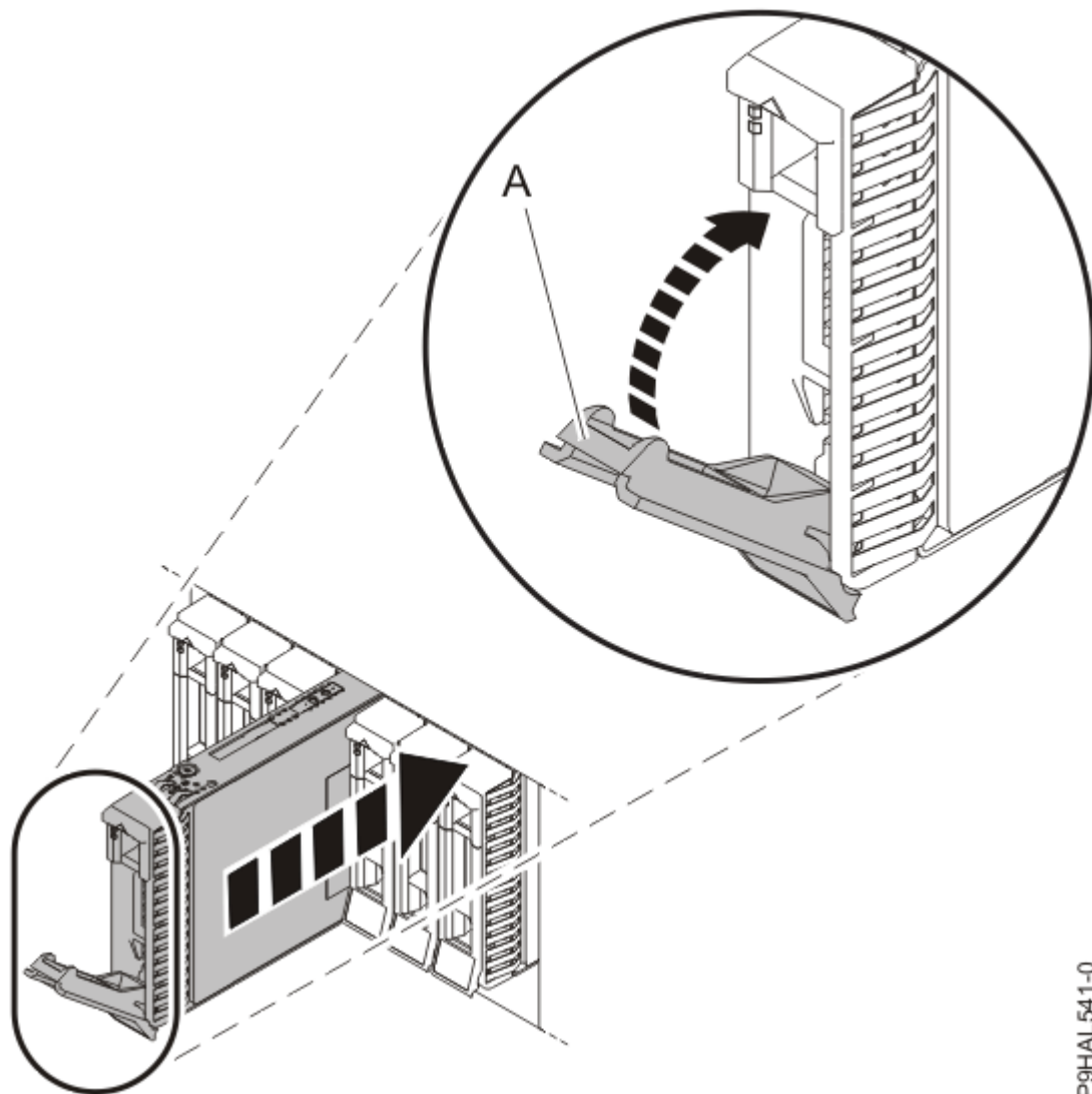
Abbildung 8. Laufwerk in einem System installieren
