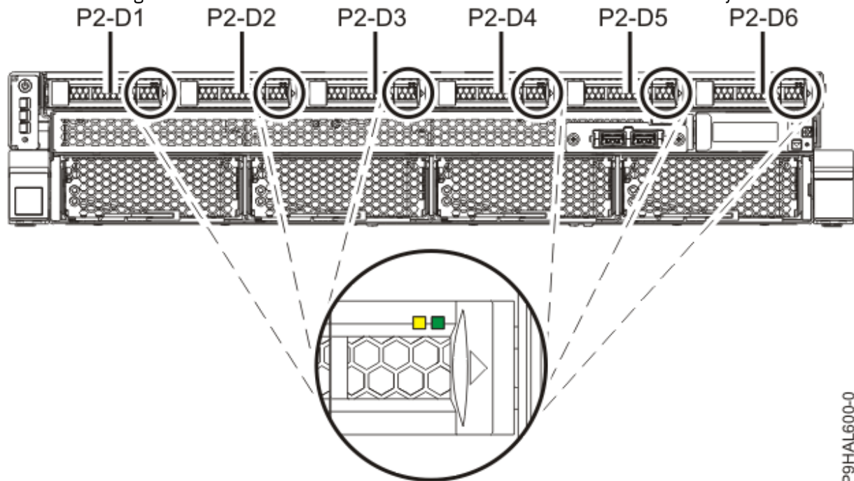
Abbildung 1. Positionen der vorderen Plattenlaufwerke und Serviceindikatoren bei einem System vom Typ 9008-22L, 9009-22A oder 9223-22H
