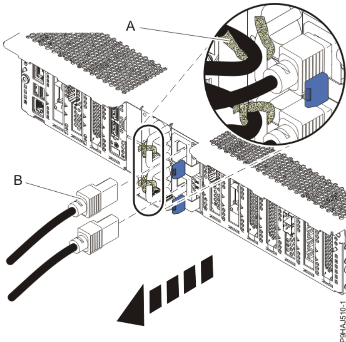
Abbildung 3. Netzkabel abziehen
