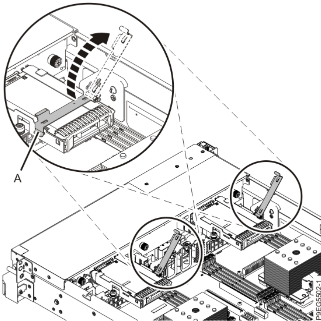
Abbildung 62. Laufwerkhalterhebel öffnen
