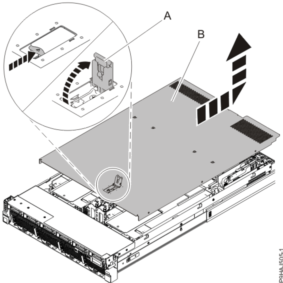
Abbildung 83. Serviceabdeckung ausbauen
