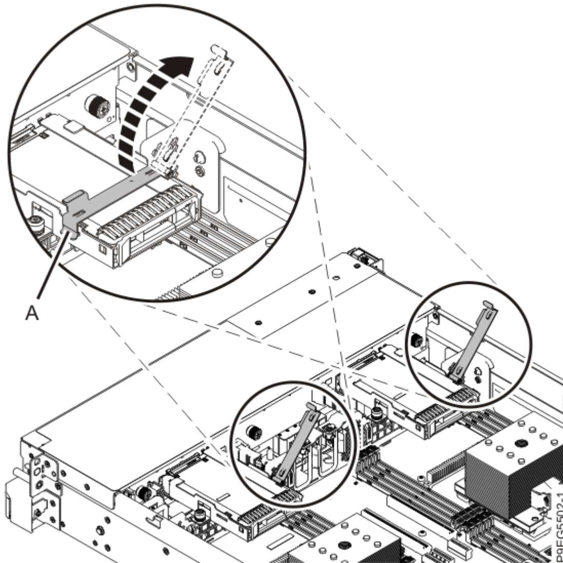
Abbildung 85. Laufwerkhalterhebel öffnen
