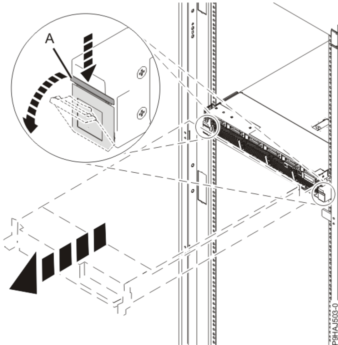
Abbildung 40. Seitliche Verriegelungen entriegeln
