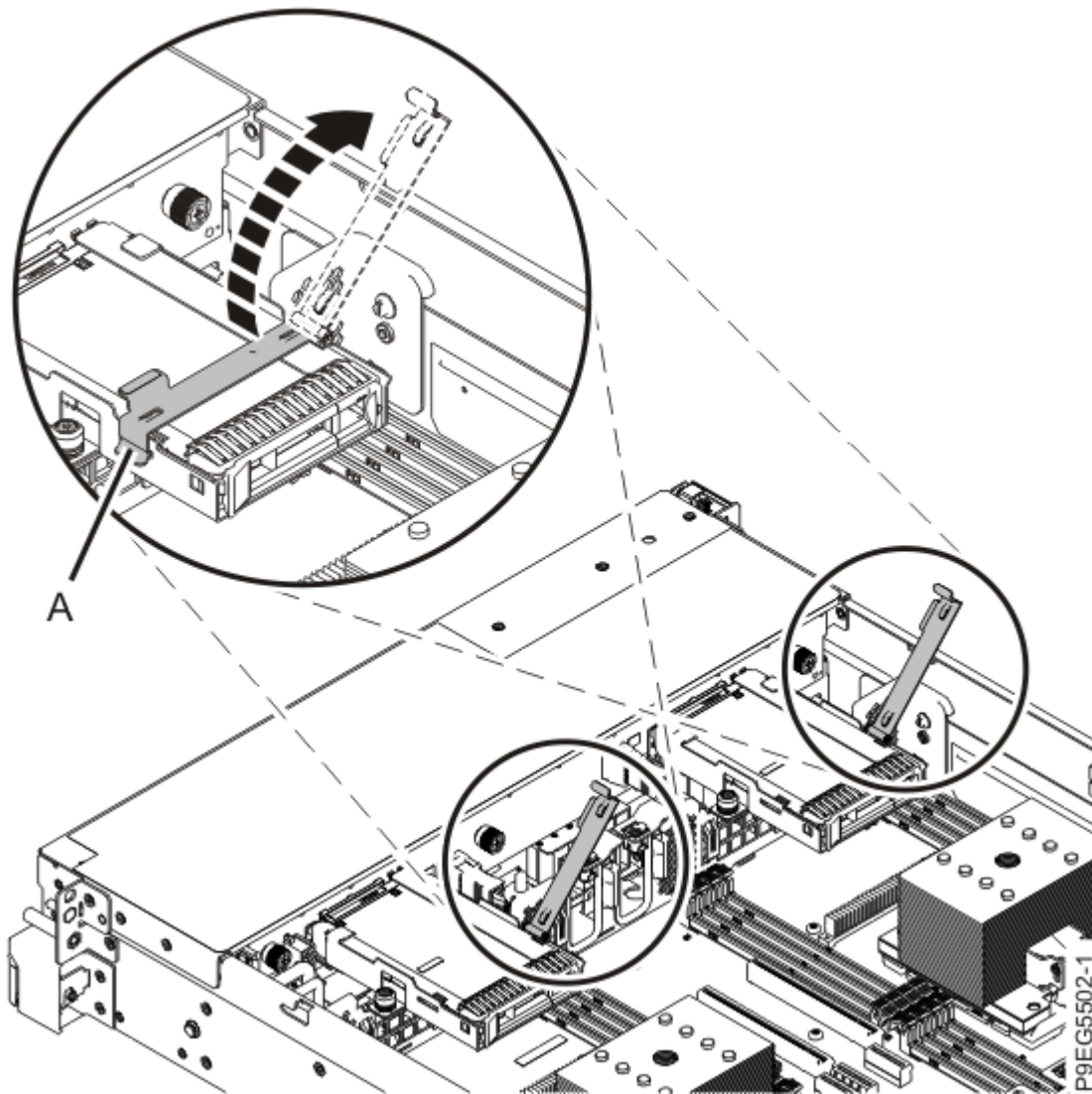
Abbildung 49. Laufwerkhalterhebel öffnen
