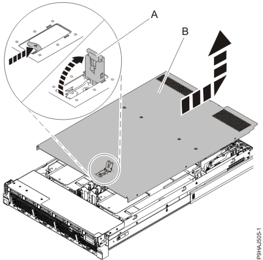
Abbildung 7. Serviceabdeckung ausbauen
