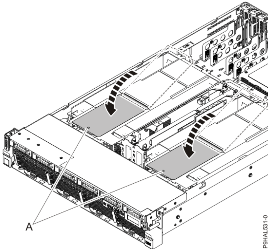
Abbildung 75. Klappbare Zugangstüren der Luftführungen im System vom Typ 9008-22L, 9009-22A oder 9223-22H schließen
