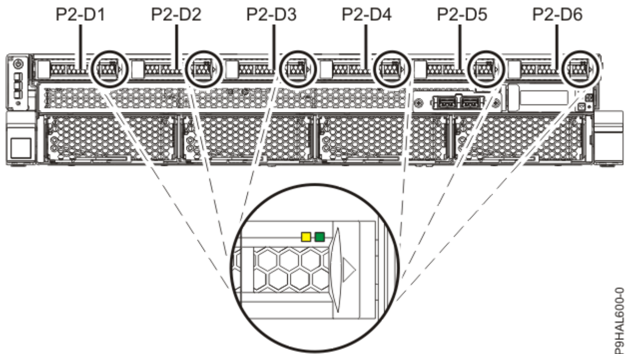
Abbildung 79. Positionen der vorderen Plattenlaufwerke und Serviceindikatoren bei einem System vom Typ 9008-22L, 9009-22A oder 9223-22H
