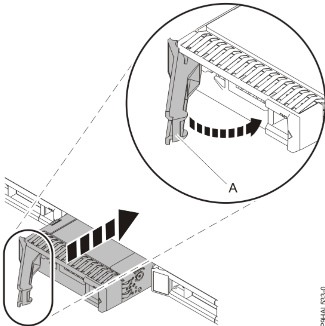
Abbildung 31. Laufwerk in einem System installieren
