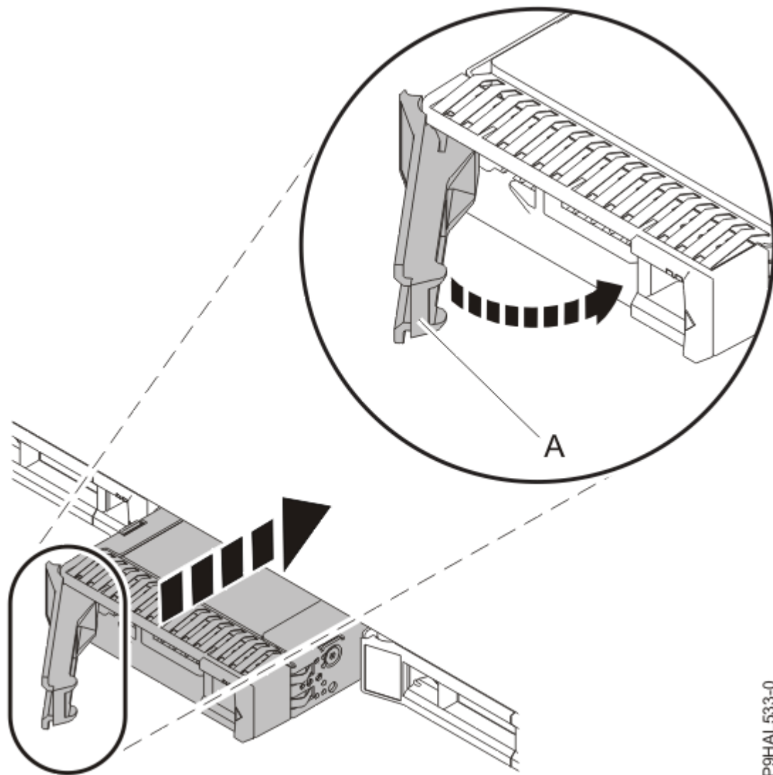
Abbildung 26. Laufwerk in einem System installieren
