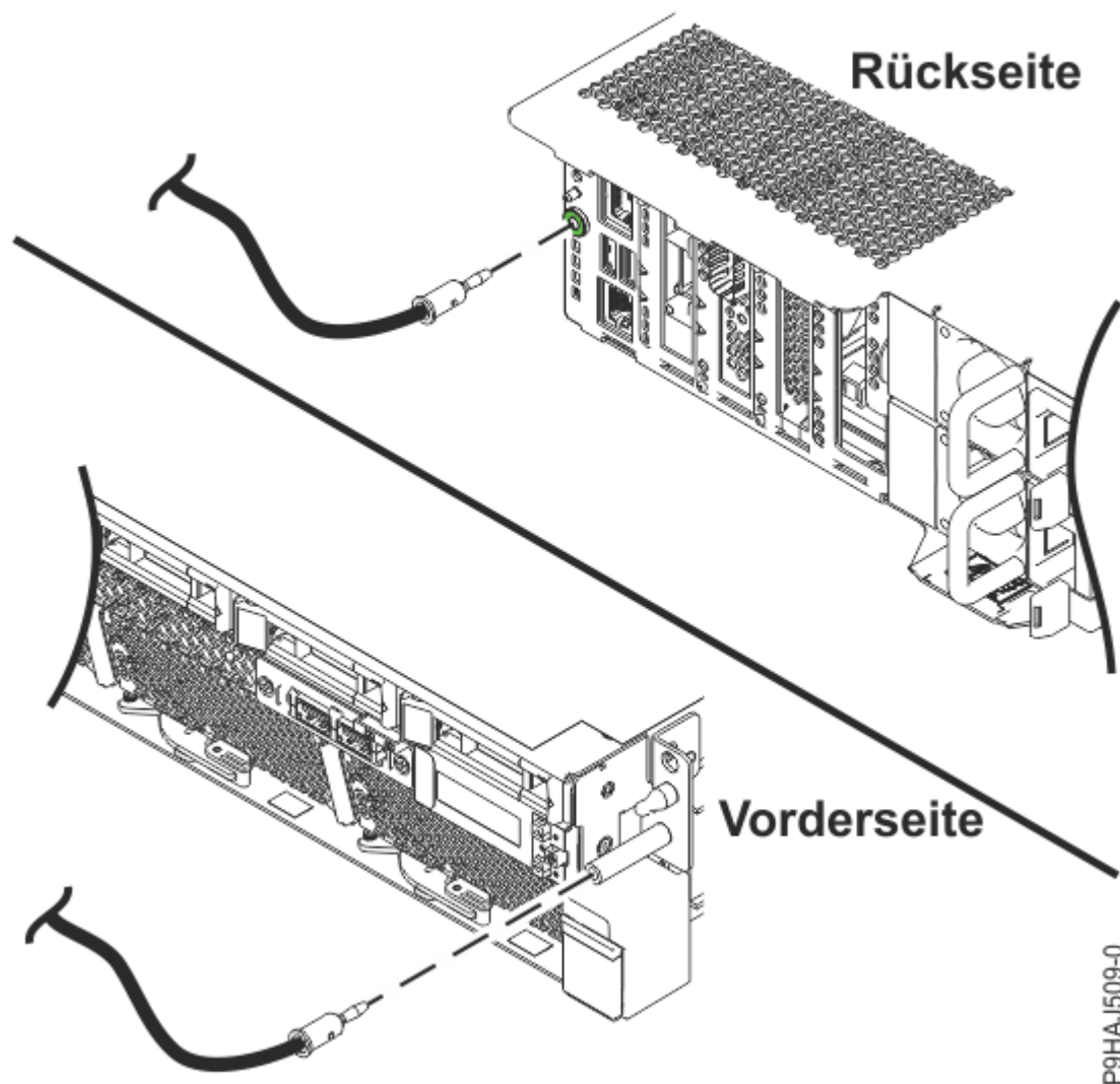
Abbildung 6. Position der ESD-Stecker bei einem System vom Typ 9008-22L, 9009-22A oder 9223-22H
