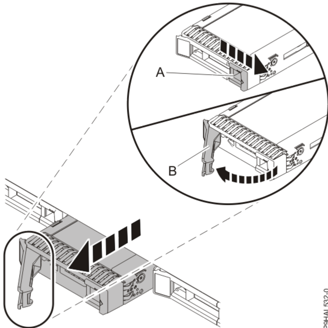
Abbildung 52. Laufwerk entriegeln und ausbauen
