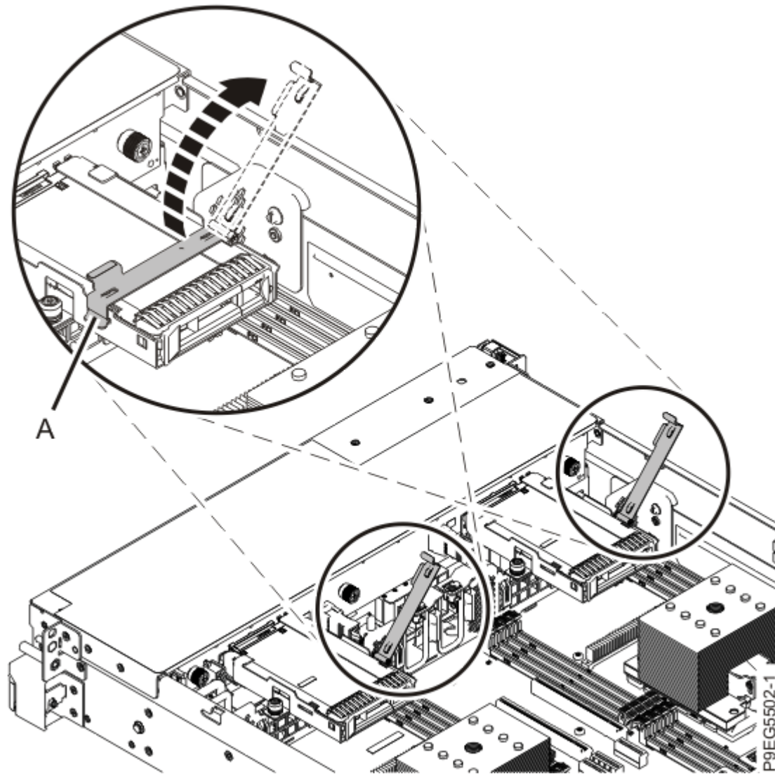
Abbildung 22. Laufwerkhalterhebel öffnen
