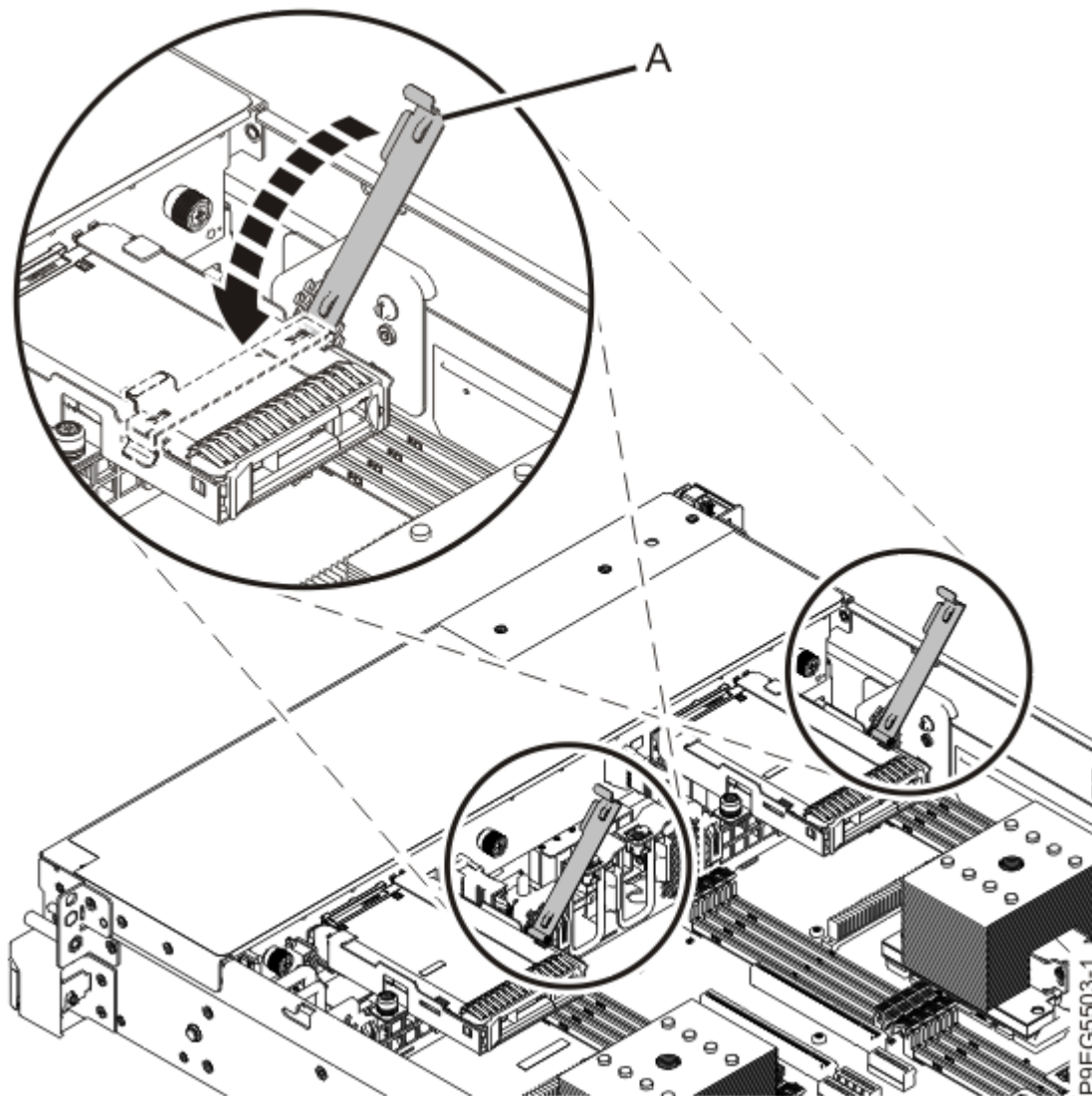
Abbildung 88. Laufwerkhalterhebel schließen
