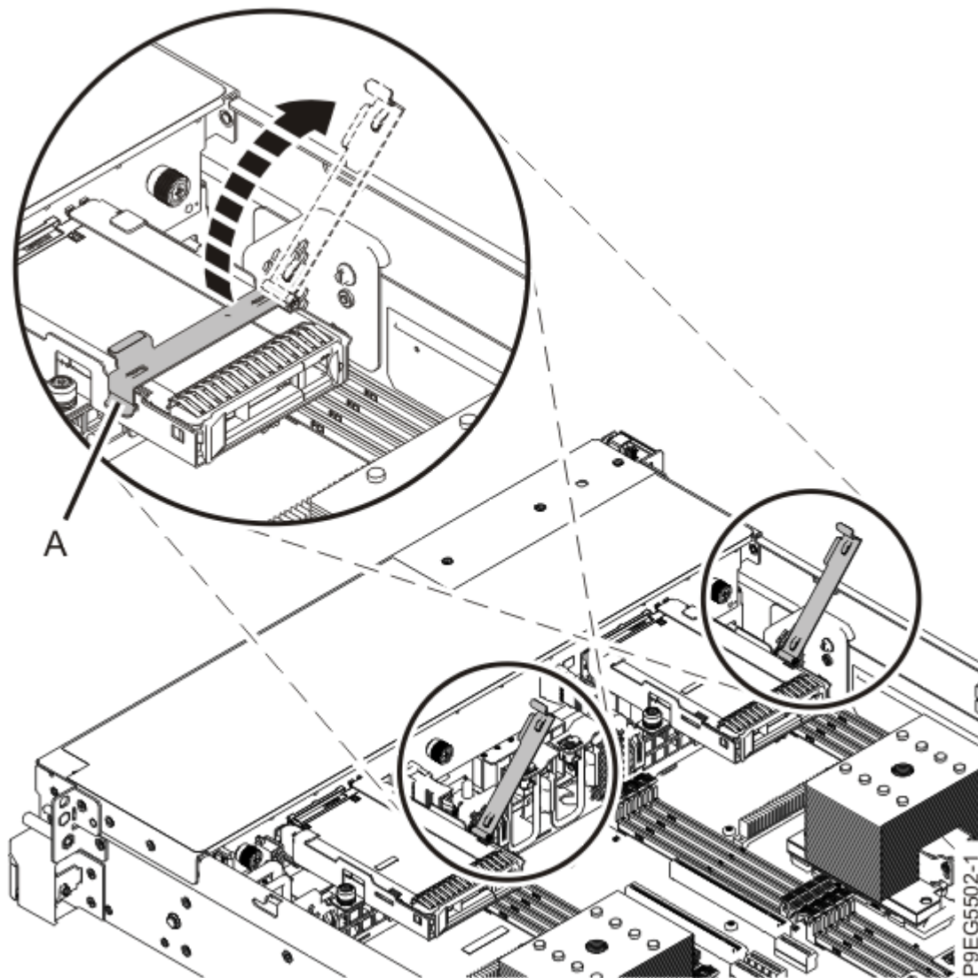
Abbildung 11. Laufwerkhalterhebel öffnen
