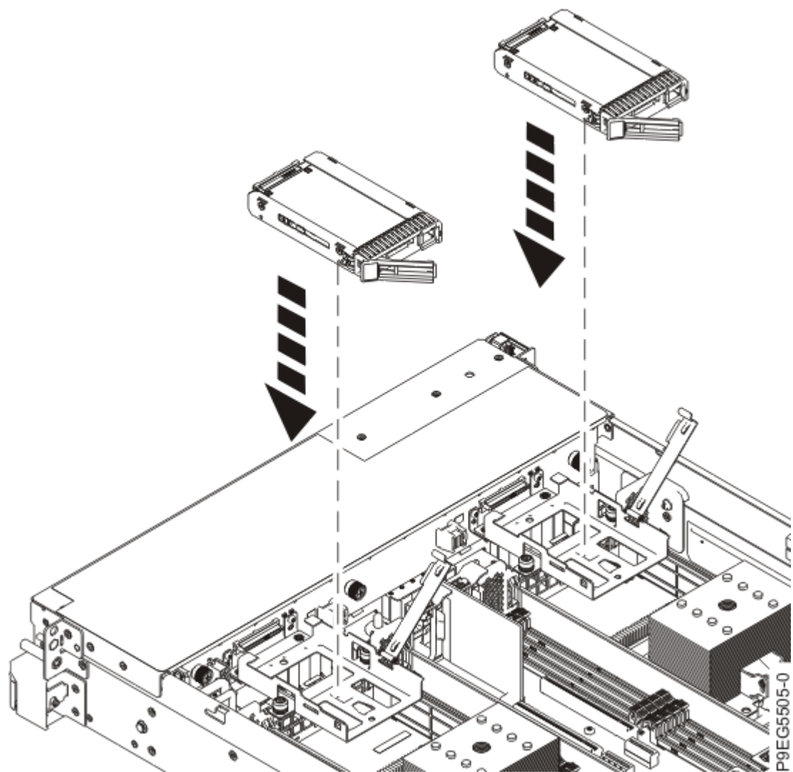
Abbildung 28. Laufwerk in Laufwerkhalterung absenken
