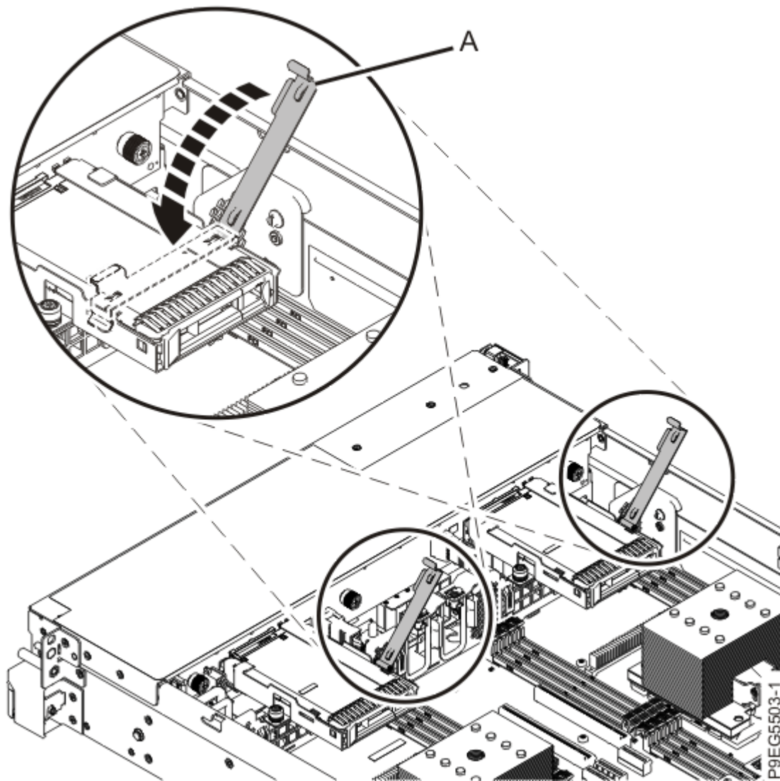
Abbildung 72. Laufwerkhalterhebel schließen
