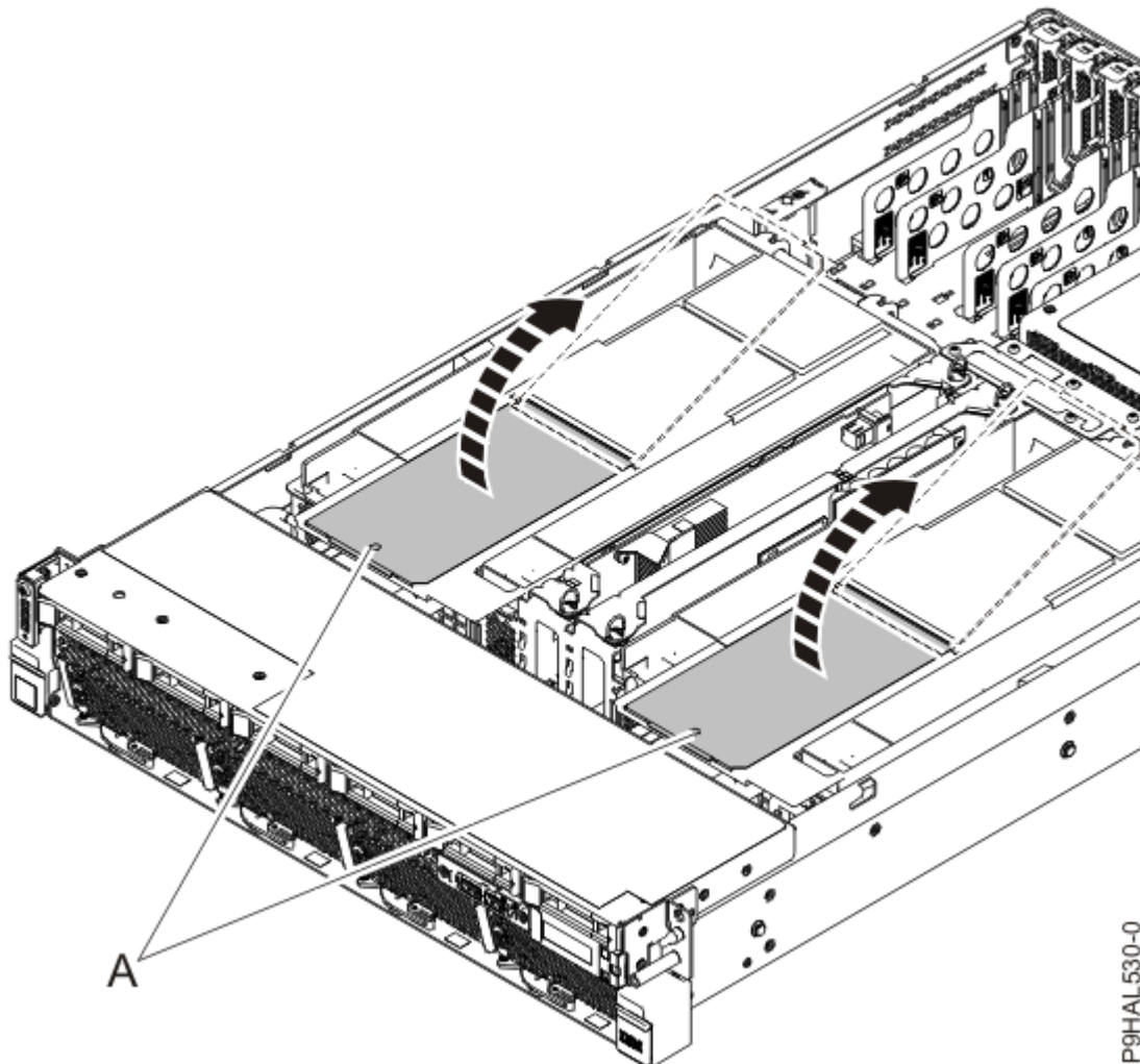
Abbildung 84. Klappbare Zugangstüren der Luftführungen im System vom Typ 9008-22L, 9009-22A oder 9223-22H öffnen
