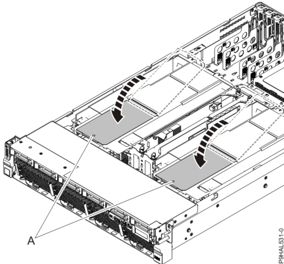
Abbildung 32. Klappbare Zugangstüren der Luftführungen im System vom Typ 9008-22L, 9009-22A oder 9223-22H schließen
