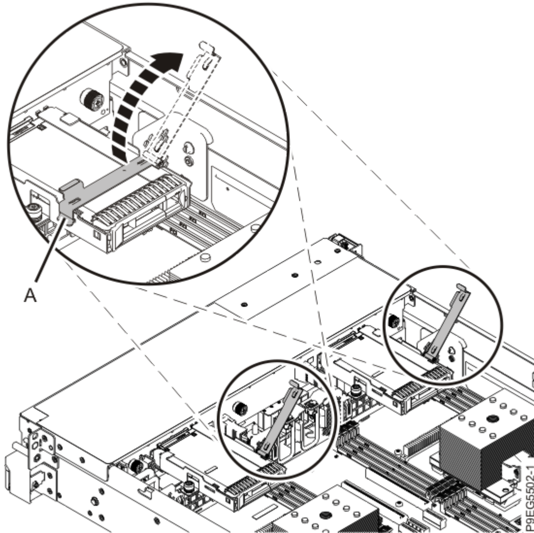
Abbildung 27. Laufwerkhalterhebel öffnen
