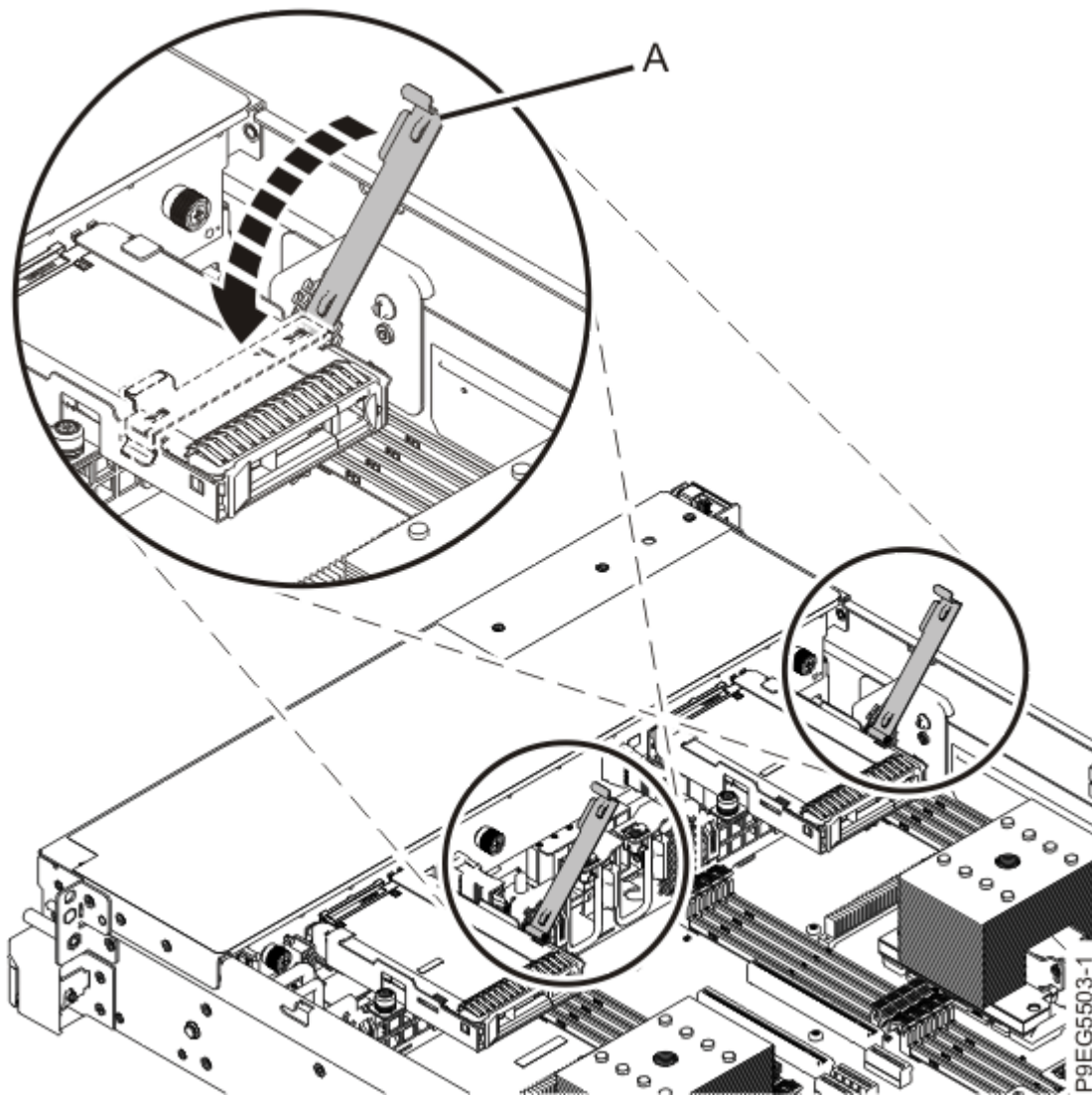
Abbildung 68. Laufwerkhalterhebel schließen
