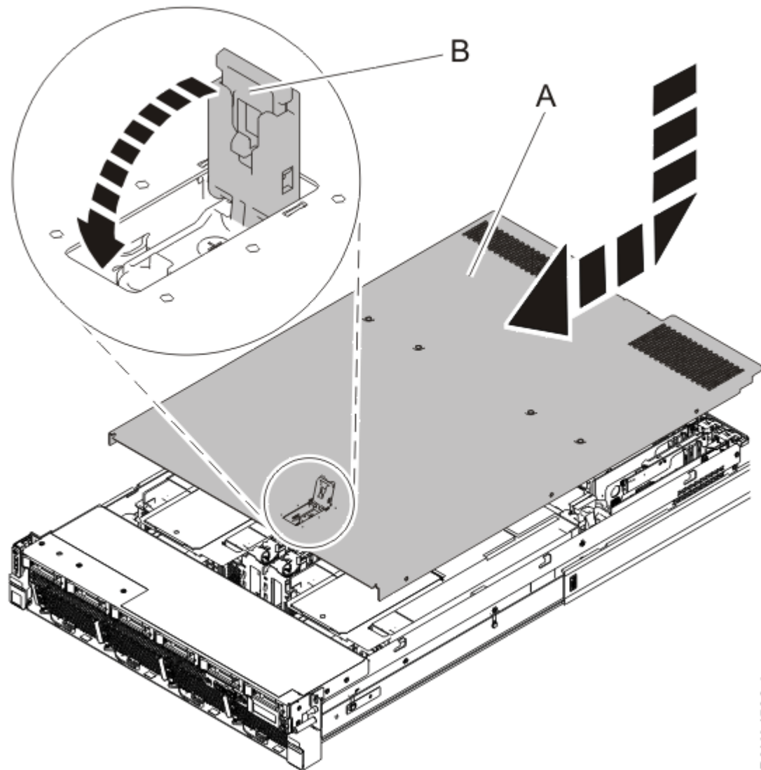
Abbildung 76. Serviceabdeckung installieren
