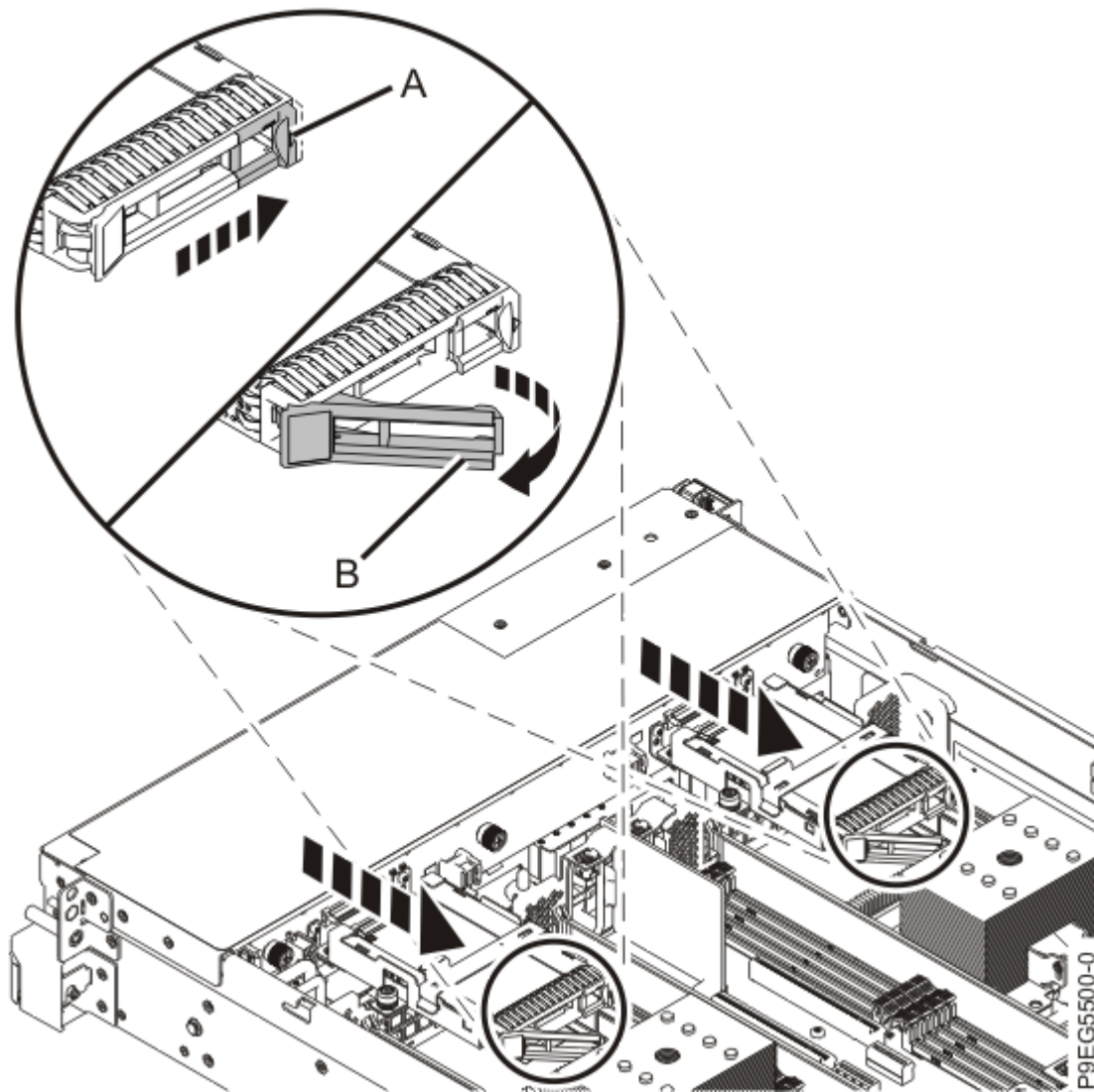
Abbildung 47. Laufwerk entriegeln
