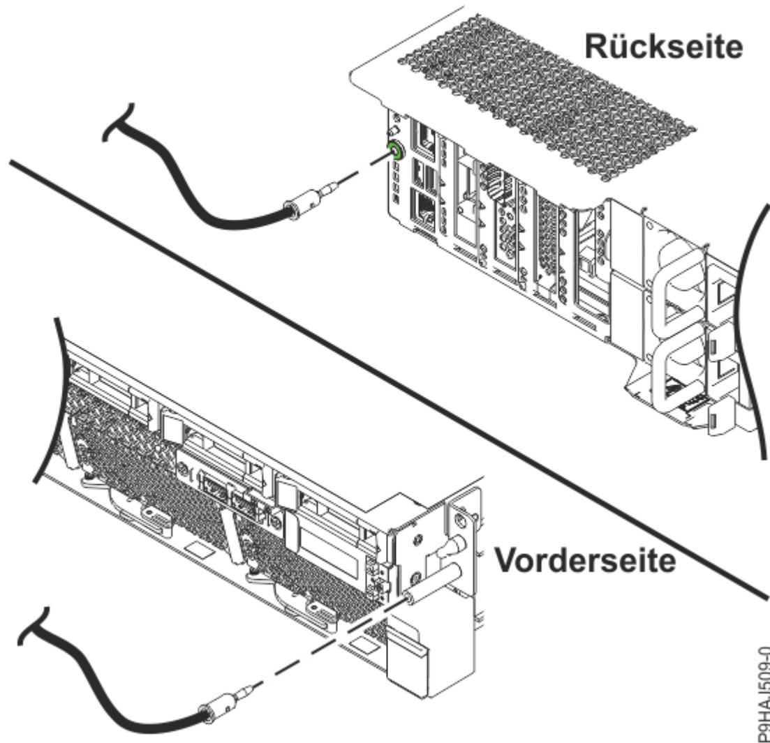
Abbildung 41. Position der ESD-Stecker bei einem System vom Typ 9008-22L, 9009-22A oder 9223-22H
