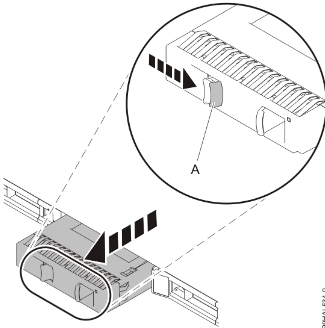
Abbildung 10. Platzhalterelement für Laufwerk ausbauen
