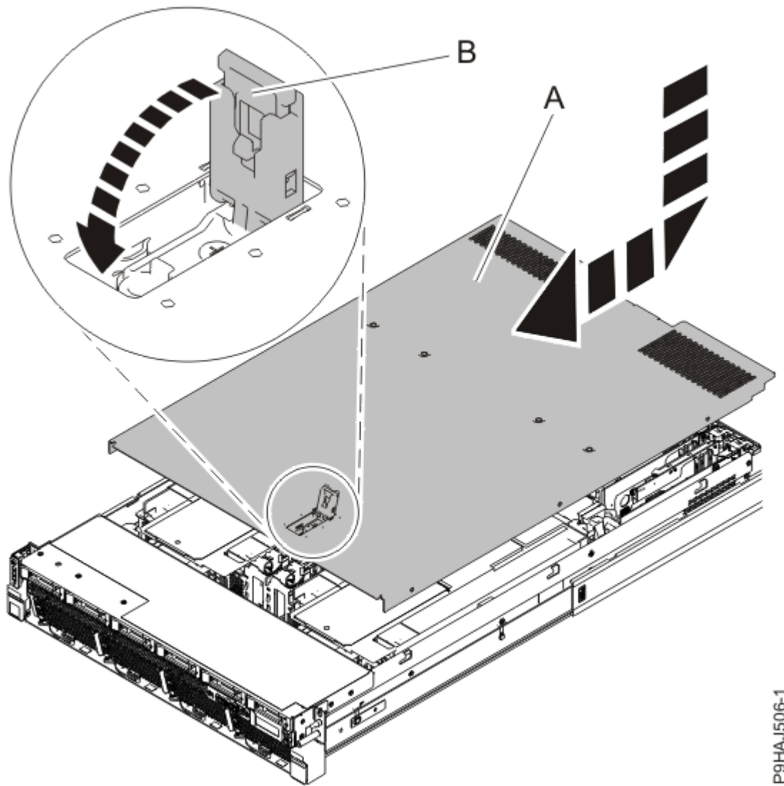
Abbildung 92. Serviceabdeckung installieren
