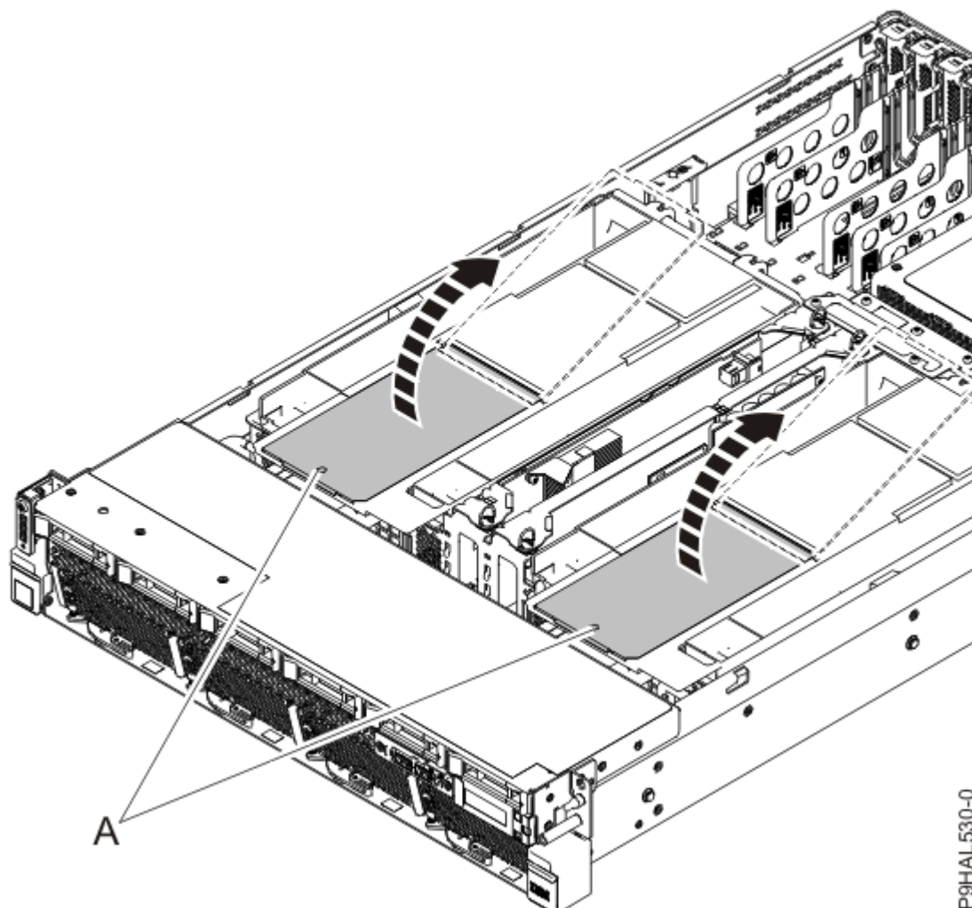
Abbildung 8. Klappbare Zugangstüren der Luftführungen im System vom Typ 9008-22L, 9009-22A oder 9223-22H öffnen
