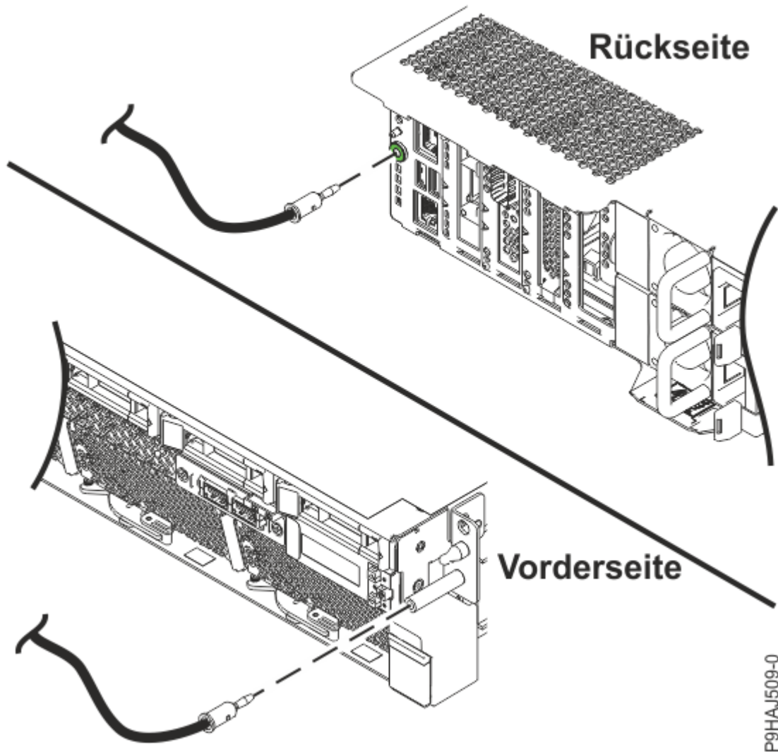
Abbildung 9. Position der ESD-Stecker bei einem System vom Typ 9008-22L, 9009-22A oder 9223-22H
