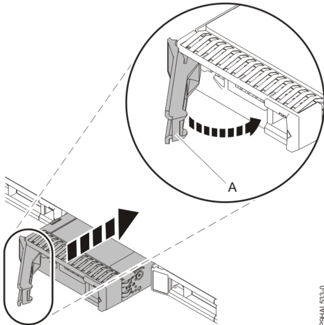
Abbildung 74. Laufwerk in einem System installieren
