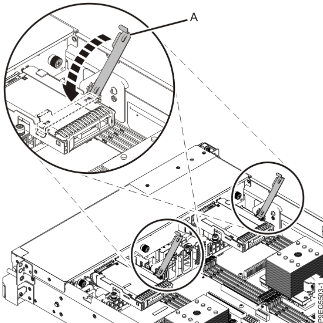
Abbildung 60. Laufwerkhalterhebel schließen
