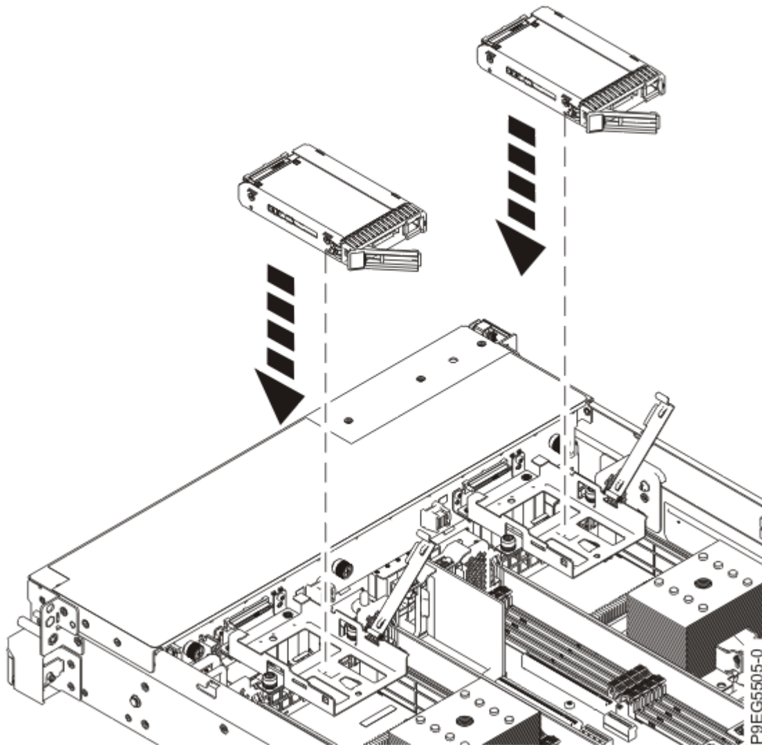
Abbildung 67. Laufwerk in Laufwerkhalterung absenken
