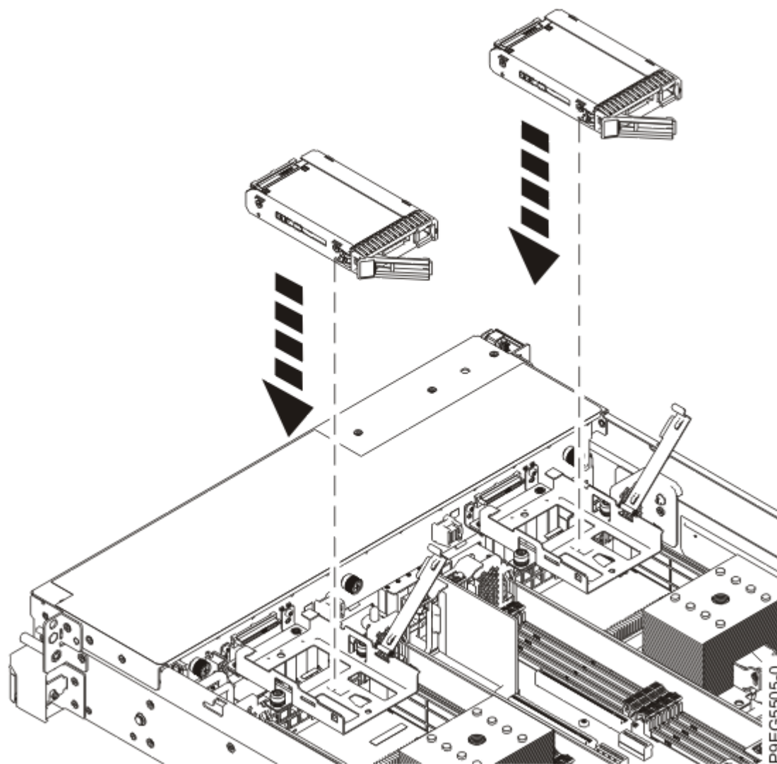
Abbildung 58. Laufwerk in Laufwerkhalterung absenken
