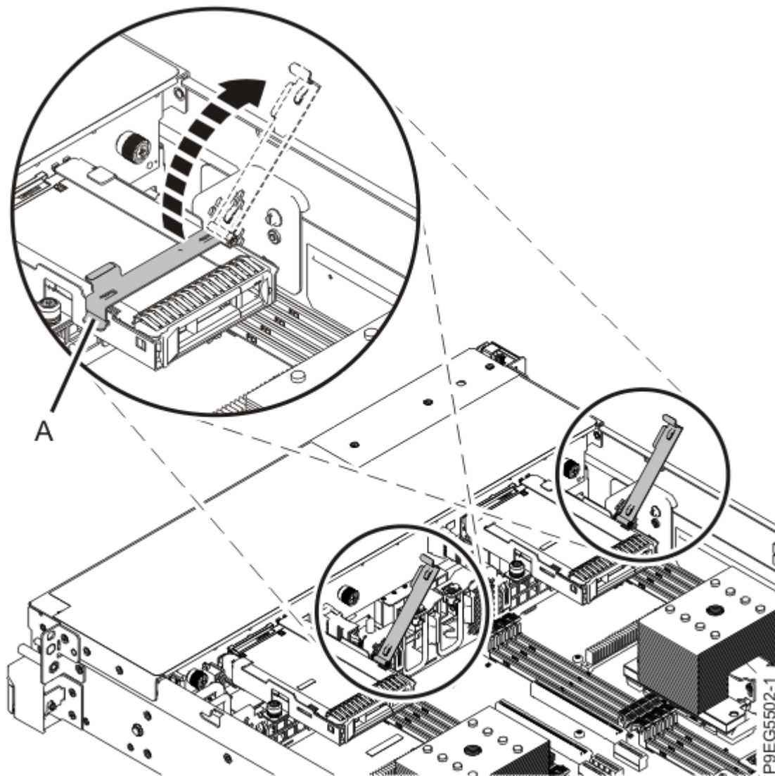
Abbildung 53. Laufwerkhalterhebel öffnen
