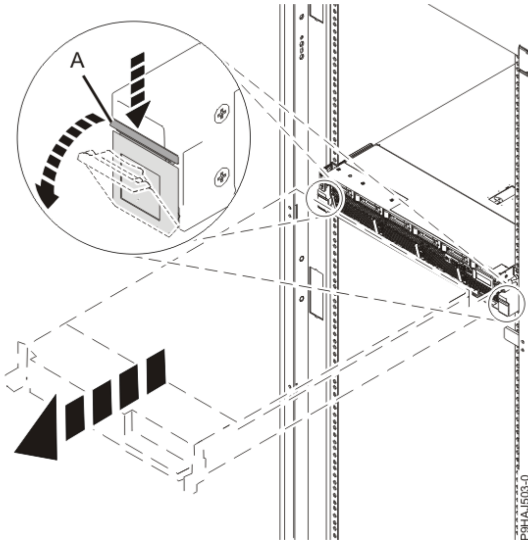
Abbildung 82. Seitliche Verriegelungen entriegeln
