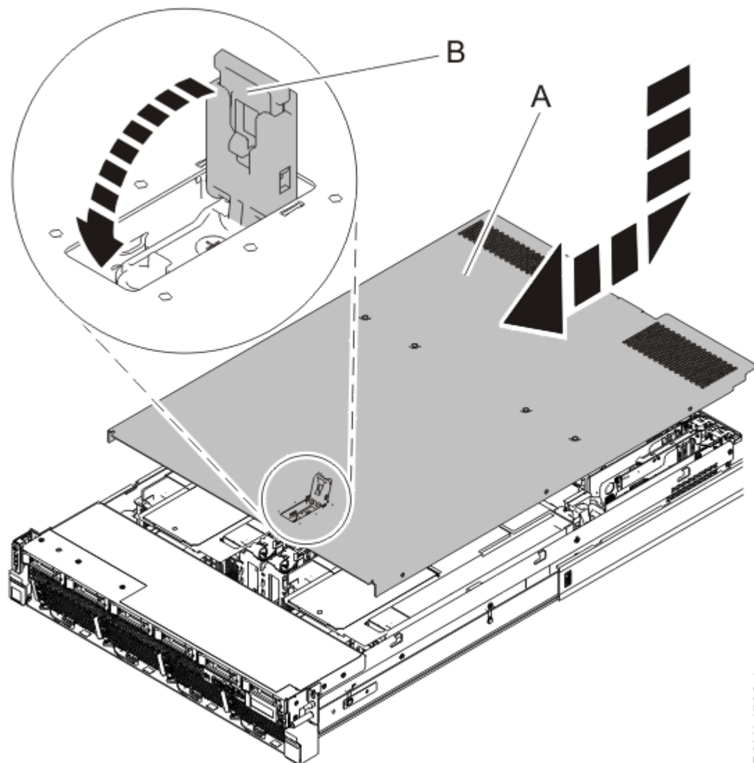
Abbildung 33. Serviceabdeckung installieren
