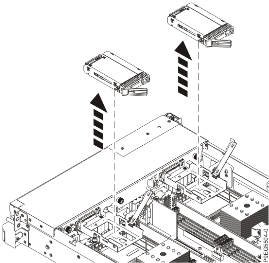
Abbildung 87. Laufwerk anheben
