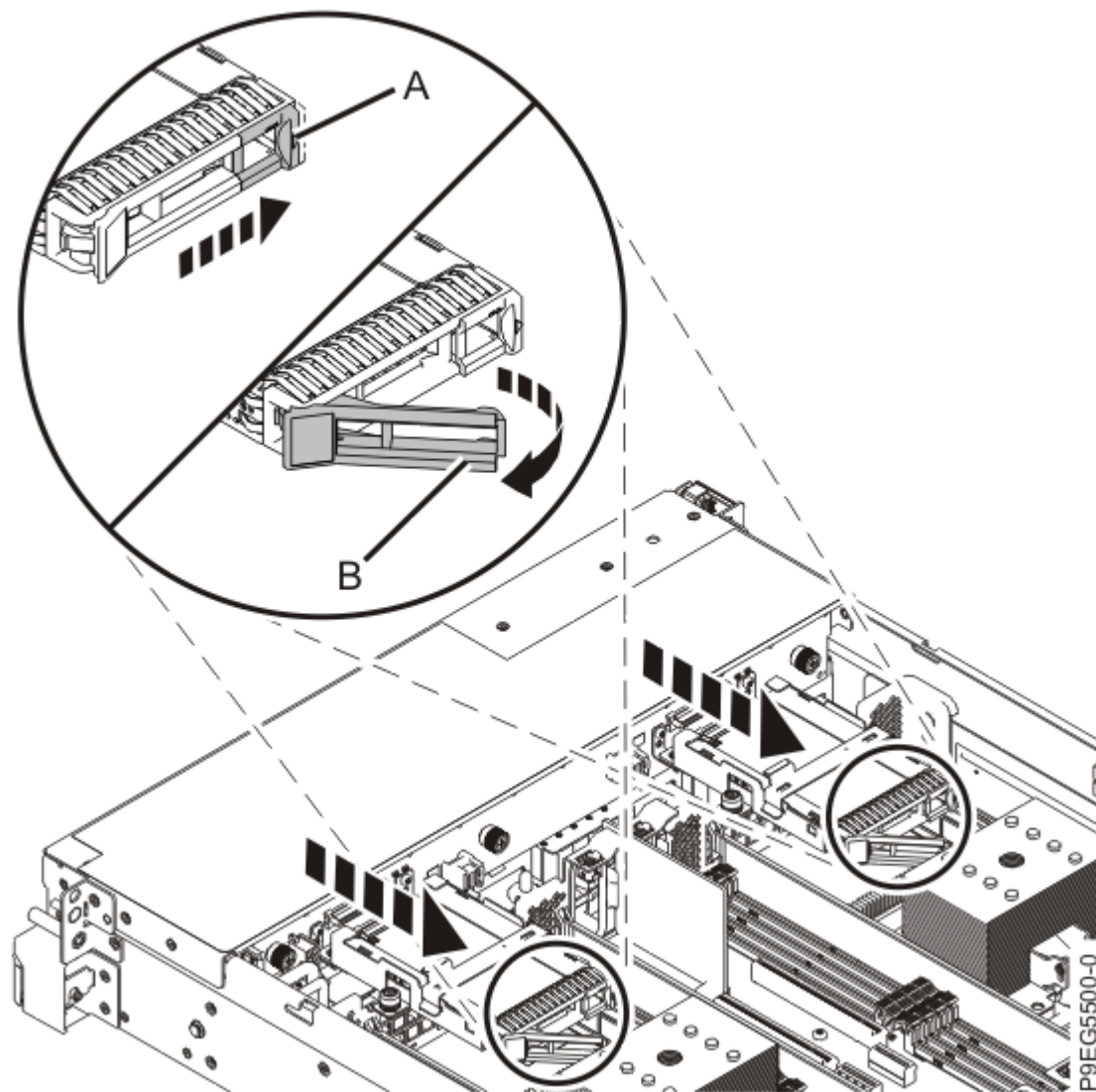
Abbildung 57. Griff für Laufwerkhalterung entriegeln
