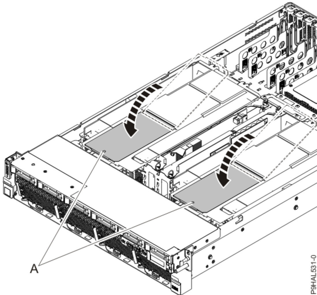
Abbildung 91. Klappbare Zugangstüren der Luftführungen im System vom Typ 9008-22L, 9009-22A oder 9223-22H schließen
