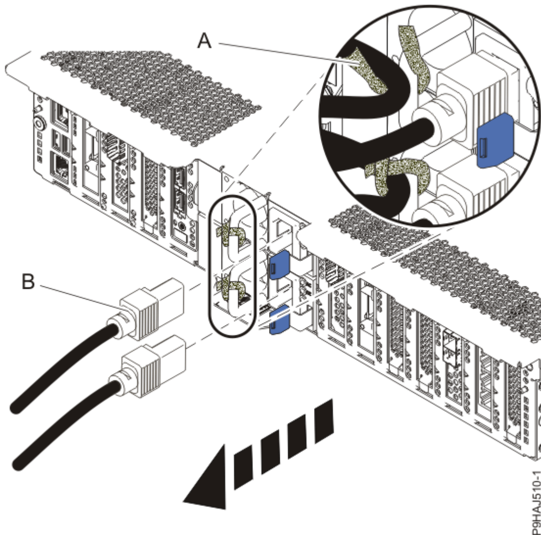
Abbildung 38. Netzkabel abziehen
