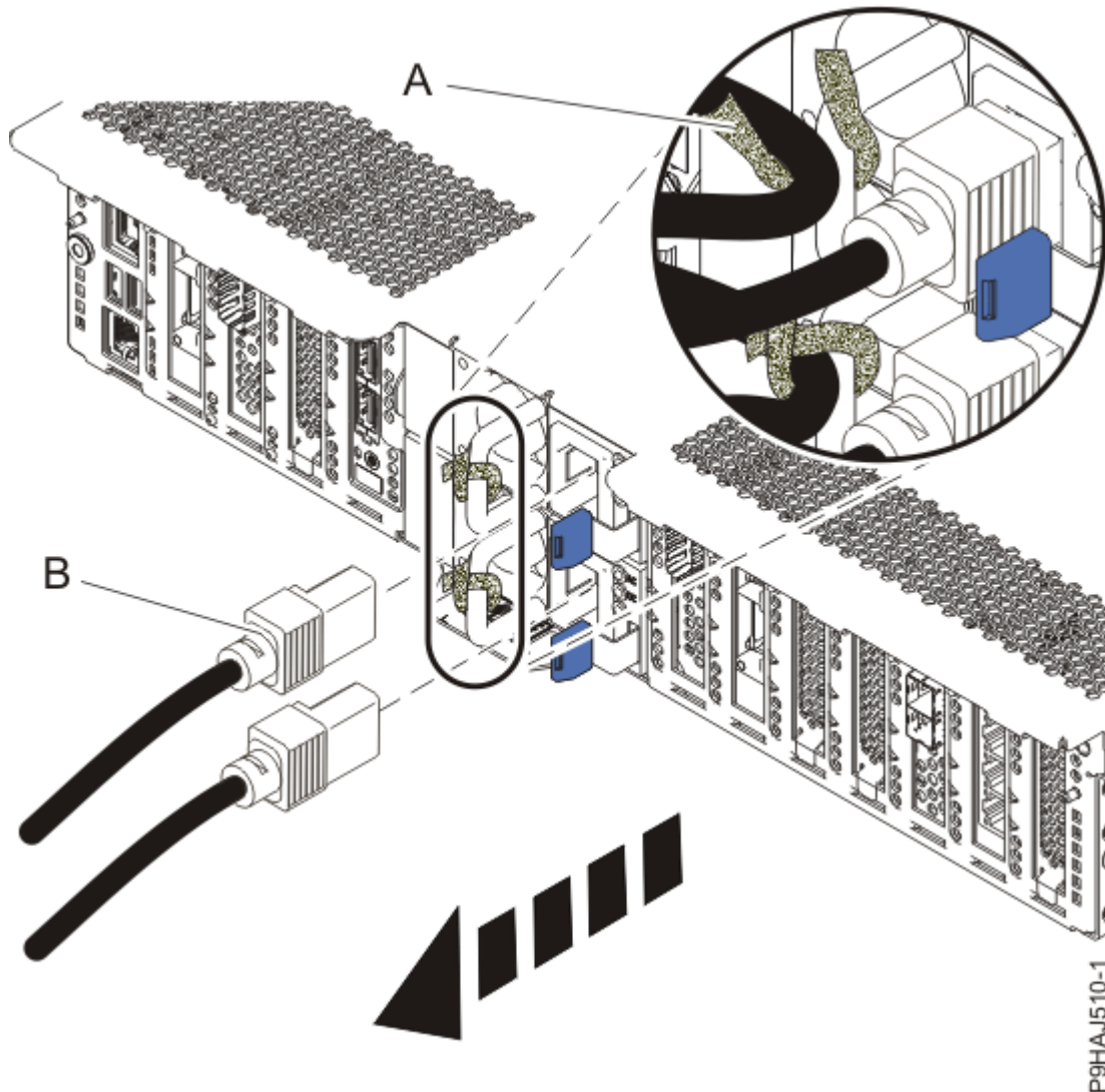
Abbildung 81. Netzkabel abziehen
