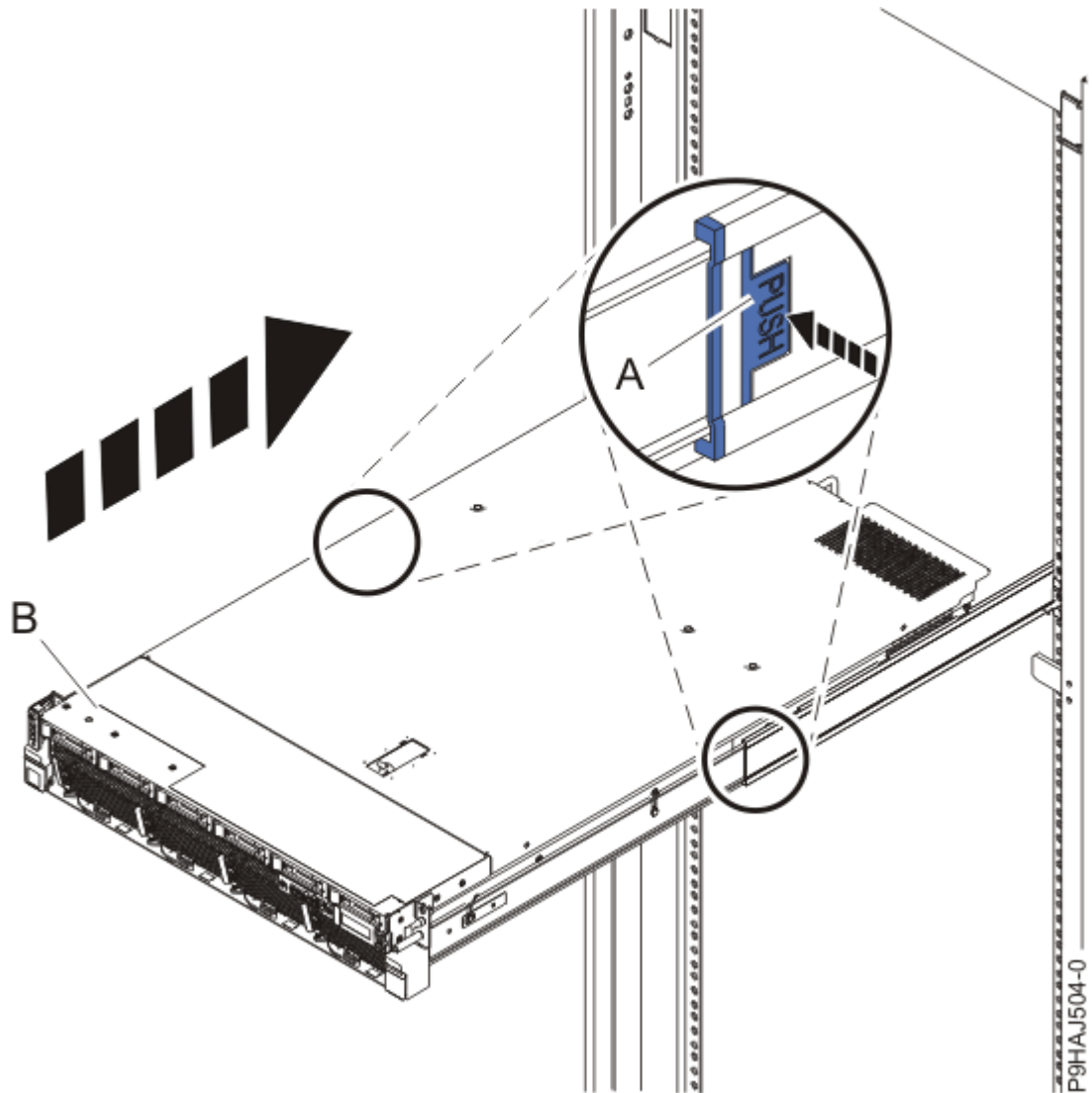
Abbildung 93. System in die Betriebsposition bringen
