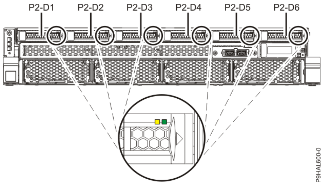
Abbildung 36. Positionen der vorderen Plattenlaufwerke und Serviceindikatoren bei einem System vom Typ 9008-22L, 9009-22A oder 9223-22H
