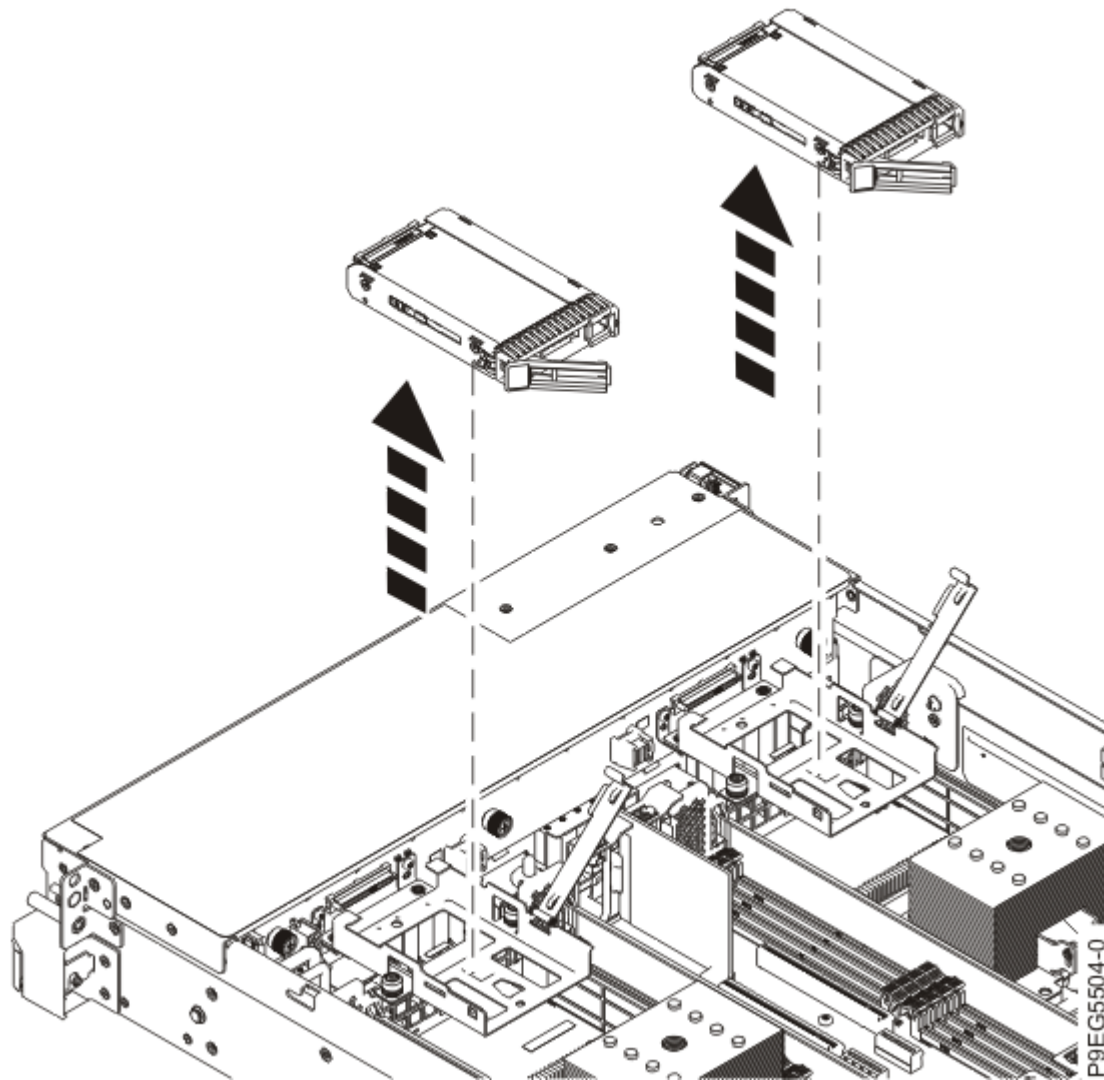
Abbildung 55. Laufwerk anheben
