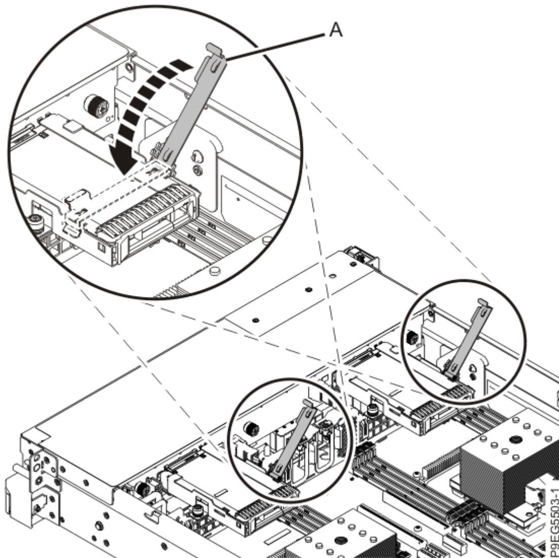
Abbildung 19. Laufwerkhalterhebel schließen
