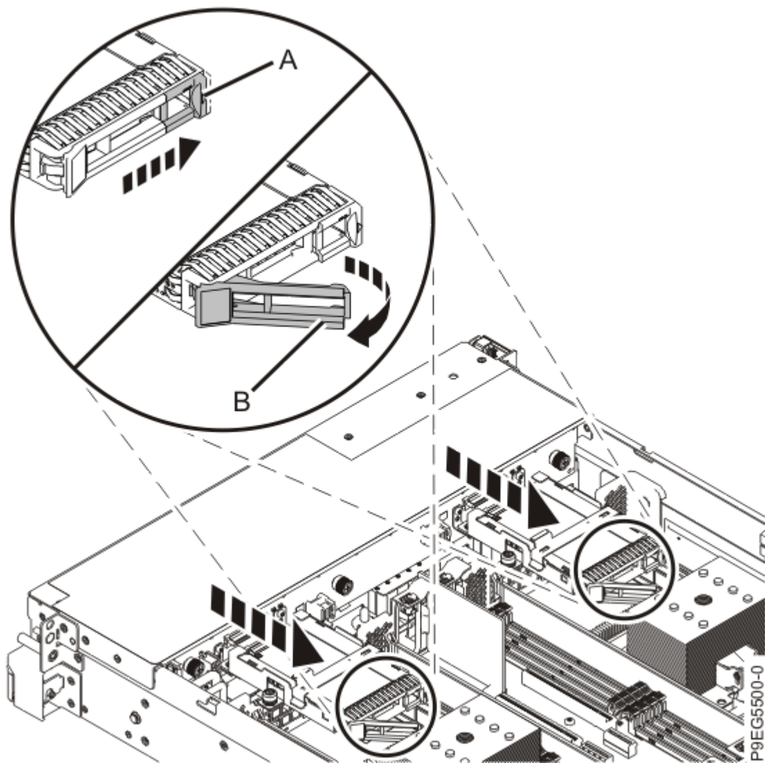
Abbildung 54. Laufwerk entriegeln
