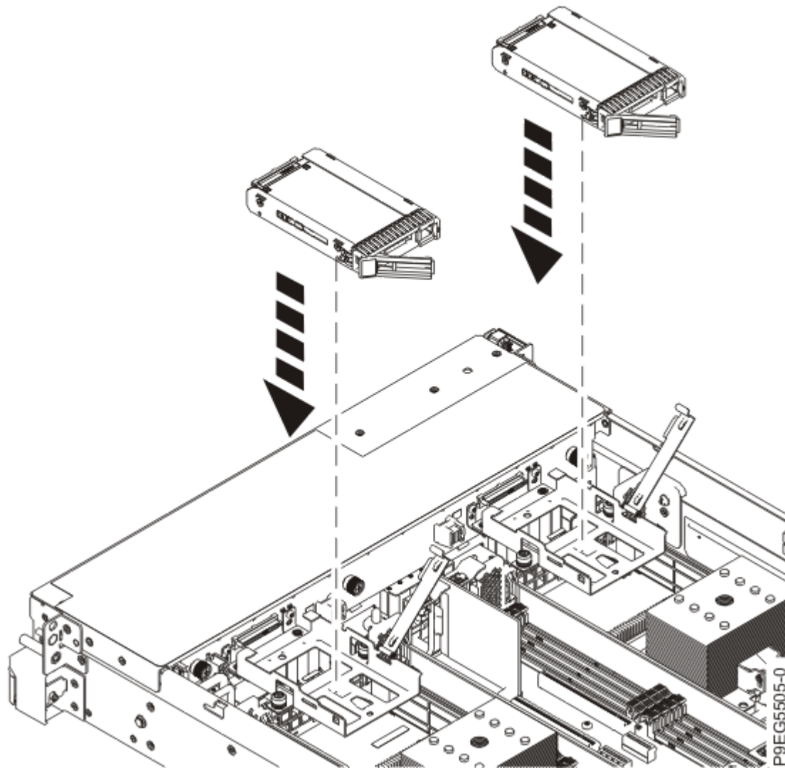
Abbildung 13. Laufwerk in Laufwerkhalterung absenken
