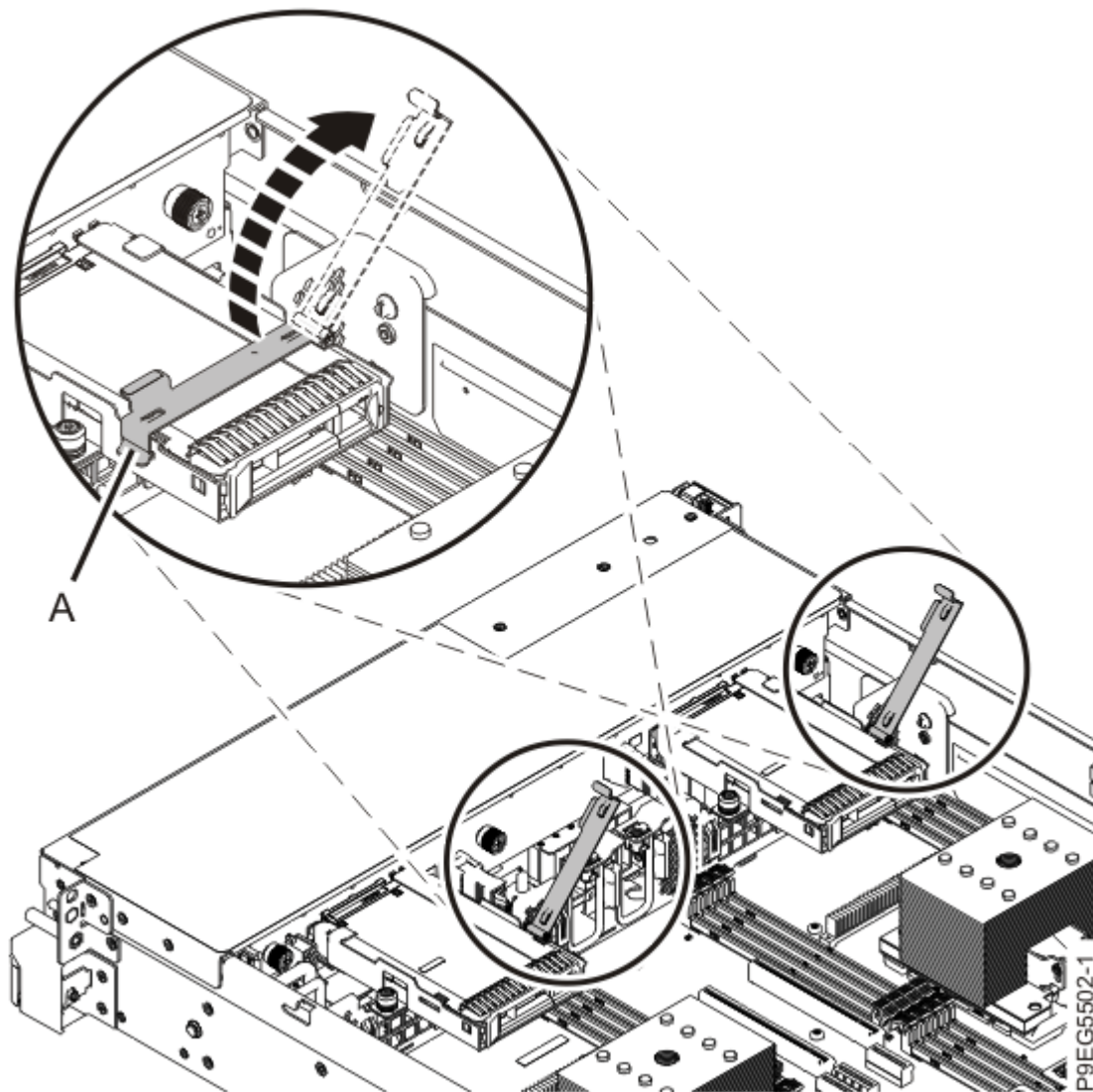
Abbildung 43. Laufwerkhalterhebel öffnen
