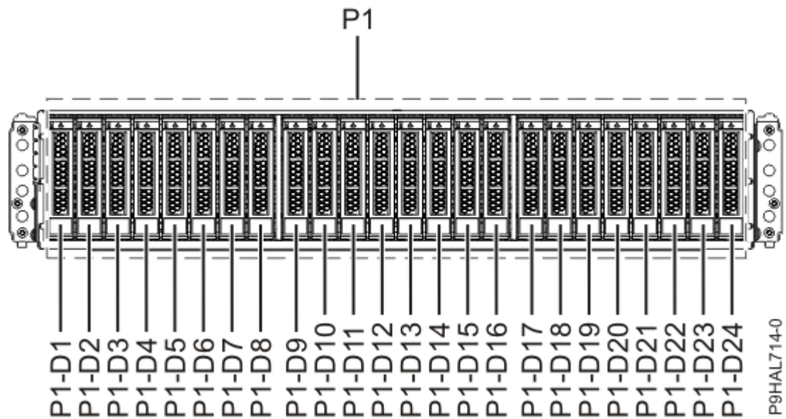
Abbildung 9. Vorderansicht des Systems 5887 Plattenlaufwerkgehäuse mit den Positionen der Plattenlaufwerke
