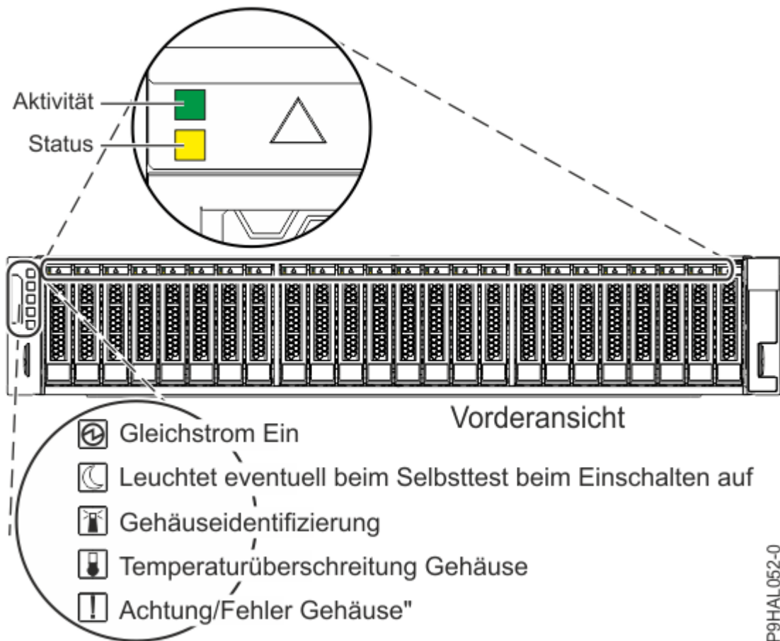
Abbildung 3. Vorderansicht des Systems 5887 Plattenlaufwerkgehäuse mit den Serviceanzeigen
