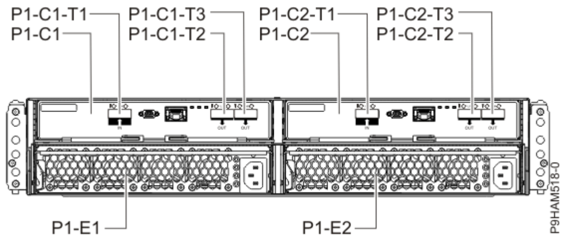
Abbildung 10. Rückansicht des Systems 5887 Plattenlaufwerkgehäuse
