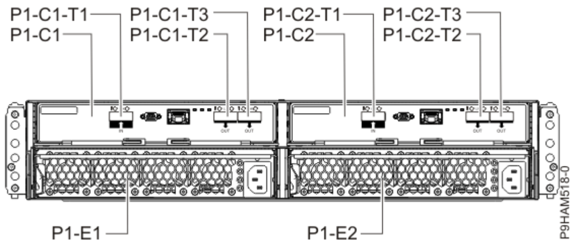
Abbildung 2. Rückansicht des Systems 5887 Plattenlaufwerkgehäuse
