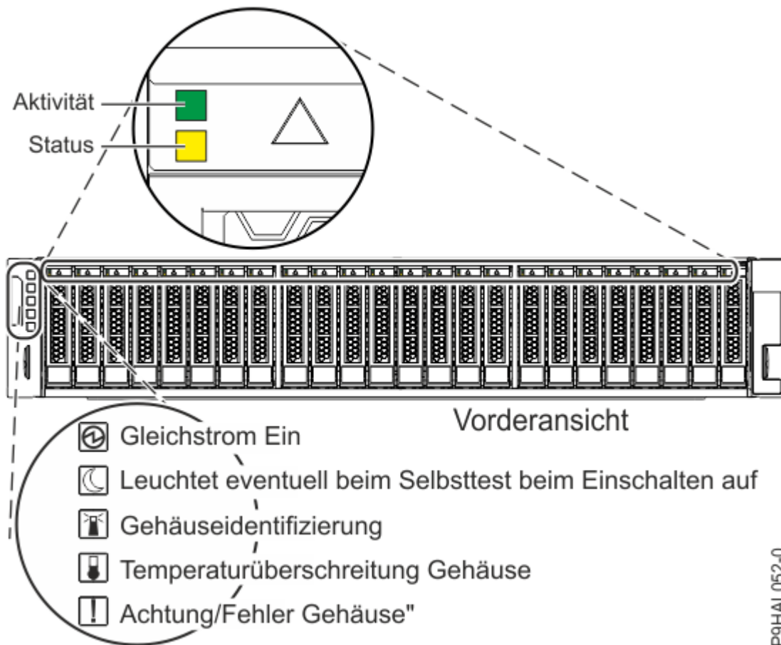
Abbildung 11. Vorderansicht des Systems 5887 Plattenlaufwerkgehäuse mit den Serviceanzeigen
