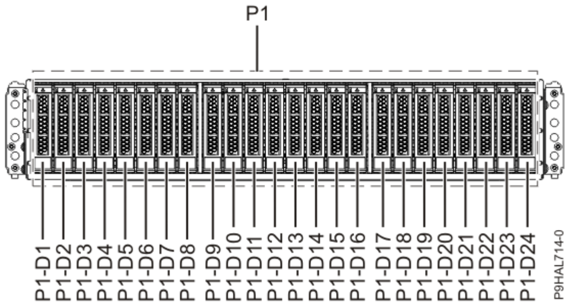
Abbildung 1. Vorderansicht des Systems 5887 Plattenlaufwerkgehäuse mit den Positionen der Plattenlaufwerke
