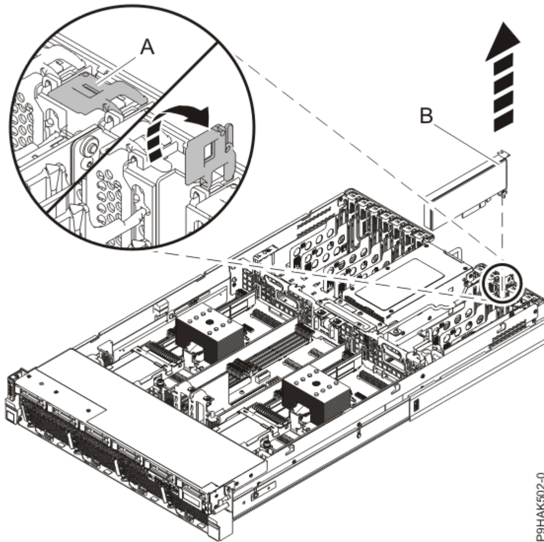
Abbildung 38. Adapter aus dem System vom Typ 5105-22E, 9008-22L, 9009-22A, 9009-22G, 9223-22H oder 9223-22S entfernen
