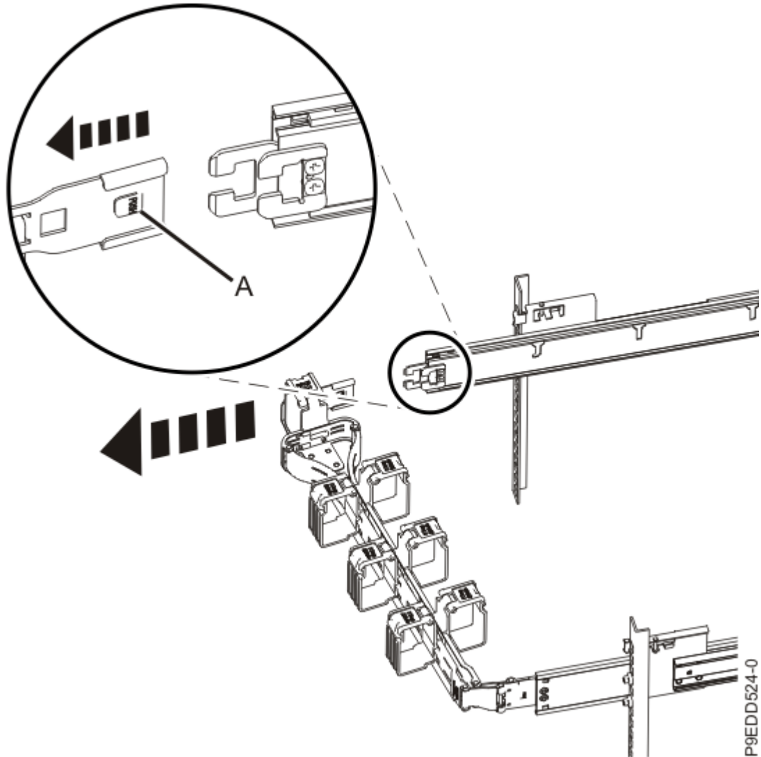
Abbildung 19. Entriegeln der Halterung
