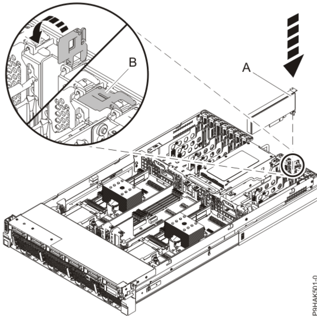
Abbildung 11. Adapter in einem System vom Typ 5105-22E, 9008-22L, 9009-22A, 9009-22G, 9223-22H oder 9223-22S installieren oder austauschen
