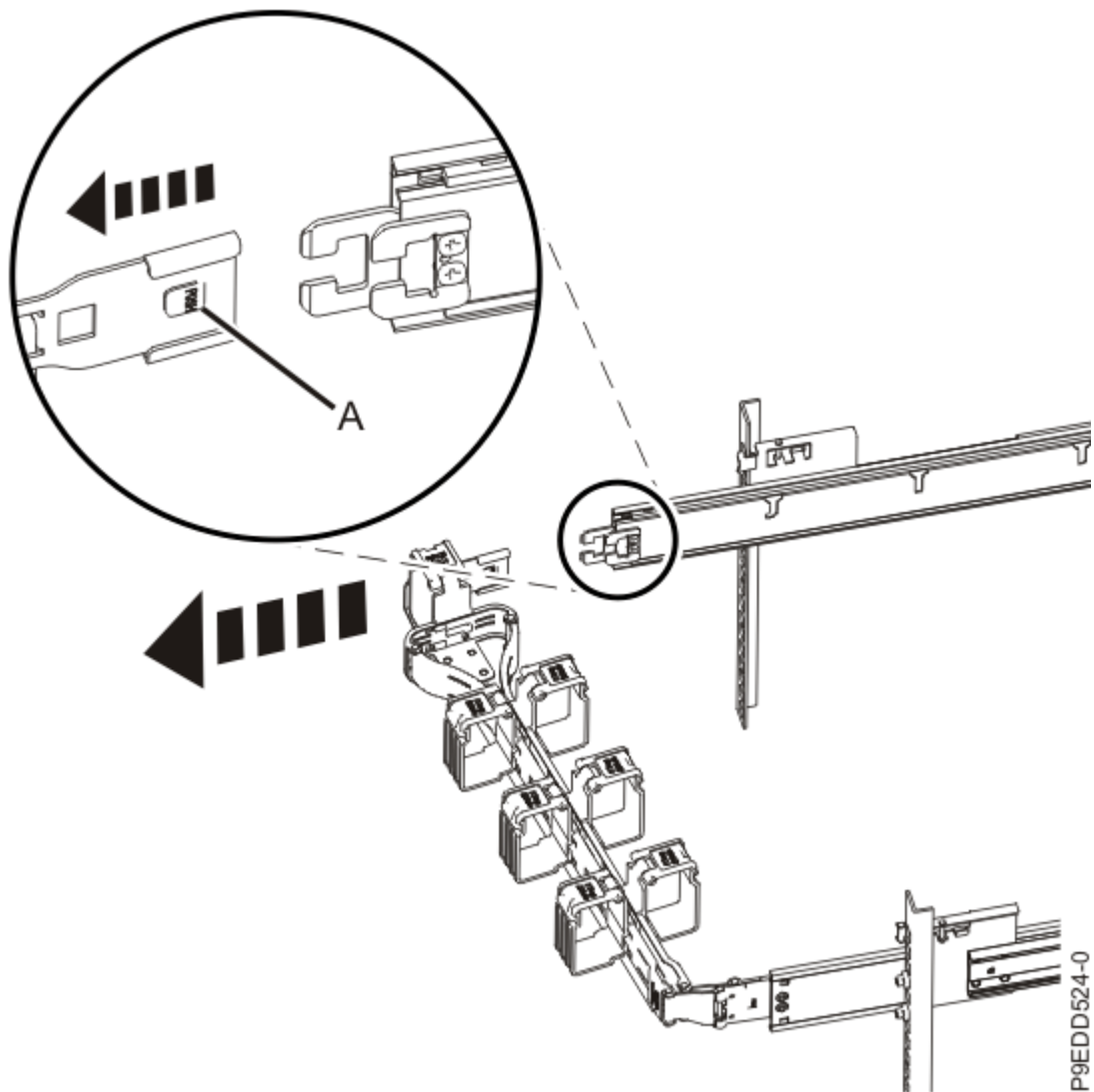
Abbildung 4. Entriegeln der Halterung
