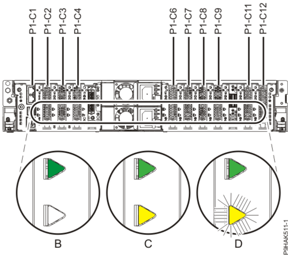
Abbildung 32. Positionen der Adaptersteckplätze und Anzeigen in einem System vom Typ 5105-22E, 9008-22L, 9009-22A, 9009-22G, 9223-22H oder 9223-22S
