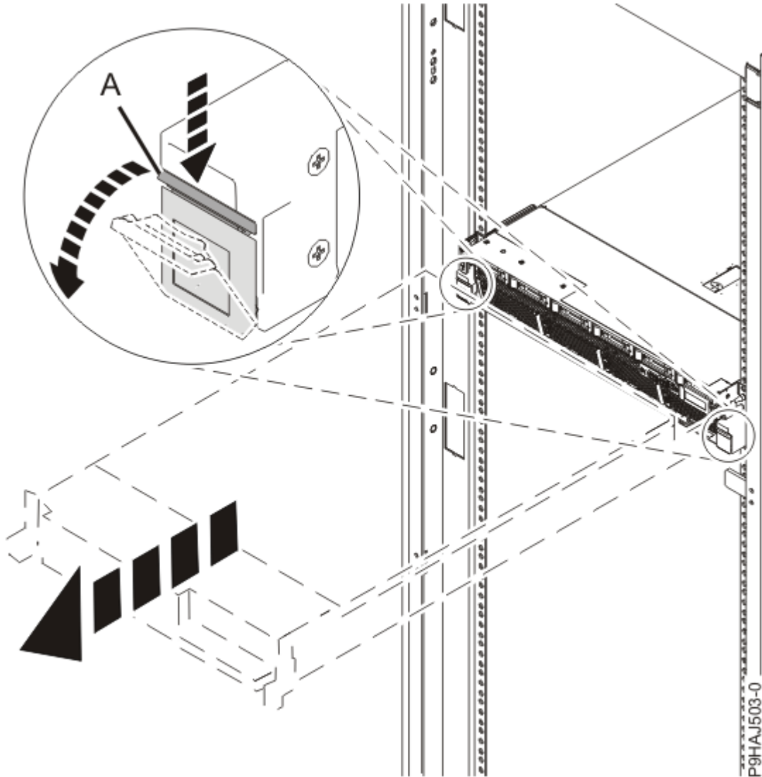
Abbildung 23. Seitliche Verriegelungen entriegeln
