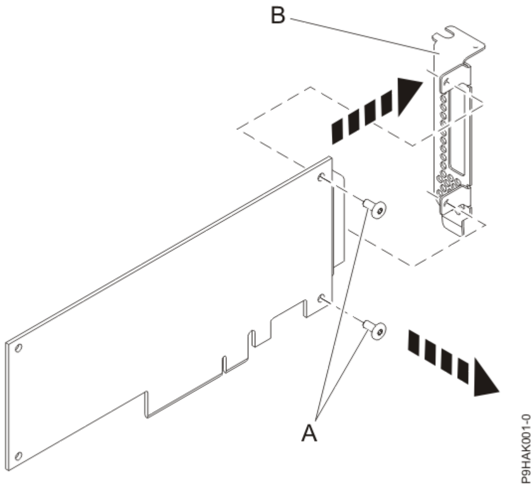
Abbildung 45. Kurzen Haltesteg aus einem Adapter ausbauen
