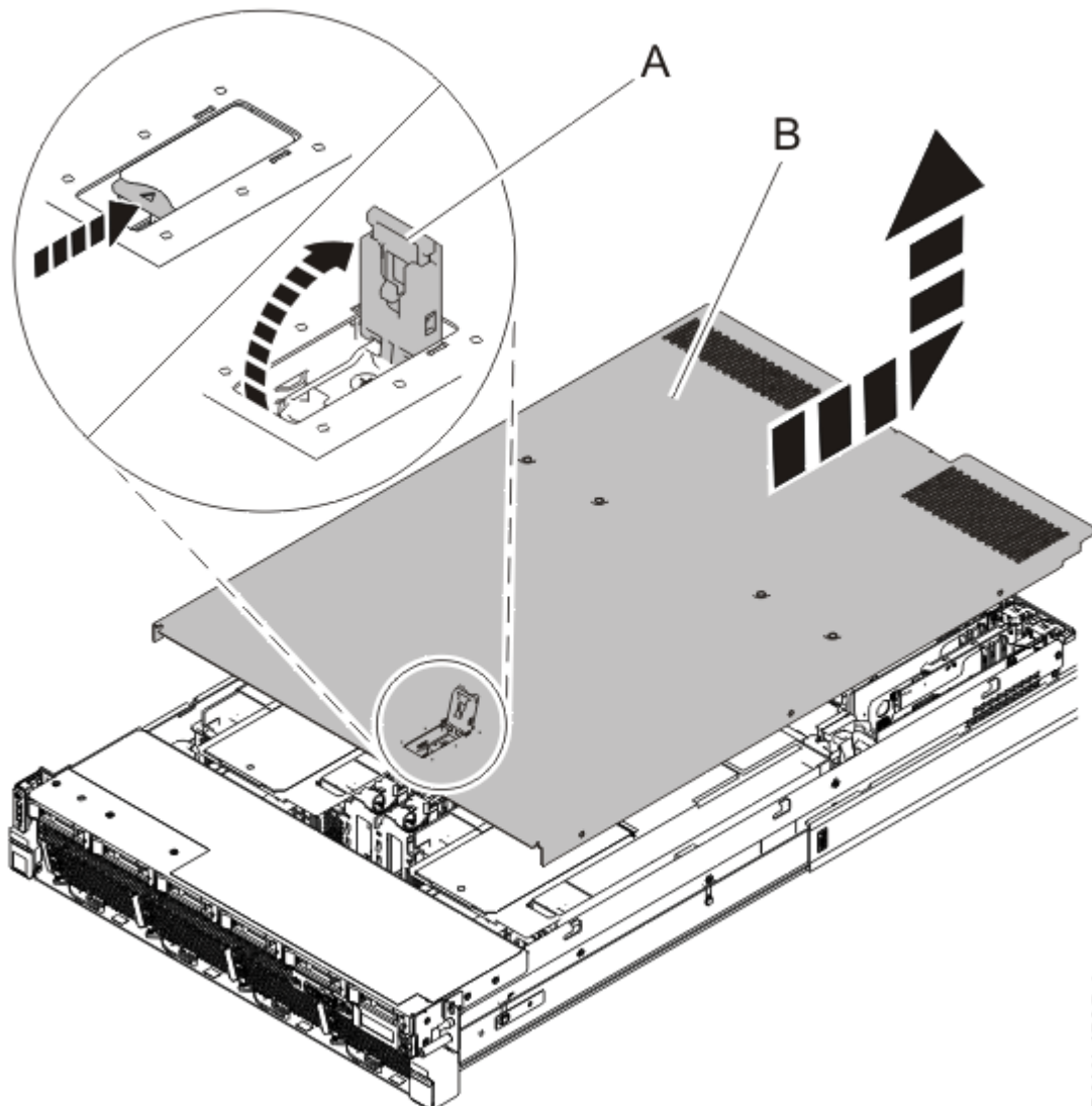
Abbildung 37. Serviceabdeckung ausbauen
