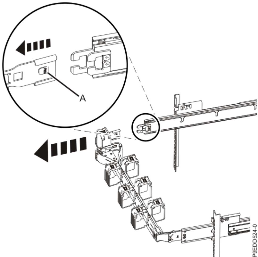
Abbildung 5. Entriegeln der Halterung
