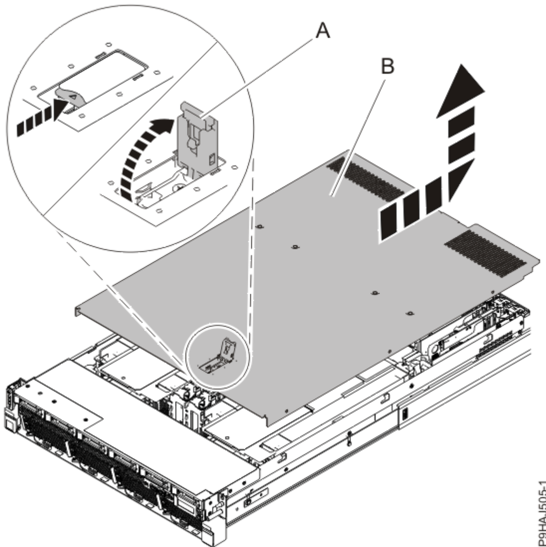
Abbildung 10. Serviceabdeckung ausbauen
