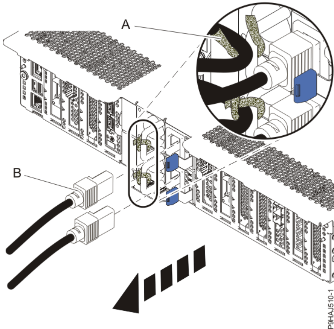
Abbildung 34. Netzkabel abziehen
