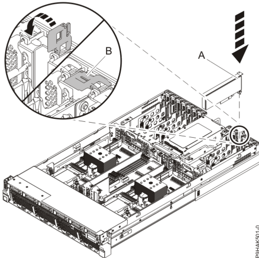
Abbildung 26. Adapter in einem System vom Typ 5105-22E, 9008-22L, 9009-22A, 9009-22G, 9223-22H oder 9223-22S installieren oder austauschen
