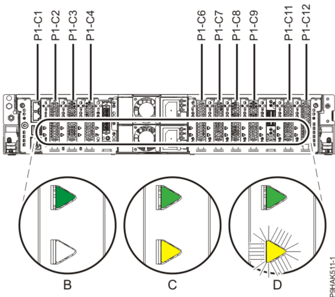
Abbildung 16. Positionen der Adaptersteckplätze und Anzeigen in einem System vom Typ 5105-22E, 9008-22L, 9009-22A, 9009-22G, 9223-22H oder 9223-22S
