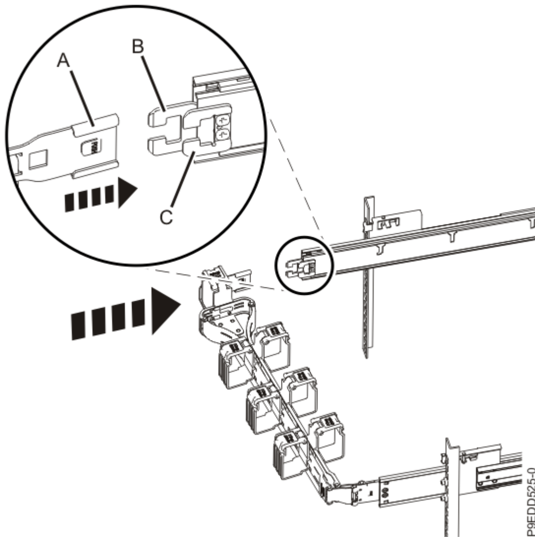
Abbildung 31. Schließen des Kabelträgers
