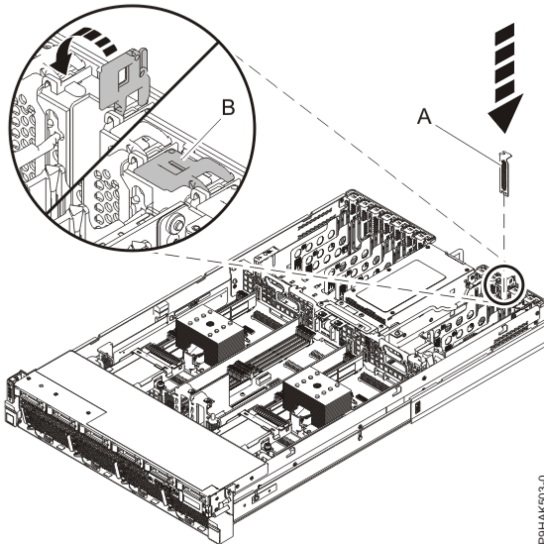
Abbildung 39. Platzhalterelement in einem Steckplatz in einem System vom Typ 5105-22E, 9008-22L, 9009-22A, 9009-22G, 9223-22H oder 9223-22S installieren
