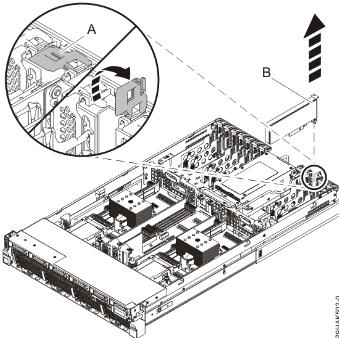
Abbildung 25. Adapter aus dem System vom Typ 5105-22E, 9008-22L, 9009-22A, 9009-22G, 9223-22H oder 9223-22S entfernen
