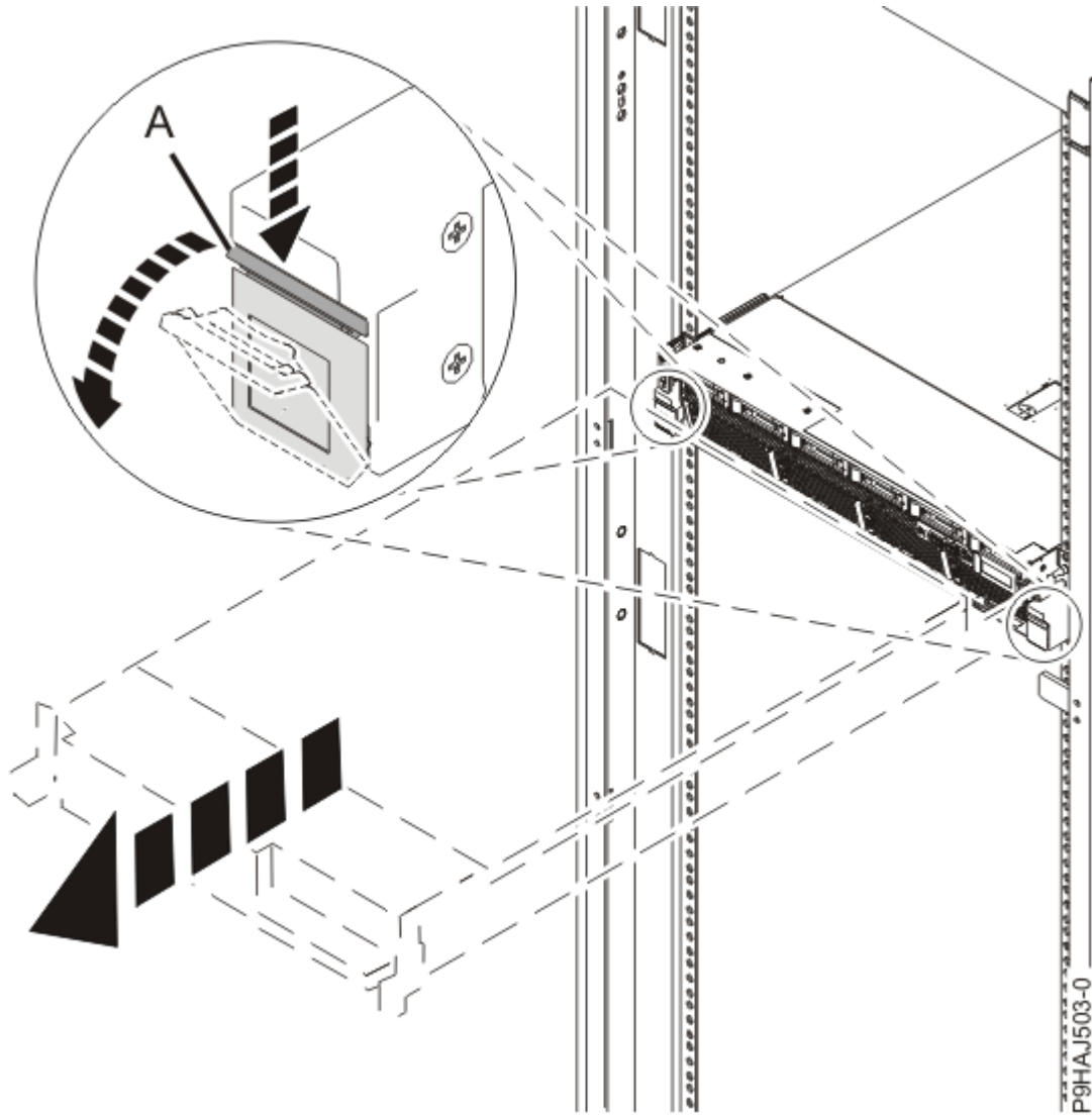
Abbildung 9. Seitliche Verriegelungen entriegeln
