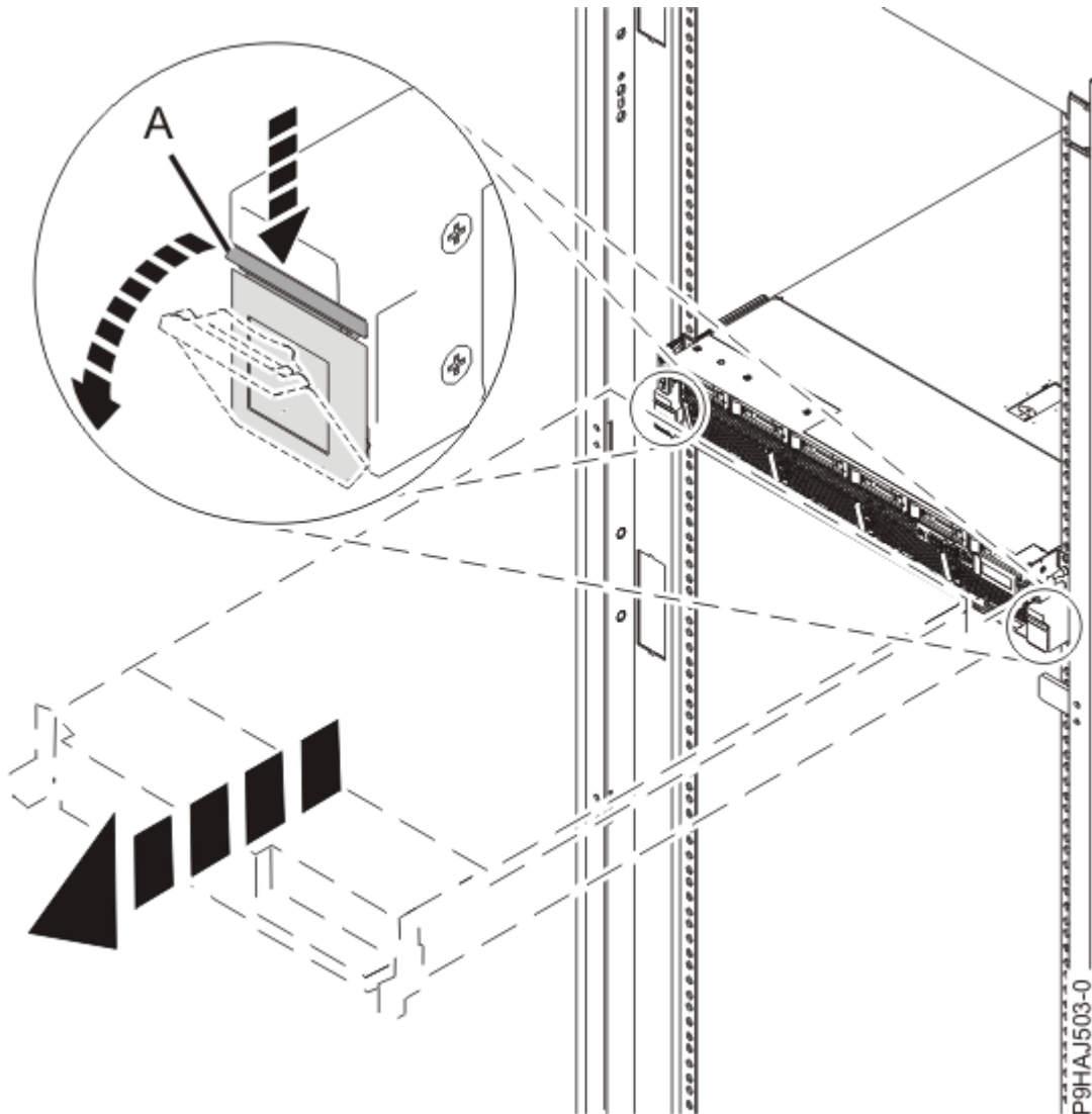
Abbildung 8. Seitliche Verriegelungen entriegeln
