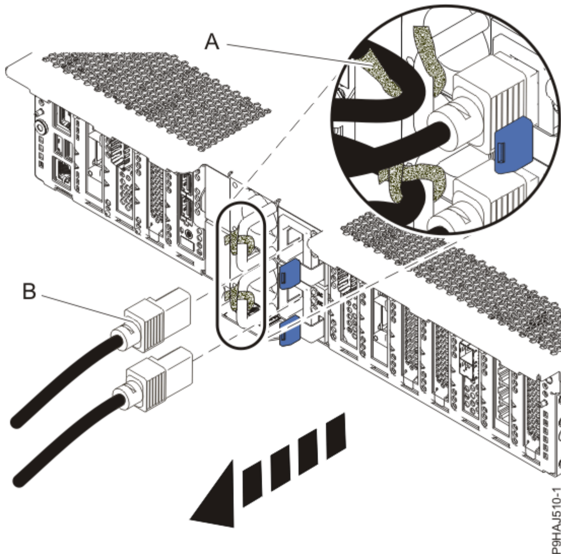
Abbildung 18. Netzkabel abziehen
