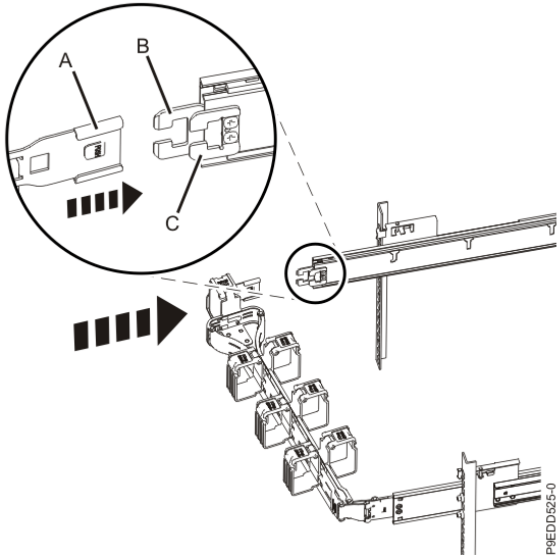
Abbildung 7. Schließen des Kabelträgers
