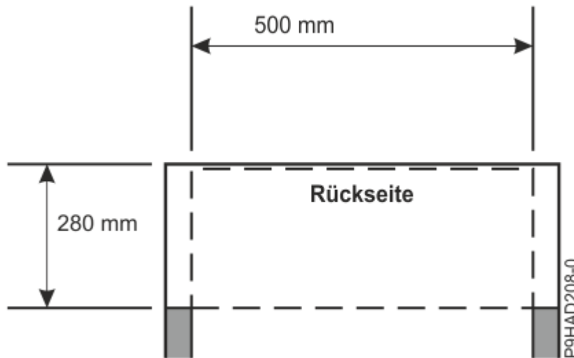
Abbildung 36. Zugänge an der Rackrückseite der Modelle 9080-M9S (enger Bereich für Installation der Rackhalterung)
