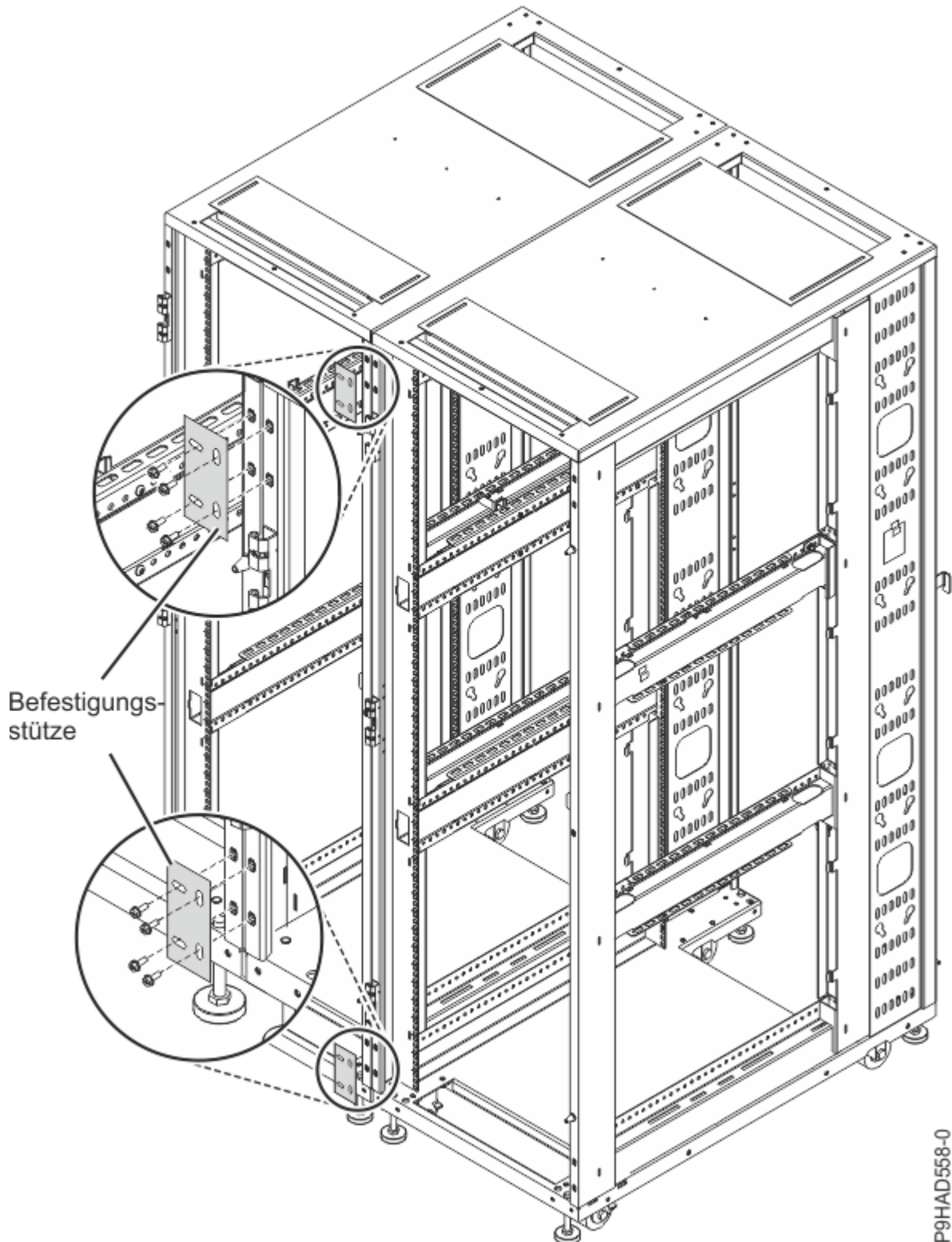
Abbildung 12. Befestigungsstützen
