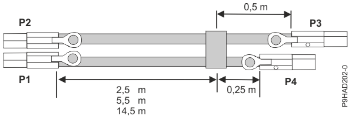
Abbildung 47. Kabellängen des externen SAS-YO-Kabelsatzes
