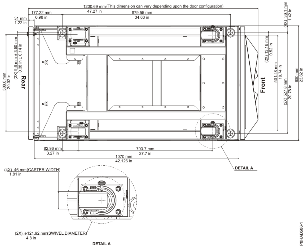
Abbildung 14. Positionen der Rollen und Nivellierfüße
