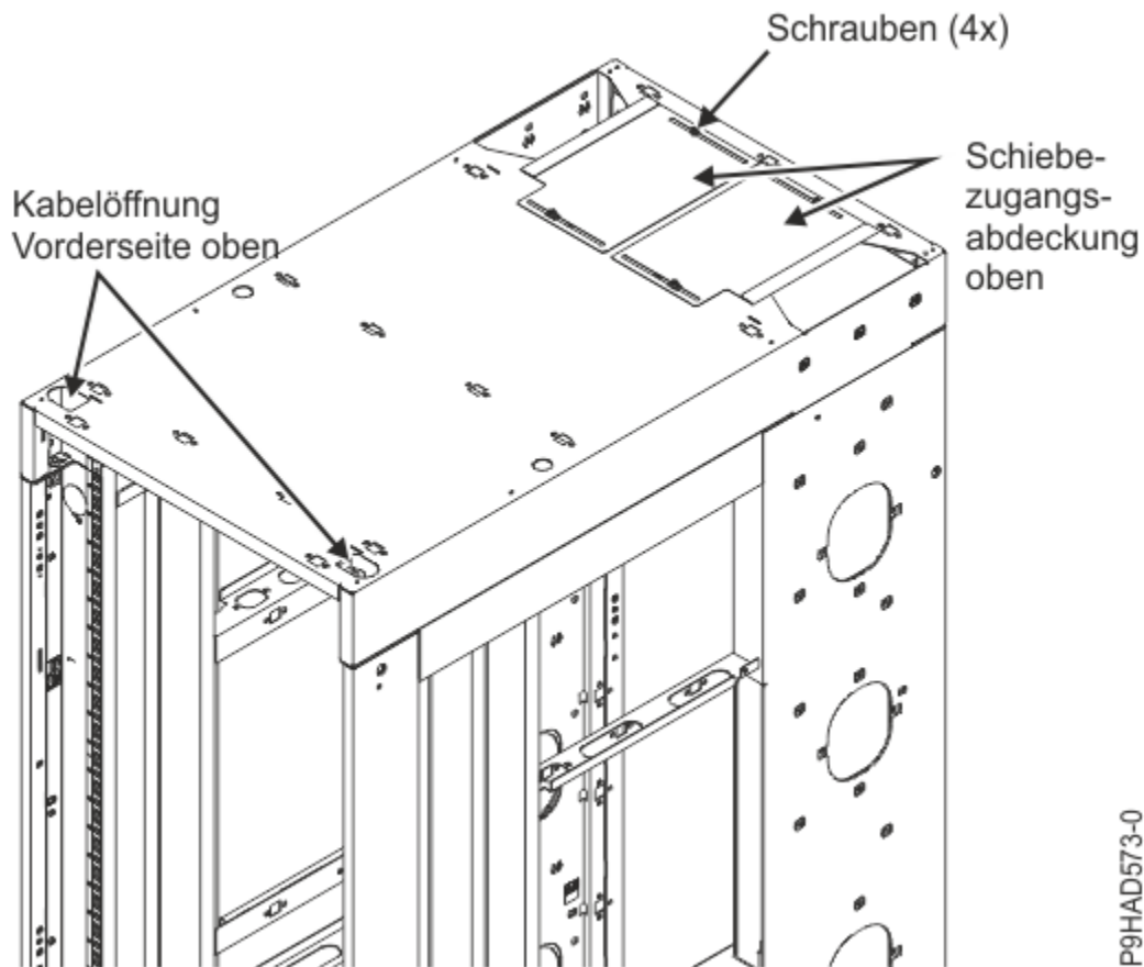
Abbildung 17. Oberseitige Verkabelung
