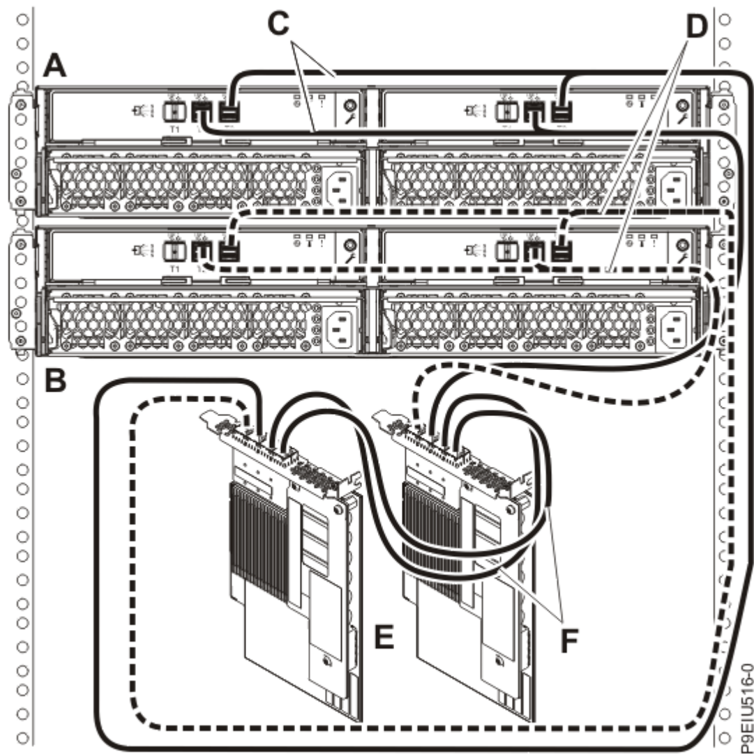
Abbildung 65. Modus 1-Anschluss von zwei ESLL- oder ESLS-Speichereinheiten mit YO12-Kabeln an ein Paar von SAS-Adaptern
