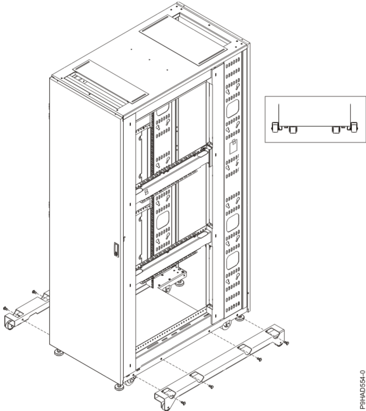
Abbildung 11. Outriggerpositionen
