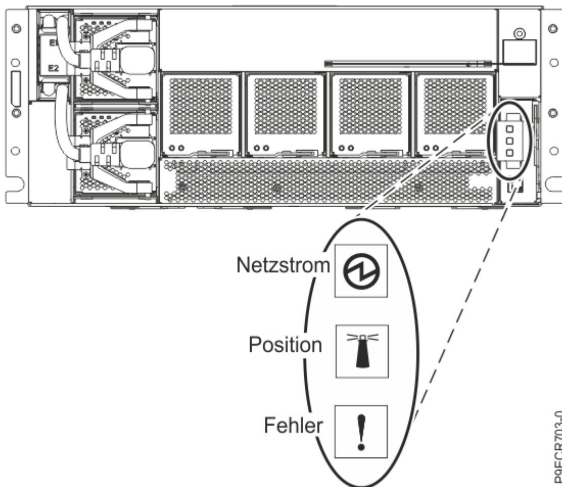
Abbildung 7. Vordere Betriebs-LED für den Einschub für EMX0-PCIe3-Erweiterungen
