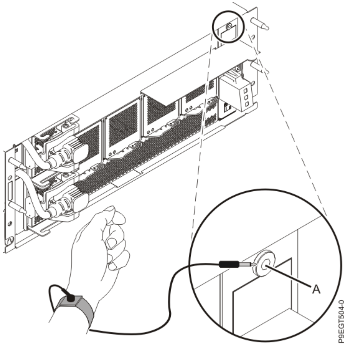
Abbildung 2. Antistatikarmband an die vordere ESD-Buchse anschließen
