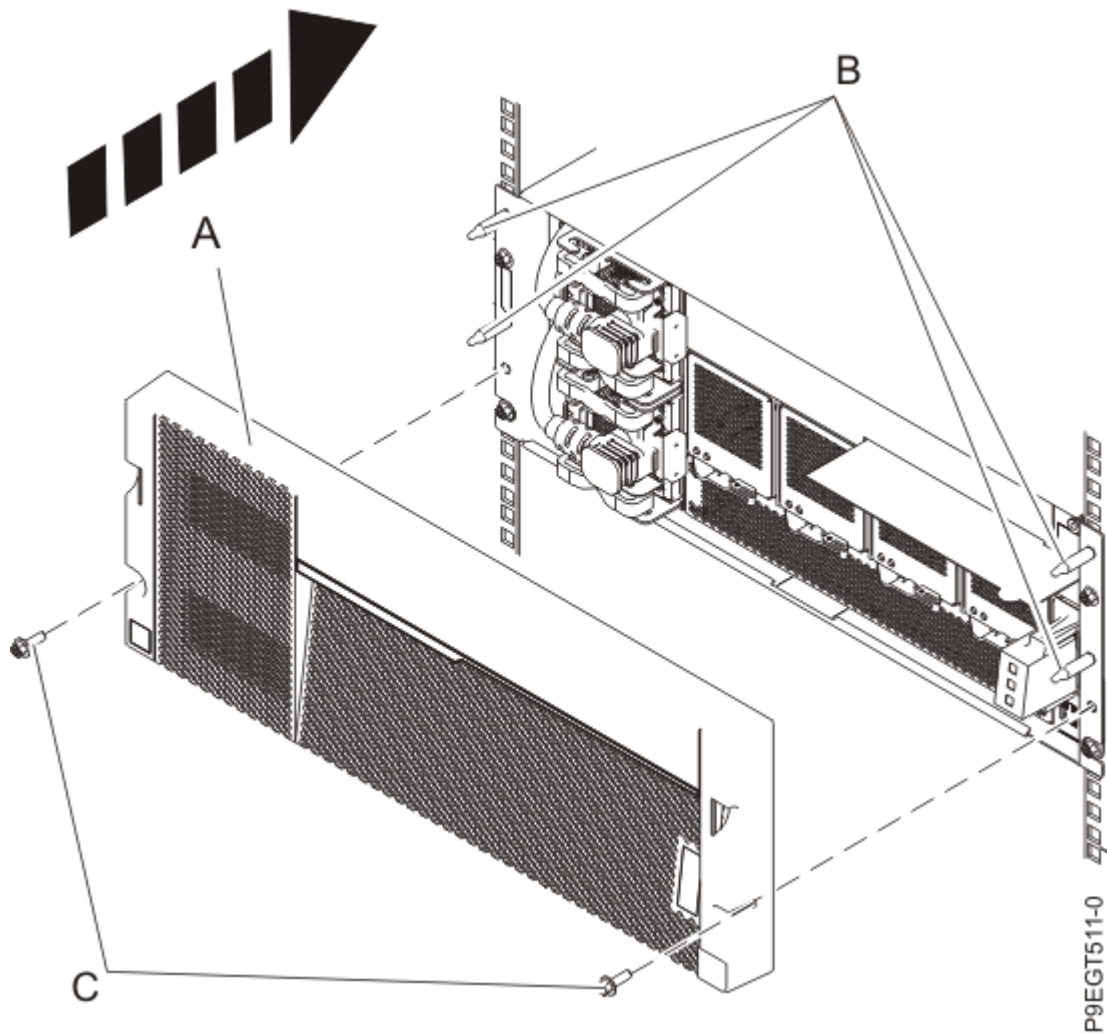
Abbildung 8. Vordere Abdeckung austauschen
