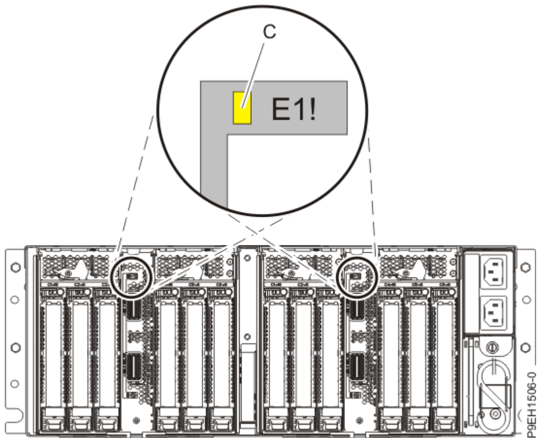
Abbildung 3. Spannungsreglermodul-LED
