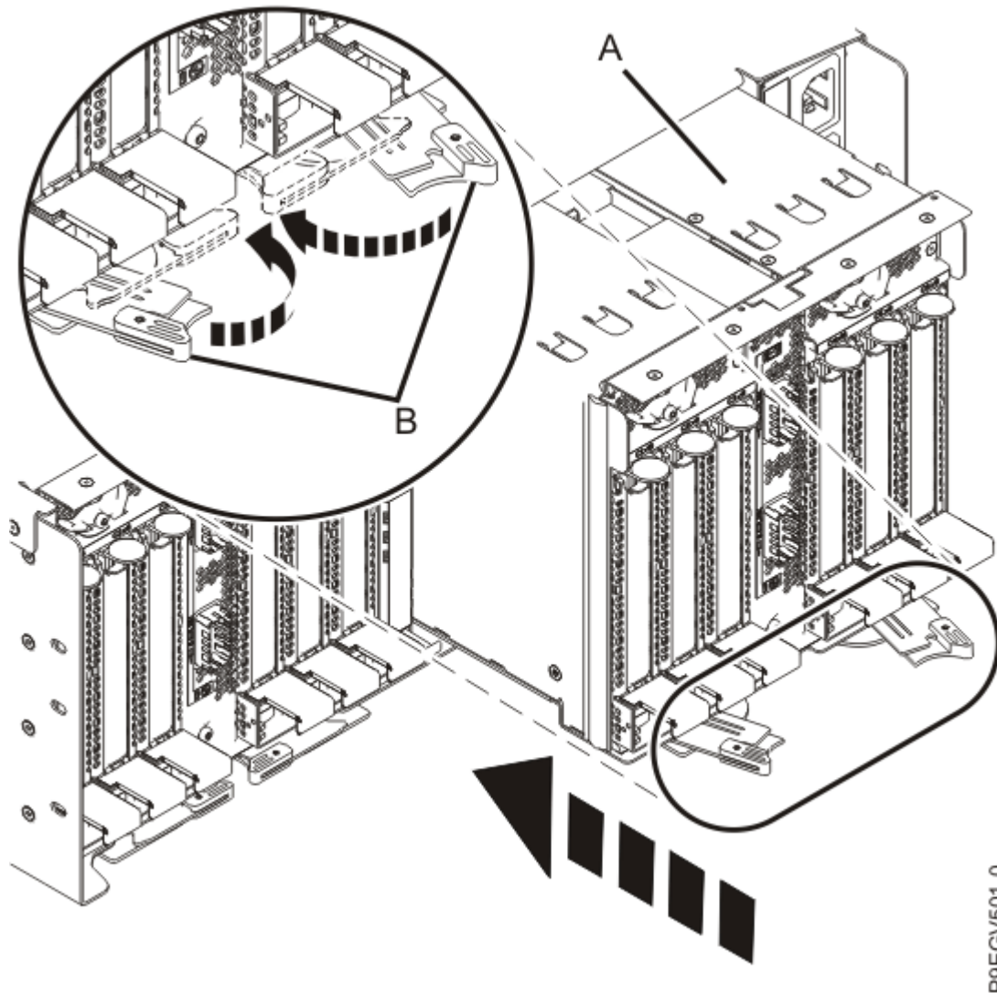
Abbildung 7. Entriegelungshebel schließen
