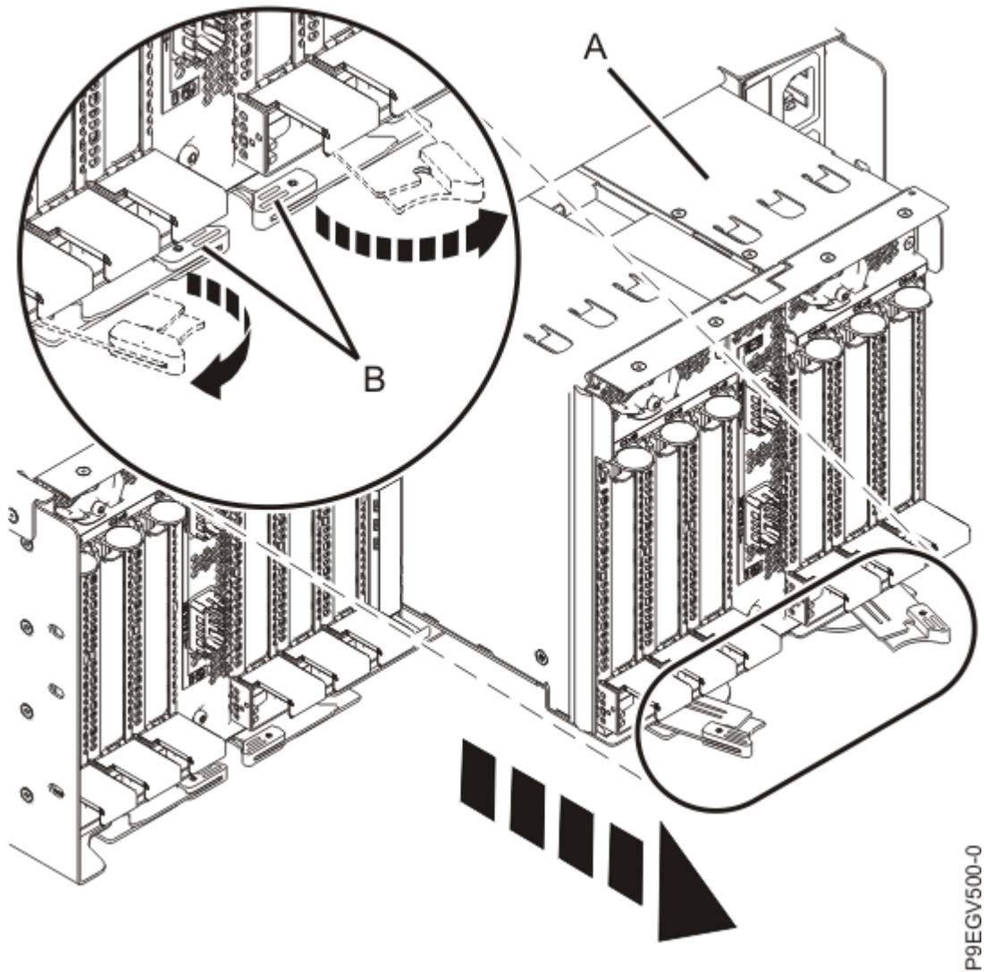
Abbildung 4. Entriegelungshebel öffnen
