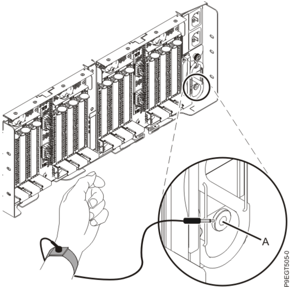
Abbildung 1. Position der ESD-Buchse an der Rückseite am Einschub für EMX0-PCIe3-Erweiterungen
