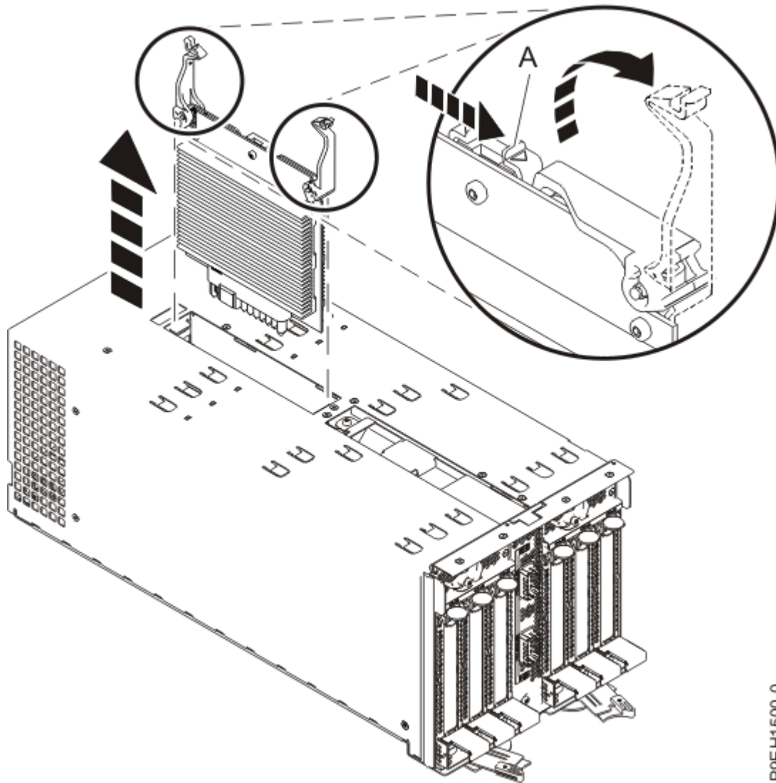
Abbildung 5. Spannungsreglermodul ausbauen
