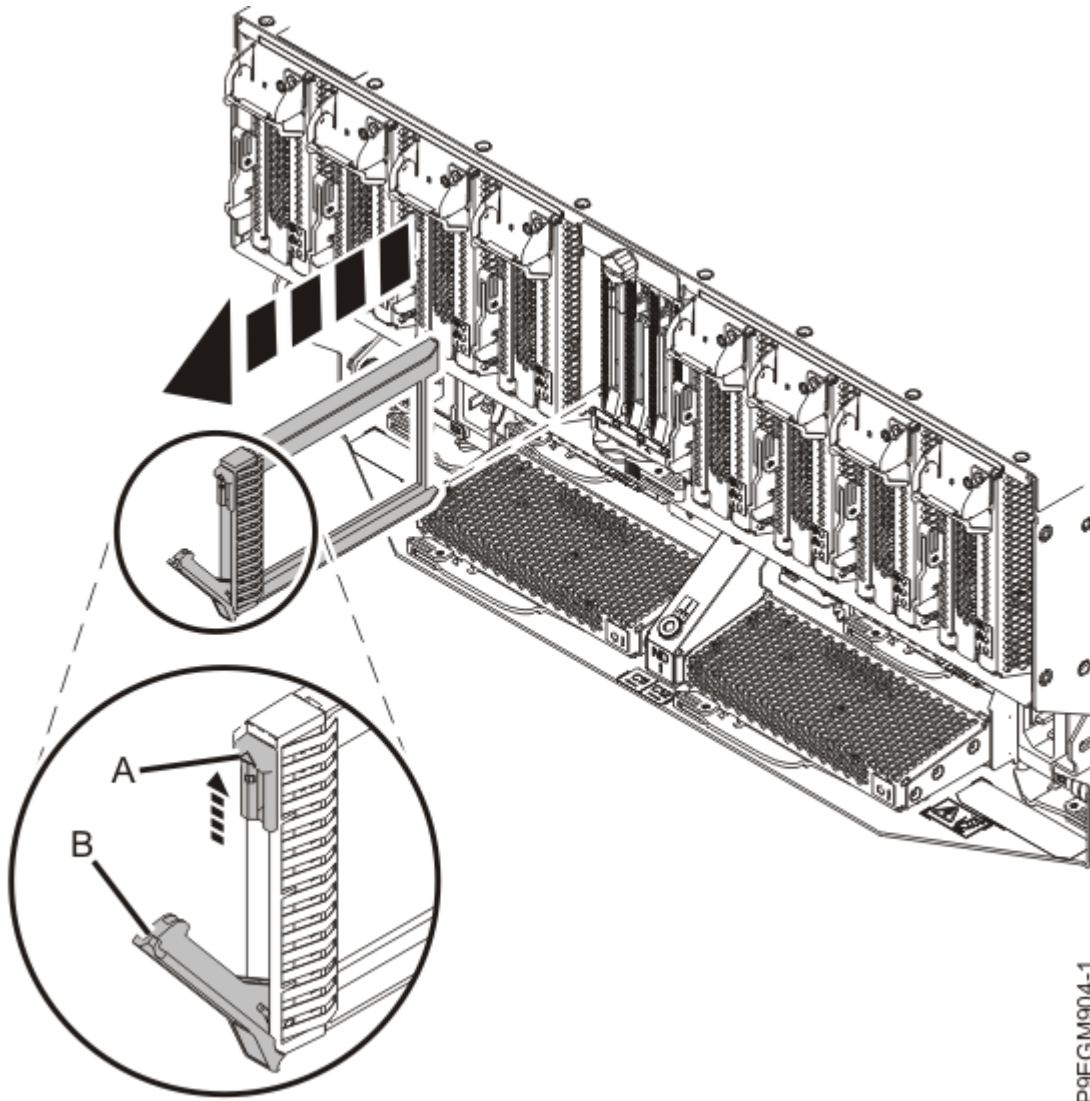
Abbildung 6. NVMe-Laufwerkabdeckblende aus dem System vom Typ 9080-M9S entfernen
