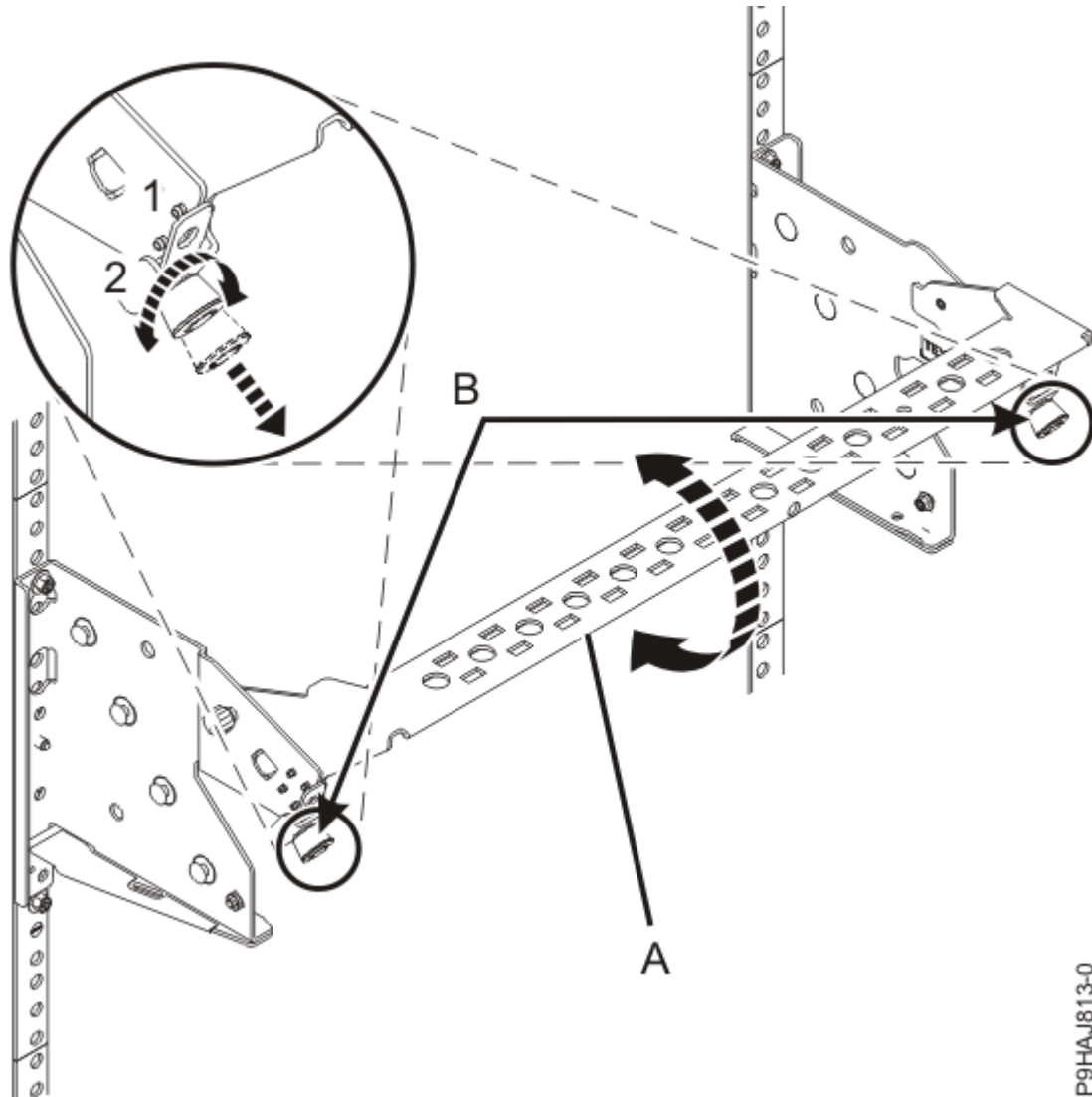
Abbildung 8. Kabelführungshalterung in die abgesenkte Betriebsposition bringen
