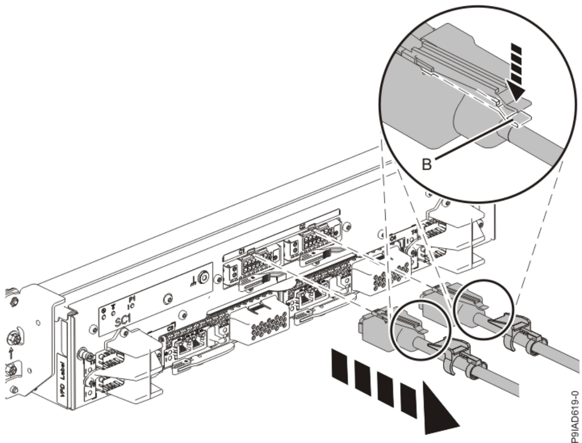
Abbildung 4. UPIC-Kabel aus dem Systemcontroller entfernen
