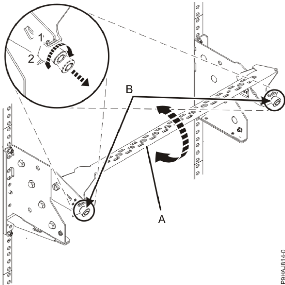
Abbildung 5. Kabelführungshalterung in die erhöhte Serviceposition bringen
