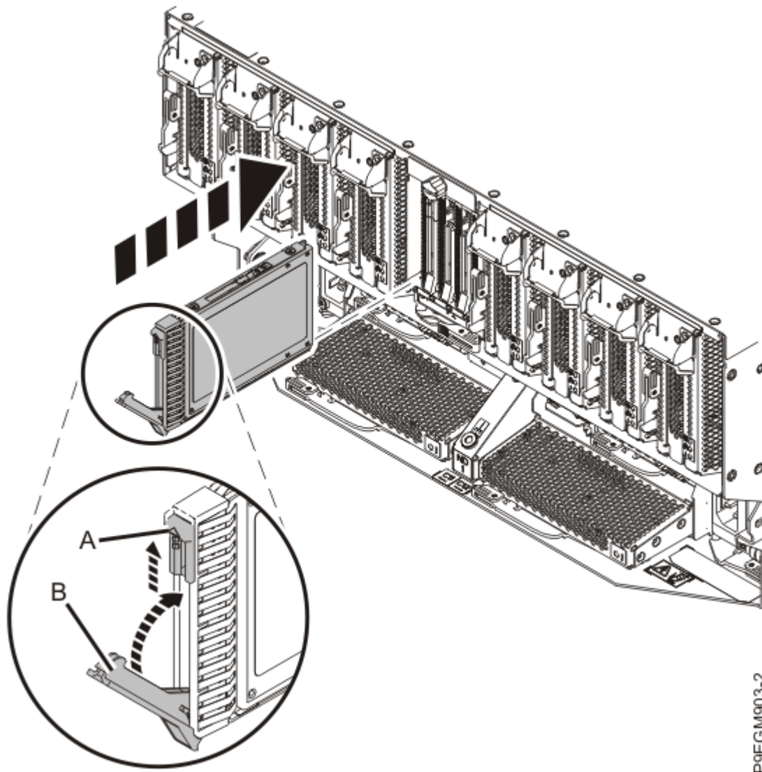
Abbildung 7. NVMe U.2-Laufwerk beim System vom Typ 9080-M9S installieren oder austauschen c) Schließen Sie den Griff für das Laufwerk (B) , damit das NVMe U.2-Laufwerk einrastet.
