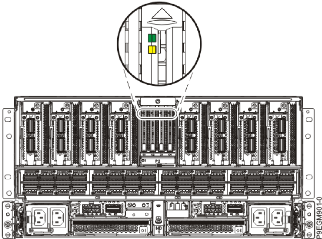
Abbildung 2. Positionen der LEDs am NVMe U.2-Laufwerk beim System vom Typ 9080-M9S
