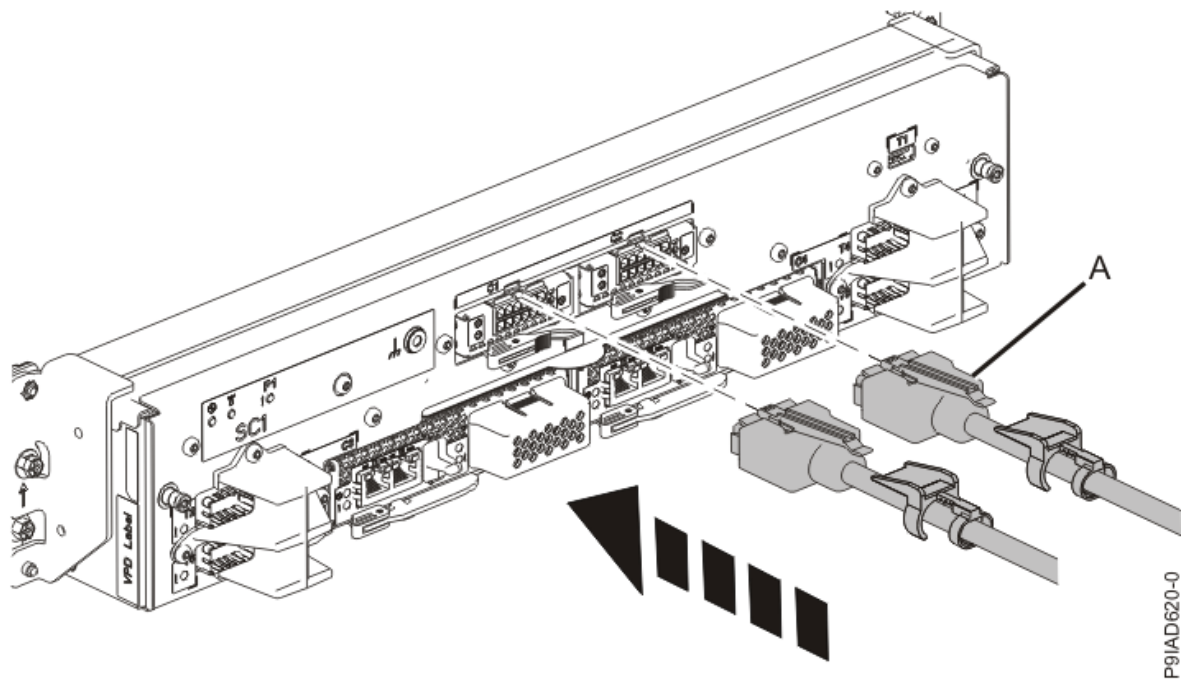
Abbildung 9. UPIC-Kabel am Systemcontroller wieder anschließen
