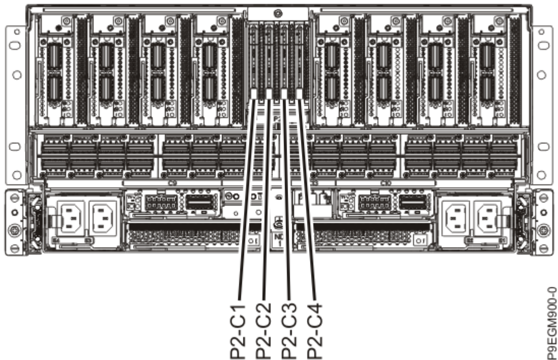
Abbildung 1. Position der NVMe U.2-Laufwerke im System vom Typ 9080-M9S
