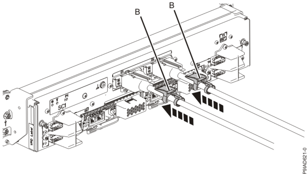
Abbildung 10. UPIC-Kabel am Systemcontroller wieder anschließen
