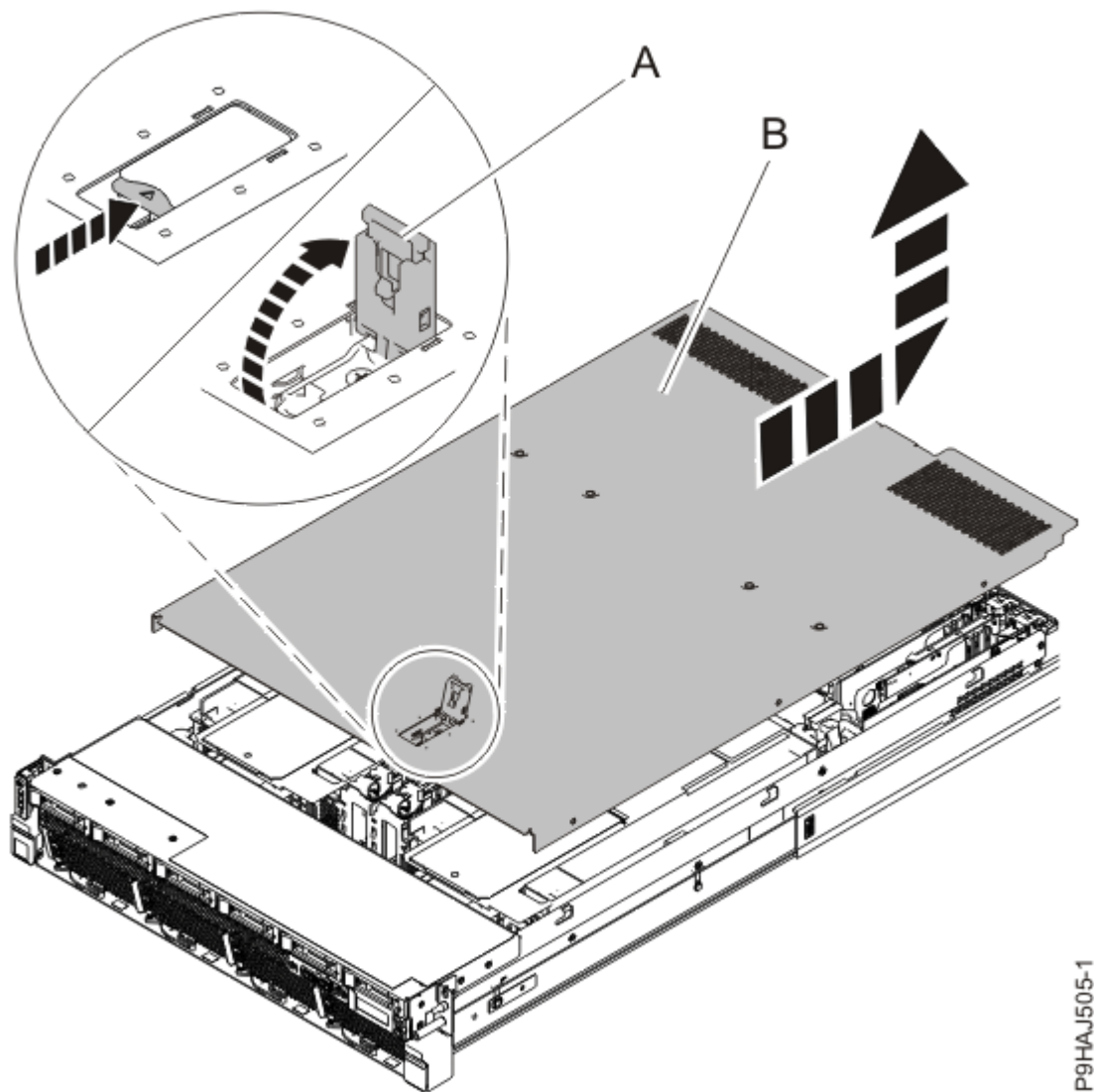
Abbildung 3. Serviceabdeckung ausbauen
