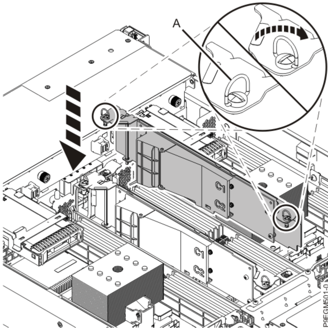
Abbildung 8. NVMe M.2-Trägerkarte einsetzen
