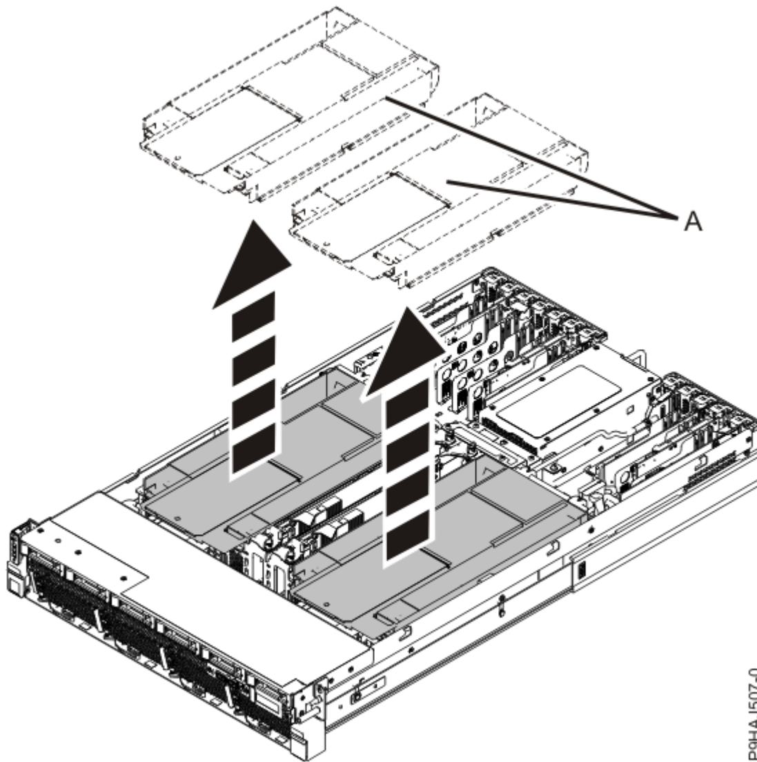
Abbildung 13. Luftführung ausbauen
