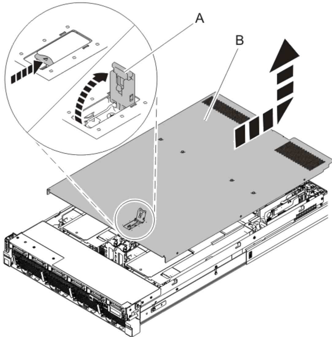
Abbildung 12. Serviceabdeckung ausbauen
