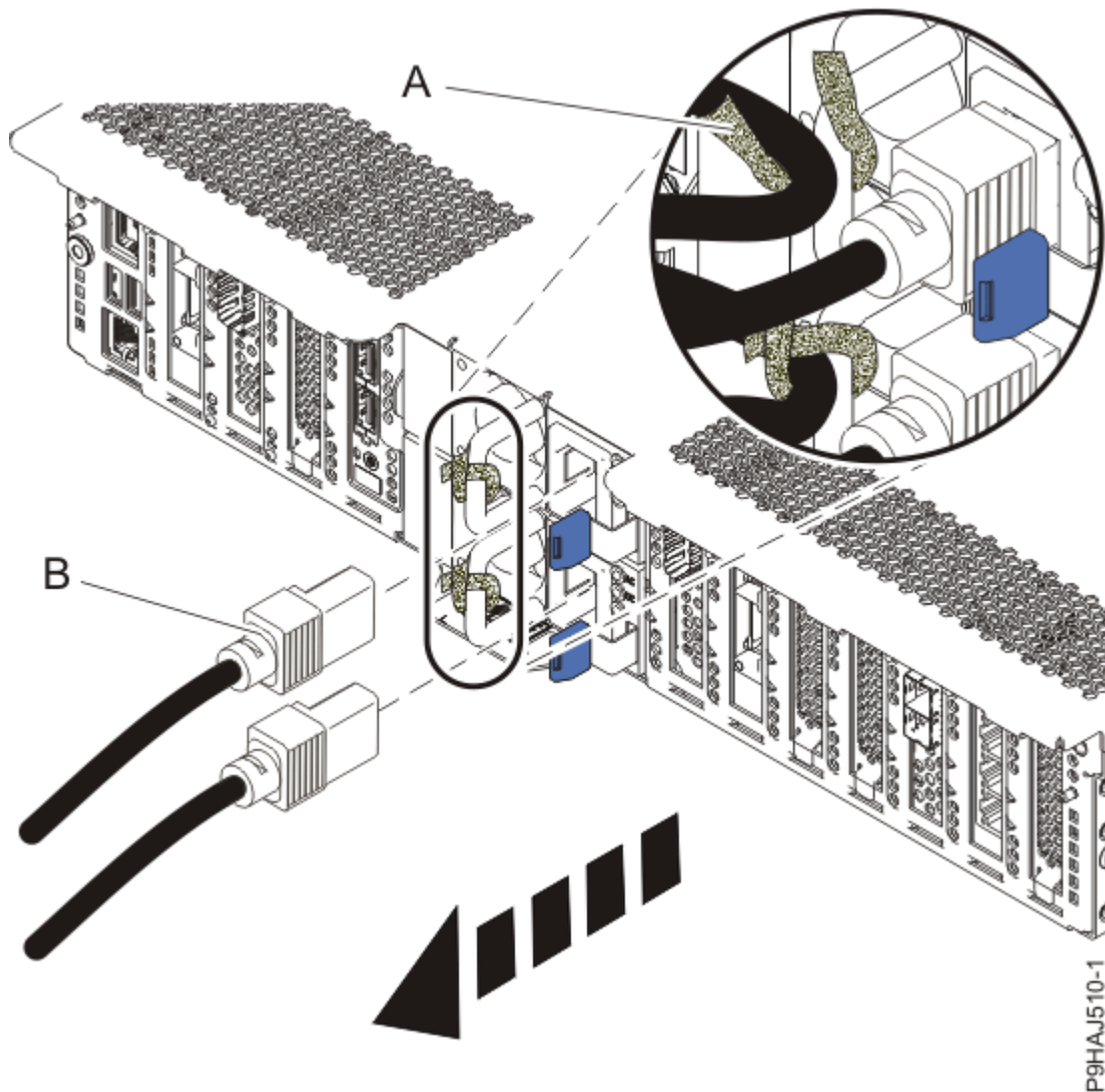
Abbildung 10. Netzkabel abziehen
