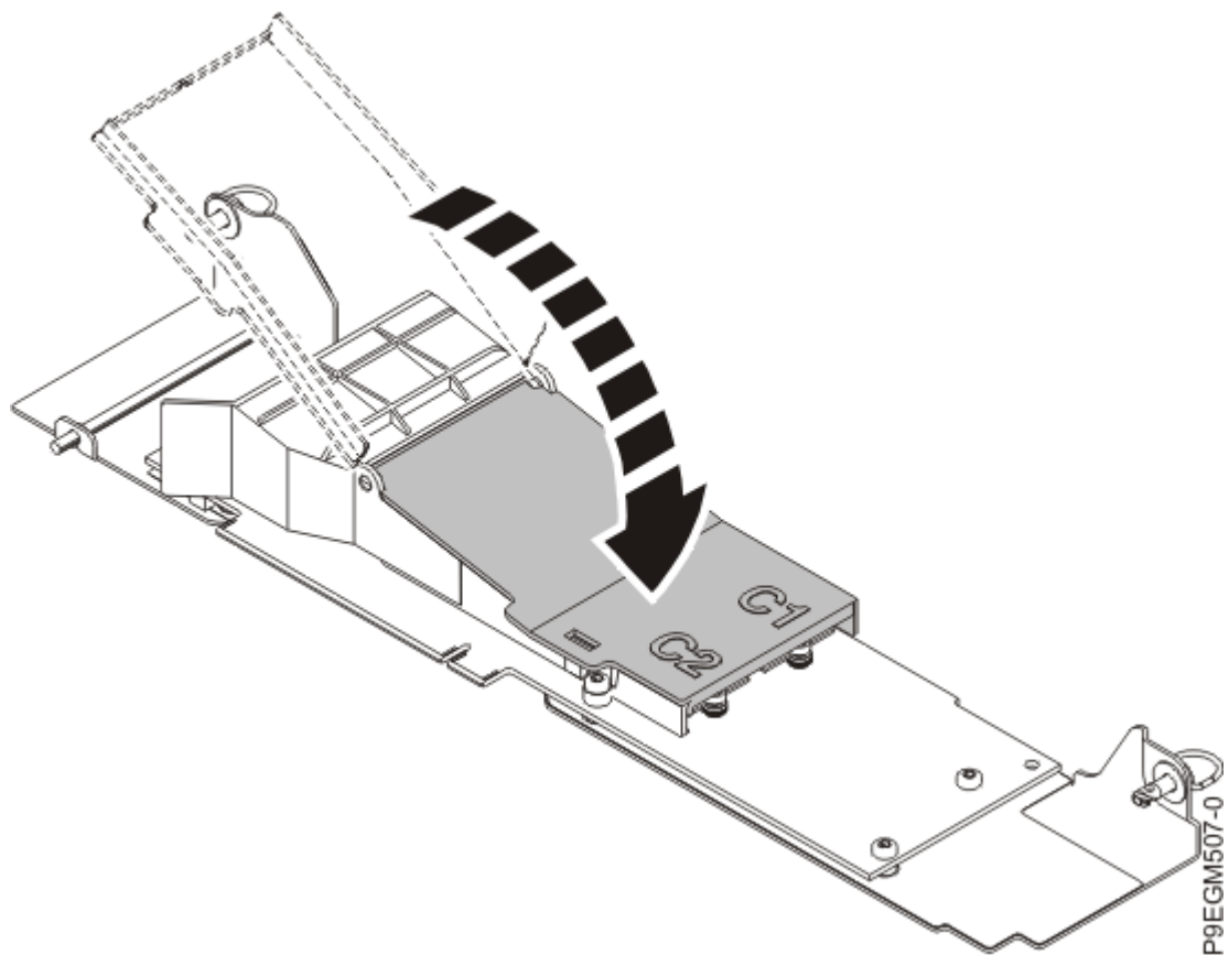
Abbildung 22. Schwarze Abdeckung der NVMe M.2-Trägerkarte schließen
